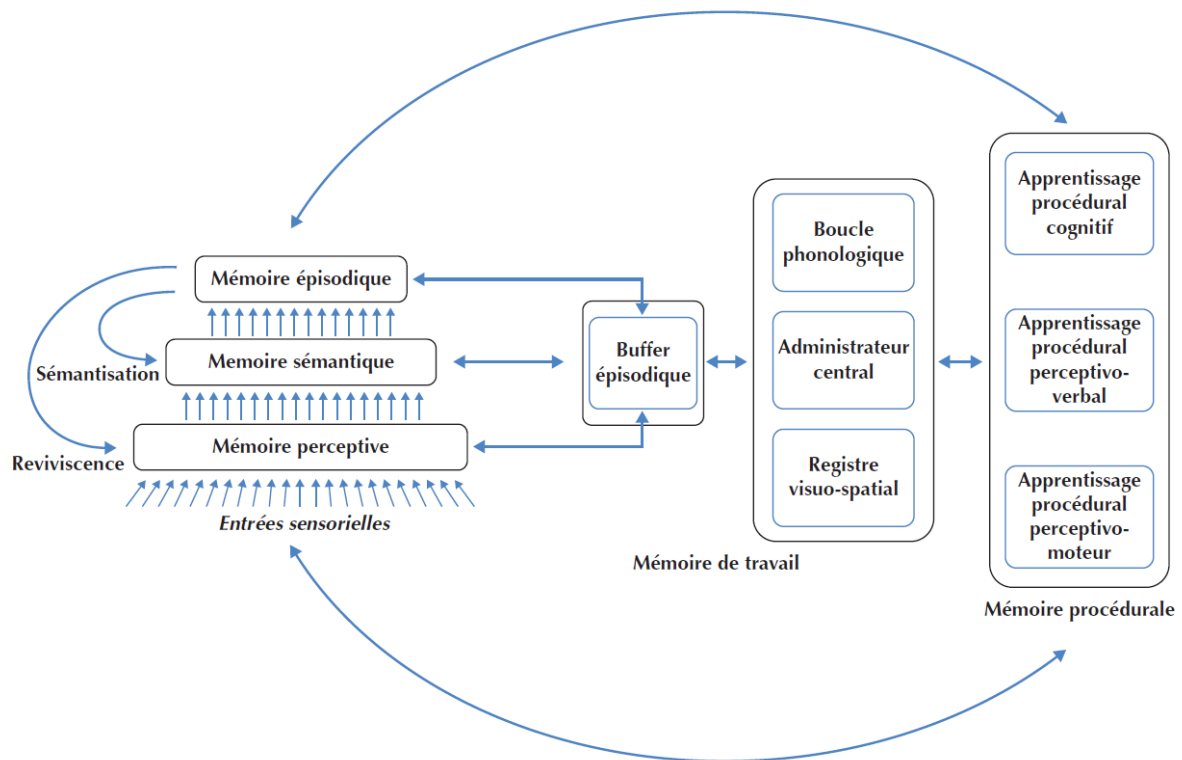
Figure 28. Modèle MNESIS.
