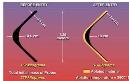
FIGURE 1.1 – Bouclier thermique de la sonde Galiléo. [LV03]
