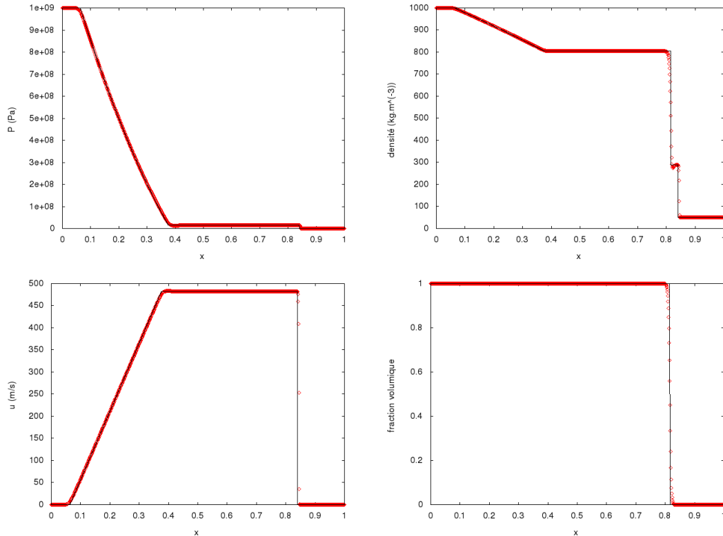
FIGURE 6.1 – Pression, densité, vitesse et fraction volumique pour la solution exacte (trait noir) et la solution numérique (points rouges) au temps t = 2.4 \times 10^{-4} \text{ s} pour le cas test mono-dimensionnel 1.
