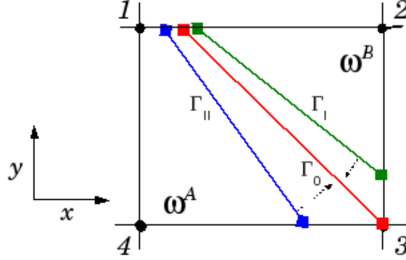
FIGURE 2.10 – Maille duale irrégulière avec trois configurations de l'interface \Gamma_I (ligne verte), \Gamma_{II} (ligne bleue) et \Gamma_0 (ligne rouge). \Gamma_0 est l'une position limite de l'interface quand l'interface passe de la configuration de type I à celle de type II , ou inversement.
