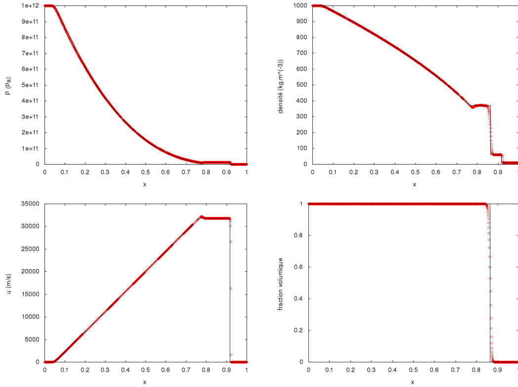
FIGURE 6.2 – Pression, densité, vitesse et fraction volumique pour la solution exacte (trait noir) et la solution numérique (points rouges) au temps t = 8.3 \times 10^{-6} \text{ s} pour le cas test mono-dimensionnel 2.
