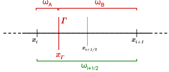
FIGURE 2.3 – Configuration géométrique dans une maille duale irrégulière. Le domaine \omega_{i+1/2} est divisé en deux sous-domaines \omega^A et \omega^B par l'interface \Gamma .
