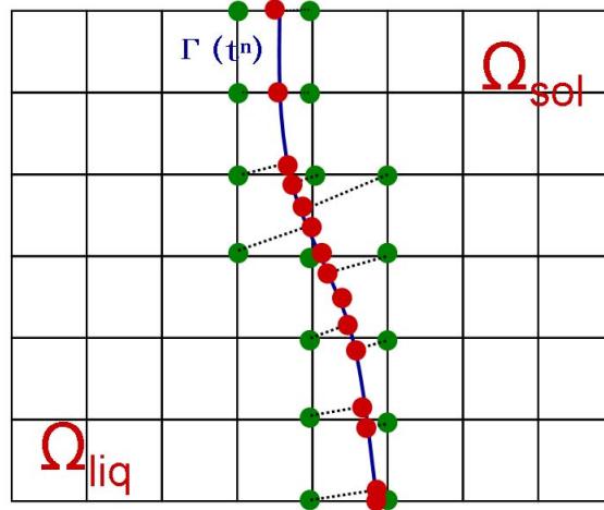
FIGURE 3.6 – L'initialisation du processus d'extension de champ de vitesse requiert de définir les vecteurs vitesse pour tous les noeuds proches (points verts) de l'interface (trait bleu) (Un noeud est dit "proche" de l'interface si au moins un des ses voisins appartient à l'autre domaine) Comme le champ de vitesse est choisi constant le long des normales à l'interface, le vecteur vitesse en chacun de ces noeuds est égal à celui de leurs projetés sur l'interface (points rouges).
