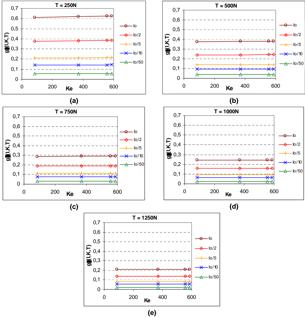
Figure 4.13. Valeurs de g_1(I, K, T) pour T = 250 \text{ N} (a), T = 500 \text{ N} (b), T = 750 \text{ N} (c), T = 1000 \text{ N} (d) et T = 1250 \text{ N} (e)
