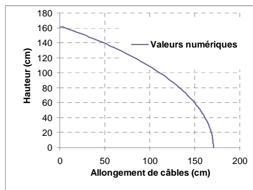
Figure 5.3. Hauteur du module en fonction de l'allongement de câbles de nappes
