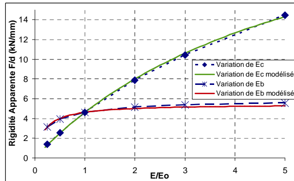
Figure 3.27. Comparaison entre les simulations numériques et le modèle rhéologique
