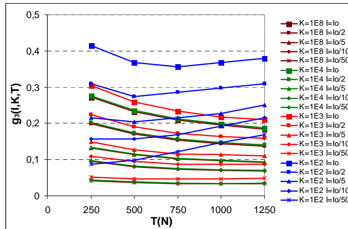
Figure 4.17. Evolutions de g_3(T) pour différentes valeurs de I et K
