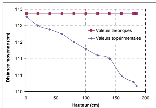
Figure 5.35. Distance des nœuds reliés par des câbles coplanaires
