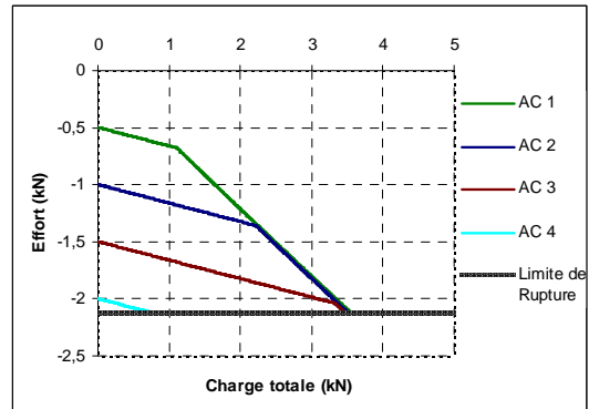
Figure 3.8. Effort dans les barres latérales en fonction du chargement total
