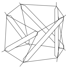
Figure 2.1. vue en perspective du modèle physique simple de 5 barres
