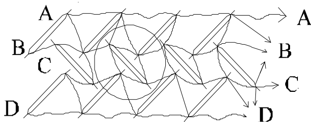
Figure 2.3. Vue en coordonnées cylindriques d'un modèle physique à 4 barres sur 3 couches
