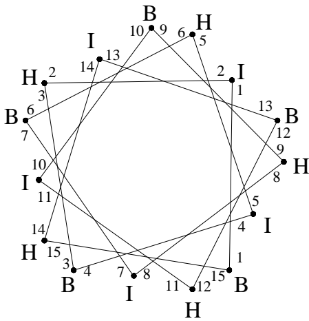
Figure 2.50. Schéma de mise en place des barres
