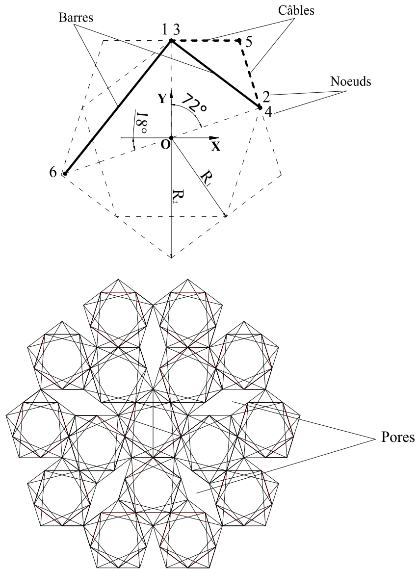
Figure A.2.Extrait d'un côté de l'anneau de tensegrité à base pentagonale et assemblage. Vues de dessus
