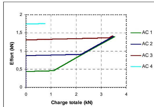
Figure 3.10. Effort dans les câbles coplanaires en fonction du chargement total
