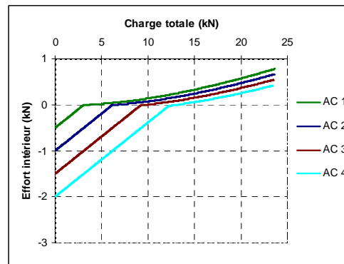
Figure 3.17. Effort dans les barres latérales en fonction du chargement total
