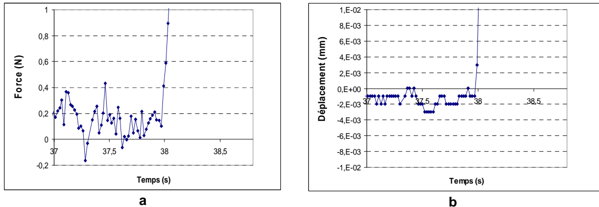
Figure 4.7. Courbes expérimentales Charge – Temps (a) et Déplacement – Temps (b)
