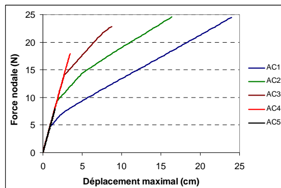
Figure 3.38. Déplacement maximal
