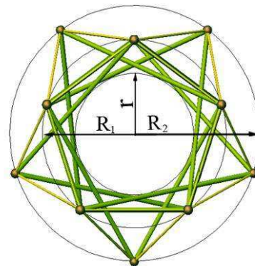
Figure 2.21. Vue de dessous
