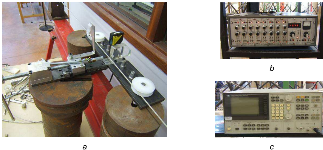
Figure 4.5. Matériels : Tensiomètre (a), Affichage du capteur de force (b), Analyseur de fréquence (c)
