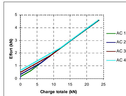
Figure 3.16. Effort dans les câbles non coplanaires en fonction du chargement total
