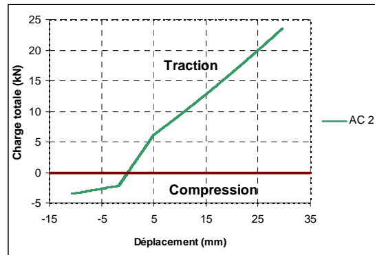
Figure 3.18. Allure de la rigidité du module
