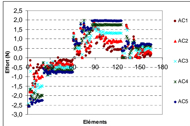
Figure 3.37. Efforts dans les éléments à la ruine pour différents niveaux d'autocontrainte
