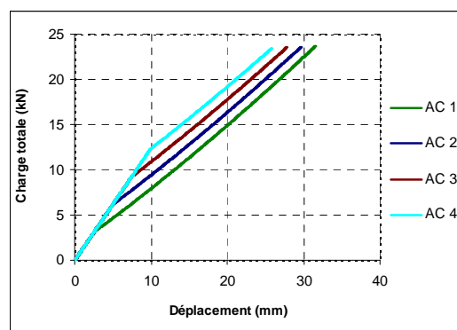
Figure 3.12. Chargement en fonction du déplacement vertical de la nappe supérieure
