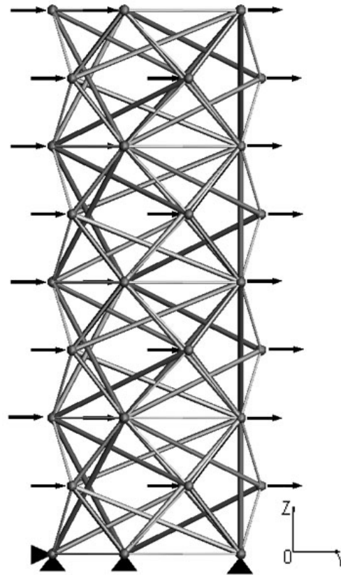
Figure 3.35. Schéma de chargement
