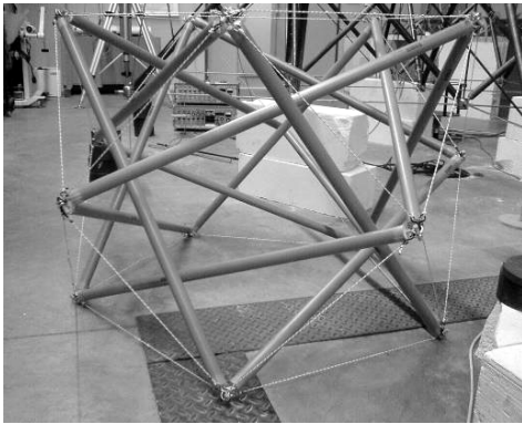
Figure 2.10. Maquette déployée
