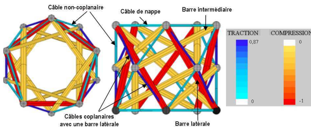
Figure 3.1. Visualisation de l'état d'autocontrainte obtenu
