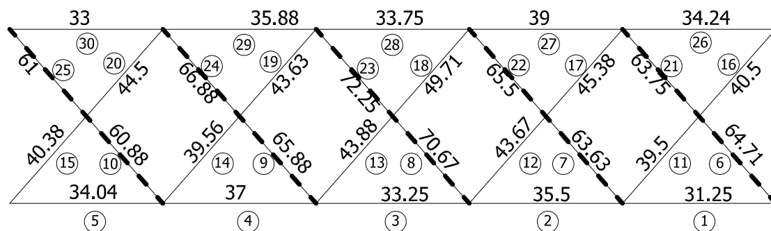
Figure 4.6. Mesure de fréquence en Hz sur les câbles (projection cylindrique)
