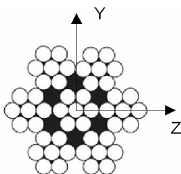
Figure 4.9. Section droite des câbles
