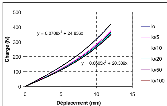
Figure 4.12. Charge – Déplacement T = 1000 \text{ N} et K = 1 \text{ E} + 8 \text{ N/mm}
