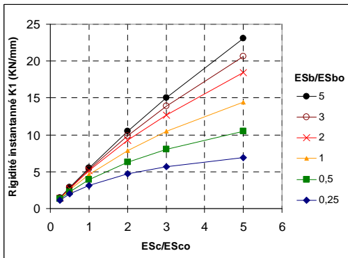
Figure 3.24. Rigidité instantanée K_1 en fonction de E_{Sc}^0 pour différentes valeurs de E_{Sb}^0
