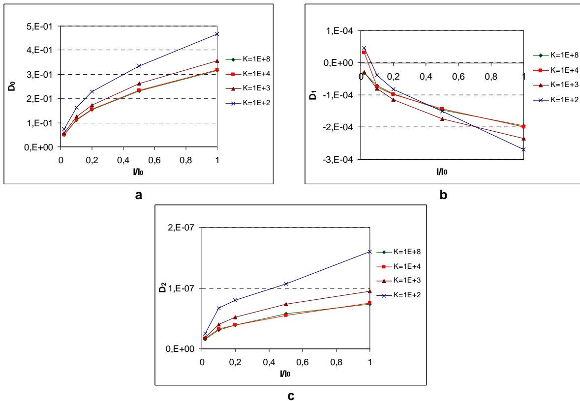
Figure 4.18. Evolutions de D_0 , D_1 et D_2 avec I/I_0 pour différentes valeurs de K
