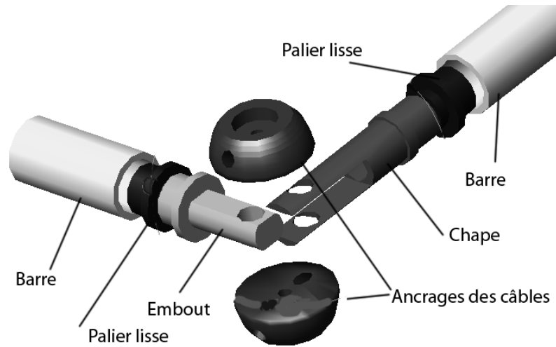
Figure 2.27. Nœud esquissé
