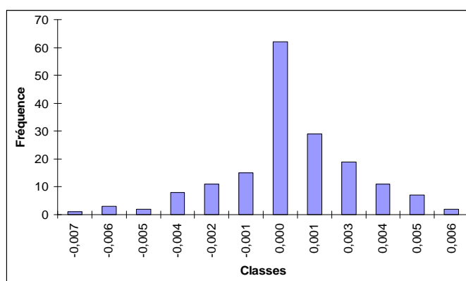
Figure 5.25. Histogramme des mesures après correction
