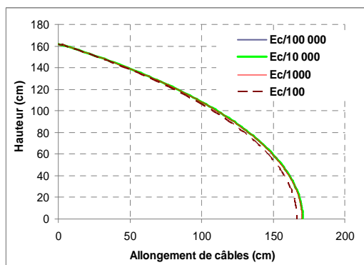
Figure 5.10. Variation de E_{c_{actif}}
