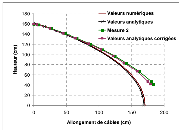
Figure 5.37. Confrontation des résultats après correction
