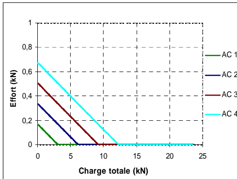
Figure 3.13. Effort dans les câbles de nappes en fonction du chargement total
