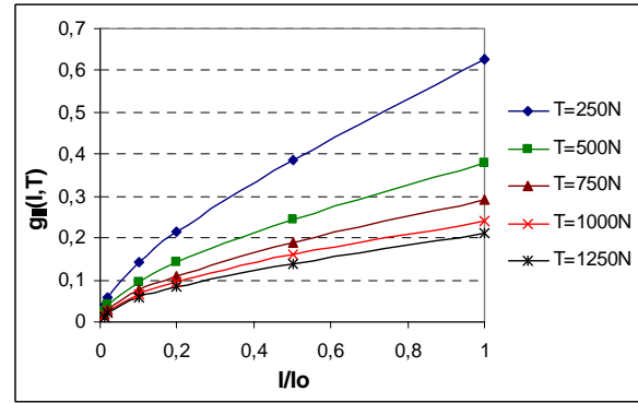
Figure 4.15. Corrélation de g_1(I,T) et I/I_0
