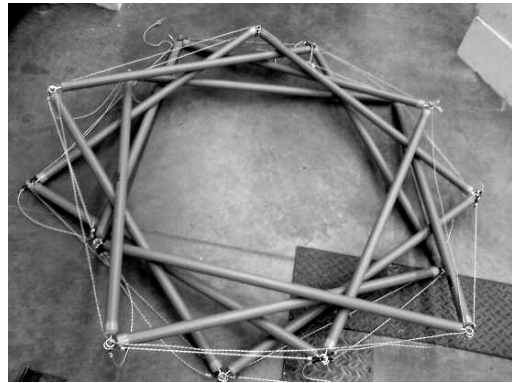
Figure 2.11. Maquette pliée
