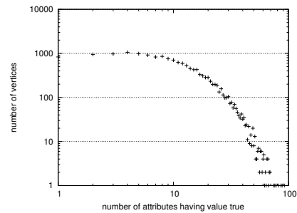
(d) Attributes distribution for \text{BioData}_{400}
