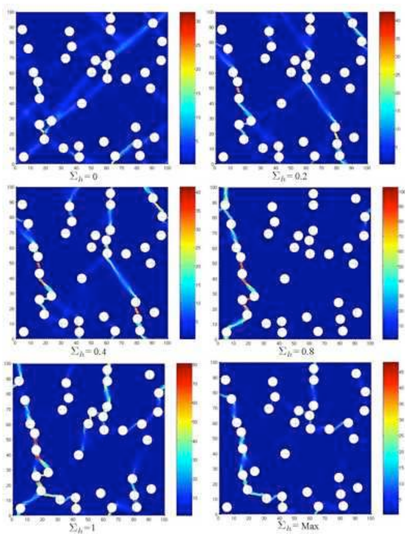
FIG. 13.4: Evolution du champ de vitesse de déformation en fonction de \Sigma_h pour le VER 3.
