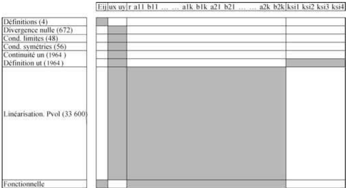
FIG. 5.5: Structure de la matrice des contraintes dans le cas cinématique plan avec la linéarisation BTN du critère de Mises.
