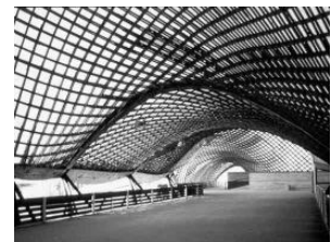
Fig. 14b F. Otto, Multihalle, Mannheim (1975)
