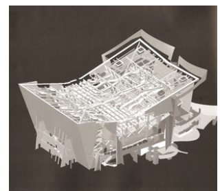
Fig. 15d Les outils couplés permettent de gérer dans un modèle unique des informations de nature différente (géométrie, mécanique, productive, etc.) F. Gehry, modèle numérique du projet EMP (2000)
