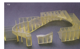
Fig. 4 Maquette stéréo lithographique (processus à contrôle numérique). G. Lynn, Artist Space, New York (1995)
