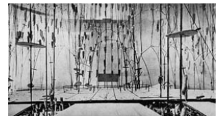
Fig. 14a A. Gaudí, maquette mécanique pour la recherche de forme de l'église Sagrada familia, Barcelone, Espagne (1898)
