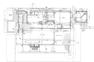
Fig. 6a R. Meier, plan du rez-de-chaussée, Smith House, (USA), 1967 [SCO94]
