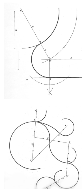
Fig. 11 Méthodes pour dessiner les raccords entre arcs de cercle de rayon différent : la rationalisation des courbes complexes à travers des arcs de cercle requière une bonne expertise géométrique et difficilement peut être réalisée de façon intuitive.
