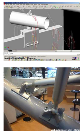
Fig. 24 Les outils numériques sont essentiels tant dans la modélisation que dans la production de l'Architecture Non Standard. B. Franken et Bollinger + Grohmann, BMW pavilions, Allemagne (2000)
