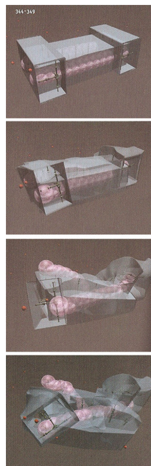
Fig. 8 La forme comme résultat d'une déformation continue. G. Lynn, House prototype, Long Island, USA (1994), modélisation numérique (en haut) et maquette (à gauche).
