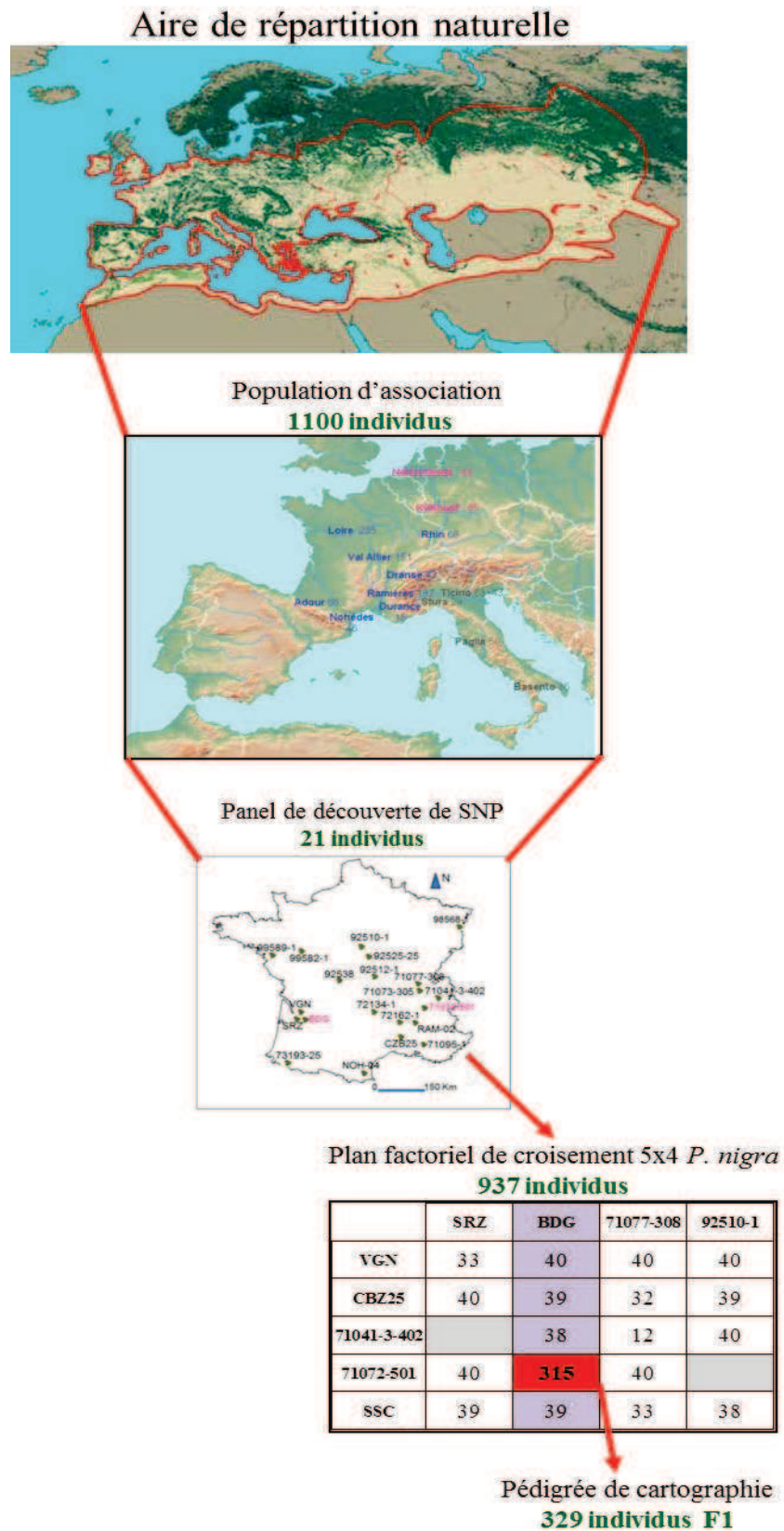
Figure 0.1 : Représentation schématique des ressources génétiques de peuplier noir disponibles et utilisées dans la thèse.
