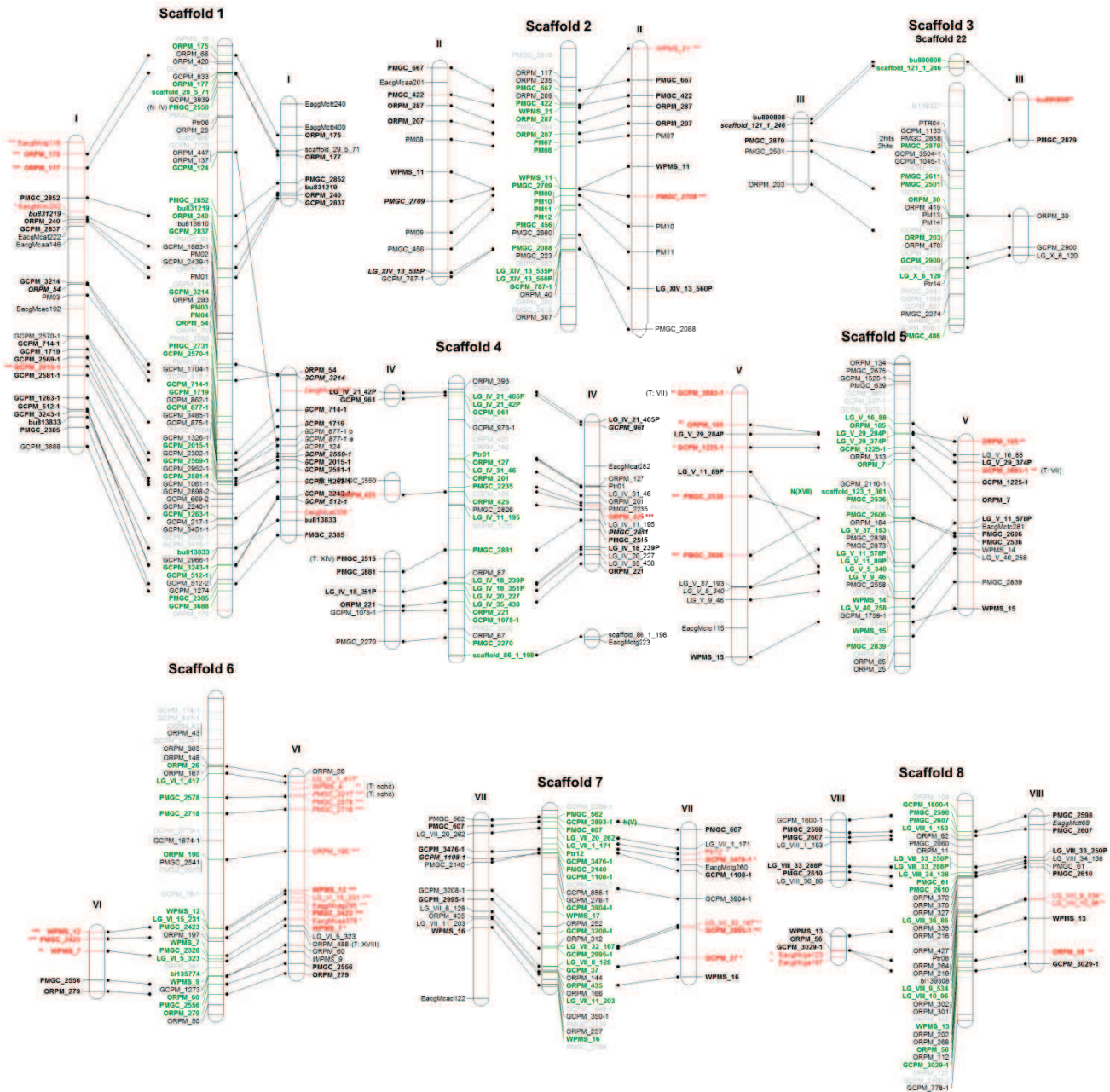
Figure III.5 : Alignement du génome de P. trichocarpa Nisqually-1 v2.0 des cartes génétiques parentales basées sur l'analyse de la ségrégation de marqueurs SSR, SNP et AFLP dans la descendance du croisement entre P. nigra 71072-501 x BDG (319 individus F1). Les cartes génétiques ont été construites avec le logiciel Mapmaker et les paramètres décrits dans le chapitre IV. La position de marqueurs sur la séquence du génome est déterminée par alignement BLAST des amorces SSR et des sondes SNP. Pour chaque chromosome, de gauche à droite, la carte génétique maternelle (71072-501), la position des marqueurs sur le génome et la carte génétique paternelle (BDG). En gras, les marqueurs ponts entre cartes génétiques ; en rouge, les marqueurs distordus, **: 0.01 < \chi^2 P-value \leq 0.05 , **: 0.001 < \chi^2 P-value \leq 0.01 , *** 0.001 \leq \chi^2 P-value; En italique, marqueurs accessoires ; Les discordances (non synthétie) entre cartes génétiques et génomes sont indiquées à côté du marqueur (par ex. : (N : IV) le marqueur est localisé sur le GL IV des cartes génétiques) ; Tous les marqueurs testés dans la thèse ont été positionnés sur la séquence du génome : en gris, les marqueurs qui n'amplifient pas ; en noir, les marqueurs monomorphes ; en vert gras, les marqueurs cartographiés (polymorphes).
