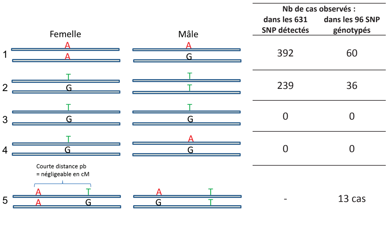
Figure III.3 : Représentation schématique des cas de figure possibles de SNP. Effectifs de ceux retrouvés dans les données de séquence de fragments de gènes chez les deux parents du pedigree F1 P. nigra .
