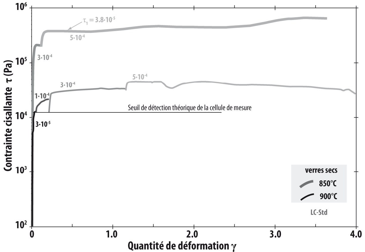
Figure VIII- 17 : courbes rhéologiques des échantillons mixtes composés de verres secs (dacite et hapltonalite) déformé en torsion lors des expériences PP302 (850°C) et PP303 (900°C).
