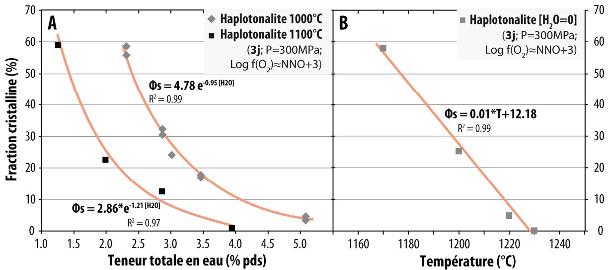
Figure IV- 8: fractions cristallines de suspensions haplotonalitiques (A) à 1000 et 1100°C pour différentes teneurs en eau, et (B) de l'haplotonalite sèche en fonction de la température.
