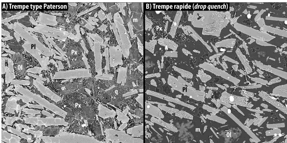
Figure IV- 17 : images MEB montrant la texture du basalte de Santorin partiellement fondu (1170°C), puis refroidi (A) à ~60°C/min (type paterson), et (B) rapidement (« drop quench »).
