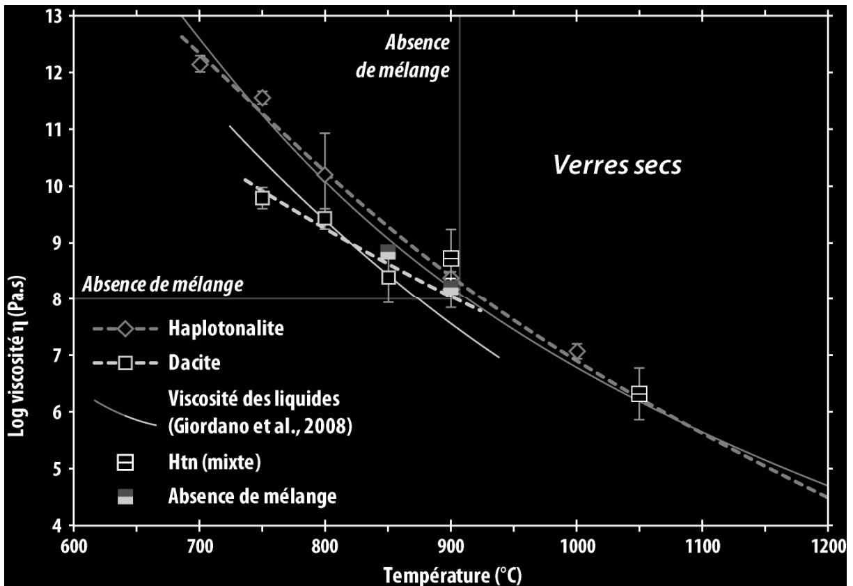
Figure VIII- 18 : viscosité des échantillons mixtes composés de verres secs (dacite et hapltonalite) en fonction de la température. Aucune figure de mélange ne fut observée.
