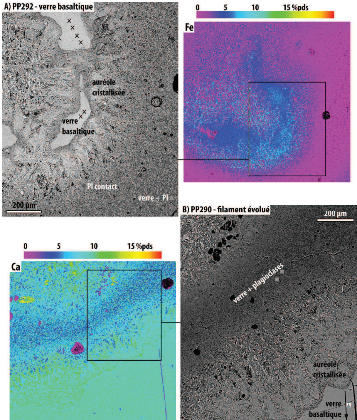
Figure VI- 8 : (A) poches de verre basaltique isolées, ceinturées par une auréole cristallisée et (B) « filament » de magma felsique situé entre 2 zones de magma basaltique. Les cartographies chimiques ont été réalisées à plus faible agrandissement et recouvrent largement la zone illustrée par l'image MEB (voir aussi annexe B).
