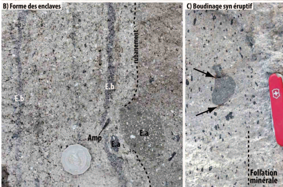
Figure C 2 : photographies de produits issus de la coulée de blocs et cendres de février 2011, vers Trants Airport, Montserrat. (A) bloc avec un rubanement de magmas de densités différentes témoignant d'un intense cisaillement tardif (conduit, dôme). (B) enclaves basiques (E.b) et andésitiques (E.a) et rubanement textural induit par le cisaillement orienté verticalement sur cette image. (C) enclave andésitique fragmentée perpendiculairement à la foliation minérale marquée par l'alignement des phénocristaux d'amphiboles.
