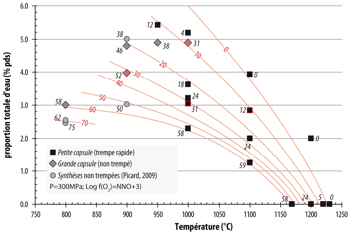
Figure IV- 7 : cristallinité de l'haplotonalite pour différentes teneurs en eau et températures. Les carrés et losanges entourés en rouge sont des suspensions présentées en Fig. IV-9.
