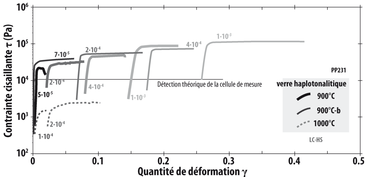
Figure VIII- 4 : courbes rhéologiques du verre haplotonalitique à haute température (900 et 1000°C) obtenues avec la cellule de mesure haute sensibilité (LC-HS).
