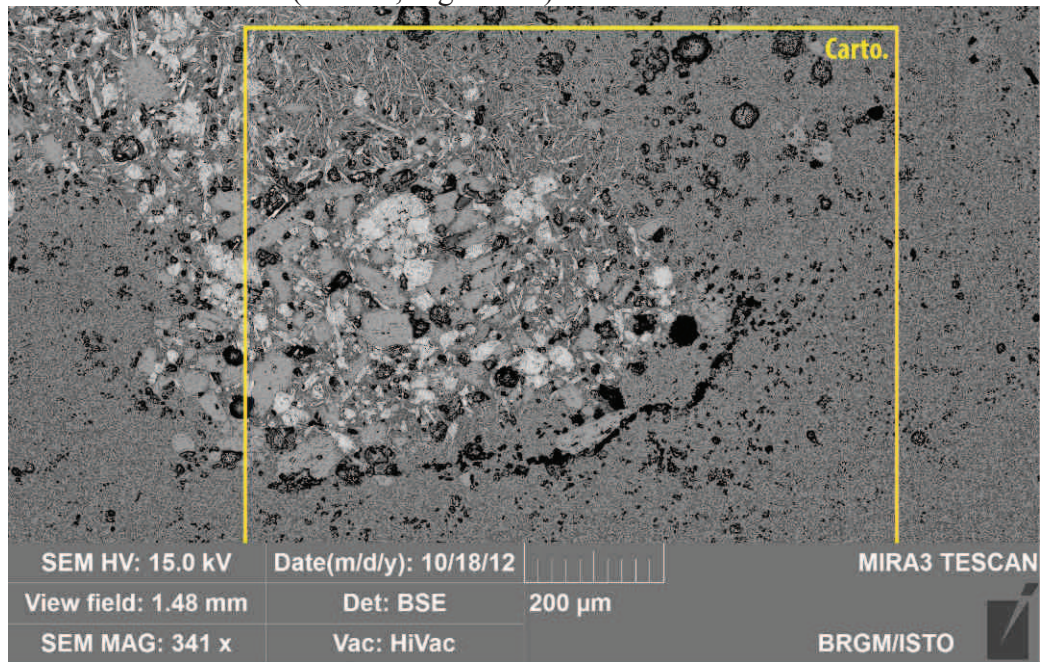
Enclave en formation (PP261 ; Fig. VI*7i)
