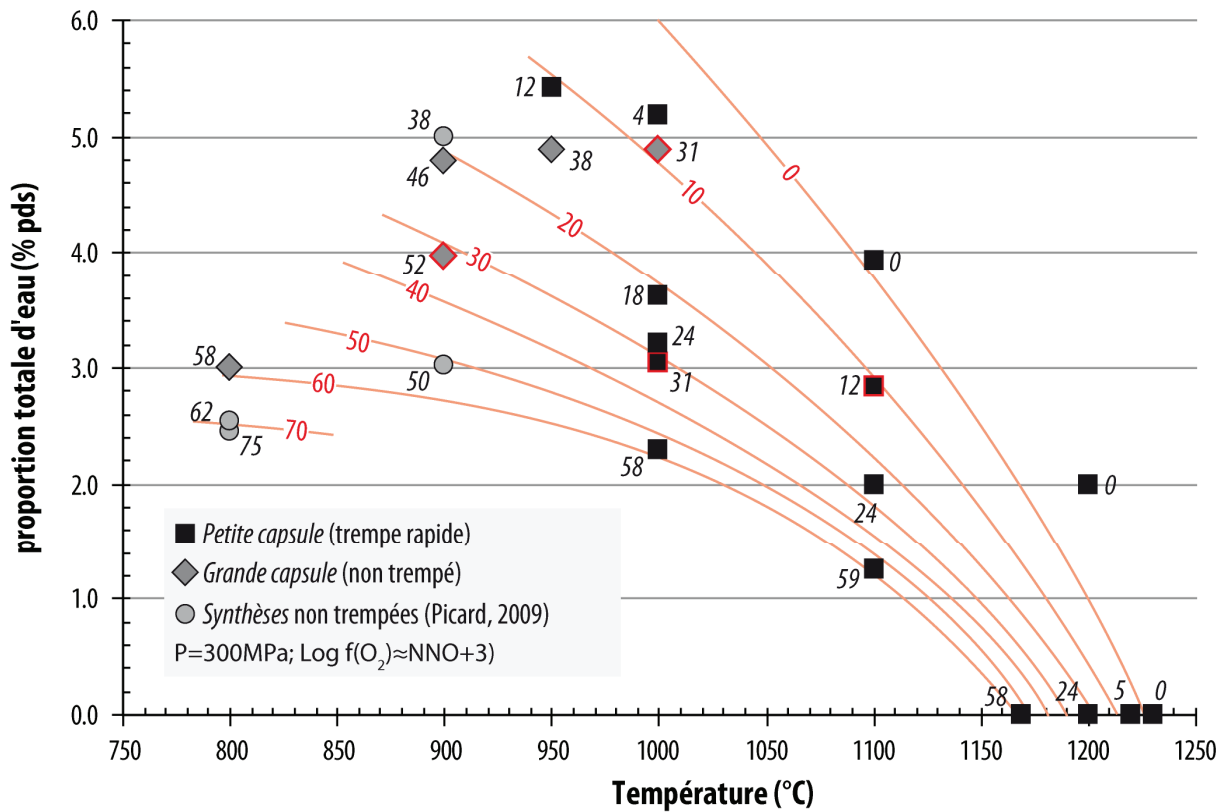
Figure IV- 7 : cristallinité de l’haplotalonite pour différentes teneurs en eau et températures. Les carrés et losanges entourés en rouge sont des suspensions présentées en Fig. IV-9.
