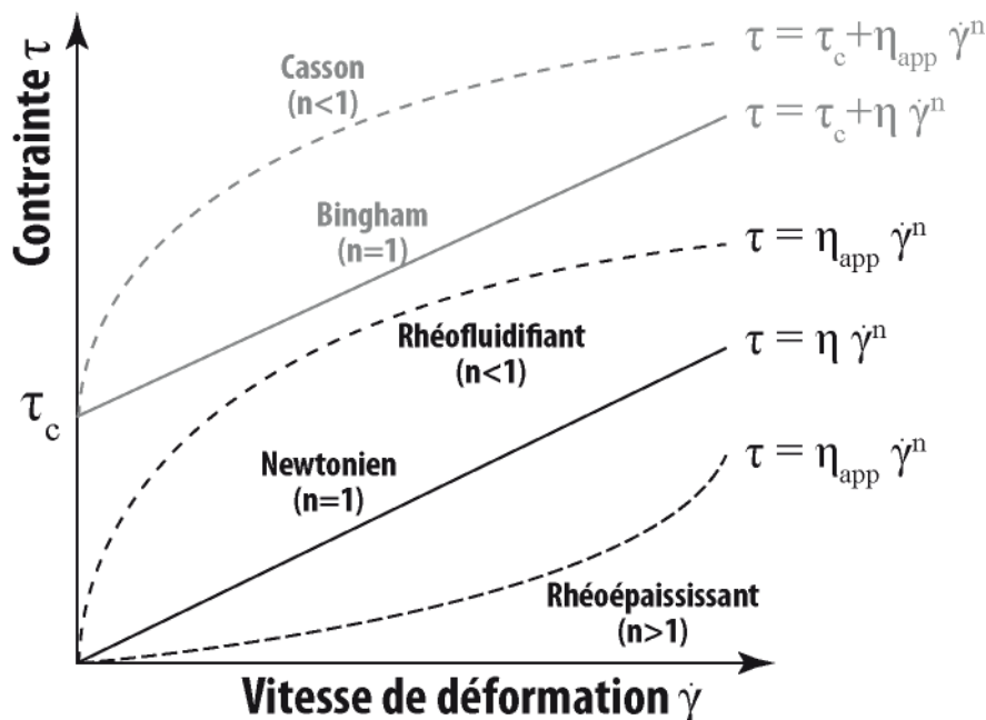
Figure A 1 : Rhéogramme synthétisant le comportement rhéologique des fluides parfaits.
