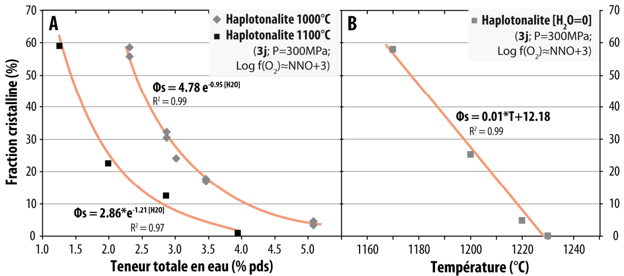
Figure IV- 8 : fractions cristallines de suspensions haplotalonitiques (A) à 1000 et 1100°C pour différentes teneurs en eau, et (B) de l’haplotalonite sèche en fonction de la température.
