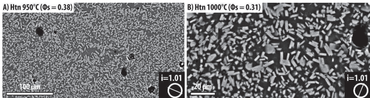
Figure IV- 14 : images MEB des produits de synthèses haplotalitiques réalisées à 950 et 1000°C. L'intensité i de la fabrication cristalline moyenne est faible dans les 2 suspensions.
