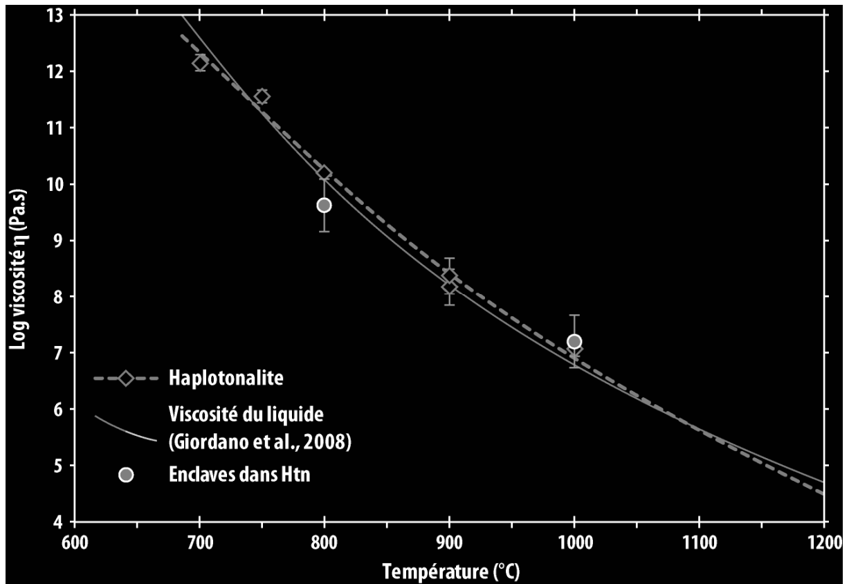
Figure VIII- 20 : viscosité des échantillons contenant des enclaves dans un verre hapltonalitique déformés lors des expériences PP178 (1000°C) et 316 (800°C). Les viscosités des échantillons peuvent être comparées avec le modèle de viscosité du verre hapltonalitique, dégageant ainsi l'effet liée à la présence d'enclaves.
