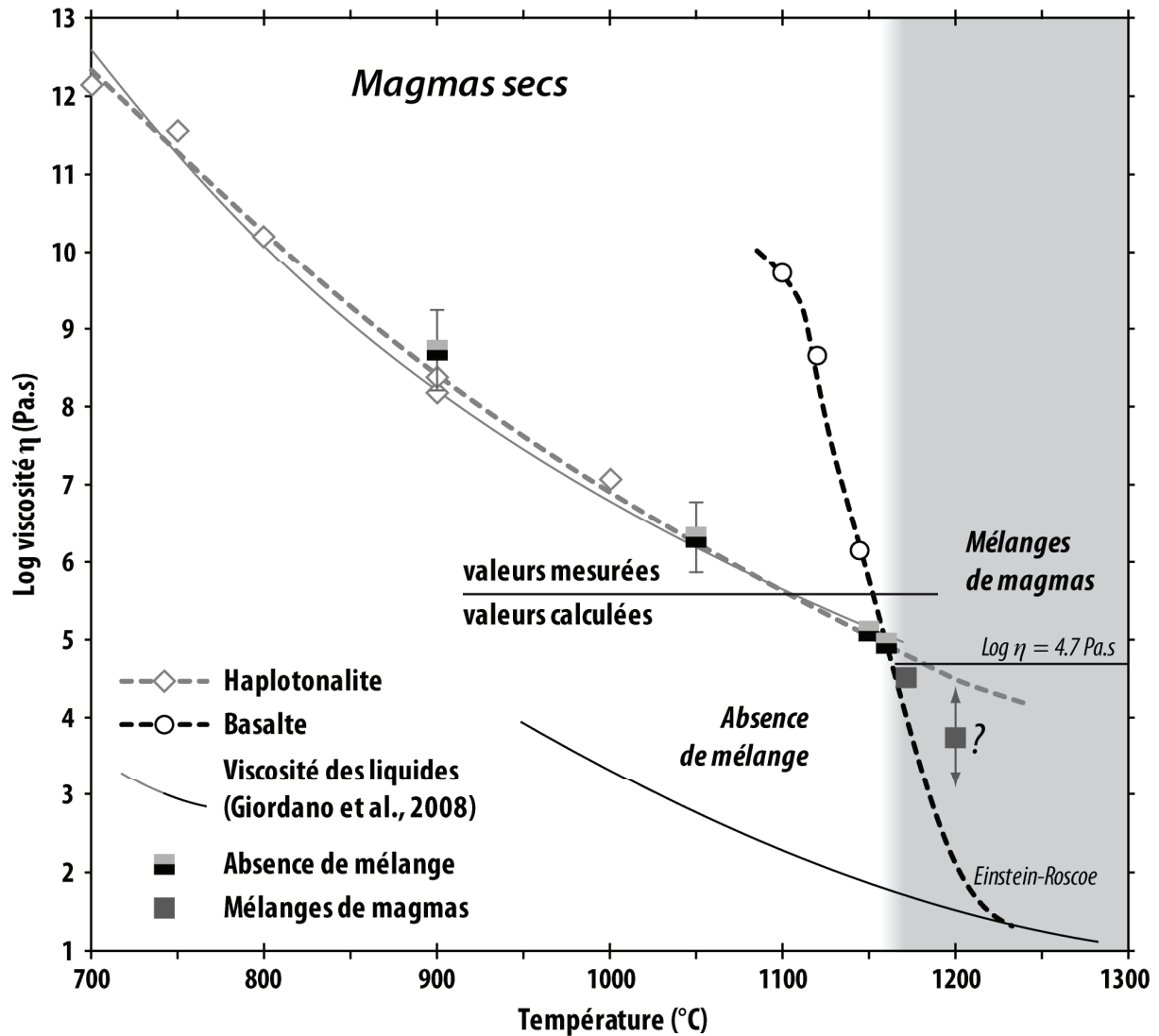
Figure VIII- 11 : viscosité des échantillons mixtes mesurée ( T < 1140^\circ\text{C} ) et calculée (à T > 1140^\circ\text{C} ) en fonction de la température. La viscosité de chacun des constituants figure également.
