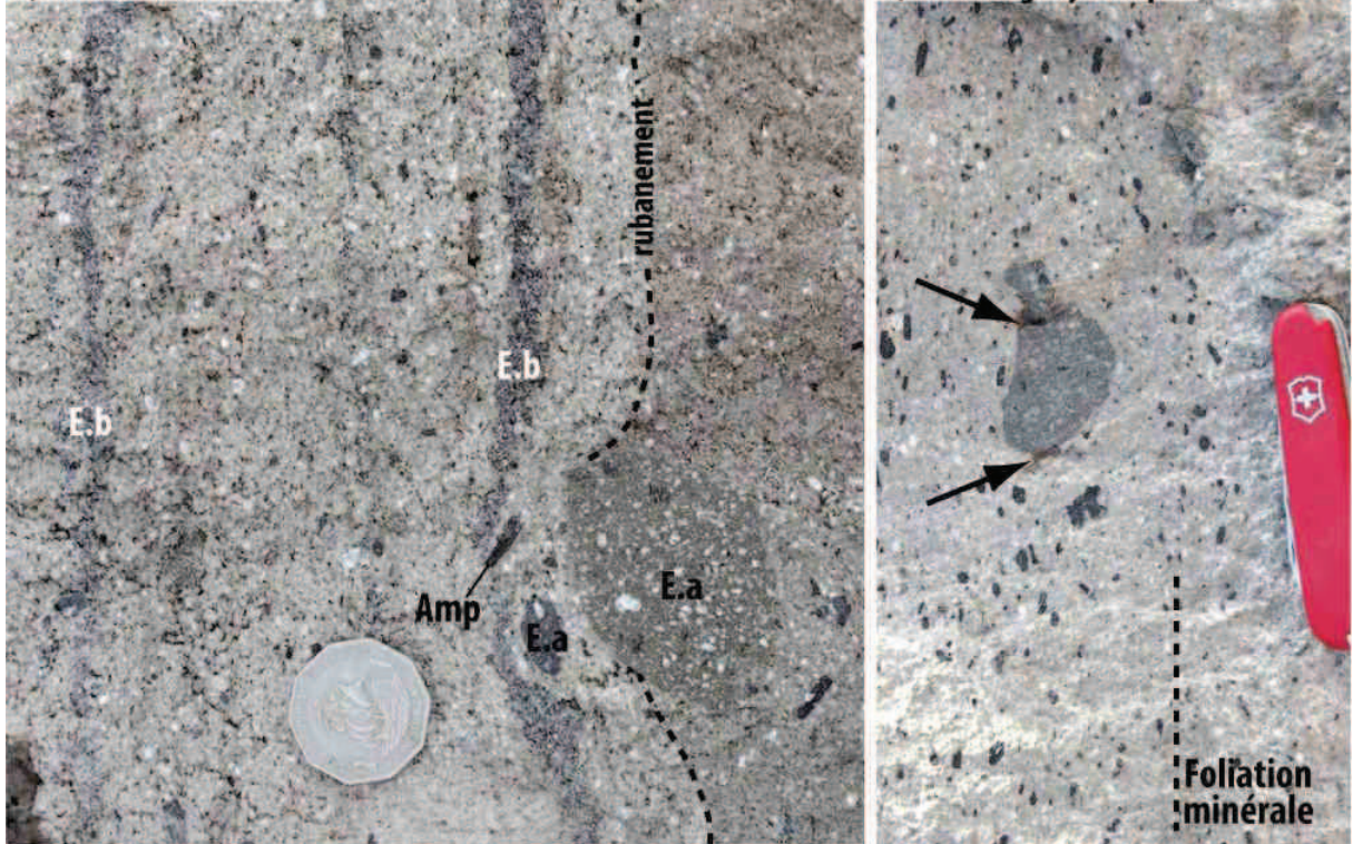
Figure C 2 : photographies de produits issus de la coulée de blocs et cendres de février 2011, vers Trants Airport, Montserrat. (A) bloc avec un rubanement de magmas de densités différentes témoignant d'un intense cisaillement tardif (conduit, dôme). (B) enclaves basiques (E.b) et andésitiques (E.a) et rubanement textural induit par le cisaillement orienté verticalement sur cette image. (C) enclave andésitique fragmentée perpendiculairement à la foliation minérale marquée par l'alignement des phénocristaux d'amphiboles.
