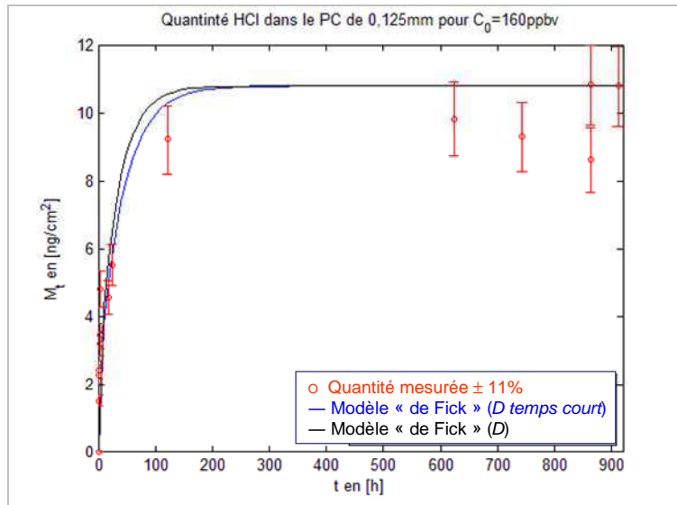
Evolution de la quantité d'HCl sorbée par les films de PC d'épaisseur 0,125 mm en fonction du temps d'exposition, pour une concentration d'exposition \sim 160 ppbv à TA et P_{atm} : \circ : points expérimentaux ; — : courbe théorique du modèle de Fick tracée avec le D temps court ; — : courbe théorique du modèle de Fick tracée avec le D déterminé par optimisation mathématique utilisant Matlab
