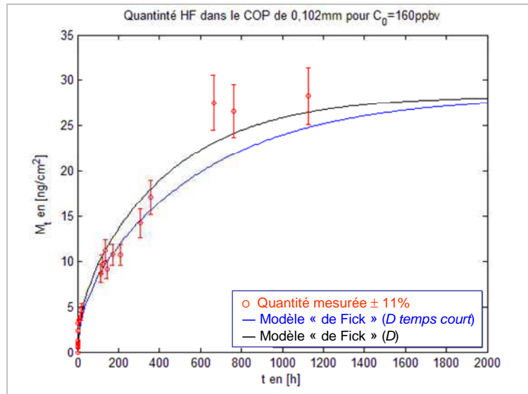
Evolution de la quantité d'HF sorbée par les films de COP d'épaisseur 0,102 mm en fonction du temps d'exposition, pour une concentration d'exposition ~ 160 ppbv à TA et P_{atm} : o : points expérimentaux ; — : courbe théorique du modèle de Fick tracée avec le D temps court ; — : courbe théorique du modèle de Fick tracée avec le D déterminé par optimisation mathématique utilisant Matlab
