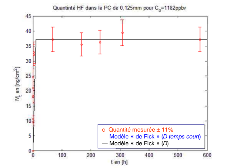
Evolution de la quantité d'HF sorbée par les films de PC d'épaisseur 0,125 mm en fonction du temps d'exposition, pour une concentration d'exposition ~ 1182 ppbv à TA et P_{am} : \circ : points expérimentaux ; — : courbe théorique du modèle de Fick tracée avec le D temps court ; — : courbe théorique du modèle de Fick tracée avec le D déterminé par optimisation mathématique utilisant Matlab
