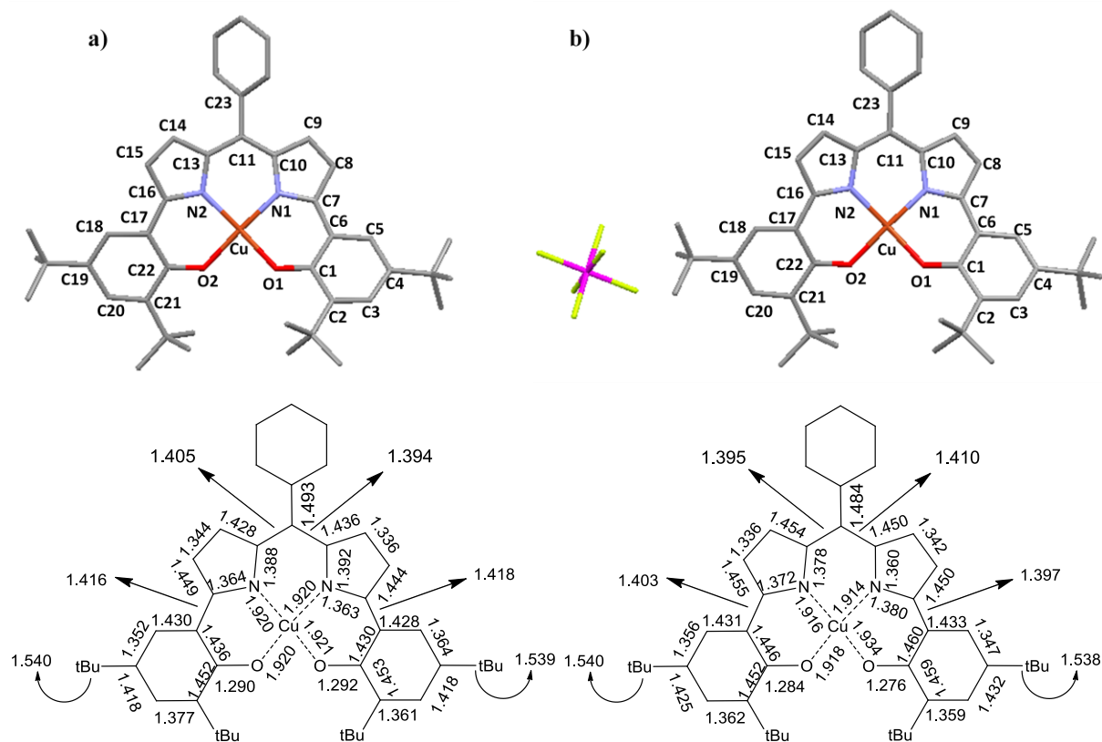
Figure 135: Structures cristallographiques des deux complexes a) monooxydé [Cu(10)•] et b) dioxydé [Cu(10)] + .SbF 6 - contenues dans la même maille élémentaire (ellipsoïdes à 30 %) et analyse des longueurs de liaison en Å (avec un erreur de ± 0.01 Å).
