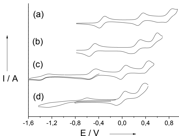
Figure 169: Courbes CV de solutions à 0.5 mM (+ 0.1 M TBAP): (a) [\text{Co}(\text{1}_{\text{N}_4}^{\text{tBu}})] dans \text{CH}_2\text{Cl}_2 ; (b) [\text{Co}(\text{1}_{\text{N}_4}^{\text{tBu}})] dans \text{CH}_2\text{Cl}_2 + 40 \mu\text{L} de pyridine pure (25 équivalents), c) [\text{Co}(\text{1}_{\text{N}_4}^{\text{tBu}})(\text{im})_2]^+ dans \text{CH}_2\text{Cl}_2 et d) [\text{Co}(\text{1}_{\text{N}_4}^{\text{tBu}})(\text{im})_2]^+ dans \text{CH}_2\text{Cl}_2 + 200 équivalents de N -méthylimidazole. Les potentiels sont donnés par rapport au couple \text{Fc}^+/\text{Fc} de référence. Vitesse de balayage: 0.1 V / s; T = 298 K.
