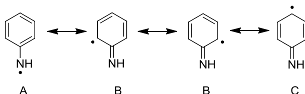
Figure 78: Formes de résonances du radical anilinye
