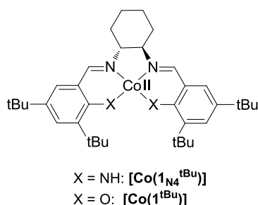
Figure 162 : Structures des complexes neutres initiaux de cobalt étudiés dans cette partie.
