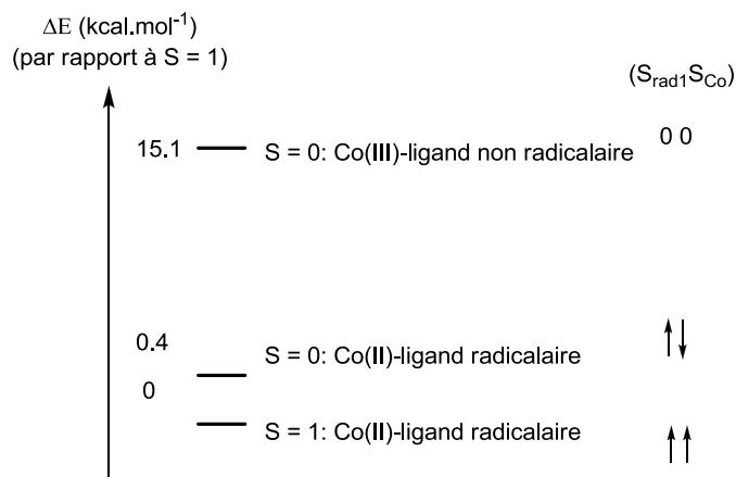
Figure 184: Représentation des énergies calculées pour les différents états de [Co(10)].
