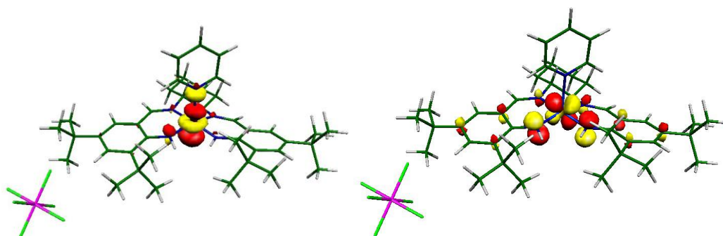
Figure 175: localisation des deux SOMOs dans [\text{Co}(1_{\text{N4}}^{\text{tBu}})(\text{pyr})]^+.\text{SbF}_6^- .
