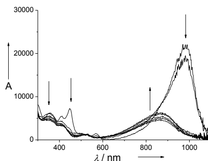
Figure 176: Titrage d'une solution à 0.05 mM dans \text{CH}_2\text{Cl}_2 de [\text{Co}(\text{1}_{\text{N}_4}^{\text{tBu}})]^+ généré par électrochimie de 0 à 74 équivalents de pyridine. Les flèches indiquent l'évolution du spectre au cours des ajouts. Trajet optique = 1.000 cm. T = 233 K.
