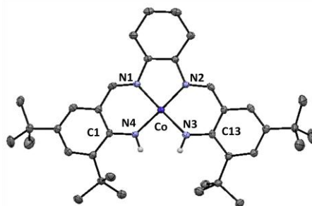
Figure 165: Structure cristallographique de [\text{Co}(\text{1}_{\text{N}_4}^{\text{tBu}})] (ellipsoïdes à 30 %). Pour plus de clarté, les atomes d'hydrogène sont omis sauf pour les phénylamidures.
