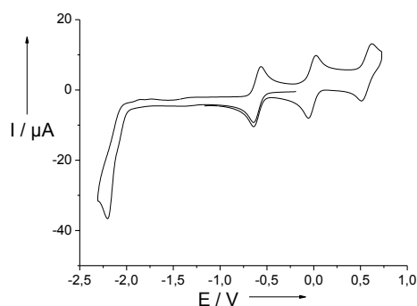
Figure 188: Courbe de voltamétrie cyclique d'une solution à 0.5 mM de [\text{Co}^{\text{II}}(10)^{\bullet}] dans \text{CH}_2\text{Cl}_2 (+ 0.1 M TBAP). Vitesse de balayage : 0.1 \text{ V}\cdot\text{s}^{-1} , T = 298 \text{ K} . Les potentiels sont donnés par rapport au couple de référence \text{Fc}^+/\text{Fc} .
