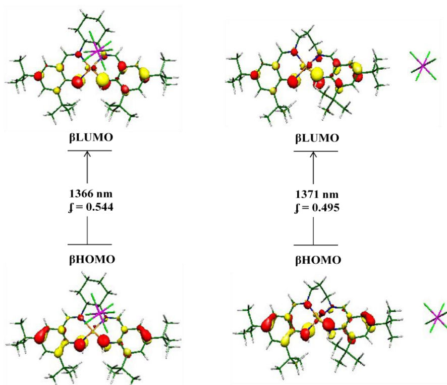
Figure 100: Attribution par TD-DFT de la transition dans le proche IR pour [\text{Cu}(1\text{N}_4^{\text{tBu}})]^+ et [\text{Cu}(4\text{N}_4^{\text{tBu}})]^+ .
