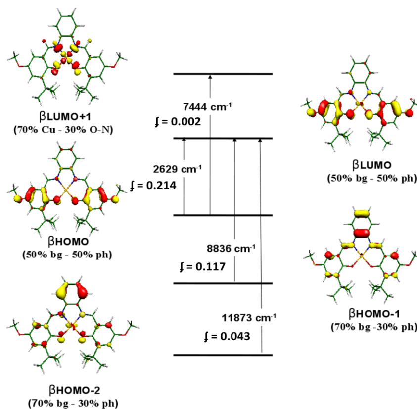
Figure 65: Attribution des transitions NIR du complexe [\text{Cu}(2\text{OMe})]^+ par TD-DFT et pourcentage des groupes aux orbitales moléculaires : bg = pont phénylènediamine, ph = phénoxyde/phénolate.
