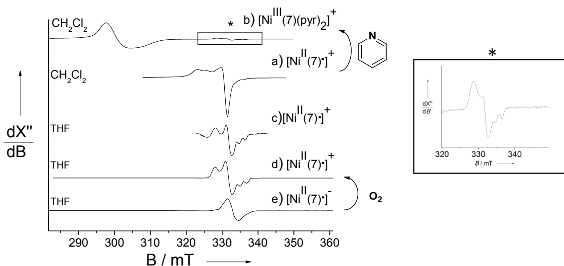
Figure 120 : Spectres RPE en bande X enregistré à 100 K de solutions des complexes : a) [\text{Ni}(7)]^{\cdot+} généré par électrochimie (1mM dans \text{CH}_2\text{Cl}_2 + 0.1M TBAP) du même échantillon en présence de 2% en volume de pyridine, c) [\text{Ni}(7)]^{\cdot+} généré par oxydation chimique (à \text{AgSbF}_6 ) (1mM dans THF), e) [\text{Ni}(7)]^{\cdot-} généré par réduction chimique en boîte à gant (par NaHg 5%) (4mM dans le THF) d) même échantillon exposé 10 minutes à l'air.
