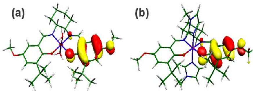
Figure 159: Localisation des SOMOs dans (a) [\text{Co}(\text{1}^{\text{OMe}})]^{2+} et (b) [\text{Co}(\text{1}^{\text{OMe}})(\text{im})_2]^{2+} .
