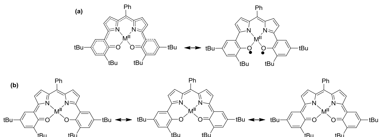
Figure 134: Représentation des différentes formulations possibles du complexe dioxydé sur le ligand: a) ligand diradicalaire [\text{Ni}(10)^{\bullet\bullet}]^+ et b) système à couche fermée [\text{Ni}(10)^{\text{ox}}]^+ .
