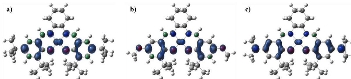
Figure 51: Représentation de la densité de spin calculée pour: a) [\text{Ni}^{\text{II}}(\text{1}^{\text{tBu}})\cdot]^+ , b) [\text{Ni}^{\text{II}}(\text{1}^{\text{OMe}})\cdot]^+ et c) [\text{Ni}^{\text{II}}(\text{1}^{\text{NMe}_2})\cdot]^+ , en utilisant la fonctionnelle B3LYP.
