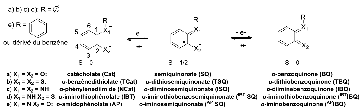
Figure 18: Etats redox accessibles de l' o -catécholates, de l' o -benzènedithiolates et de l' o -phénylènediimides et numérotation du cycle.
