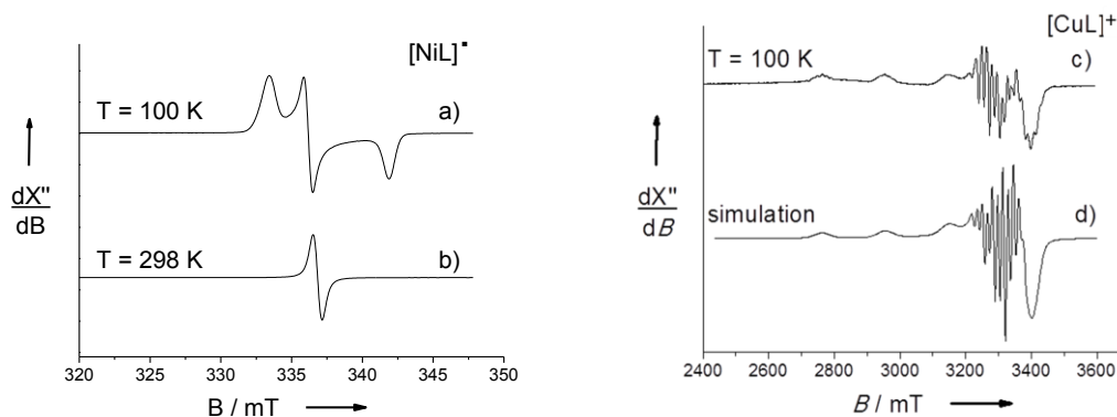
Figure 137: Spectres RPE en bande X de solutions à 0.5 mM dans \text{CH}_2\text{Cl}_2 anhydre des complexes : a) monoxydé [\text{Ni}(10)^{\bullet}] enregistré à 100K et b) enregistré à 298 K ; et c) dioxydé [\text{Cu}(10)^{\text{ox}}]^{\bullet+} généré par électrochimie (+ 0.1M TBAP) enregistré à 100 K. Le spectre d) représente la simulation du spectre c) en utilisant les paramètres détaillés dans le texte.
