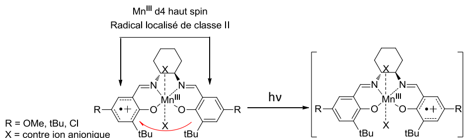
Figure 36 : Localisation du radical dans des complexes salen de \text{Mn}^{\text{III}} .
