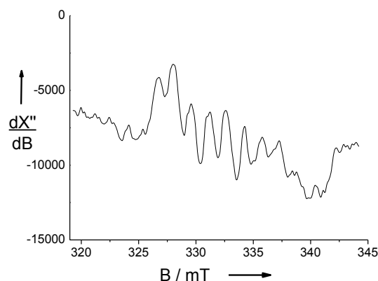
Figure 180: Spectre RPE en bande X d'une solution à 0.5 mM dans \text{CH}_2\text{Cl}_2 (+0.1 M TBAP) du dication [\text{Co}(\text{1}_{\text{N}_4}^{\text{tBu}})]^{2+} généré par électrochimie. T = 220 K.
