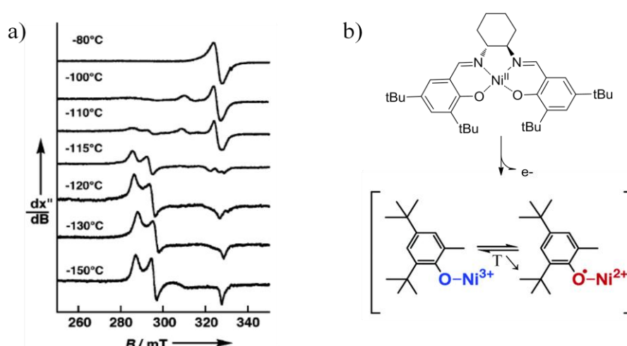
Figure 39: a) Spectre RPE en bande X en fonction de la température de [\text{Ni}^{\text{II}}(1^{\text{tBu}})] monoxydé à 0.5 mM dans \text{CH}_2\text{Cl}_2 . Puissance microonde : 1 mW, amplitude de modulation : 0.63 mT. b) représentation des deux tautomères de valence en équilibre dans \text{CH}_2\text{Cl}_2 .
