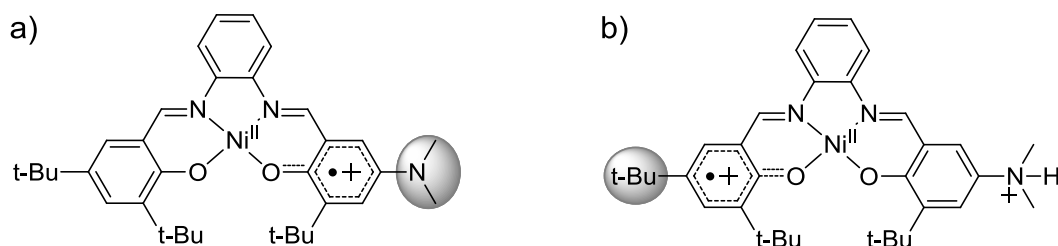
Figure 77: Structures électroniques des complexes a) [\text{Ni}(\text{3})]^+ et b) [\text{Ni}(\text{3H})]^{2+} .
