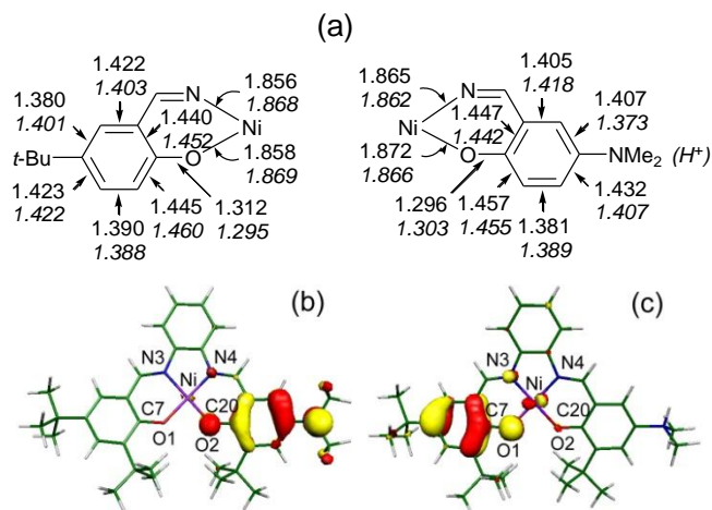
Figure 75: (a) Longueurs de liaison (en Å) dans les cycles phénolate/phénoxyde de [\text{Ni}(3')]^+ (texte normal) et [\text{Ni}(3\text{H})]^{2+} (texte en italique) obtenues par optimisation de géométrie (pour plus de clarté seul le substituant en para est représenté) et localisation de la SOMO de [\text{Ni}(3')]^+ (b) et [\text{Ni}(3\text{H})]^{2+} (c).
