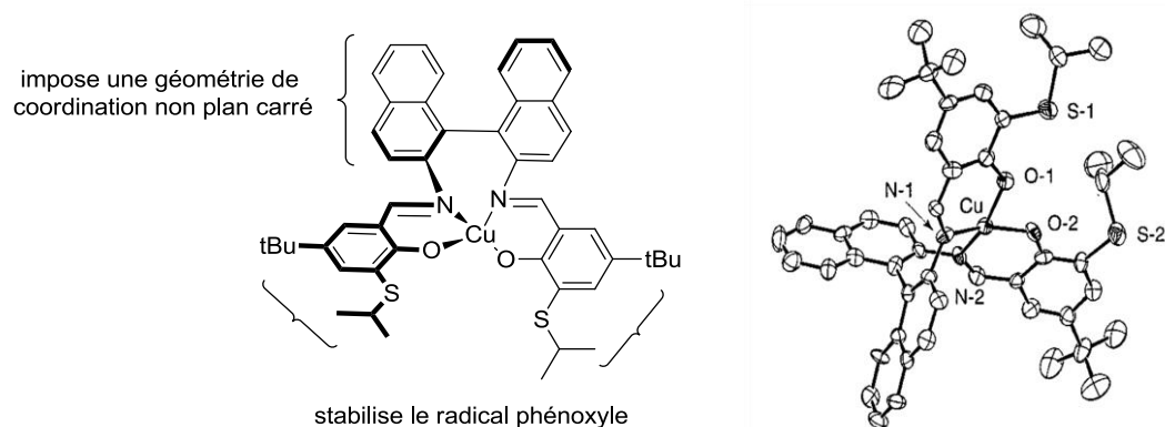
Figure 44: Représentation du complexe [Cu II (18)] (à gauche) et de sa structure cristallographique par diffraction des rayons X (à droite). 128
