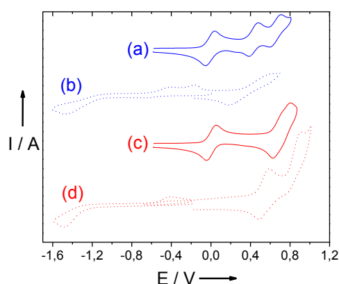
Figure 152: Courbes CV de solutions à 0.5 mM dans \text{CH}_2\text{Cl}_2 (+ 0.1 M TBAP) de: (a) [\text{Co}(\mathbf{1}^{\text{OMe}})] , (b) [\text{Co}(\mathbf{1}^{\text{OMe}})(\text{im})_2]^+ en présence de 10 eq de N -méthylimidazole, (c) [\text{Co}(\mathbf{1}^{\text{tBu}})] et (d) [\text{Co}(\mathbf{1}^{\text{tBu}})(\text{im})_2]^+ en présence de 10 eq de N -méthylimidazole. Les potentiels sont donnés par rapport au couple \text{Fc}^+/\text{Fc} de référence. Vitesse de balayage: 0.1 V / s; T = 298 K.
