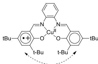
Figure 45: Pont phénylènediamine rigidifiant la structure [Cu II (2 tBu )] + : communication électronique accrue.
