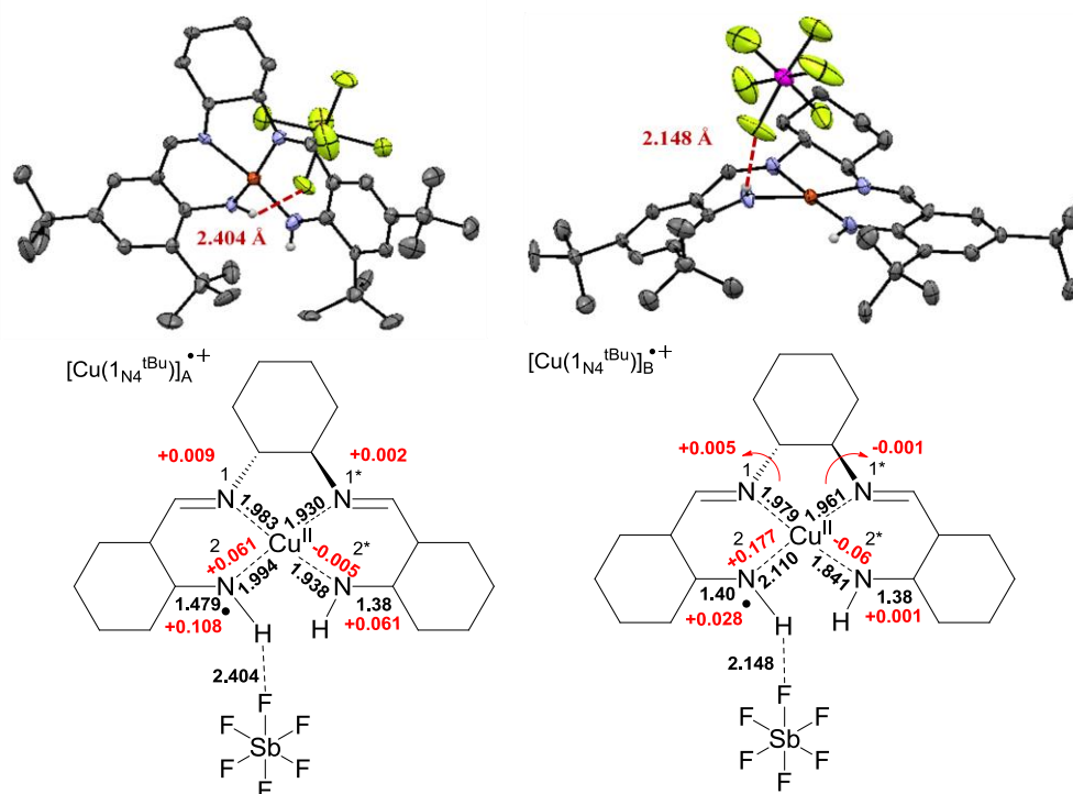
Figure 92: Structure cristallographique du complexe monoxydé [\text{Cu}(\text{1N}_4^{\text{tBu}})]^{\text{A}+\text{}} \cdot \text{SbF}_6^- (ellipsoïdes à 30 %) et comparaison des longueurs de liaison par rapport au complexe neutre [\text{Cu}(\text{1N}_4^{\text{tBu}})] .
