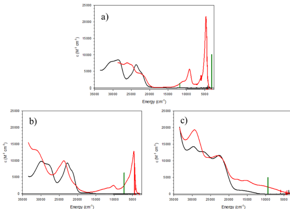
Figure 55: Spectres UV-vis-proche IR des complexes de Ni (neutre: ligne noire; monoxydé: ligne rouge): a) [\text{Ni}^{\text{II}}(\mathbf{1}^{\text{tBu}})] et [\text{Ni}^{\text{II}}(\mathbf{1}^{\text{tBu}})]^{\bullet+} ; b) [\text{Ni}^{\text{II}}(\mathbf{1}^{\text{OMe}})] et [\text{Ni}^{\text{II}}(\mathbf{1}^{\text{OMe}})]^{\bullet+} ; c) [\text{Ni}^{\text{II}}(\mathbf{1}^{\text{NMe}_2})] et [\text{Ni}^{\text{II}}(\mathbf{1}^{\text{NMe}_2})]^{\bullet+} .
