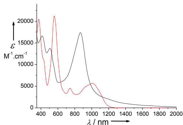
Figure 186: Spectres UV-vis-NIR de solutions à 0.51 mM dans CH 2 Cl 2 de [Co II (10) * ] (ligne rouge), et [Co(10)] + (ligne noire) généré par oxydation chimique par AgSbF 6 . T = 298 K, trajet optique = 1.000 mm.
