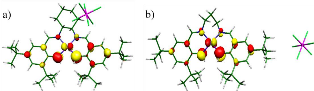
Figure 95: Représentation de la SOMO des complexes [\text{Ni}(\text{1}_{\text{N}_4}^{\text{tBu}})]^{*+} et [\text{Ni}(\text{4}_{\text{N}_4}^{\text{tBu}})]^{*+} .
