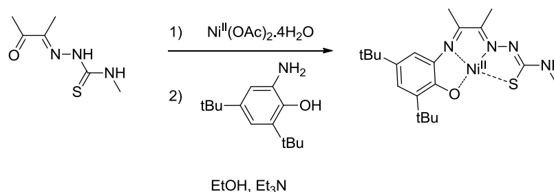
Figure 113: Synthèse par effet gabarit du complexe [Ni(7)].
