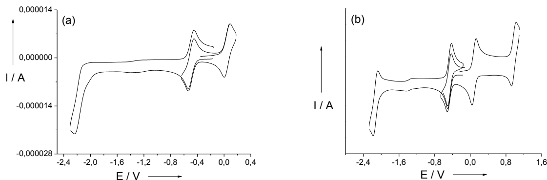
Figure 132: Courbes de voltamétrie cyclique de solutions à 0.5 mM des complexes [Ni(10)•] a) et [Cu(10)•] b) dans CH 2 Cl 2 contenant 0.1 M TBAP. Vitesse de balayage : 0.1 V.s -1 , T=298 K. Les potentiels sont donnés par rapport au couple de référence Fc + /Fc.
