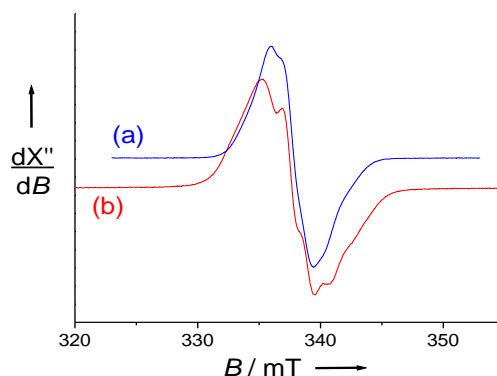
Figure 158: Spectres RPE en bande X de solutions à 0.5 mM dans \text{CH}_2\text{Cl}_2 (+ 0.1 M TBAP) des dications générés par électrochimie a) [\text{Co}(\text{1}^{\text{OMe}})]^{2+} et b) [\text{Co}(\text{1}^{\text{tBu}})]^{2+} . Freq. Microonde: 9.45 GHz; Puissance: 5.5 mW; Amp. Mod. 0.1 mT, Freq. 100 KHz. T = 100 K.
