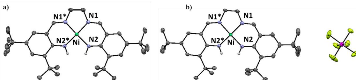
Figure 94: Structure cristallographique de a) [\text{Ni}(\text{5}_{\text{N4}}^{\text{tBu}})] et b) [\text{Ni}(\text{5}_{\text{N4}}^{\text{tBu}})]^{+\cdot} (ellipsoïdes à 30 %).
