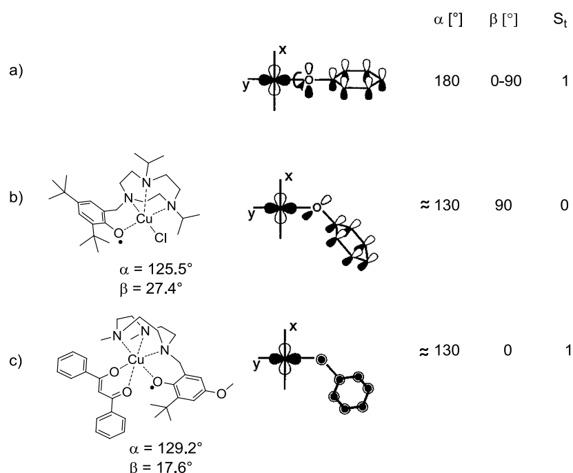
Figure 16: Orientations relatives des orbitales magnétiques de l'ion \text{Cu}^{\text{II}} d_{x^2-y^2} dans le plan x,y relatif à celui de l'orbitale \pi à demi occupée du radical phénoxye. 54
