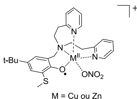
Figure 195: Représentation des complexes [\text{Cu}^{\text{II}}(\text{L})\cdot(\text{NO}_3)]^+ et [\text{Zn}^{\text{II}}(\text{L})\cdot(\text{NO}_3)]^+ .
