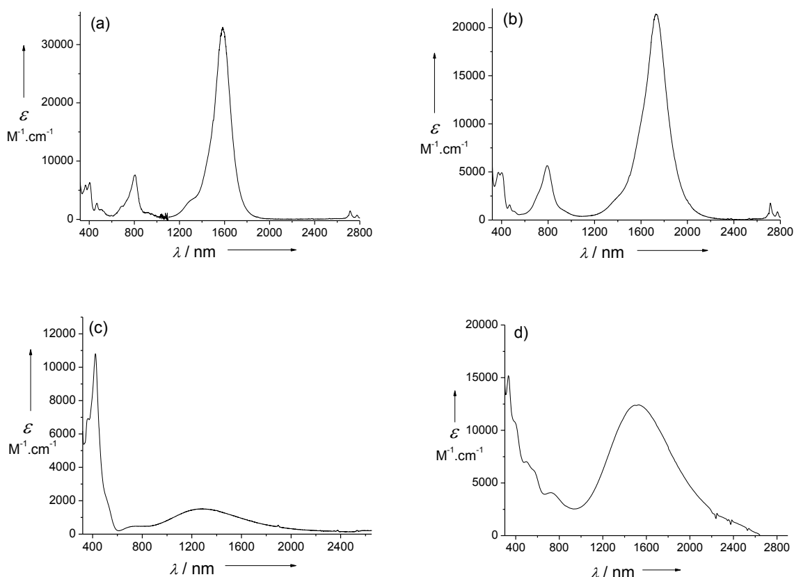
Figure 98: Spectres électroniques de solutions à 0.05 mm des complexes monoxydés générés chimiquement par oxydation des complexes neutres par un sel d' \text{AgSbF}_6 a) [\text{Ni}(\text{1}_{\text{N}_4}^{\text{tBu}})]^+ \cdot \text{SbF}_6^- , b) [\text{Ni}(\text{4}_{\text{N}_4}^{\text{tBu}})]^+ \cdot \text{SbF}_6^- , c) [\text{Cu}(\text{1}_{\text{N}_4}^{\text{tBu}})]^+ \cdot \text{SbF}_6^- et d) [\text{Cu}(\text{4}_{\text{N}_4}^{\text{tBu}})]^+ \cdot \text{SbF}_6^- , à 298K dans \text{CH}_2\text{Cl}_2 anhydre.
