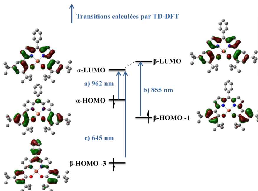
Figure 143: [\text{Cu}(10)^{\text{ox}}]^+ : Attribution des transitions calculées par TD-DFT ( S = \frac{1}{2} (ligand à couche fermé), fonctionnelle B3LYP, isovalue = 0.035)
