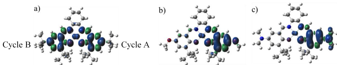
Figure 50 : Représentation de la densité de spin calculée pour: a) [\text{Ni}^{\text{II}}(\text{1}^{\text{tBu}})\cdot]^+ , b) [\text{Ni}^{\text{II}}(\text{1}^{\text{OMe}})\cdot]^+ , et c) [\text{Ni}^{\text{II}}(\text{1}^{\text{NMe}_2})\cdot]^+ en utilisant la fonctionnelle CAM-B3LYP.
