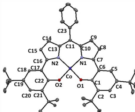
Figure 182: Structure cristallographique du complexe monoxydé [ \text{Co}^{\text{II}}(10) ] (ellipsoïdes à 30 %). Pour plus de clarté, les atomes d'hydrogène sont omis.
