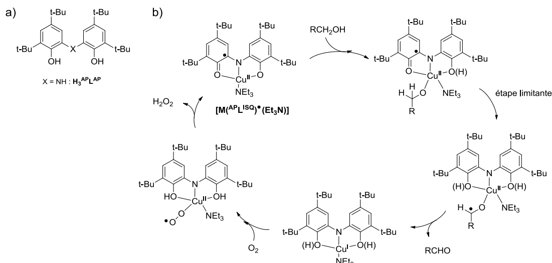
Figure 197: a) Ligand H_3^{APL^{AP}} et b) mécanisme proposé pour l'oxydation catalytique d'alcools primaires par [Cu^{II}(APL^{ISQ})\cdot(NEt_3)] . Les protons sont placés arbitrairement pour les intermédiaires réactionnels non caractérisés au niveau structural.
