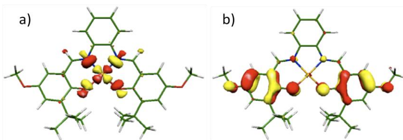
Figure 62: Localisation des SOMOs (a) centrées sur le métal et b) sur le ligand) dans le complexe [\text{Cu}(\text{2}^{\text{OMe}})\cdot]^+
