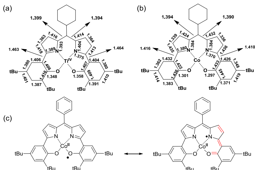
Figure 183 : Longueurs de liaison dans le complexe a) [\text{Ti}^{\text{IV}}(10)(\text{Cl})(\text{THF})] (cette représentation omet la coordination des ligands axiaux, avec une erreur de \pm 0.01 Å), b) [\text{Co}(10)] (erreur de \pm 0.005 Å) et c) représentation de deux formes mésomères de [\text{Co}^{\text{II}}(10)^{\bullet}] (liaisons possédant un caractère double liaison en rouge).
