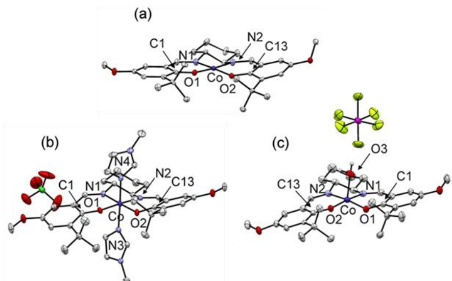
Figure 147: Structures cristallographiques obtenues par diffraction des rayons X de (a) [\text{Co}(\mathbf{1}^{\text{OMe}})] ; (b) [\text{Co}(\mathbf{1}^{\text{OMe}})(\text{im})_2]^+ ; (c) [\text{Co}(\mathbf{1}^{\text{OMe}})]^+ (ellipsoïdes à 30 %). Les atomes d'hydrogène sont omis à l'exception de la molécule d'eau coordonnée dans [\text{Co}(\mathbf{1}^{\text{OMe}})]^+ .
