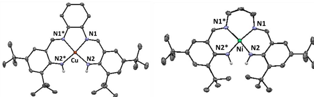
Figure 85: Structure cristallographique par diffraction des rayons X de [Cu(1 N4 tBu )] et [Ni(4 N4 tBu )] (ellipsoïdes à 30 %).
