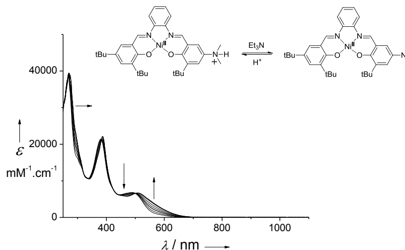
Figure 70: Titrage de [\text{Ni}(3\text{H})]^+ (0.05 mM dans \text{CH}_2\text{Cl}_2 ) par 0 à 1 équivalent molaire de \text{Et}_3\text{N} (2.5 mM). Les flèches indiquent les changements du spectre lors de l'ajout de \text{Et}_3\text{N} . T = 298 K, l = 1.000 cm.
