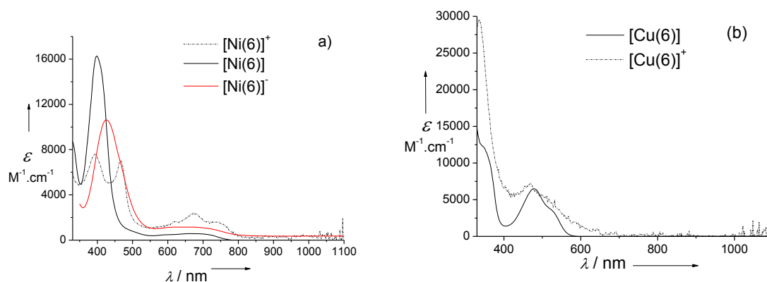
Figure 104: Spectres électroniques de solutions à 0.05 mM des complexes a) [Ni(6)] (ligne noire), [Ni(6)] + (ligne en pointillés) et [Ni(6)] - (ligne rouge) et b) [Cu(6)] (lignes noires), [Cu(6)] + (lignes en pointillés). Espèces monoxydées
