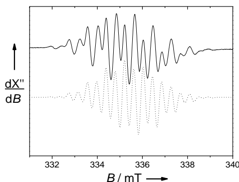
Figure 74: Spectre RPE isotrope d'une solution à 1 mM dans \text{CH}_2\text{Cl}_2 (contenant 0.1 M TBAP) de [\text{Ni}(3')]^+ . Ligne pleine: spectre expérimental, ligne en pointillés: simulation réalisée en utilisant les paramètres donnés dans le texte. T = 223 \text{ K} , fréquence microonde 9.42 GHz, puissance 20 mW, modulation de fréquence 100 KHz, amplitude 0.1 mT.
