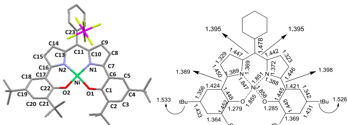
Figure 133: Structure cristallographique du complexe dioxydé [\text{Ni}(10)]^+ \cdot \text{SbF}_6^- (ellipsoïdes à 30 %) et analyse des longueurs de liaison en Å (avec une erreur de \pm 0.01 Å).
