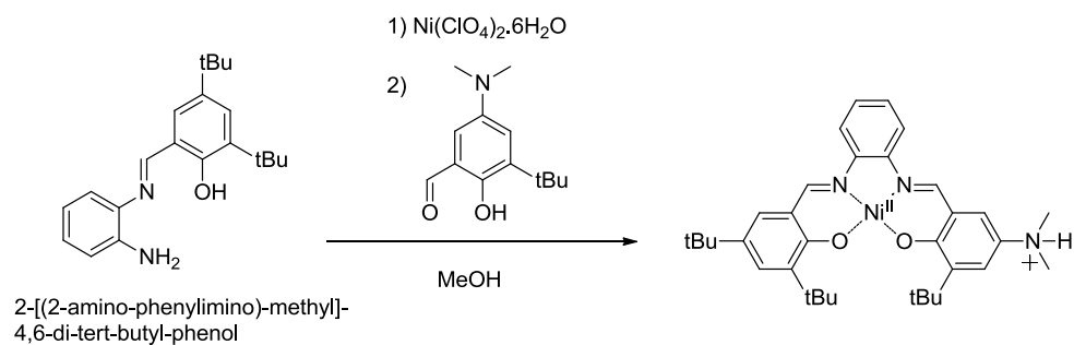
Figure 69: Synthèse de [\text{Ni}(3\text{H})]^+ .
