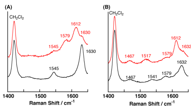
Figure 54: Spectres de Résonance Raman des complexes [\text{Ni}^{\text{II}}(\text{1}^{\text{OMe}})] (A) et [\text{Ni}^{\text{II}}(\text{1}^{\text{NMe2}})] (B) et de leurs espèces monoxydées enregistrés à la longueur d'onde d'excitation \lambda_{\text{ex}} = 413.1 \text{ nm} à -60 \text{ }^{\circ}\text{C} . Lignes noires : complexes neutres, lignes rouges : complexes monoxydés.
