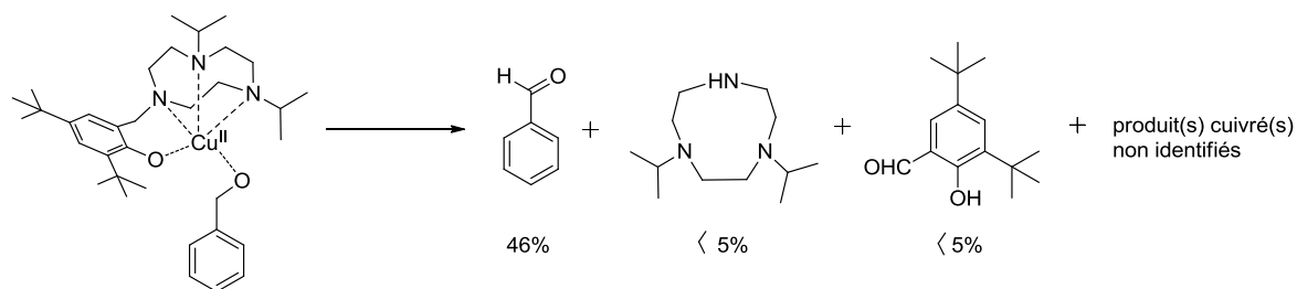
Figure 194: Produits résultant de l'électrolyse de [\text{Cu}^{\text{II}}(\text{L})(\text{OCH}_2\text{Ph})] .
