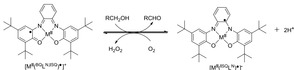
Figure 198: Mécanisme proposé pour l'oxydation catalytique d'alcools primaires par [M^{II}(BQL^{N,ISQ})\cdot]^+ .
