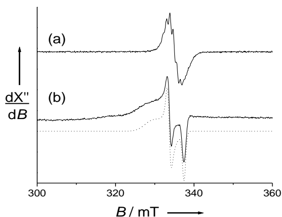
Figure 73: Spectres RPE en bande X de solution à 1mM dans \text{CH}_2\text{Cl}_2 (contenant 0.1 M TBAP) de (a) [\text{Ni}(3)]^{2+} et (b) [\text{Ni}(3\text{H})]^{2+} . Les lignes pleines représentent les spectres expérimentaux, la ligne en pointillé représente la simulation réalisée en utilisant les paramètres donnés dans le texte. T = 100 K, fréquence microonde 9.42 GHz, puissance 20 mW, modulation de fréquence 100 KHz, amplitude 0.04 mT (a) et 0.16 mT (b).
