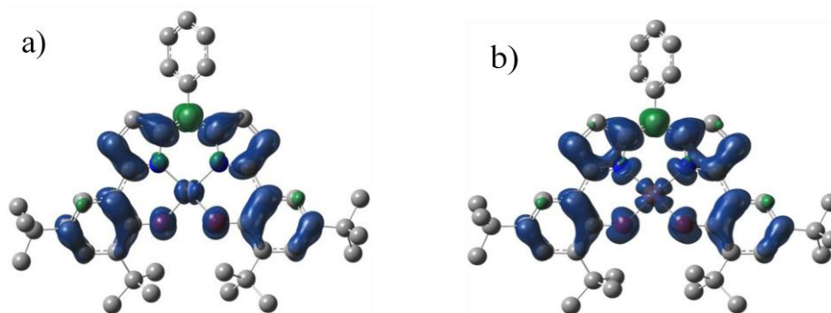
Figure 130: Localisation de la densité de spin calculée dans les complexes a) [Ni II (10) • ] et b) [Cu II (10) • ]
