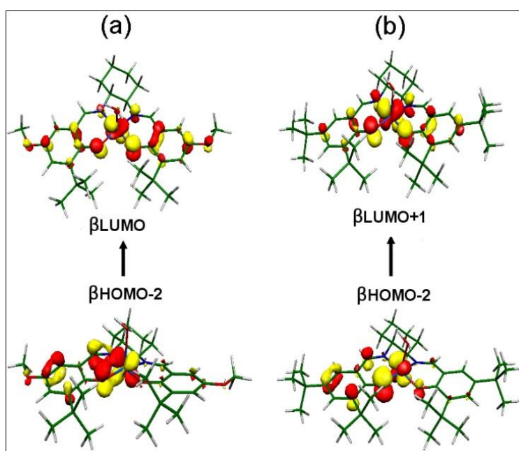
Figure 156: Attribution de la nature de la transition à plus basse énergie par TD-DFT dans (a) [\text{Co}(\text{1}^{\text{OMe}})]^+ et (b) [\text{Co}(\text{1}^{\text{tBu}})]^+ .
