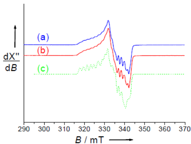
Annexe 4: spectre RPE en bande X de (a) [Co(1 OMe )] (bleu) et (b) [Co(1 tBu )] (rouge) en solution à 0.5 mM dans CH 2 Cl 2 +10 équivalents de N -méthylimidazole après 30 sec. (c) Simulation en utilisant les paramètres : g_x = 2.013 , g_y = 2.083 , g_z = 1.990 , Euler angle 20 ° (tenseur g ), A_x = 25 MHz, A_y = 56 MHz, A_z = 27 MHz. Conditions: fréquence, 9.45 GHz; puissance, 7 mW; modulation de fréquence, 100 kHz; amplitude, 0.1 mT; T = 100 K.
