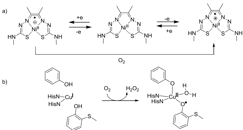
Figure 109: a) Différentes formes redox du complexe [\text{Ni}(\text{6})] et b) oxygénation de la GO réduite.
