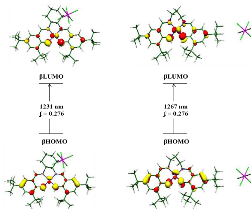
Figure 99: Attribution par TD-DFT de la transition dans le proche IR pour [\text{Ni}(1\text{N}_4^{\text{tBu}})]^+ et [\text{Ni}(4\text{N}_4^{\text{tBu}})]^+ .
