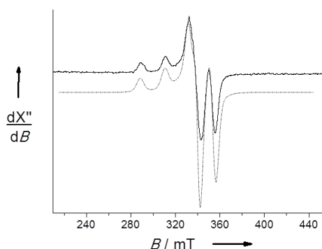
Figure 88 : Spectres RPE en bande X d'une solution à 0.5 mM dans \text{CH}_2\text{Cl}_2 anhydre de [\text{Cu}(\text{1N}_4^{\text{tBu}})] à 12 K. Le spectre en pointillés représente la simulation du spectre en utilisant les paramètres g_1 = 2.292 , g_2 = 2.03 et g_3 = 1.96 .
