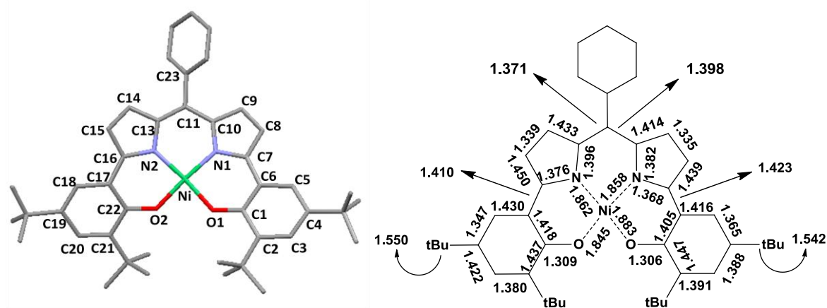
Figure 127: Structure cristallographique et analyse des longueurs de liaison en Å (avec une erreur de \pm 0.01 Å) dans le complexe [\text{Ni}(10)^{\bullet}] (ellipsoïdes à 30 %).
