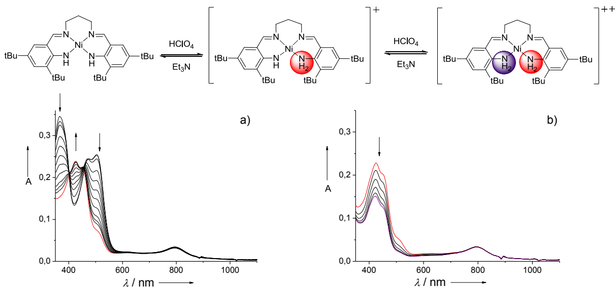
Annexe 2: Titrage du complexe neutre [\text{Ni}(\mathbf{4}_{\text{N}_4}^{\text{tBu}})] (0.05 mM dans \text{CH}_2\text{Cl}_2 ) par une solution de \text{HClO}_4 (0.005 M dans \text{CH}_3\text{CN} ) de 0 jusqu'à 1 équivalent a) puis jusqu'à 2 équivalents b). Trajet optique 1.000 cm T = 298K. Les flèches indiquent l'évolution du spectre lors de l'ajout d'acide.
