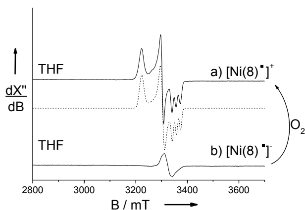
Figure 121 : Spectres RPE en bande X de solution à 4 mM enregistrés à 100K dans le THF : b) [\text{Ni}(8)^{\bullet-}] (réduit chimiquement par NaHg en boîte à gant) et a) du même échantillon exposé 2 minutes à l'oxygène. Le spectre en pointillé représente la simulation du spectre a) en utilisant les paramètres détaillés dans le texte.
