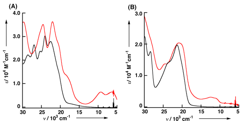
Figure 63: Spectres électroniques des complexes neutres (lignes noires) et monoxydés générés par oxydation chimique (lignes rouges): (A) [Cu(OMe) 2 ] et [Cu(OMe) 2 ] •+ , (B) [Cu(2OMe)] et [Cu(2OMe)] •+
