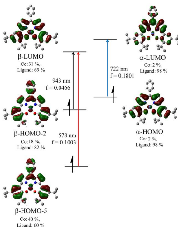
Figure 187: [\text{Co}^{\text{II}}(10)^{\bullet}] : Attribution des transitions calculées par TD-DFT ( S = 1 , fonctionnelle B3LYP)
