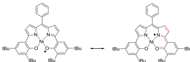
Figure 129: Deux formes mésomères de [\text{Ni}^{\text{II}}(10)^{\bullet}] (liaisons possédants un caractère double liaison en rouge).
