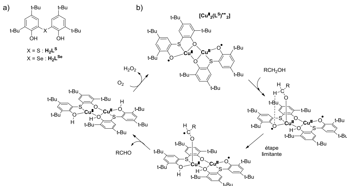
Figure 196 : a) ligands H_2L^S et H_2L^{Se} et b) mécanisme proposé pour l'oxydation catalytique d'alcools primaires et secondaires par [Cu_2^{II}(L^S)^{\bullet\bullet}_2]^{2+} .
