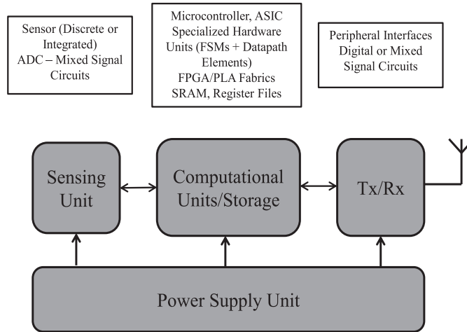
FIGURE 1: Un réseau de capteurs typique.
