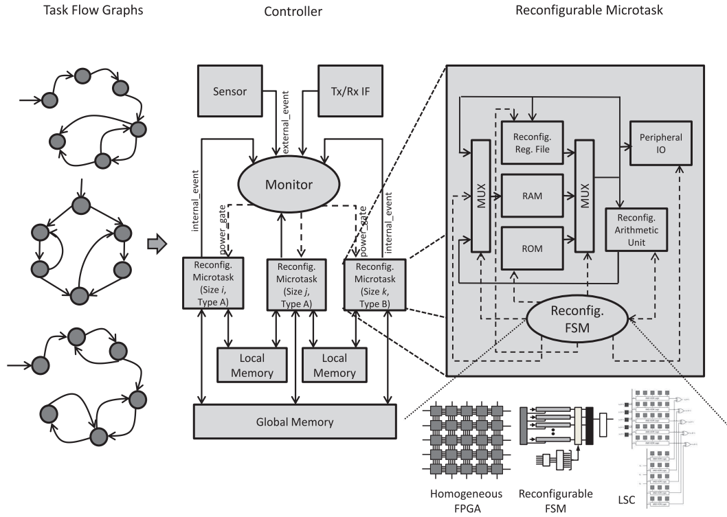
FIGURE 5: Structure d'un contrôleur flexible pour micro-tâche reconfigurable.
