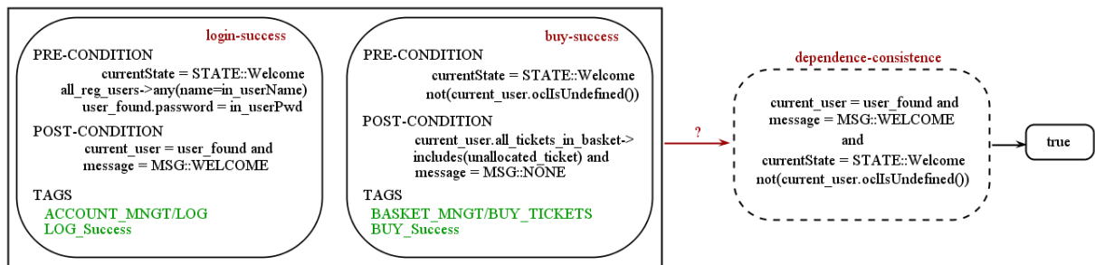
FIGURE 7.6 – Dépendance positive dans le cas d' eCinema
