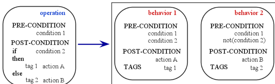
FIGURE 7.1 – Transformation d'une opération en comportements
