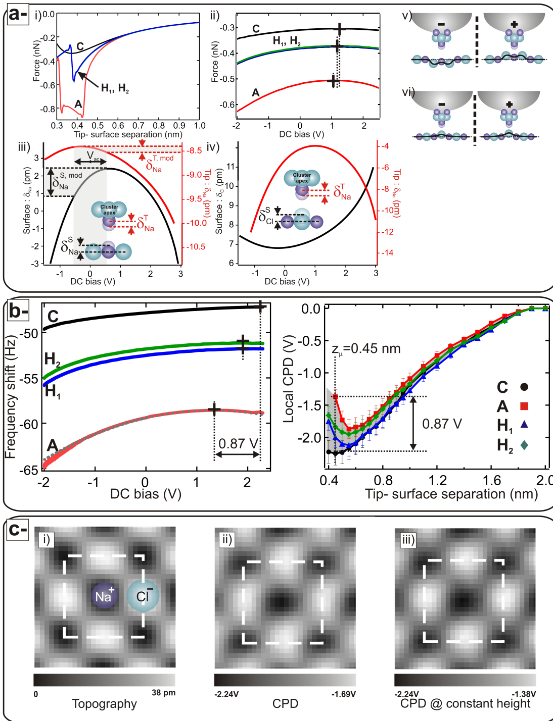
FIGURE 59: a- Données du champ de force ab initio. i) Force en fonction de la distance au-dessus de chacun des sites (A=Anion, C=Cation, H 1,2 =points de selle) montrés en figure 54c-. ii) Évolution de la force au-dessus de chacun de ces sites en fonction du bias. Les courbes sont déduites pour une hauteur de la pointe de 4,5 Å. iii) Déplacements des ions interfaciaux (ion Na + en position apicale sur la pointe en face d'un cation de la surface) en fonction du bias appliqué. iv) Mêmes types de courbes, mais pour le Na + de la pointe placé au-dessus d'un anion. v) et vi) Schémas illustratifs. b- Gauche : Courbes spectroscopiques \Delta f vs. bias calculées avec le simulateur nc-AFM/KPFM à partir du champ de force ab initio au-dessus des quatre sites particuliers de la surface. Droite : CPD déduit des précédentes courbes (position des extrema) en fonction de la distance. c- Images calculées avec le simulateur à partir du champ de force ab initio. i) et ii) Images topographique (contraste vertical \approx 40 pm, typique des valeurs expérimentales) et CPD (contraste vertical \approx 0,55 V) calculées à 4,5 Å au-dessus de la surface. Les données spectroscopiques prédisent un contraste CPD de 0,87 V. En faisant une image à hauteur constante, l'image CPD donne 0,87 V (iii). Dans le régime courte portée, le régulateur de distance influence les mesures de CPD.
