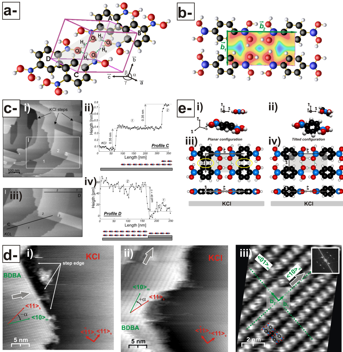
FIGURE 43: a - Organisation de BDDBA dans le cristal moléculaire 3D. Le cristal est constitué de feuillets 2D de molécules liées par liaisons H. b - Configuration la plus stable du film moléculaire 2D auto-soutenu calculé en DFT. La structure, liée par liaisons H, est proche de celle des feuillets moléculaires du cristal. La maille est rectangulaire, de paramètres b_1 = 5,2 \text{ \AA} et b_2 = 10,0 \text{ \AA} . c - Images topographiques grand champ de BDDBA sur KCl(001). Les images montrent des domaines mono-couche. La hauteur apparente d'une monocouche déduite des divers profils est de 350 pm, ce qui est compatible avec la hauteur entre feuillets dans le cristal moléculaire (370 pm). d - Images haute résolution d'une monocouche de BDDBA sur KCl(001) laissant apparaître l'organisation structurale de la couche et l'orientation du substrat. Les calculs DFT de la couche auto-soutenue sont compatibles avec les données expérimentales, ce qui confirme son caractère supramoléculaire (liaisons H). e - Modèle structural de la configuration d'adsorption des molécules. Une molécule en conformation planaire (i), rend impossible la formation de la monocouche par encombrement stérique (iii). Au contraire, une rotation du cycle benzénique central par rapport au plan des liaisons B(OH) 2 , permet le développement de la phase supramoléculaire 2D par liaisons H, ce qui est confirmé en DFT.
