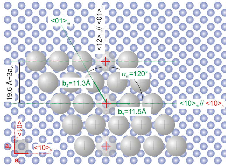
FIGURE 49: Modèle structural postulé pour HHTP/KBr(001), construit selon les paramètres structuraux déduits expérimentalement. On retrouve la maille moléculaire alignée sur la \langle 10 \rangle_s définissant l'épitaxie POL-IB (cf. texte).
