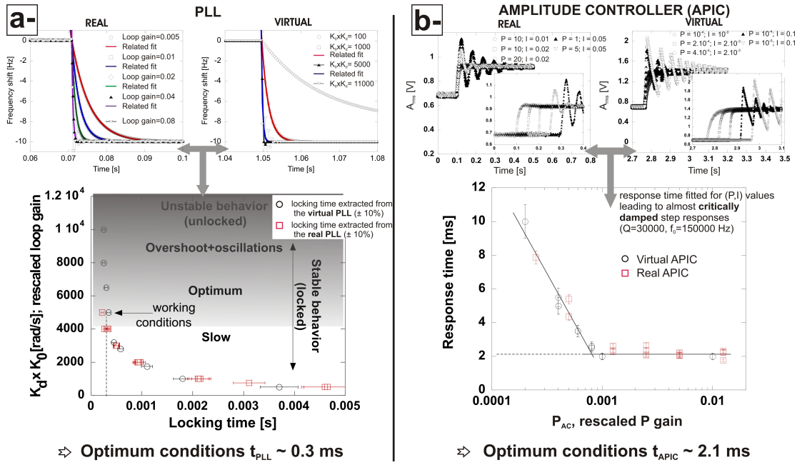
FIGURE 52: a- Comparisons des performances entre les PLL instrumentale et simulée. On a reporté en haut leurs réponses impulsionnelles à un échelon en \Delta f en fonction de leurs gains. En bas, on reporte la courbe maîtresse du temps de verrouillage des PLL déduite des mesures précédentes. En ajustant correctement les gains, les deux PLL présentent des caractéristiques dynamiques similaires. Le temps de verrouillage optimal des PLL (conditions expérimentales) est de 0,35 ms. b- Même type d’approche avec le régulateur d’amplitude. La constante de temps du régulateur est limitée à 2,1 ms à cause du détecteur d’amplitude (RMS-to-DC).
