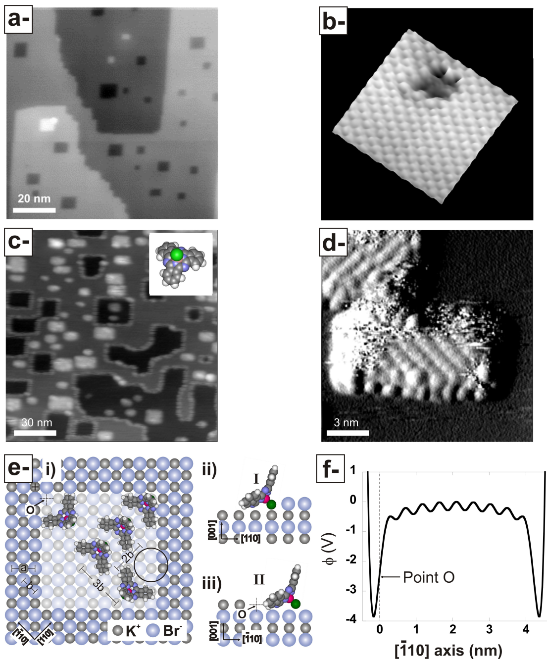
FIGURE 42: a- Image grand champ d'une surface de \text{KBr}(001) après irradiation électronique (1 keV, 1 s). La surface présente des lacunes régulières, profondes d'une monocouche de \text{KBr} non chargées. Elles résultent d'un processus de désorption stimulée connue avec les cristaux ioniques. b- Image haute résolution de l'une de ces lacunes de dimensions atomiques. c- Image grand champ de molécules de SubPC déposées sur le \text{KBr} irradié. Les domaines moléculaires tendent à se développer à l'intérieur des lacunes les plus petites, et uniquement là. d- Image haute résolution d'un domaine à l'intérieur d'une lacune qui laisse apparaître les arrangements moléculaires. Des molécules de deuxième couche, brouillent sporadiquement l'image. e- Schéma de la configuration d'adsorption des molécules. Les molécules se piègent dans le potentiel de Madelung qui se développe dans les lacunes. Il est probable qu'elles s'alignent avec le moment dipolaire vers le bas pointant dans le coin de la lacune contenant un halogène (i et ii). Ainsi, la configuration d'adsorption iii) est peu vraisemblable. Dans la lacune, elles interagissent entre elles via des interactions dipolaires. f- Potentiel de Madelung calculé qui se développe dans la lacune. Il est fortement accru dans les coins de celle-ci.
