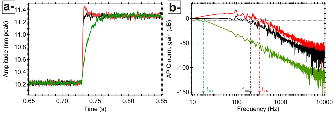
FIGURE 25: a -Réponse impulsionnelle du contrôleur d'amplitude à un échelon d'amplitude de consigne pour plusieurs couples de gains (P,I) caractéristiques des régimes d'amortissement sous-critique, critique et sur-critique (respectivement courbes rouge, noire et verte). Les gains du contrôleur sont toujours ajustés pour obtenir un régime d'amortissement critique (courbe noire). Le temps de réponse du contrôleur est alors de l'ordre de 2 ms. b -Réponse harmonique associée (module de la transformée de Fourier normalisée de la réponse impulsionnelle), en représentation monolatérale. On n'a pas reporté la phase de la transformée de Fourier. L'inverse de la fréquence de coupure à -3 dB donne aussi une estimation du temps de réponse du contrôleur. Dans le régime d'amortissement critique (courbe noire) f_{-3dB} \simeq 200 ms, on a la réponse la plus rapide qui assure le fonctionnement linéaire du contrôleur.
