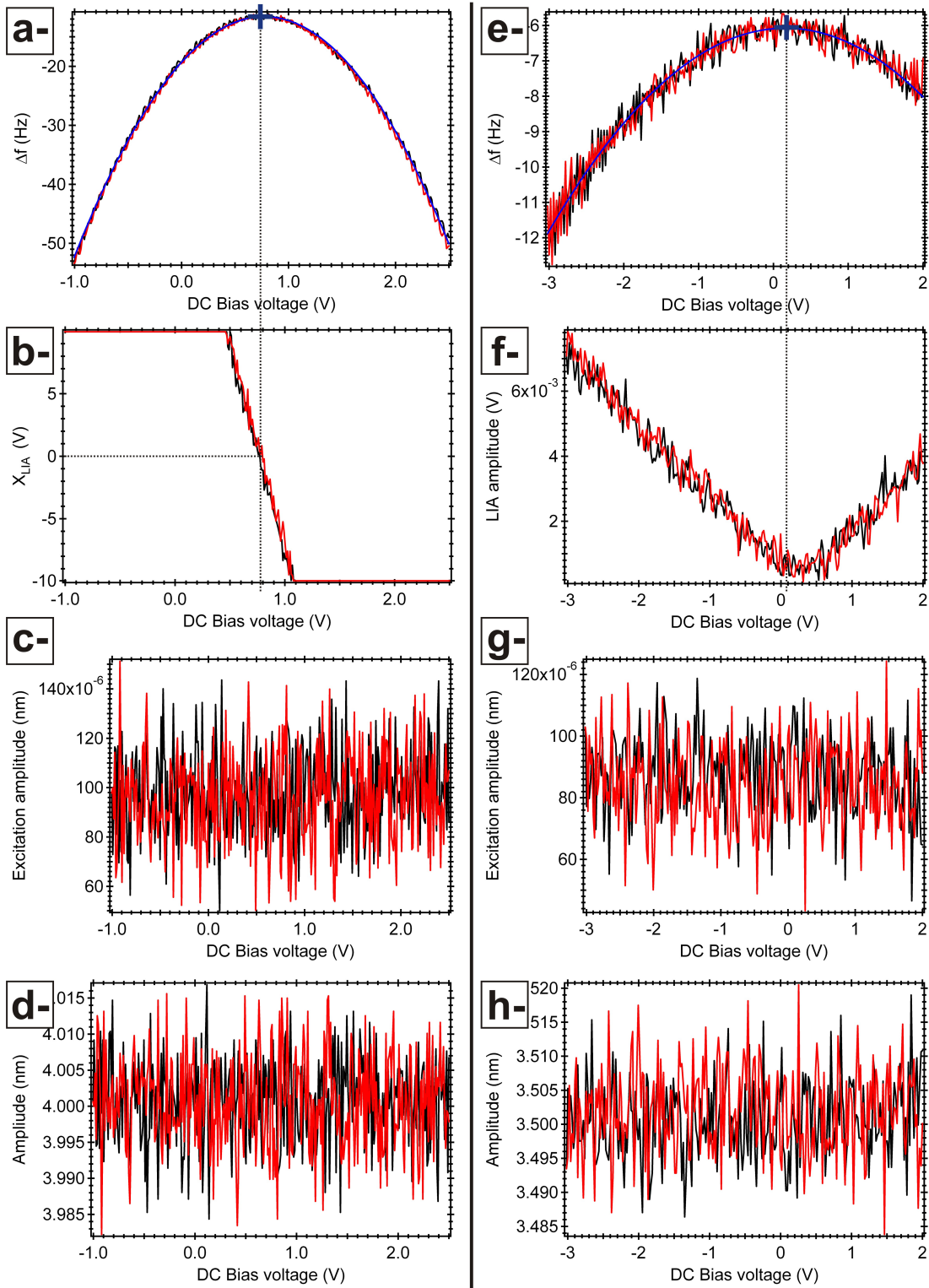
FIGURE 32: Courbes spectroscopiques de bias mesurées sur HOPG (a- à d-) et NaCl (e- à h-). On a reporté, \Delta f (a-, e-), le signal X (b-) et R (f-) de la détection synchrone, l'amplitude d'excitation (c-, g-) et l'amplitude d'oscillation (d-, h-). Les courbes de \Delta f sont ajustées avec une fonction parabolique (courbe bleue) dont le maximum donne la valeur du CPD. Pour HOPG, on a +0,77 V, pour NaCl, +0,16V.
