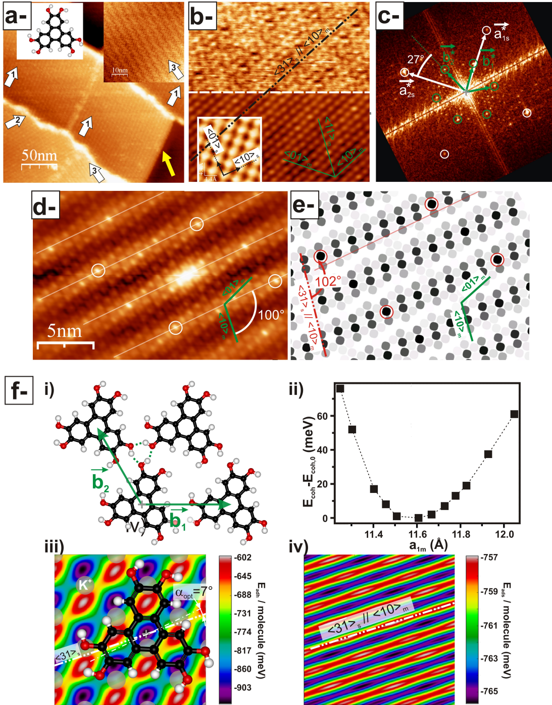
FIGURE 44: a -Image grand champ de HHTP (inset à gauche) sur \text{KCl}(001) . Les domaines moléculaires se développent sur les terrasses avec quatre directions équivalentes sous forme de franges de Moiré (inset à droite). b -Image haute résolution d'un domaine moléculaire (partie supérieure) et autocorrélation de la partie inférieure montrant le réseau hexagonal d'HHTP. L'inset est l'image de l'orientation du substrat dont on déduit l'épitaxie LOL \langle 31 \rangle_s (cf. texte). c - FFT d'une image expérimentale (non reportée) avec l'orientation du substrat (spots blancs) et du domaine moléculaire (spots verts) qui confirme l'épitaxie LOL. d - et e - Image expérimentale autocorrélée d'un domaine moléculaire avec des franges de Moiré et simulation validant l'hypothèse de quasi-coïncidences entre le réseau moléculaire et le substrat. f - Considérations énergétiques. i ) Réseau auto-supporté calculé en DFT. Il est 4 % plus grand que celui observé expérimentalement. ii ) Evolution de l'énergie de cohésion du film calculé en DFT en fonction d'une compression uniaxiale. Une compression de 4 % est défavorable. iii ) Configuration d'adsorption d'une seule molécule sur la surface calculée en Potential Energy (énergie d'adhésion \approx -1 eV). iv ) Energie d'adsorption d'un cluster de 3600 molécules qui confirme l'épitaxie.
