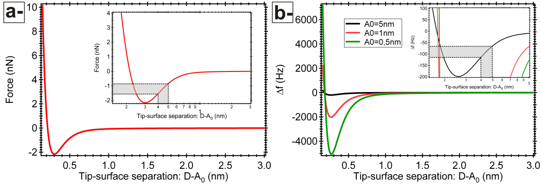
FIGURE 16: a -Force d'interaction pointe-surface en fonction de la distance z_{\mu} = D - A_0 . Les paramètres utilisés pour la calculer sont indiqués dans le texte. L'axe des abscisses de l'inset est en échelle log. b - \Delta f déduit de la courbe de force précédente (équation 15) pour A_0 = 5, 1 et 0,5 nm (courbes respectivement noire, rouge et verte). Les autres paramètres de l'oscillation sont f_0 = 150 kHz, k_0 = 30 N/m et Q = 40000 . L'inset permet de mieux voir les variations du \Delta f pour A_0 = 5 nm dans une gamme de distances inférieures au nm (échelle log). La variation rapide du \Delta f dans cette zone explique la grande sensibilité de la technique.
