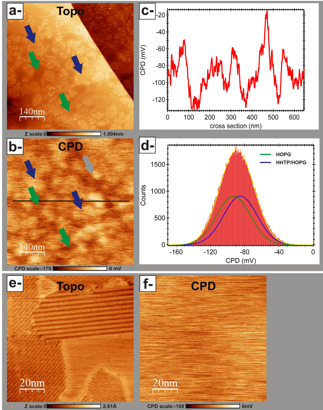
FIGURE 31: a- & b-Images topographique et CPD ( F_N -FM-KPFM, f_K = 3456 Hz, V_{ac} = 0,5 V) de HOPG avec 1/3 de monocouche de molécules d'HHTP dessus : 700 \times 700 nm 2 , A_0 = 2,4 nm, \gamma = -0,016 nN. \sqrt{\text{nm}} . Le contraste vertical de CPD est de 150 mV. La marche du substrat est un peu visible dans le CPD (flèche grise). Les domaines moléculaires présentent un CPD plus faible que celui mesuré sur le substrat (flèches bleues vs. vertes). c -Section le long de la ligne en b . d -Histogramme de l'image CPD et ajustement gaussien (courbe jaune). Les deux types de contrastes (domaines moléculaires/substrat) peuvent être ajustés avec deux gaussiennes (courbes bleue et verte, respectivement) indiquant une CPD de l'ordre de -85 mV pour les molécules et -93 mV pour le substrat. La courbe jaune est la superposition des courbes gaussiennes précédentes. e- & f -Images topographique et CPD du même échantillon : 100 \times 100 nm 2 , A_0 = 2,4 nm, \gamma = -0,028 nN. \sqrt{\text{nm}} .
