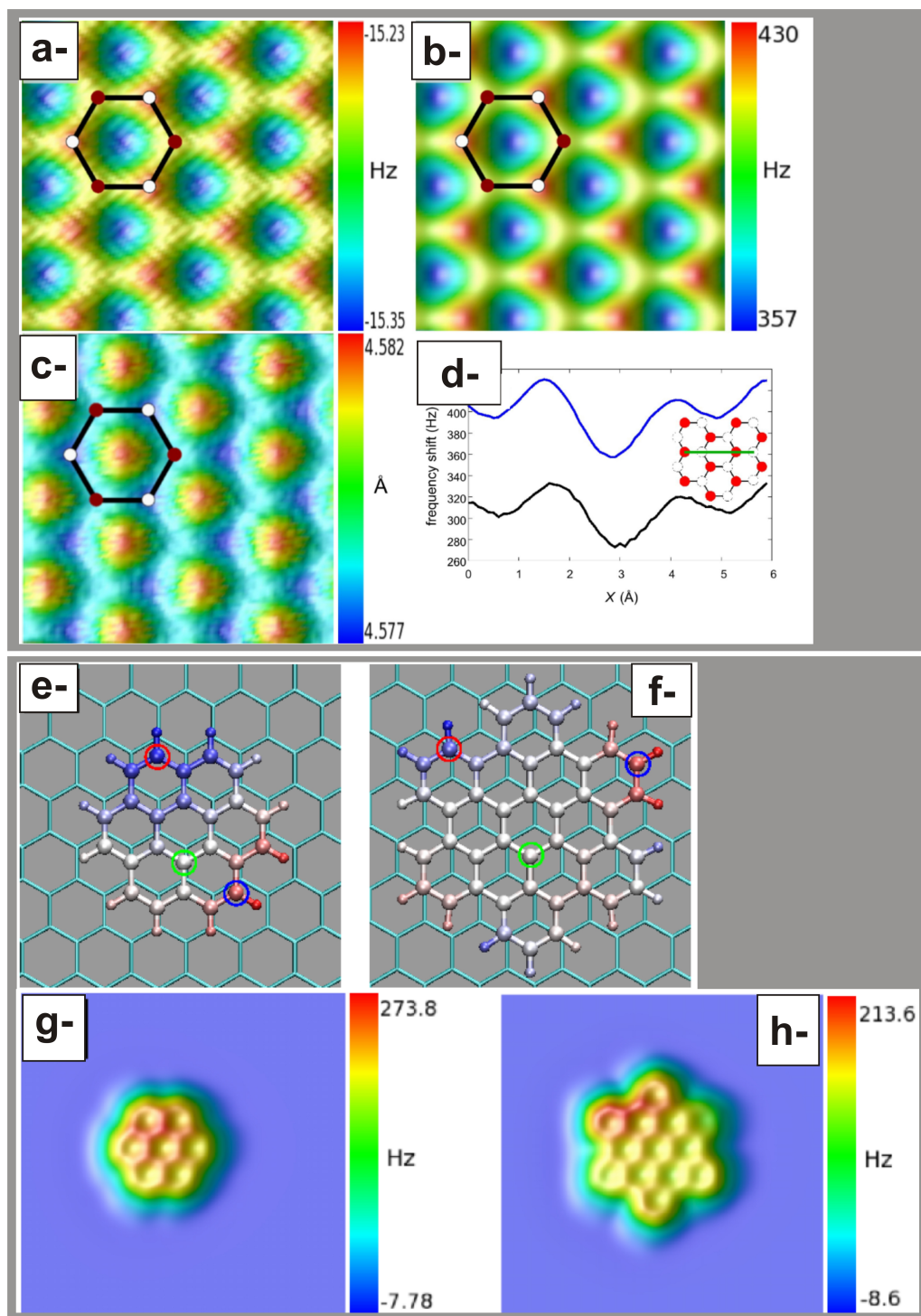
FIGURE 53: a-d- Images simulées d'une surface de graphite en mode tuning fork, d'après [32]. a-Image à hauteur constante du graphite ( z = 4,3 \text{ \AA} ). b- Même chose qu'en a-, sauf z = 2,75 \text{ \AA} . c- Image du graphite à \Delta f = -13 \text{ Hz} constant. La taille des image est 9 \times 9 \text{ \AA}^2 . d- Coupe selon la ligne indiquée en inset dans l'image à hauteur constante ( z = 2,75 \text{ \AA} ). e-h- D'après [33]. e- et f- Configuration d'adsorption d'une molécule de coronène (e-) et d'hexabenzocoronène (f-) sur graphite calculées à partir de potentiels empiriques. L'échelle de couleur traduit la hauteur des atomes par rapport à la surface située en z = 0 . Du rouge au bleu : 3,10 - 3,19 \text{ \AA} . g- et h- Images à hauteur constante ( z = 6,065 \text{ \AA} ) des mêmes molécules (g-coronène, h-hexabenzocoronène) sur graphite en mode tuning fork calculées avec le simulateur. La taille des images est de 2,59 \times 2,59 \text{ \AA}^2 . L'apex de la pointe utilisée pour tous les calculs est constituée d'un cluster de 87 atomes de carbone en configuration cristalline type diamant. Bien que la hauteur d'imagerie corresponde à un régime non-contact dominant (cf. zones de \Delta f négatif), la pointe vient sonder le régime répulsif très courte portée sur la molécule (cf. zones de \Delta f positif), à l'origine du contraste intra-moléculaire.
