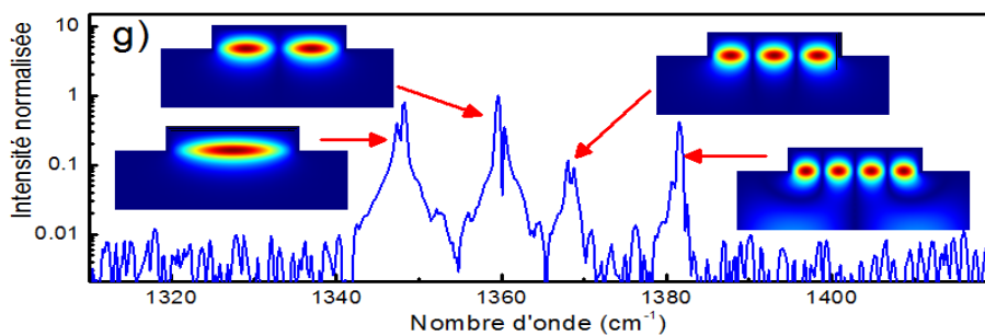
Figure 2-46 : spectres de laser à contre réaction répartie émettant à 7.4\mu\text{m} avec une cavité de largeur 20\mu\text{m} et une longueur de 2mm. Les différents encarts représentent la cartographie des modes latéraux obtenus par éléments finis. Les indices effectifs obtenus par simulation correspondent aux mesures.
