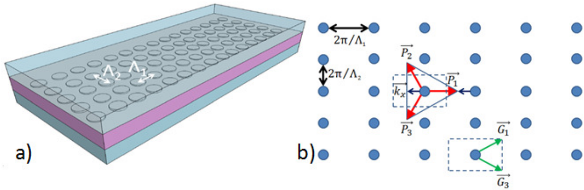
Figure 3-4 : a) schéma d'un laser avec une cohérence transverse, la périodisation dans l'axe perpendiculaire à l'axe de propagation dans la cavité permet de favoriser le mode fondamental TM_{00} . b) Mécanisme de couplage dans l'espace réciproque : le vecteur d'onde \vec{P}_1 est couplé aux vecteurs d'onde \vec{P}_2 et \vec{P}_3 quand il y a accord de phase \vec{P}_1 - \vec{P}_2 = \vec{G}_1 (l'accord \vec{P}_1 - \vec{P}_3 = \vec{G}_3 étant automatiquement satisfait). \vec{G}_1, \vec{G}_3 = 2\pi/\Lambda_1 \vec{i} \pm 2\pi/\Lambda_2 \vec{j} .
