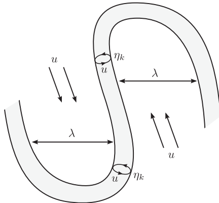
FIGURE 5.2 – Structure de l'écoulement à petite échelle, d'après le modèle de Tennekes [110].
