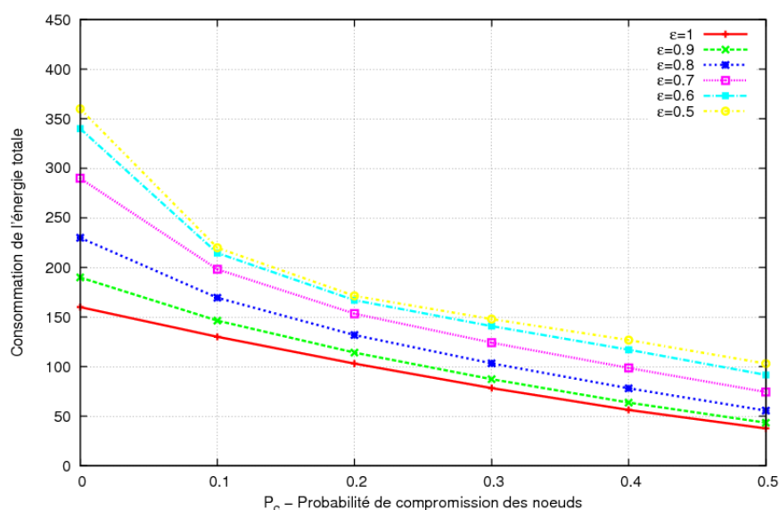
FIGURE 6.13: Consommation d'énergie totale en cas d'attaque : avec 2 réplifications
