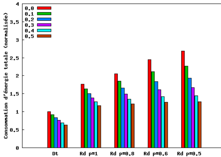
FIGURE 5.14: Consommation totale d'énergie (normalisée par GBR-Dt sans réplication) en cas d'attaque Selective forwarding : avec répliquions uniformes.
