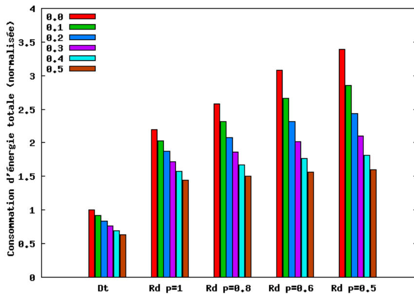
FIGURE 5.15: Consommation totale d'énergie (normalisée par GBR-Dt sans réplication) en cas d'attaque Selective forwarding : avec répliquions adaptatives.
