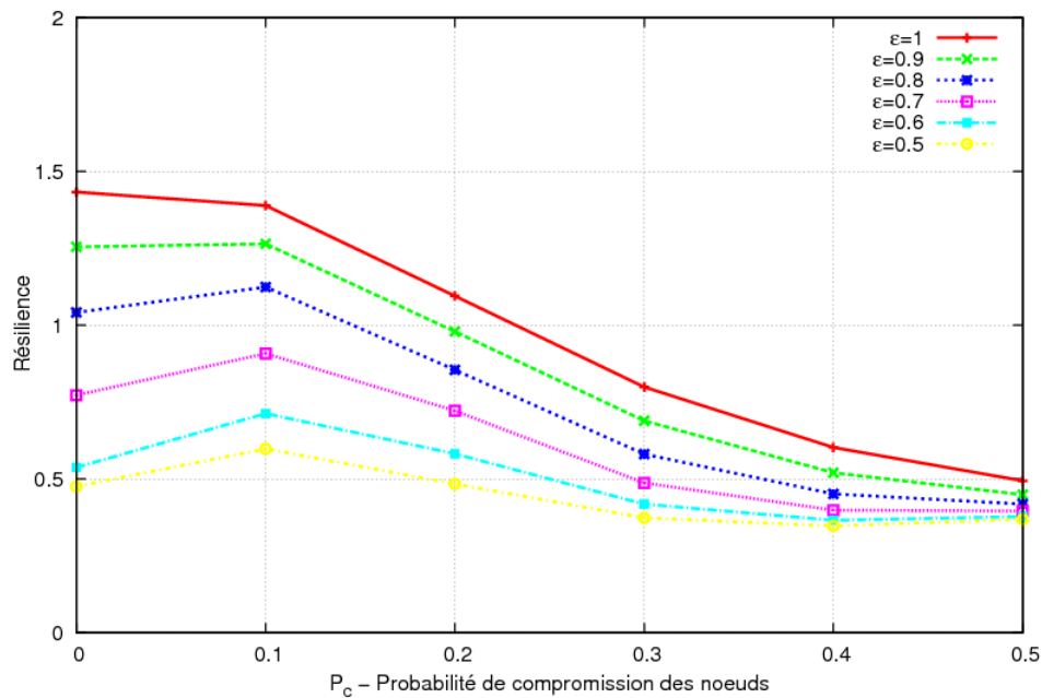
FIGURE 6.22: Résilience des marches aléatoires biaisées avec répliquions adaptatives.
