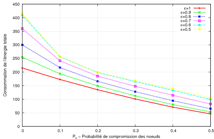
FIGURE 6.16: Consommation d'énergie totale en cas d'attaque : avec réplifications adaptatives
