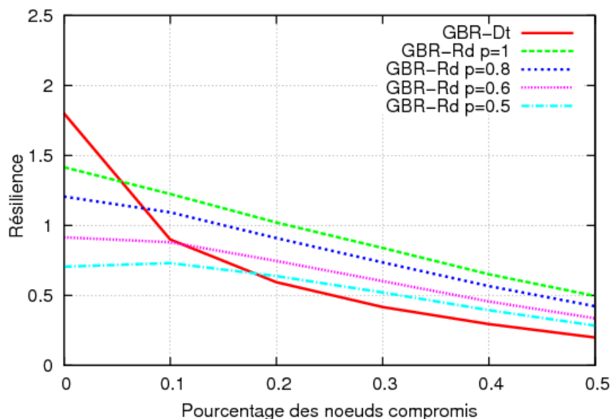
FIGURE 5.24: Résilience en cas d'attaque Sybil : avec réplifications adaptatives.
