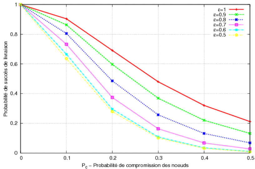
FIGURE 6.15: Succès de livraison moyen en cas d'attaques ( P_c ) : avec réplifications adaptatives
