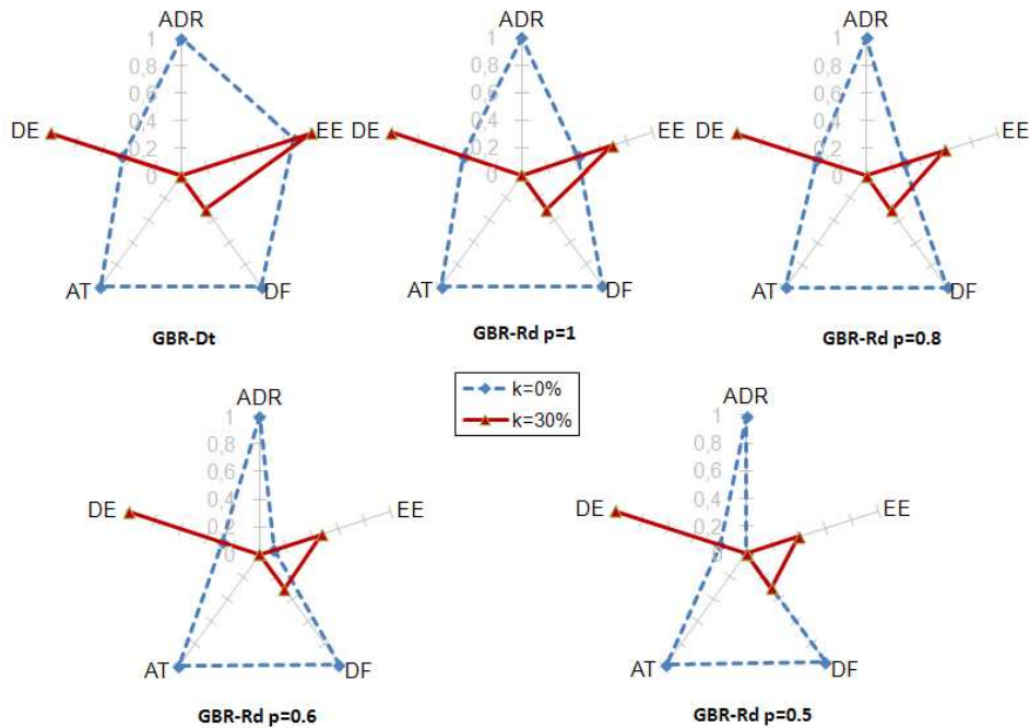
FIGURE 5.33: Surface de résilience en cas d'attaque Sinkhole : avec répliquions adaptatives.
