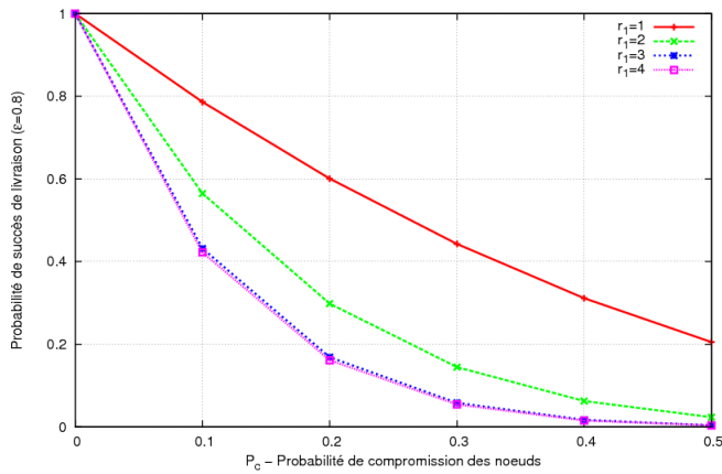
FIGURE 6.4: Succès de livraison d'un nœud à la position r_1 en cas d'attaque ( P_c ).
