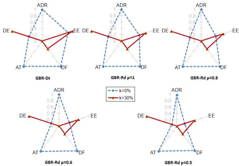
FIGURE 5.32: Surface de résilience en cas d'attaque Sinkhole : avec répliquions uniformes.
