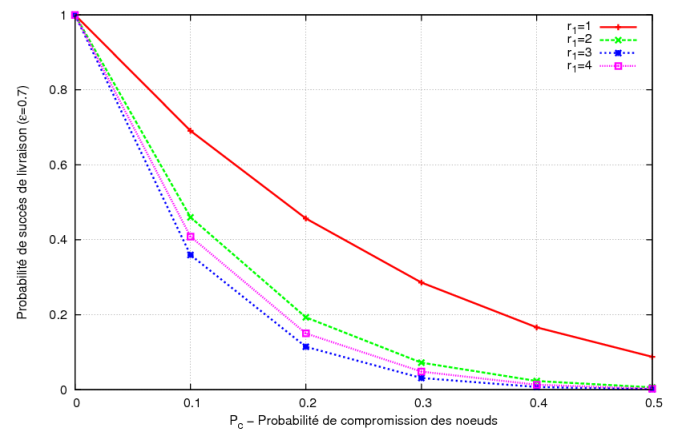
FIGURE 6.4: Succès de livraison d'un nœud à la position r_1 en cas d'attaque ( P_c ).
