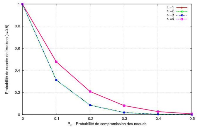
FIGURE 6.5: Succès de livraison d'un nœud à la position r_1 en cas d'attaque ( P_c ).
