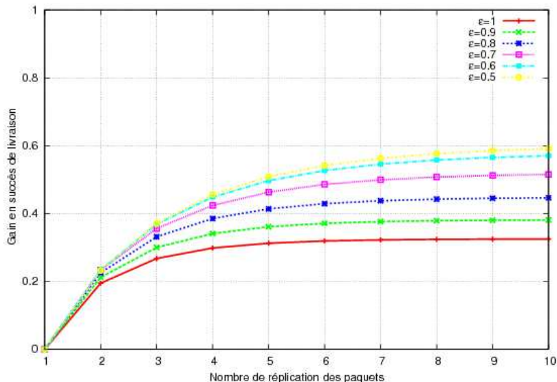
FIGURE 6.12: Gain en taux de livraison en fonction de taux de réplications x avec P_c = 0.1 d'attaques.
