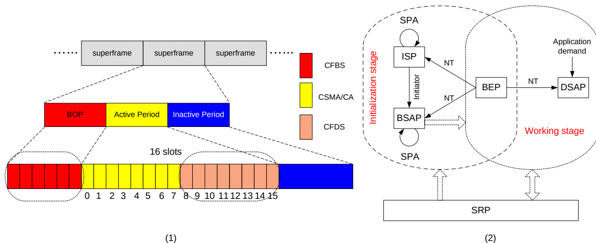
Figure 1 Le structure de super frame et le schéma de fonctionnement d'ADCF
