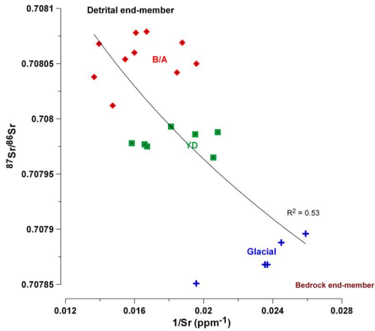
Figure IV. 3.: diagramme ^{87}\text{Sr}/^{86}\text{Sr} = f(1/\text{Sr}) tracé à partir des échantillons ^{87}\text{Sr}/^{86}\text{Sr} et de l'interpolation à ces points des valeurs élémentaires.
