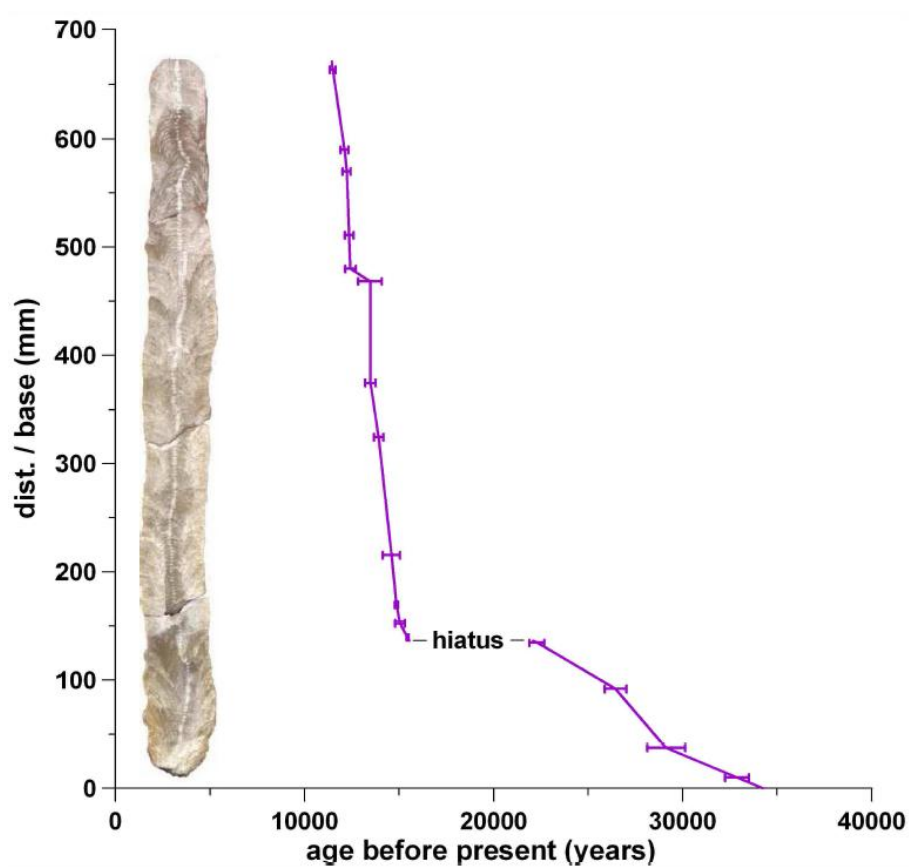
Figure IV. 1. Courbe de croissance de la stalagmite Chau-stm-6 à côté de sa section polie. Le modèle d'âge ici présenté a été établi à partir de datations U-Th.
