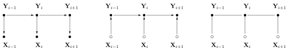
FIG. 2.18: Représentation graphique de 3 types de modélisation d’une séquence de trames. Illustration extraite de [Lafferty 2001]. X représente la séquence de trames à reconnaître et Y la séquence de modèles. De gauche à droite : un MMC gauche-droite, une combinaison hybride MMC-réseau de neurones et un CRF. Les cercles blancs indiquent que les variables ne sont pas générées par le modèle.
