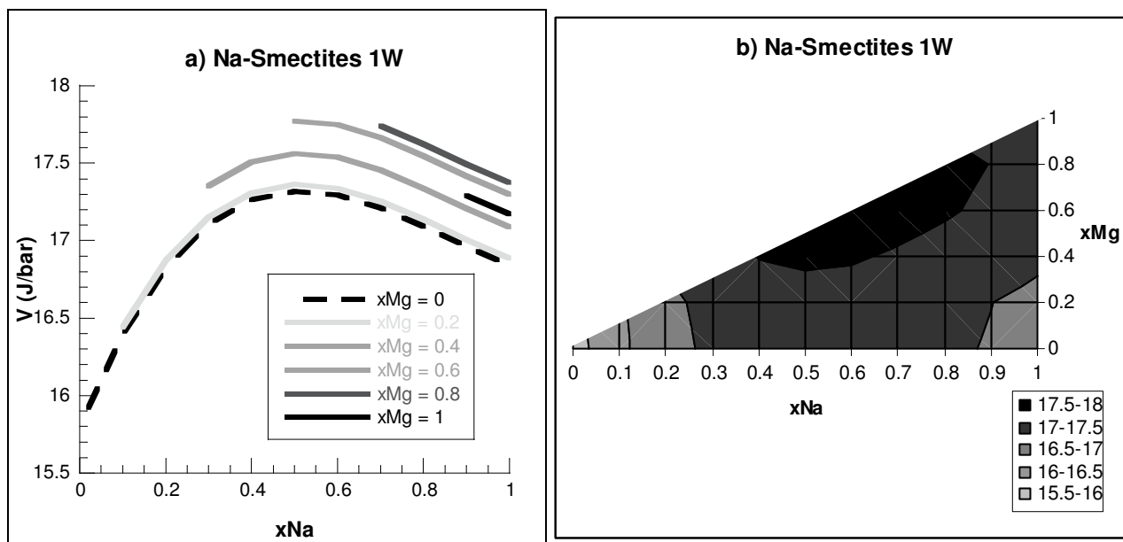
Figure 35 : Variations de volumes molaires pour les Na-smectites 1W ; a) V = f(x_{Na}) avec l'influence de x_{Mg} en nuances de gris ; b) Projection des variations de volume sur le plan (x_{Na}, x_{Mg})
