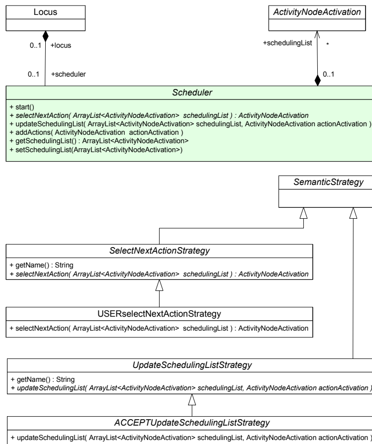
FIGURE 4.1 – Description de l'ordonnanceur dans le modèle d'exécution de fUML
