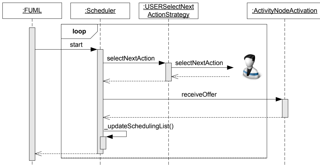
FIGURE 4.9 – Trace d’exécution avec ordonnanceur
