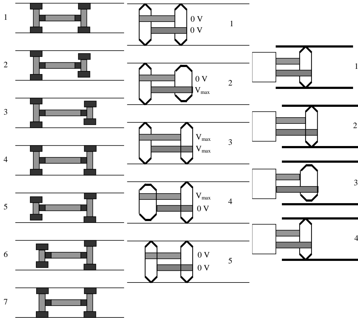
(a) Translation par Inchworm classique
