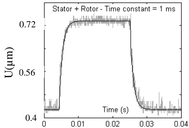
Figure 3.25 - Réponse à un échelon de phase
