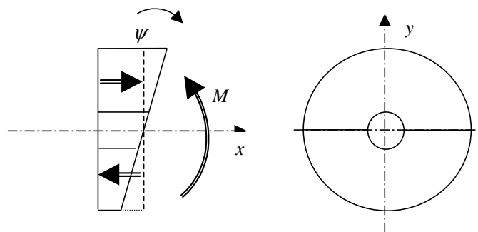
Figure 2.39 - Déformation d'une céramique du stator sous l'action d'une tension
