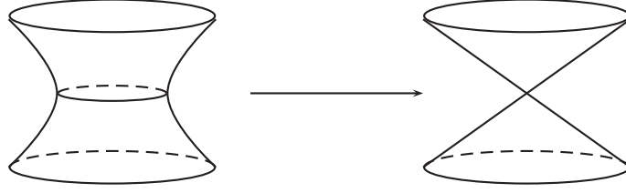
\mathcal{M}_\theta(1) qui se projette sur \mathcal{X}_0(1) \simeq \mathbb{C}^2/\mu_2 , pour \theta_1 \neq 0
