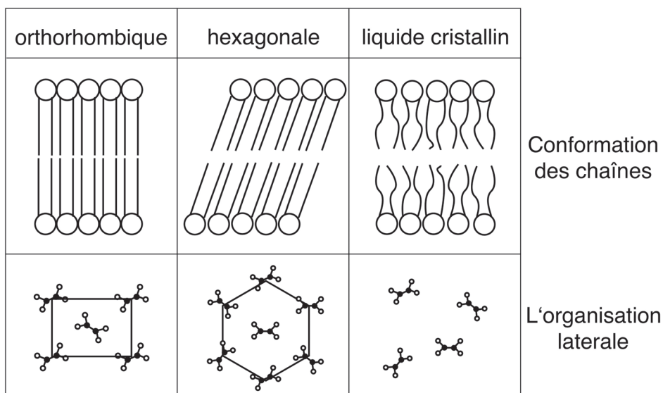
Figure 1-2 : L'organisation des lipides du stratum corneum . Schéma de la conformation des chaînes et de l'organisation latérale des chaînes dans une phase orthorhombique, hexagonale et cristalline liquide.
