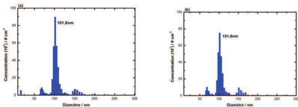
Figure V.26. Distribution en taille des particules de sulfate d'ammonium de 100 nm avant l'entrée (a) et à la sortie (b) du tube à écoulement des aérosols. Maximum à 101,8 nm.
