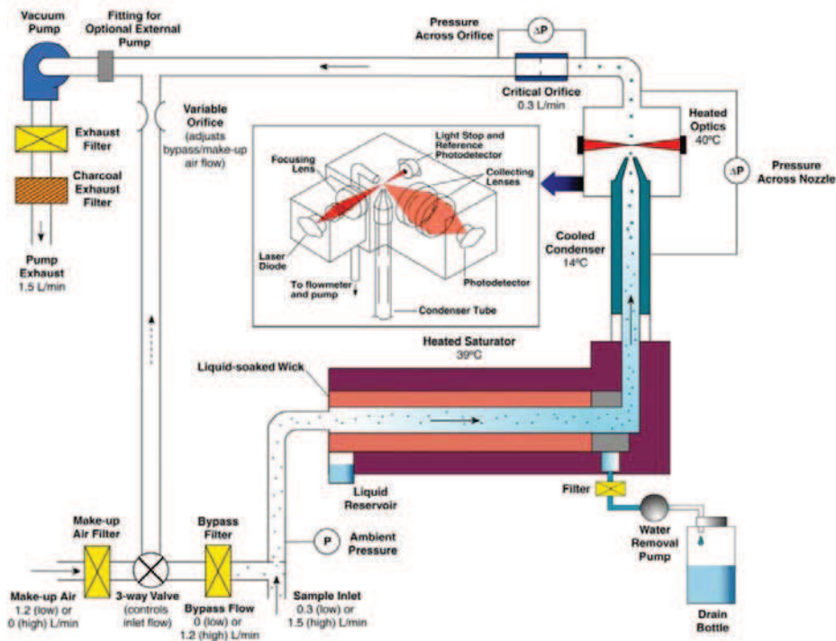
Figure III.12. Schéma du CPC modèle 3776, TSI
