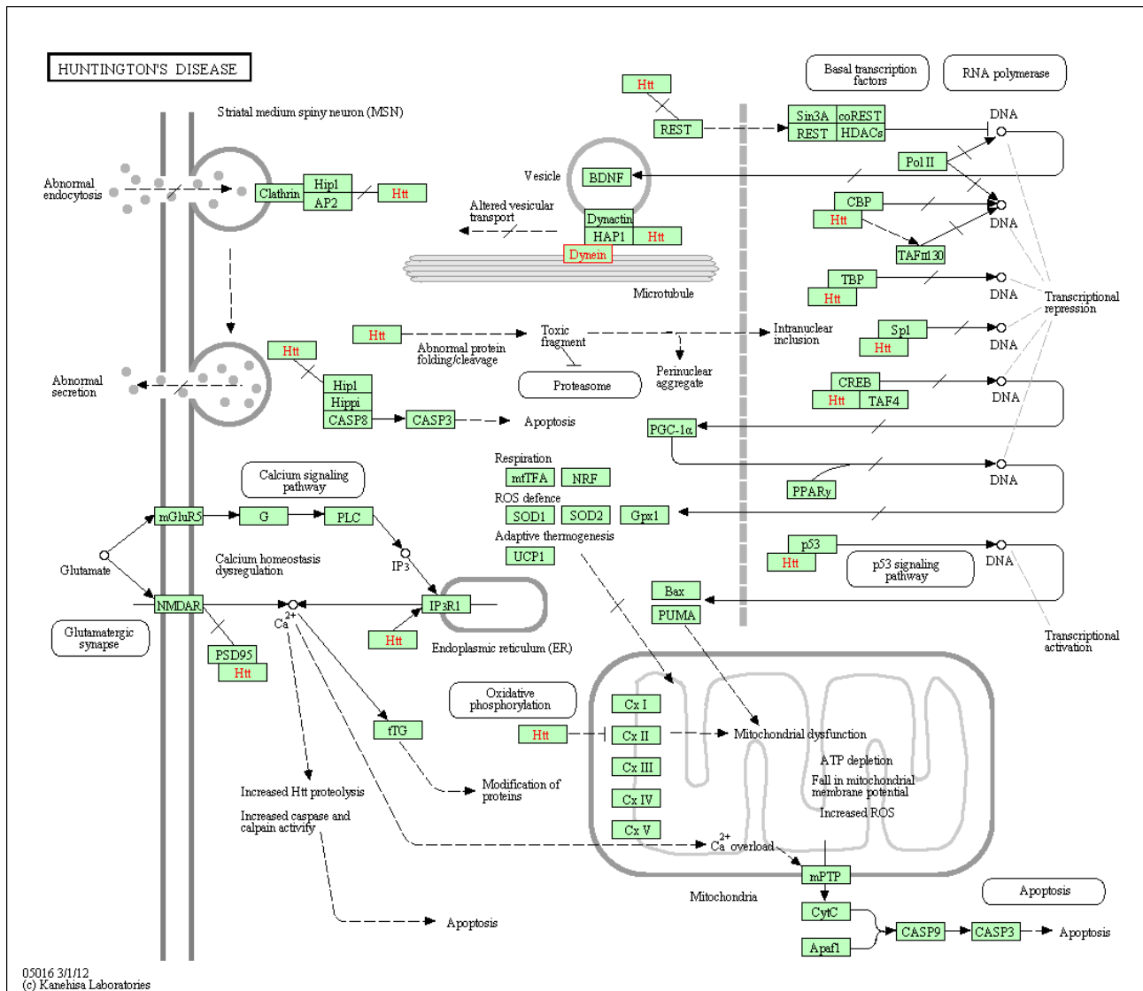
Figure 21. Voie métabolique de Huntington. Les nœuds rouges caractérisent les gènes impliqués dans des maladies de type Ciliopathie. Image générée à partir de la sous-banque de données spécialisée dans l'analyse des ciliopathies (instance SM2PH-Ciliopathy).
