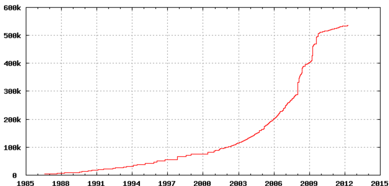
Figure 18. Evolution du nombre d'entrées de la banque Swiss-Prot depuis sa création en 1986. Adaptée de http://web.expasy.org/docs/relnotes/relnstat.html .
