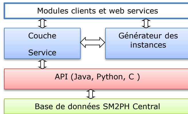
Figure 31. Architecture Orientée Service de SM2PH Central.
