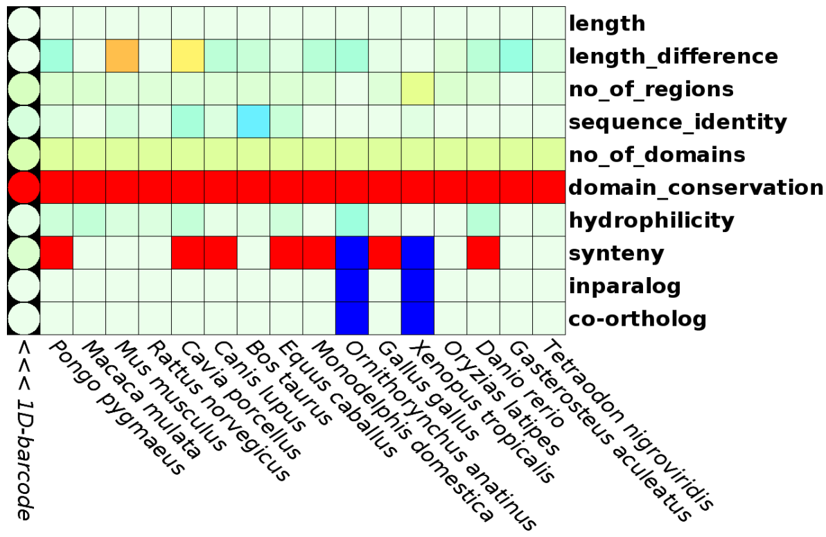
Figure 24. Visualisation d'un code-barre évolutif (EvoluCode) sous sa forme 2D pour le gène LIPC impliqué dans la Dégénérescence Maculaire Liée à l'Âge. Le code-barre 1D est sur la gauche. Les couleurs bleues et rouges correspondent aux valeurs atypiques pour les différents paramètres attribués selon une courbe gaussiennes (rouge = paramètre atypiquement fréquent, bleu = paramètre atypiquement rare).
