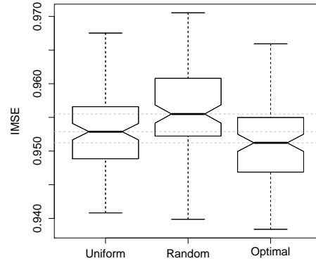
(d) d = 1, T = 50, n = 10, \theta = 5.10^{-3} k(\cdot, \cdot) : 3/2-Matérn, \eta(x) = \mu_U(x)
