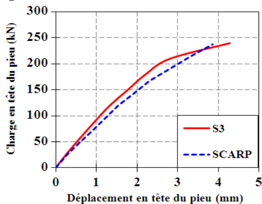
Figure 1. Comparaison d'un essai de chargement statique S3 sur le pieu de CRAN et une simulation SCARP.
