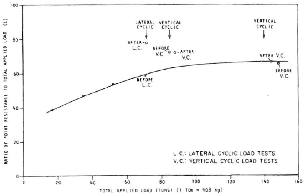
Figure I-34 : Évolution du pourcentage de la pointe en fonction de la charge appliquée (Lu et al, 1979)
