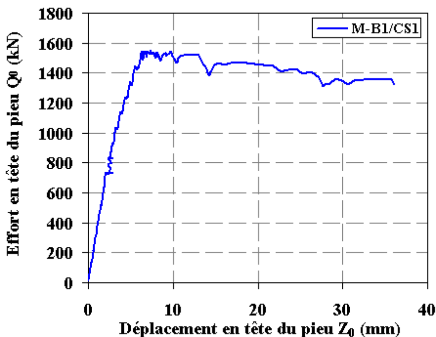
Figure III-7 : Courbe effort-déplacement de l’essai de chargement statique NF en compression M-B1/CS1 (Merville)
