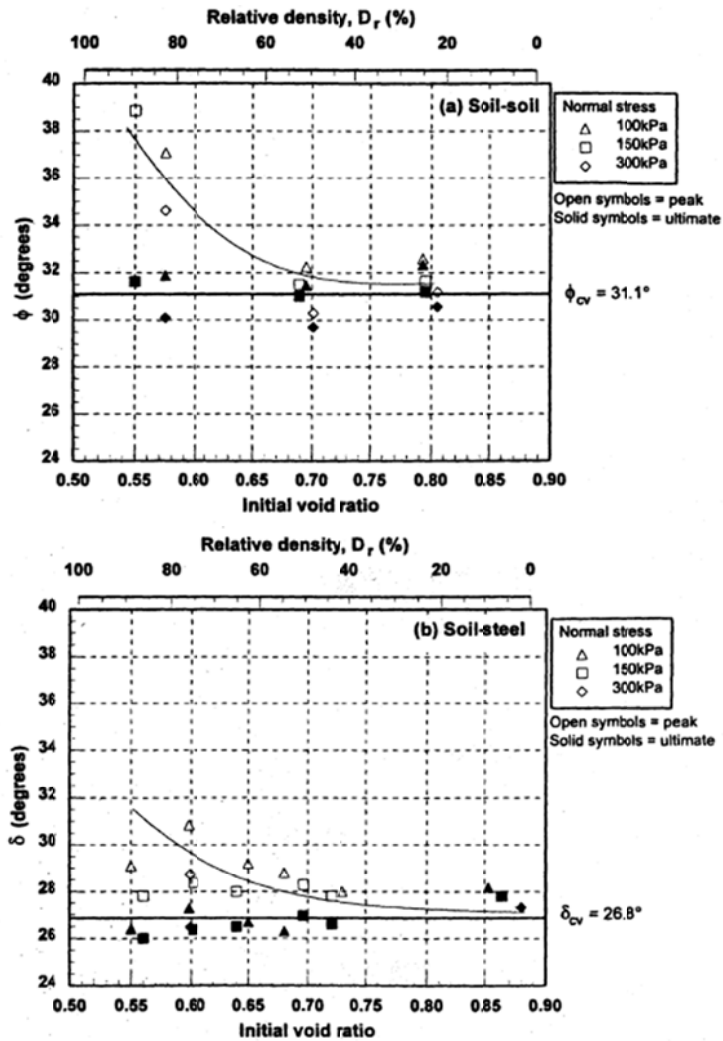
Figure II-11 : Angle d'interface sol-sol et sol-acier (Kuwano, 1999)
