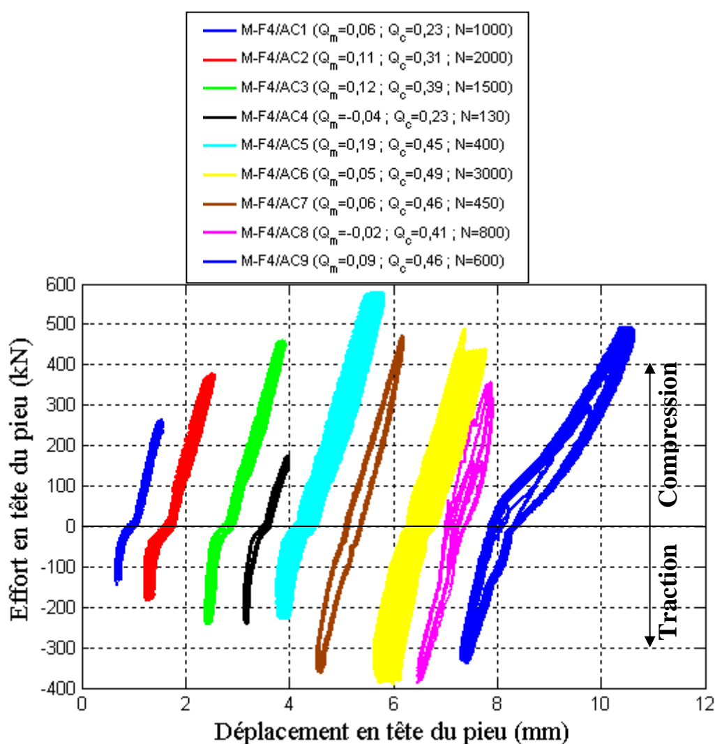
Figure III-41 : Historique de chargements sur le pieu foré F4
