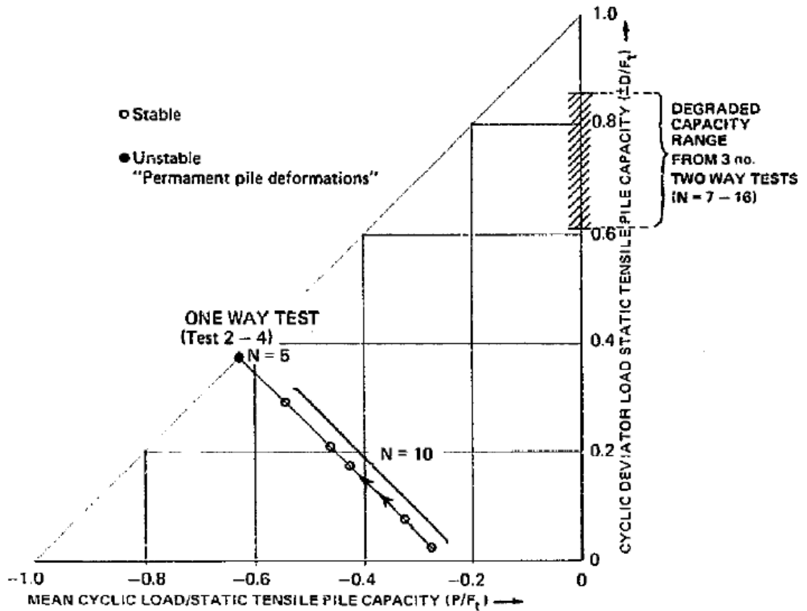
Figure I-26 : Diagramme de stabilité des essais de chargements cycliques de pieu effectués dans l'argile de la Baie de San Francisco (Doyle et Pelletier, 1985)
