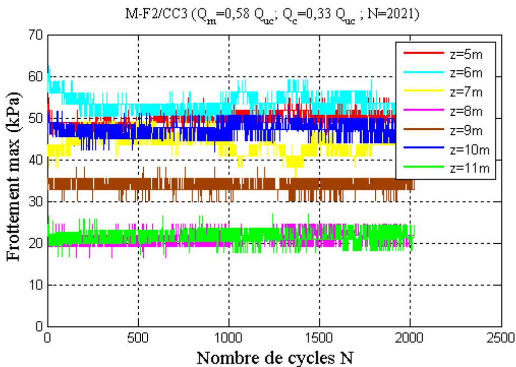
Figure III-35 : Frottement maximal développé sur les couches de l’argile des Flandres durant la séquence M-F2/CC3
