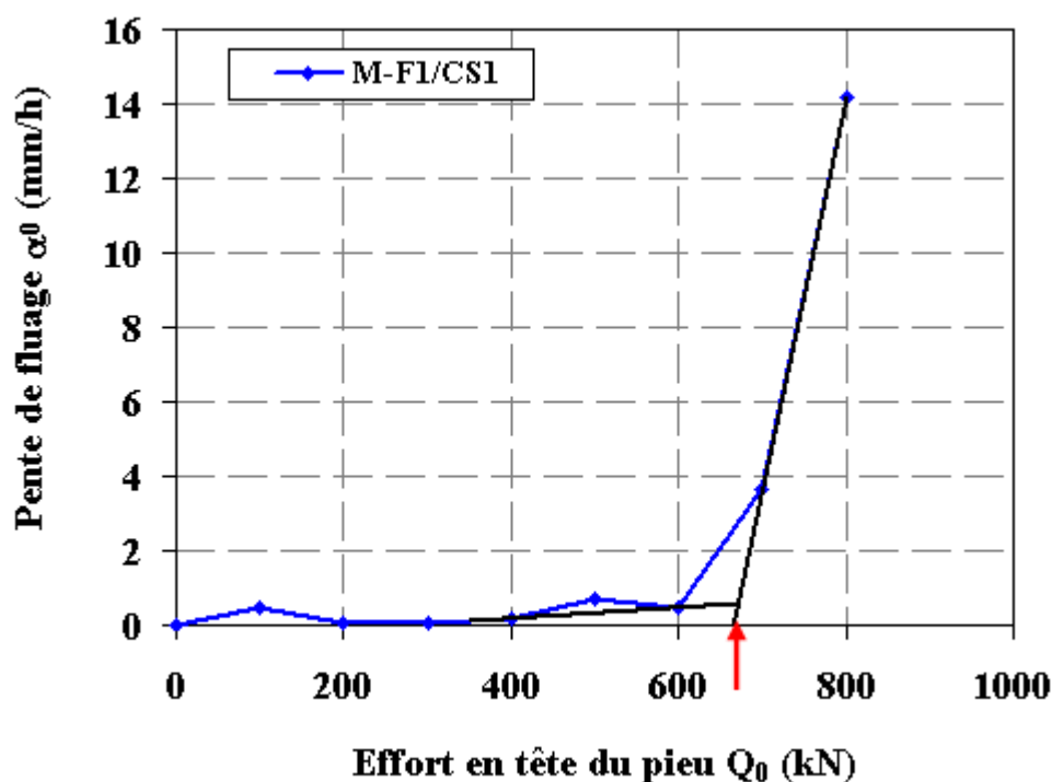
Figure III-2 : Pente de fluage \alpha_0 en fonction du chargement en tête Q_0 de l’essai M-F1/CS1
