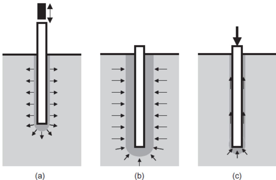
Figure I-4 : Trois phases principales pendant l'histoire du pieu battu ou enfoncé : (a) installation ; (b) reconsolidation ; (c) chargement (Randolph, 2003)
