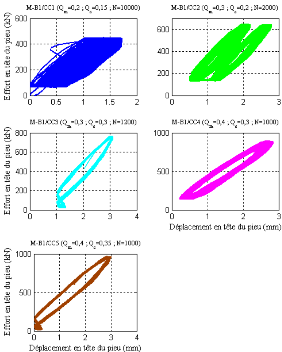
Figure III-47 : Courbes effort-déplacement des essais cycliques sur le pieu B1
