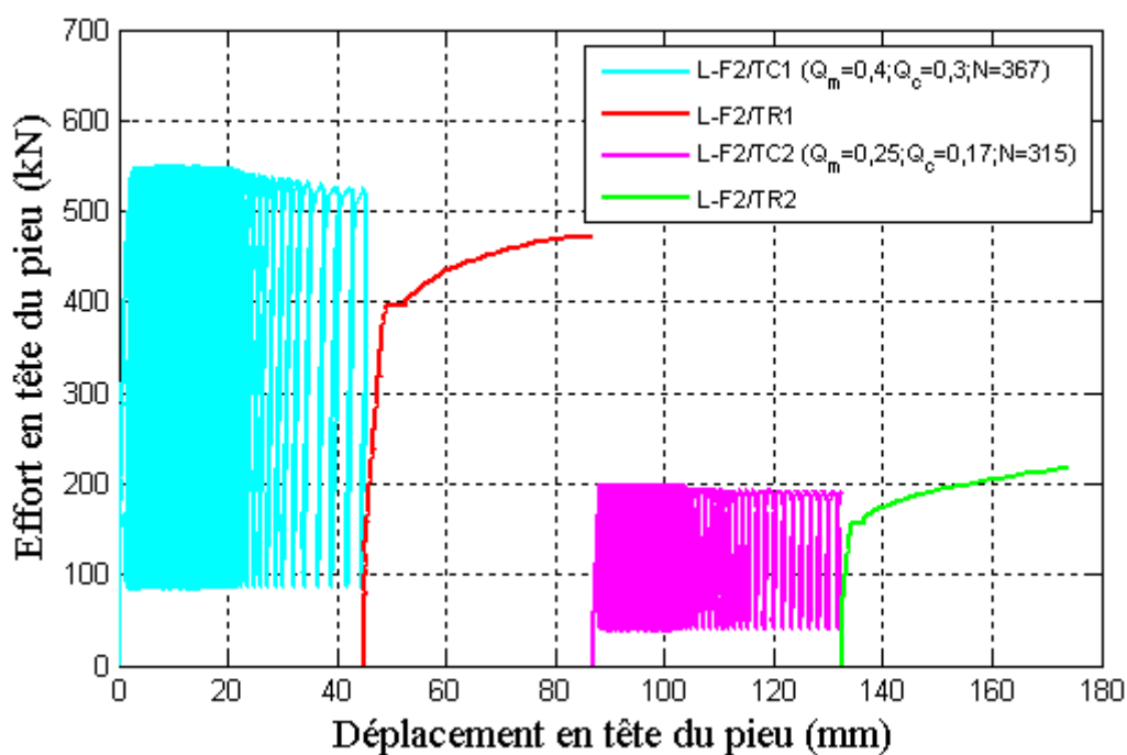
Figure IV-11 : Historique de chargements sur le pieu foré F2
