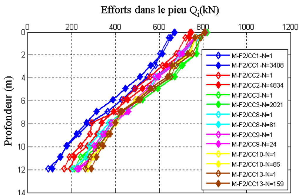
Figure III-34 : Les efforts mesurés le long du pieu F2 au premier et au dernier cycle des différents essais cycliques.
