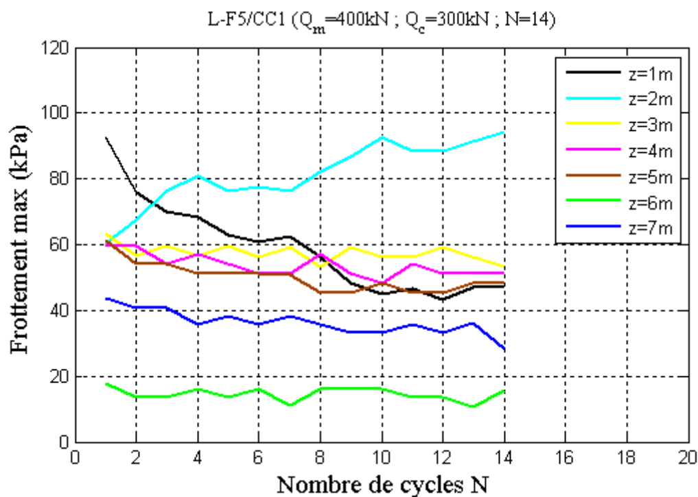
Figure IV-28 : Frottement maximal développé sur tous les niveaux pour la séquence effectuée sur le pieu vierge L-F5/CC1.
