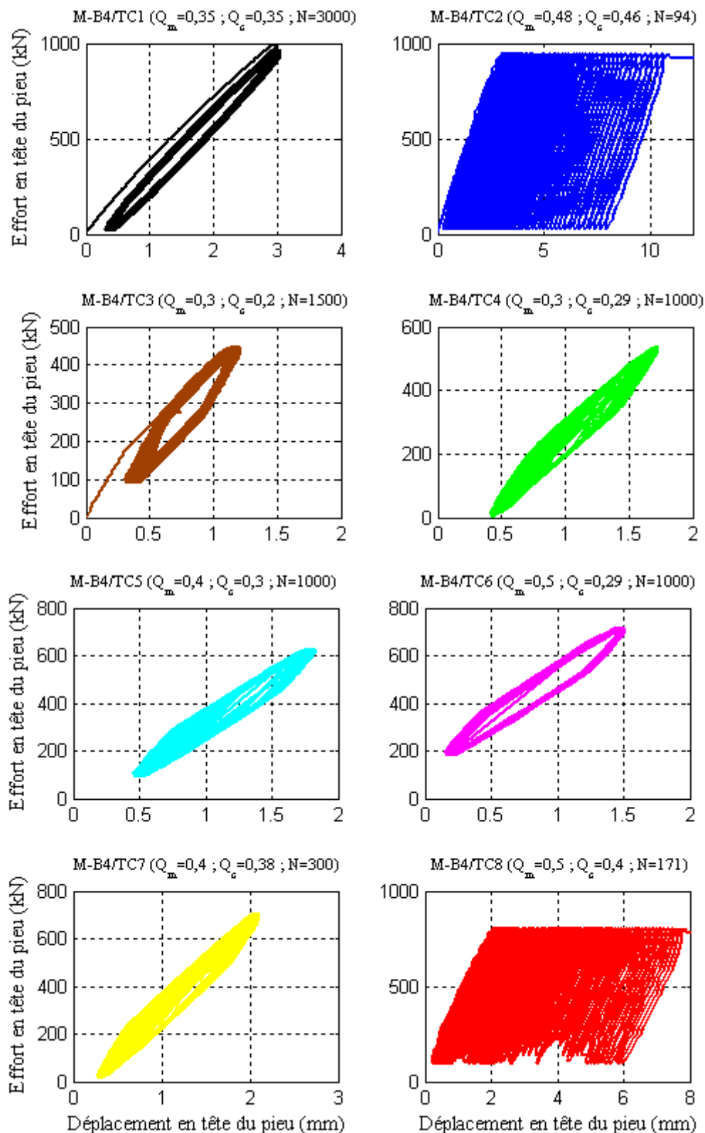
Figure III-50: Courbes effort-déplacement des essais cycliques sur le pieu B4
