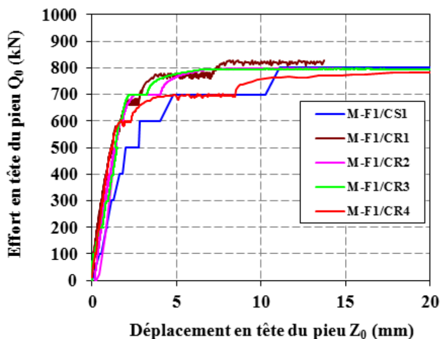
Figure III-6 : Comparaison des courbes effort-déplacement des essais de chargements rapides et celle de l'essai statique NF en compression (Merville)
