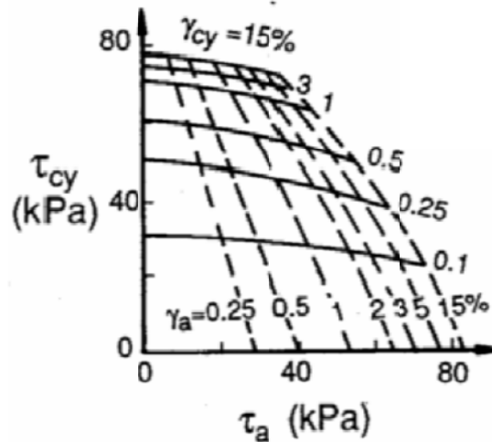
Figure I-48 : Diagramme de Contour définissant les contraintes de cisaillement moyenne et cyclique \tau_c en fonction des distorsions moyenne \gamma_a et cyclique \gamma_c pour un nombre de cycles.
