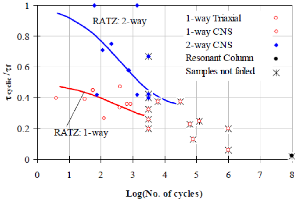
Figure I-46 : Courbes de fatigue obtenues par RATZ et comparées à des essais cycliques de laboratoire (Randolph, 2003)
