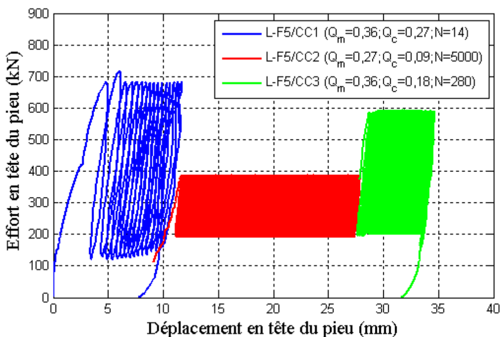
Figure IV-20 : Historique de chargements sur le pieu foré F5
