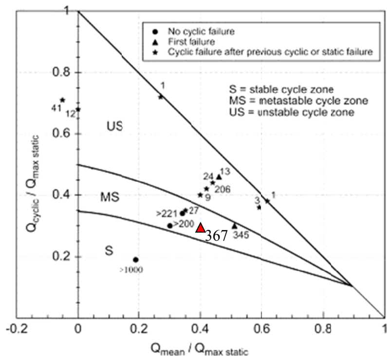
Figure IV-18 : Diagramme de stabilité des essais de chargements cycliques de pieux battus dans le sable de Dunkerque (Jardine and Standing, 2012).
