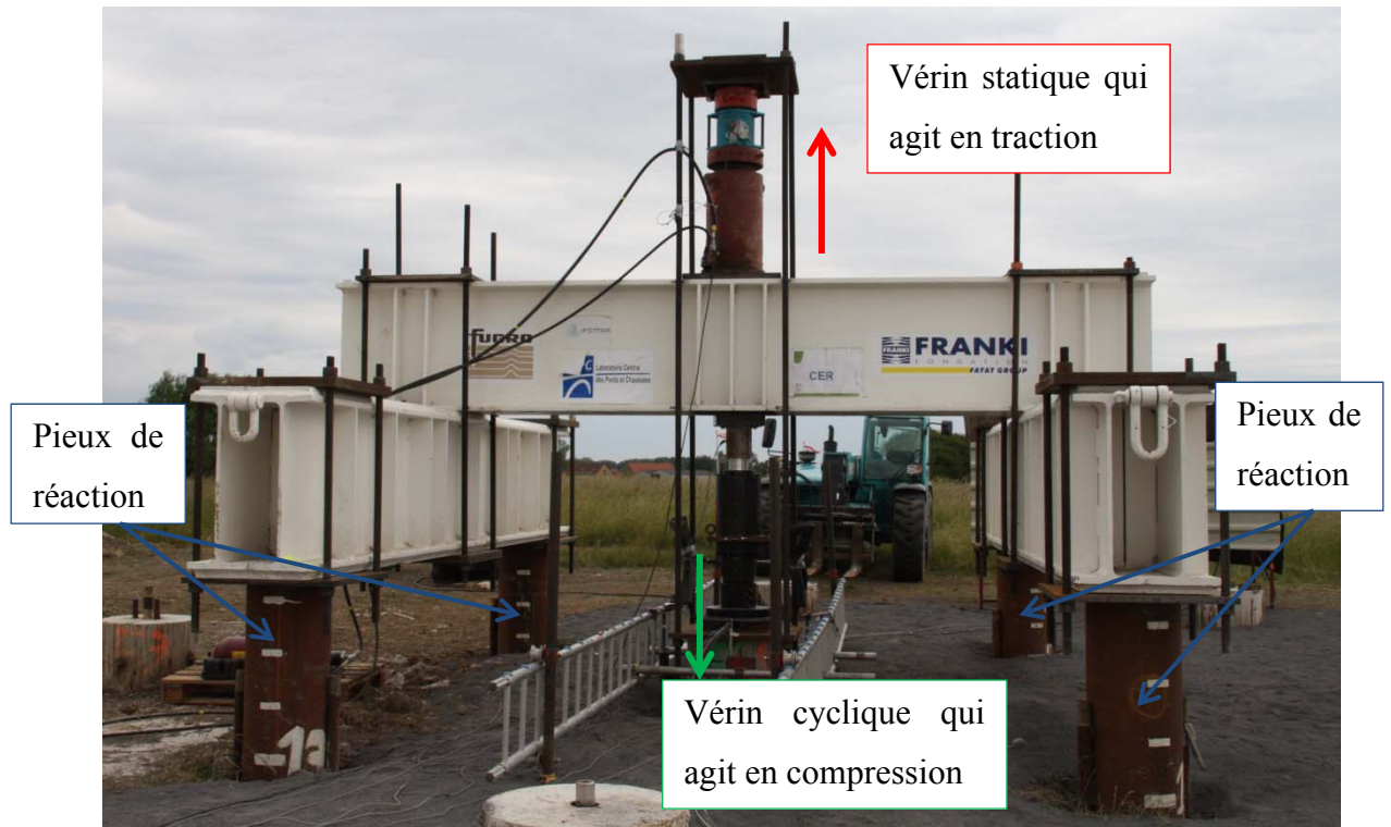
Figure II-28 : Photo du montage d'un essai de chargement cyclique alterné
