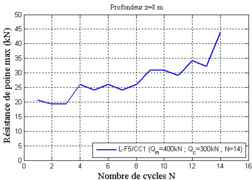
Figure IV-30 : Évolution de la résistance de pointe du pieu vierge sous l'essai L-F5/CC1.
