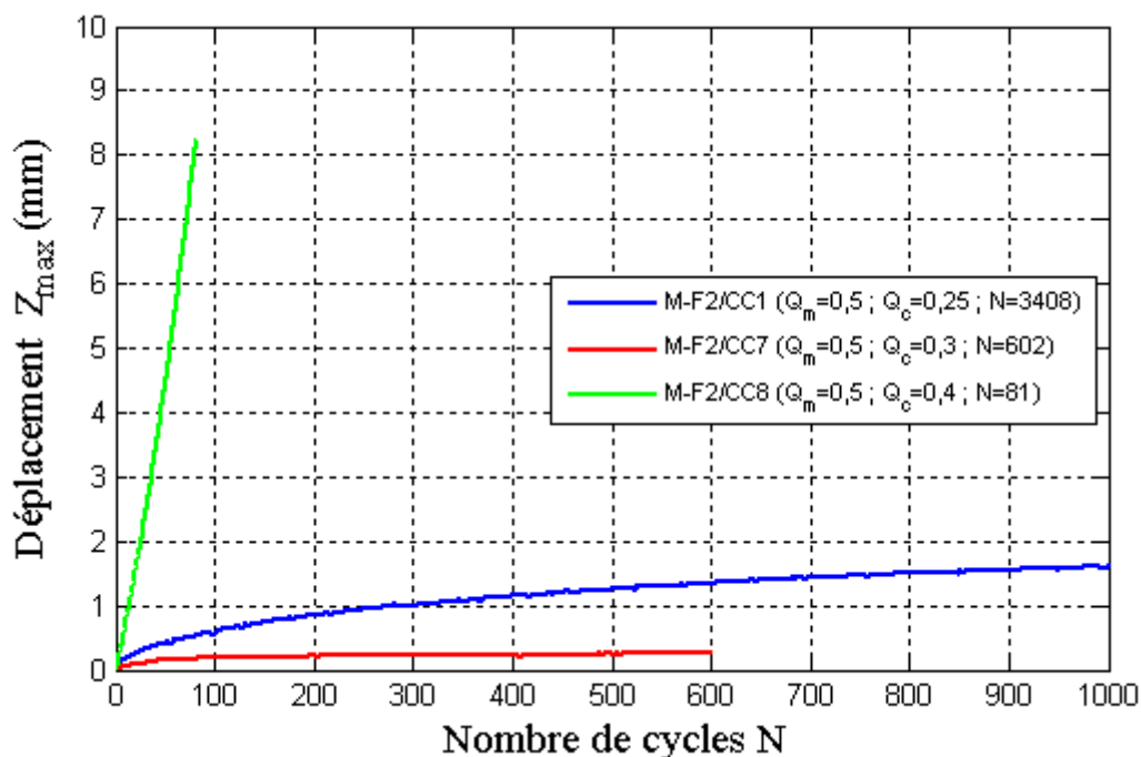
Figure III-32 : Influence de l’amplitude cyclique sur l’accumulation de déplacement en tête du pieu F2
