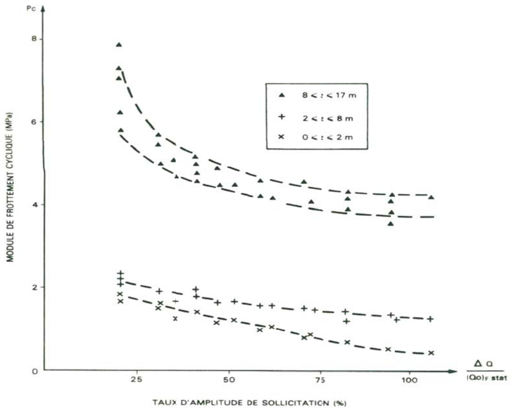
Figure I-25 : Évolution des modules cycliques par couche de sol avec le niveau de l'amplitude de chargement cyclique (Pieu de Cran)
