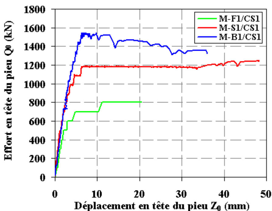
Figure III-19 : Comparaison des courbes effort-déplacement des essais de chargements statique NF en compression sur trois types de pieux.
