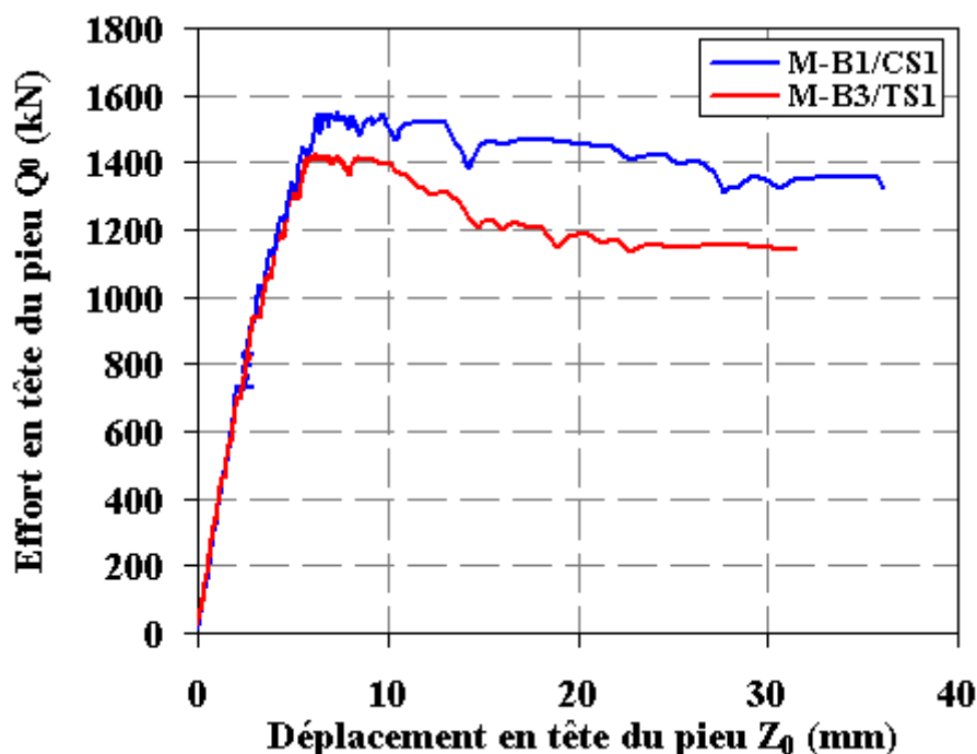
Figure III-13 : comparaison des courbes d'effort déplacement en tête entre l'essai statique N-F en compression sur le pieu B1 (M-B1/CS1) et celui en traction sur le pieu B3 (M-B3/TS1)
