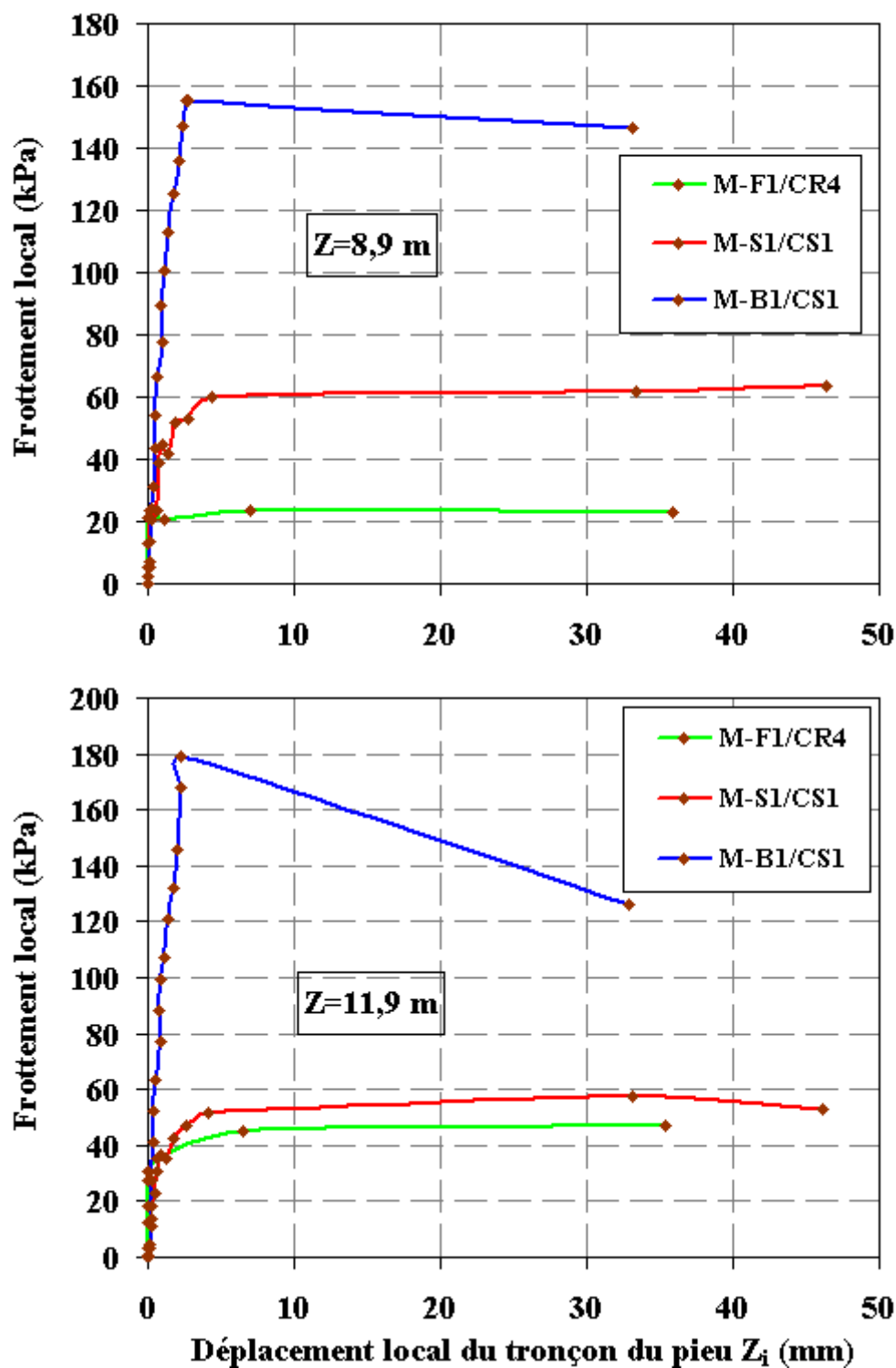
Figure III-20 : Frottements latéraux mobilisés le long des trois types de pieux des couches a) 8 et b) 11.
