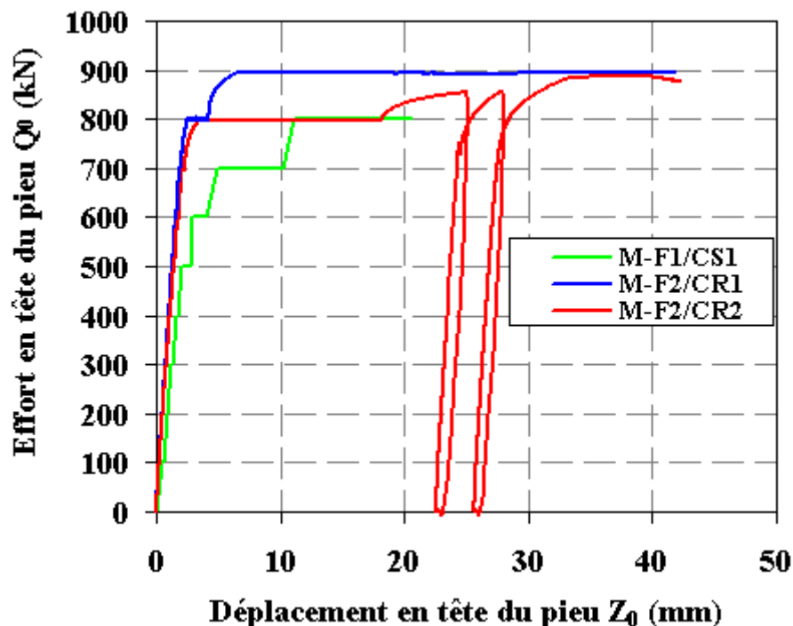
Figure III-33 : Comparaison entre l’essai statique N-F effectué sur le pieu F1 et les différents essais statiques rapides effectués sur le pieu F2.
