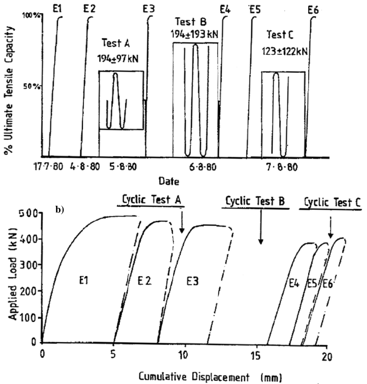
Figure I-17 : a) Historique de chargement et b) Déplacement cumulatif en tête du pieu de Cowden (McAnoy et al., 1982)
