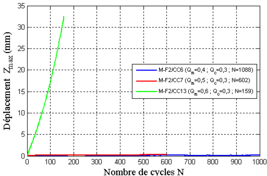
Figure III-31 : Influence de la charge moyenne sur l’accumulation de déplacement en tête du pieu F2
