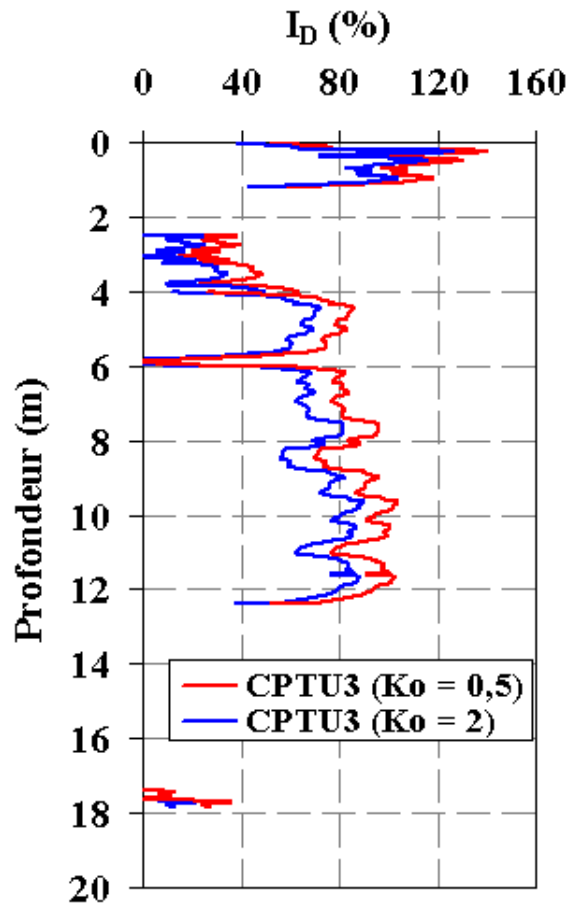
Figure II-10 : Profils pénétrométriques à Loon-Plage : résistance au cône q_c et indice de densité I_D .
