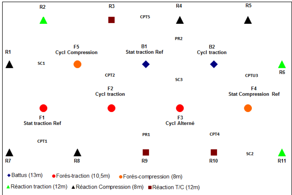
Figure II-16 : Configuration du plot d'essais de pieux de Loon-Plage (Fi = pieu test de type foré; Bi = pieu test de type battu; SCi= carottages continus, CPTi= pénétromètre statique, PRi=pressiomètre Ménard)
