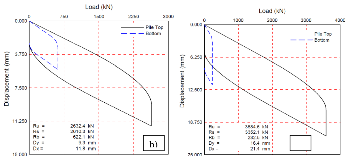
Figure IV-8 : L'estimation des courbes effort-déplacement sous l'énergie a) de 30,4 kJ et b) de 51kJ.
