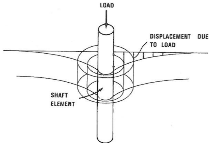
Figure I-11 : Mécanisme de mouvement du pieu par le cisaillement de cylindres concentriques. (Randolph et Wroth, 1978)
