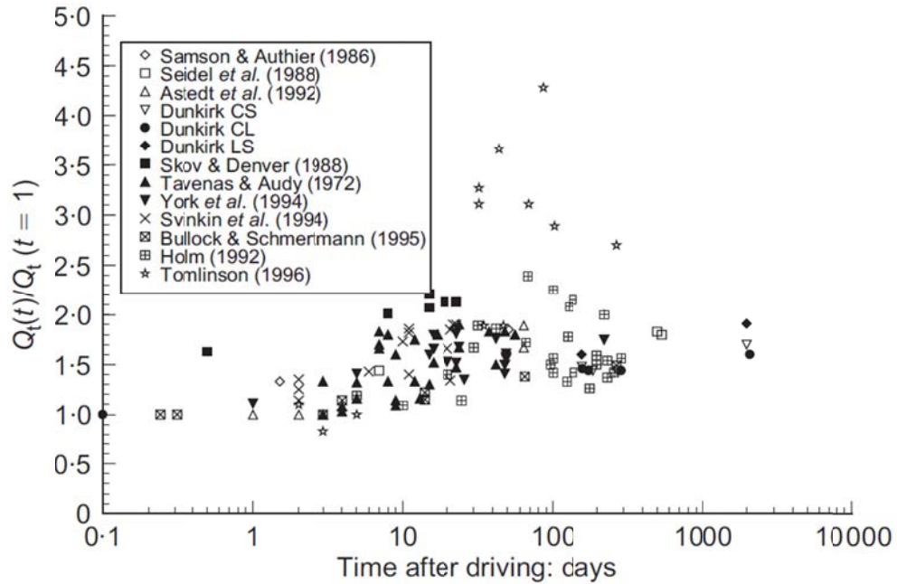
Figure I-5 : Base de données de l'augmentation de la capacité portante des pieux battus dans le sable en fonction du temps d'après (Chow et al., 1997)
