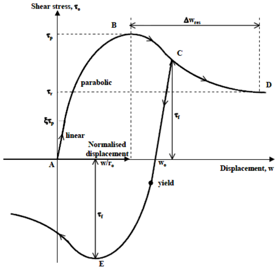
Figure I-44 : Allure générale des courbes de transfert utilisée dans RATZ
