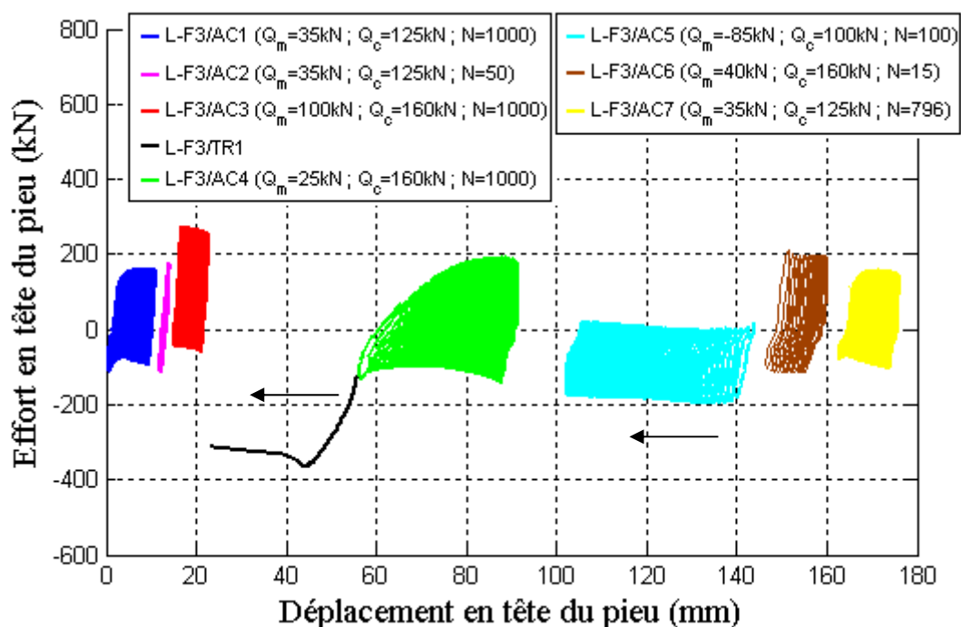
Figure IV-33 : Historique de chargements sur le pieu foré F3
