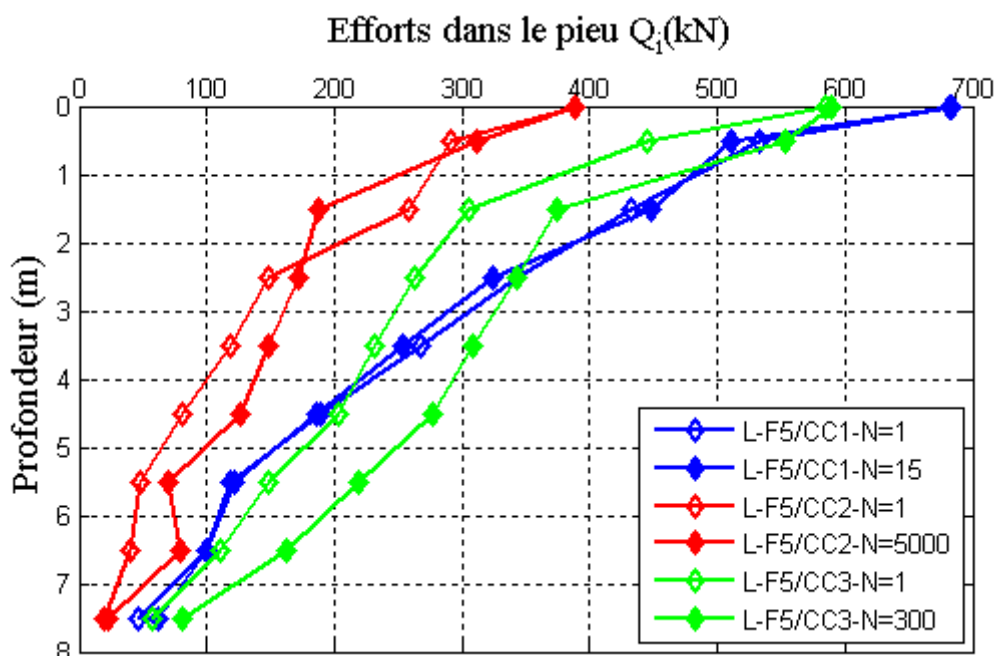
Figure IV-27 : Les efforts mesurés le long du pieu F5 au premier et au dernier cycle des trois essais cycliques.
