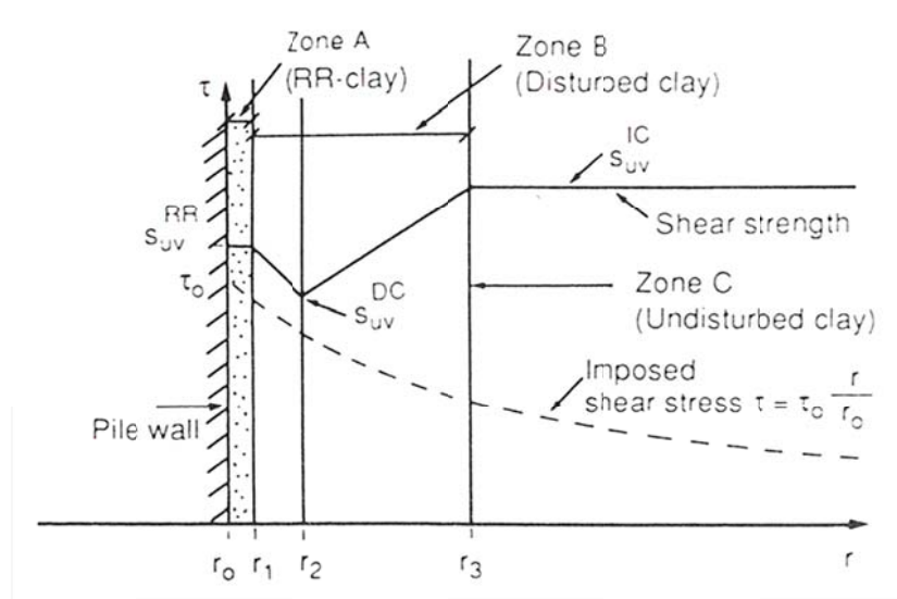
Figure I-47: variation de la résistance au cisaillement non drainée autour du pieu (Karlsrud et al., 1992b).
