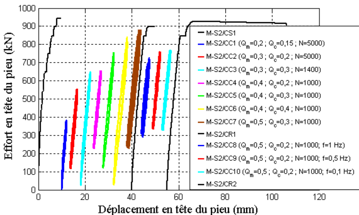
Figure III-44 : Historique de chargements en traction sur le pieu vissé S2
