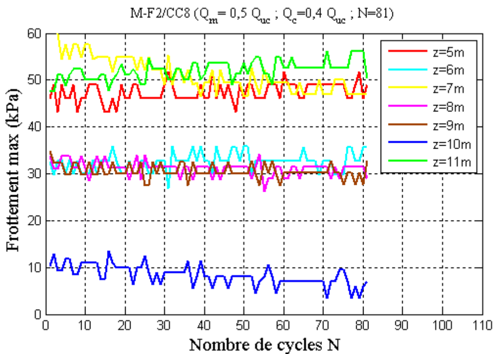
Figure III-36 : Frottement maximal développé sur les couches de l’argile des Flandres durant la séquence M-F2/CC8
