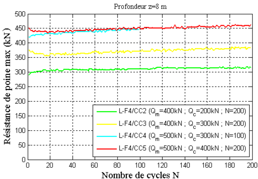
Figure IV-31 : Évolution de la résistance de pointe du pieu F5 durant les essais (L-F4/CC2, L-F4/CC3, L-F4/CC4, L-F4/CC5).
