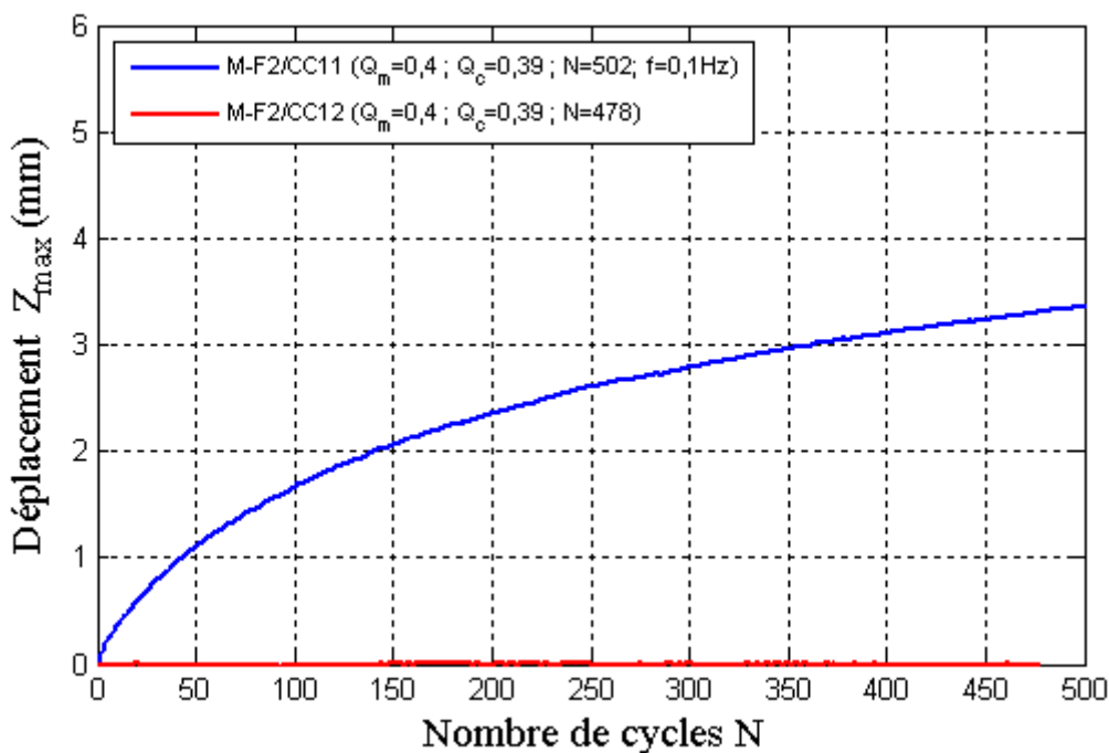
Figure III-30 : Influence de la fréquence sur l'accumulation de déplacement en tête du pieu F2 sous la combinaison de chargement cyclique ( Q_m= 0,4 et Q_c=0,39 )
