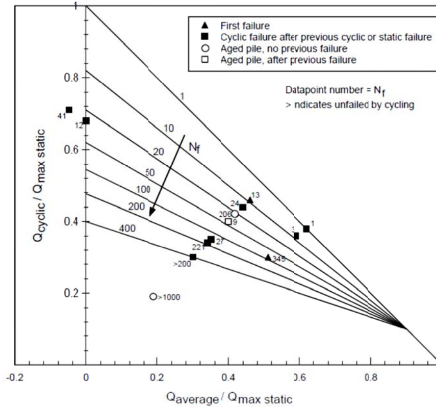
Figure I-37 : Diagramme sommaire des essais de chargements cycliques de pieux battus dans le sable de Dunkerque (Jardine and Standing, 2000).
