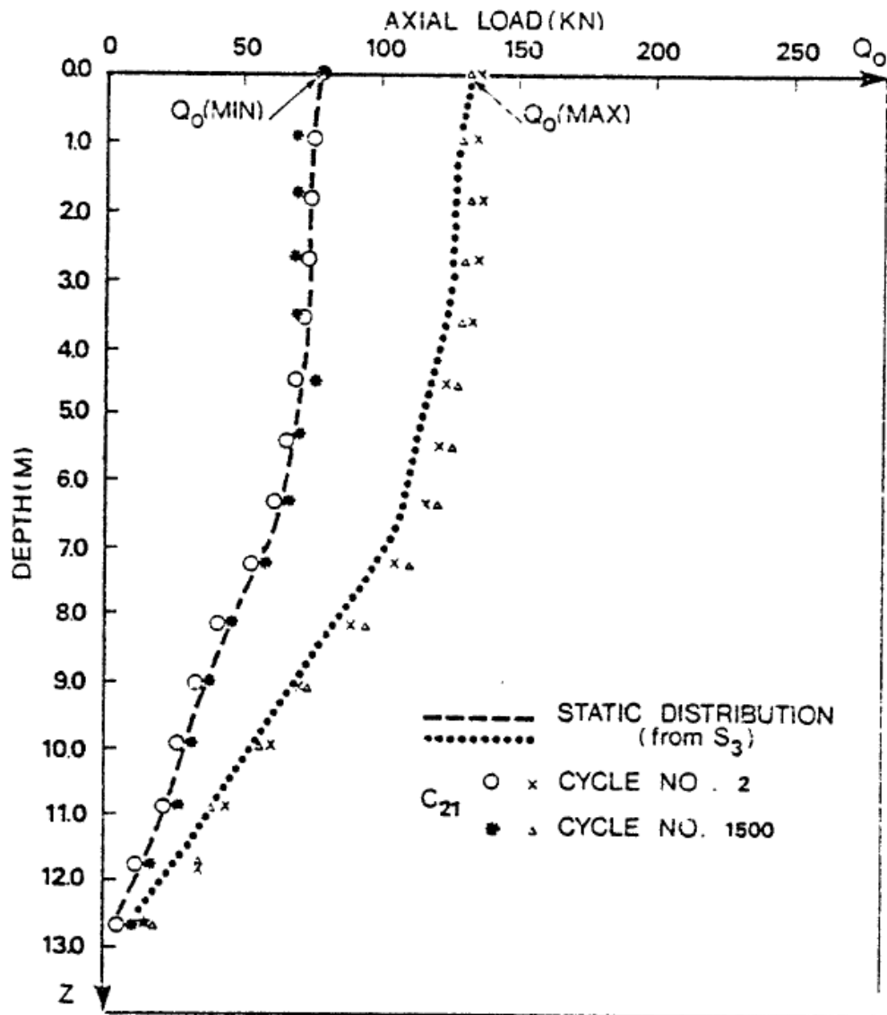
Figure I-22 : Comparaison des répartitions des efforts le long du pieu de Plancoët pendant l'essai statique S3 et cyclique C21.
