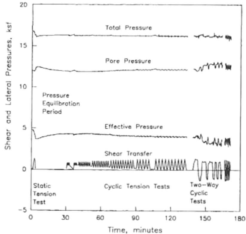
Figure I-31 : Exemple de d'essais de chargements sur un pieu d'Empire (Bogard et Matlock, 1990)
