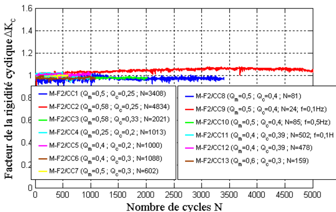
Figure III-28 : Facteur d’évolution de la rigidité cyclique en fonction du nombre de cycle des différentes combinaisons cycliques effectuées sur le pieu F2.
