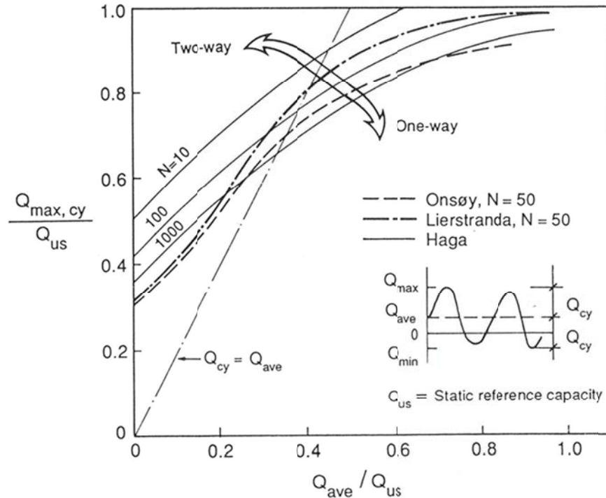
Figure I-30 : Comparaison des résultats obtenus d'essai de chargement cycliques des pieux d'Onsoy et de Lierstranda à ceux de Haga (Karlsruud et al., 1992b).
