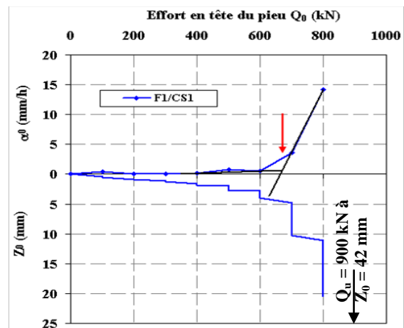
Figure 5. Courbe charge-déplacement en tête et courbe de fluage obtenues pour l'essai statique de référence sur le pieu F1.
