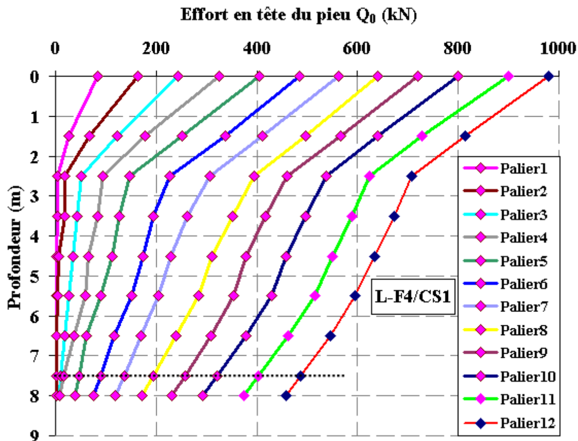
Figure IV-5 : Répartition des efforts le long du pieu lors de l'essai du chargement statique L-F4/CS1
