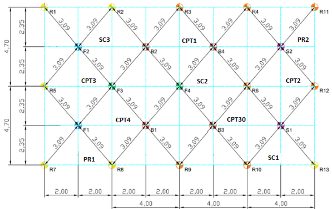
Figure II-15 : Configuration du plot d'essais de pieux de Merville ( F_i = pieu test de type foré; B_i = pieu test de type battu; S_i = pieu test de type vissé, SC_i = carottages continus, CPT_i = pénétromètre statique, PR_i =pressiomètre Ménard)
