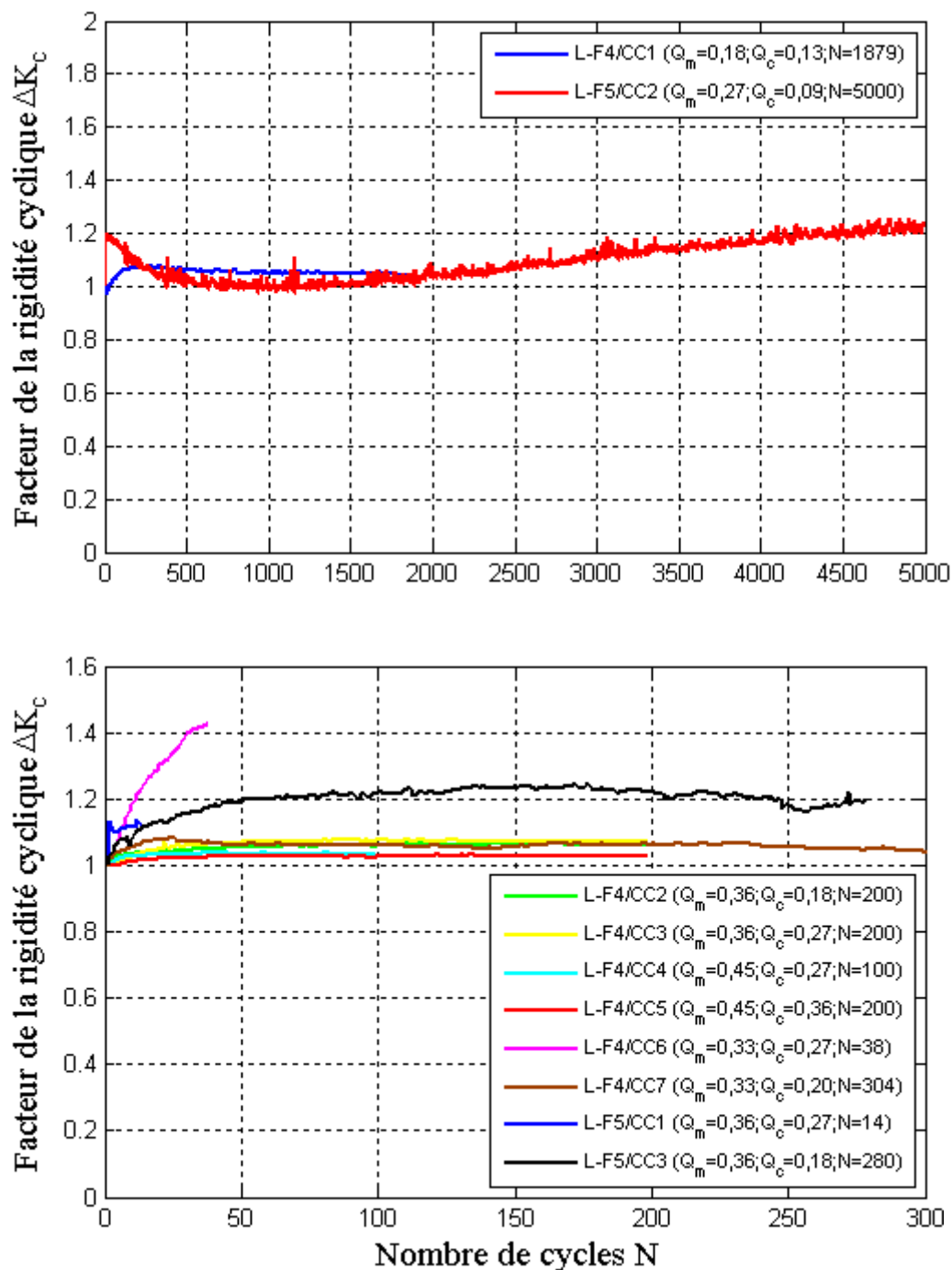
Figure IV-24 : Facteur d'évolution de la rigidité cyclique en fonction du nombre de cycle des différentes combinaisons cycliques effectuées sur les deux pieux F4 et F5.
