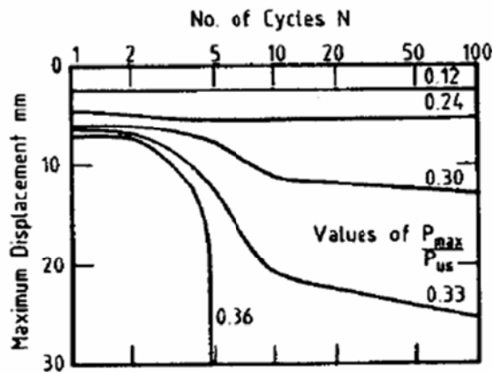
Figure I-40 : Evolution du déplacement permanent avec le nombre de cycles dans le cas de l'essai non alterné en compression (Poulos, 1988)
