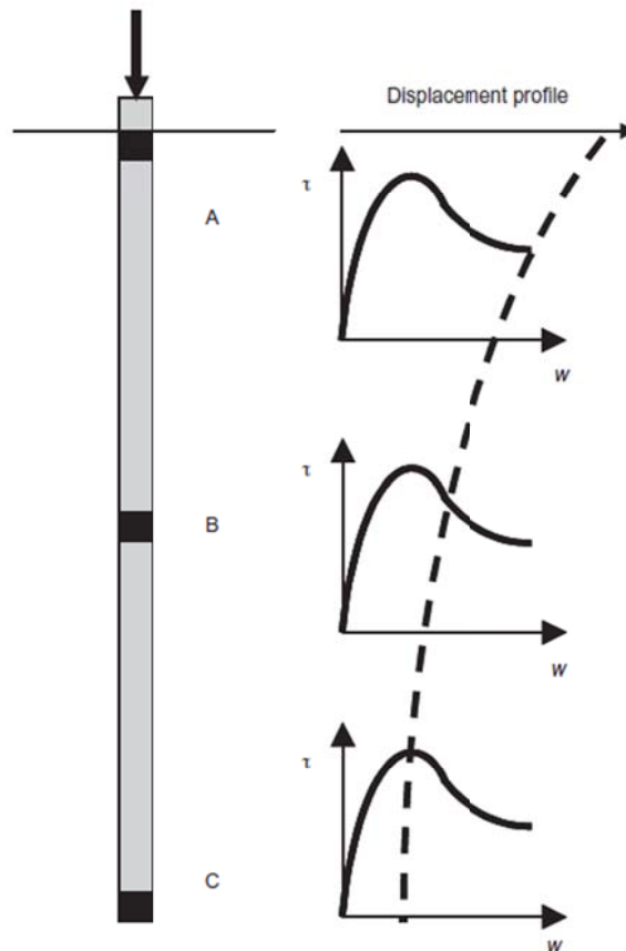
Figure I-2 : Rupture progressive d'un pieu souple installé dans un sol ayant un comportement radoucissant (Randolph, 2003)
