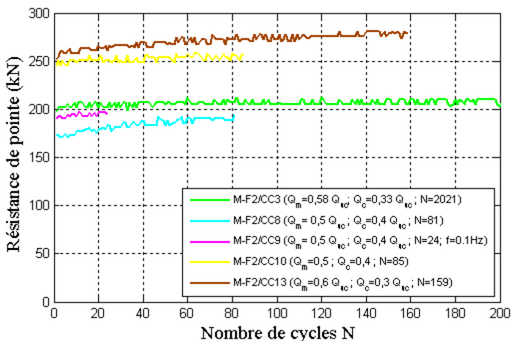
Figure III-40 : Évolution de la résistance de pointe du pieu F2 durant les essais (M-F2/CC3, M-F2/CC8, M-F2/CC9, M-F2/CC10 et M-F2/CC13).
