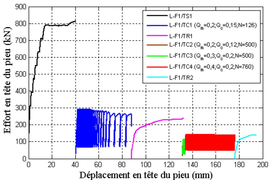
Figure IV-10 : Historique de chargements sur le pieu foré F1
