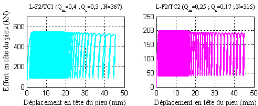
Figure IV-13 : Courbes effort-déplacement des essais cycliques sur le pieu F2
