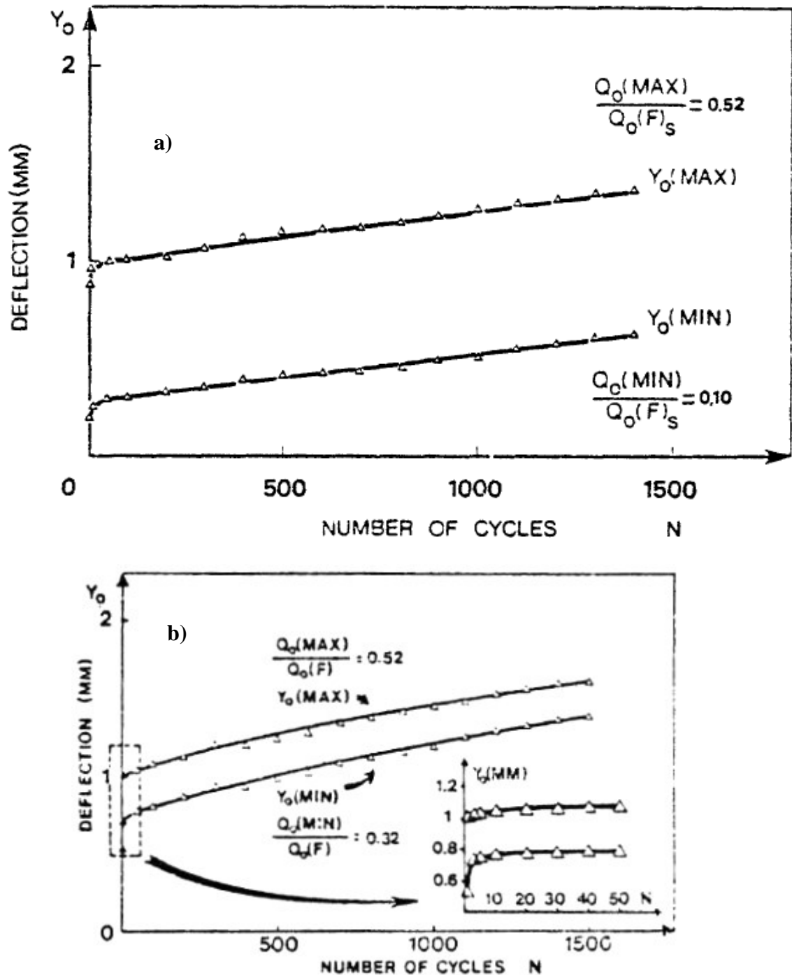
Figure I-20 : Évolution du déplacement du pieu de Plancoët pendant : a) l'essai cyclique C12 b) l'essai cyclique C21
