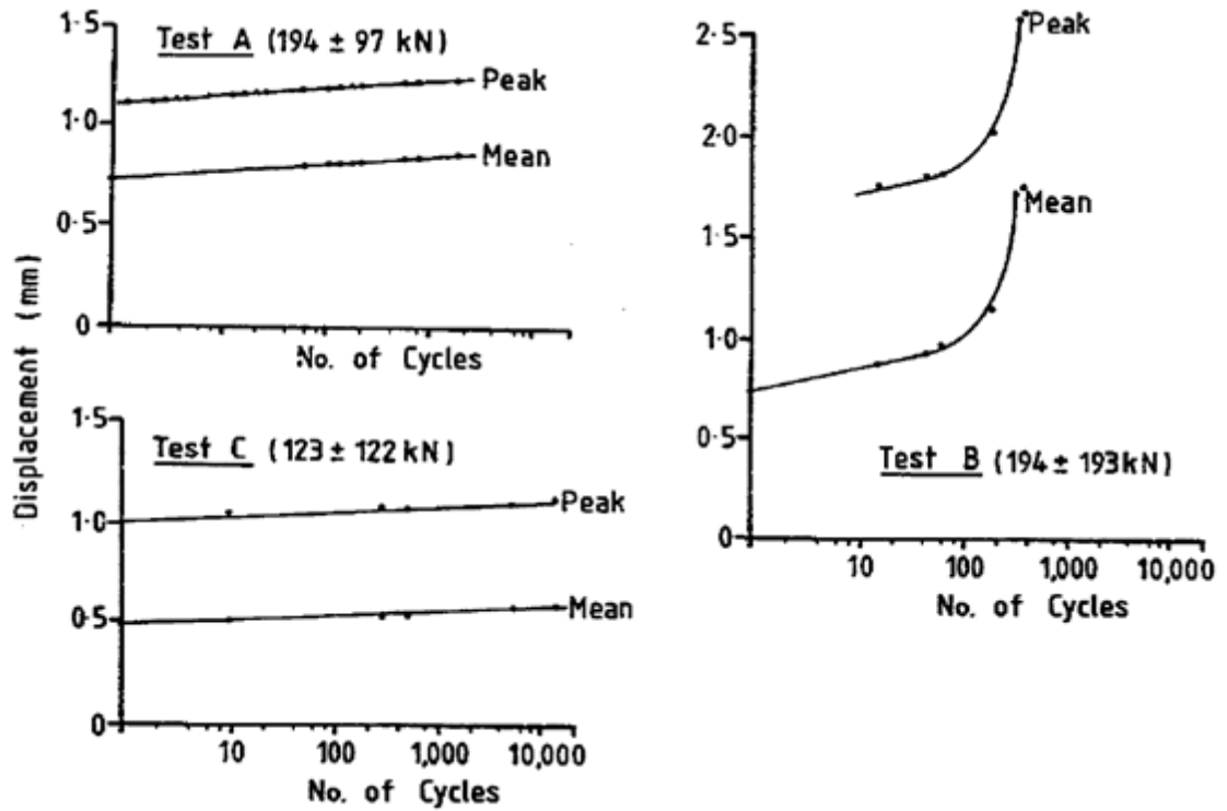
Figure I-18 : Déplacements moyens et maximaux durant les essais cycliques (A, B, C) (McAnoy et al., 1982)
