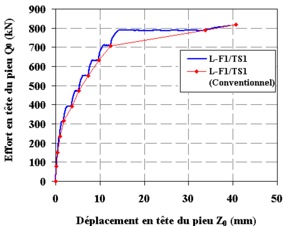
Figure IV-1 : Courbe effort-déplacement de l'essai de chargement statique NF en traction L-F1/TS1 (Loon-Plage)
