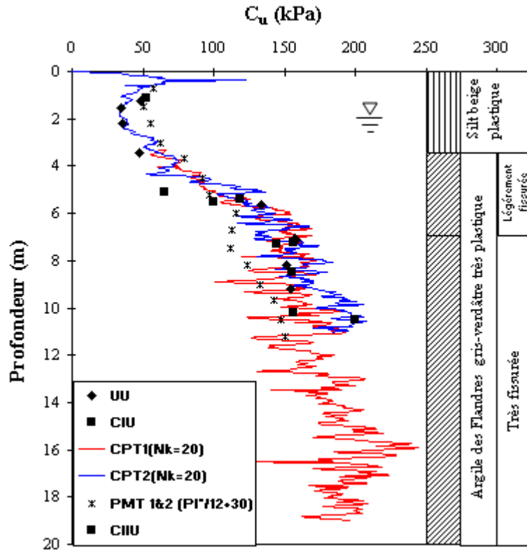
Figure II-5 : Variation de la résistance au cisaillement non drainée en fonction de la profondeur.
