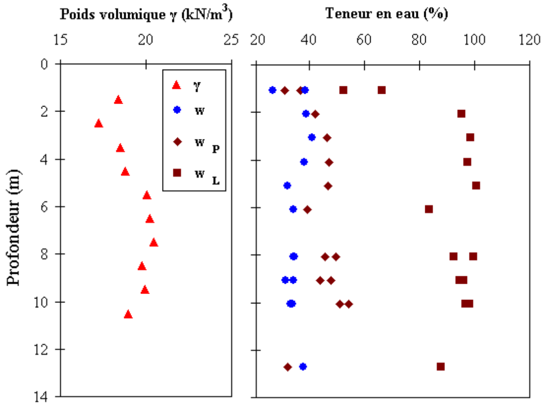
Figure II-4 : Variation du poids \gamma volumique, de la teneur en eau w , de la limite de plasticité w_p ainsi que de la limite de liquidité w_l en fonction de la profondeur.
