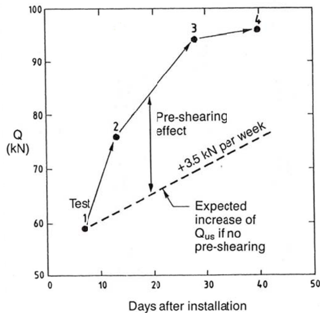
Figure I-6: Influence du temps et du pré-chargement sur la capacité portante du pieu installé dans l'argile surconsolidée de Haga (Karlsrud and Haugen, 1985a)
