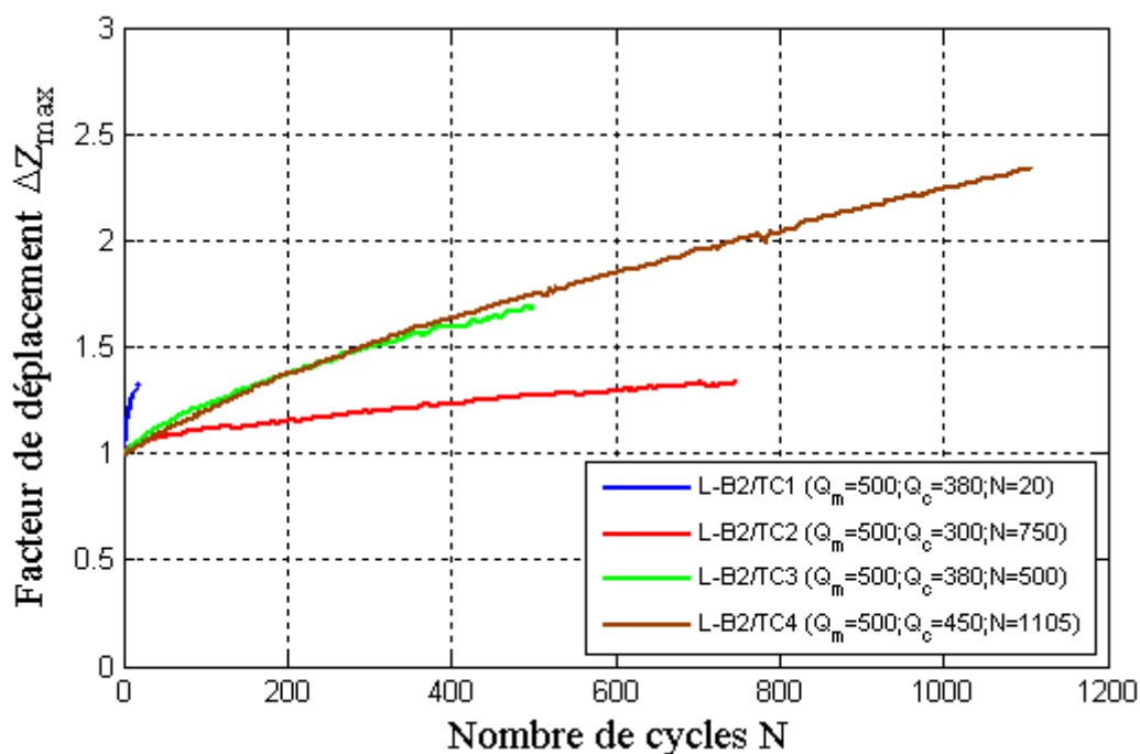
Figure IV-40 : Facteur d'évolution du déplacement en fonction du nombre de cycle des différentes combinaisons cycliques effectuées sur le pieu B2.
