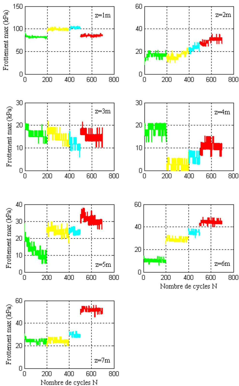
Figure IV-29 : Frottement maximal cyclique développé sur tous les tronçons du pieu F4 durant les essais (L-F4/CC2, L-F4/CC3, L-F4/CC4, L-F4/CC5).
