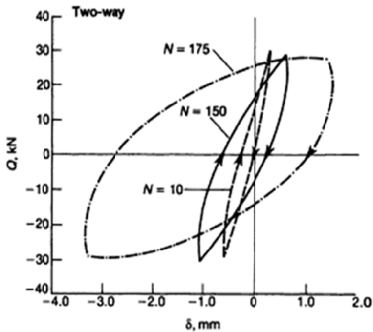
Figure I-28 : Courbe d'effort-déplacement d'un pieu soumis à un chargement cyclique alterné (Karlsrud et Haugen, 1985)
