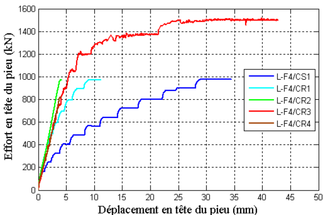
Figure IV-25 : Comparaison entre les différents essais statiques effectués sur le pieu F4.
