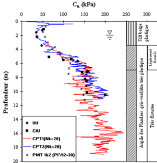
Figure 2. Conditions de sol au niveau du plot d'essais de Merville
