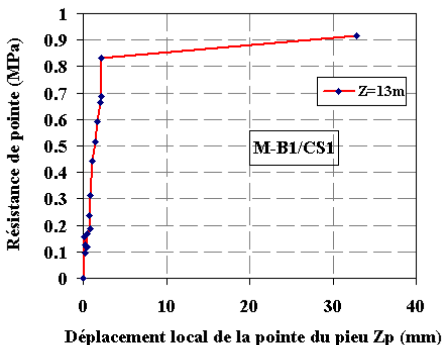
Figure III-11 : Évolution de la résistance de pointe du pieu battu lors de l’essai du chargement statique M-B1/CS1
