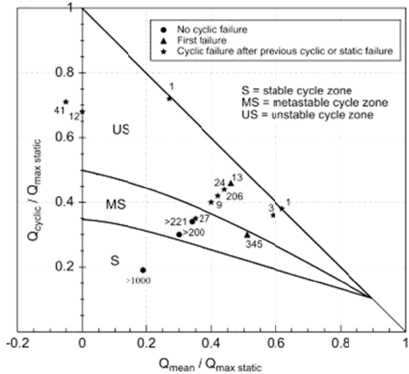
Figure I-38 : Diagramme de stabilité des essais de chargements cycliques de pieux battus dans le sable de Dunkerque (Jardine and Standing, 2012).
