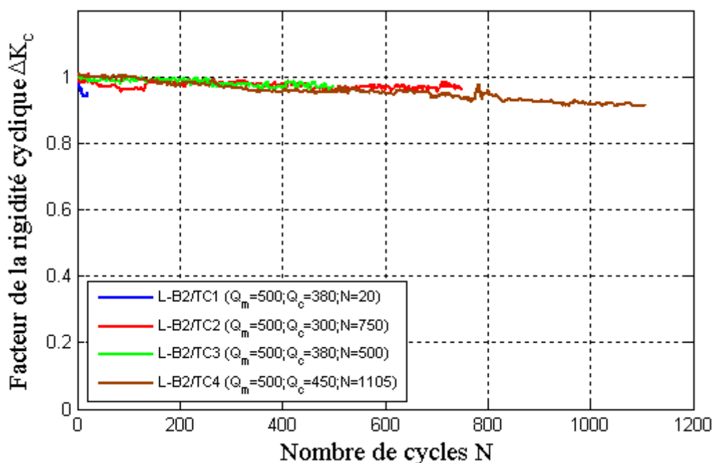
Figure IV-41 : Facteur d'évolution de la rigidité cyclique en fonction du nombre de cycle des différentes combinaisons cycliques effectuées sur le pieu B2.
