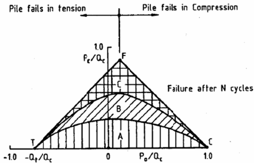
Figure I-42 : Diagramme de stabilité cyclique (Poulos, 1988)
