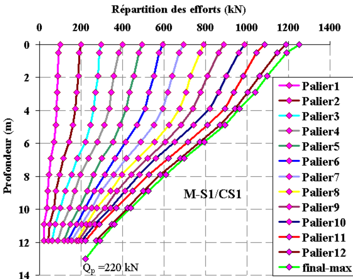
Figure III-16 : Répartition des efforts Q_i le long du pieu lors de l’essai du chargement statique M-S1/CS1
