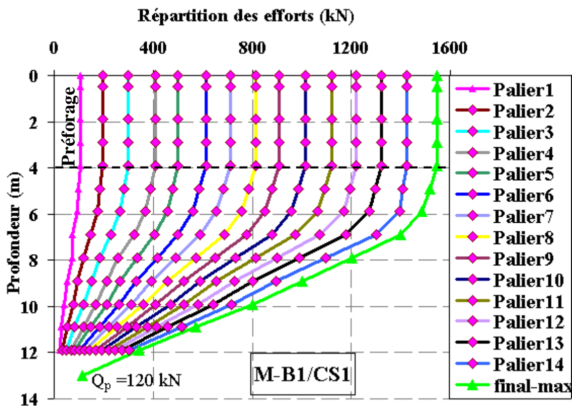
Figure III-9 : Répartition des efforts Q_i le long du pieu battu lors de l'essai du chargement statique M-B1/CS1
