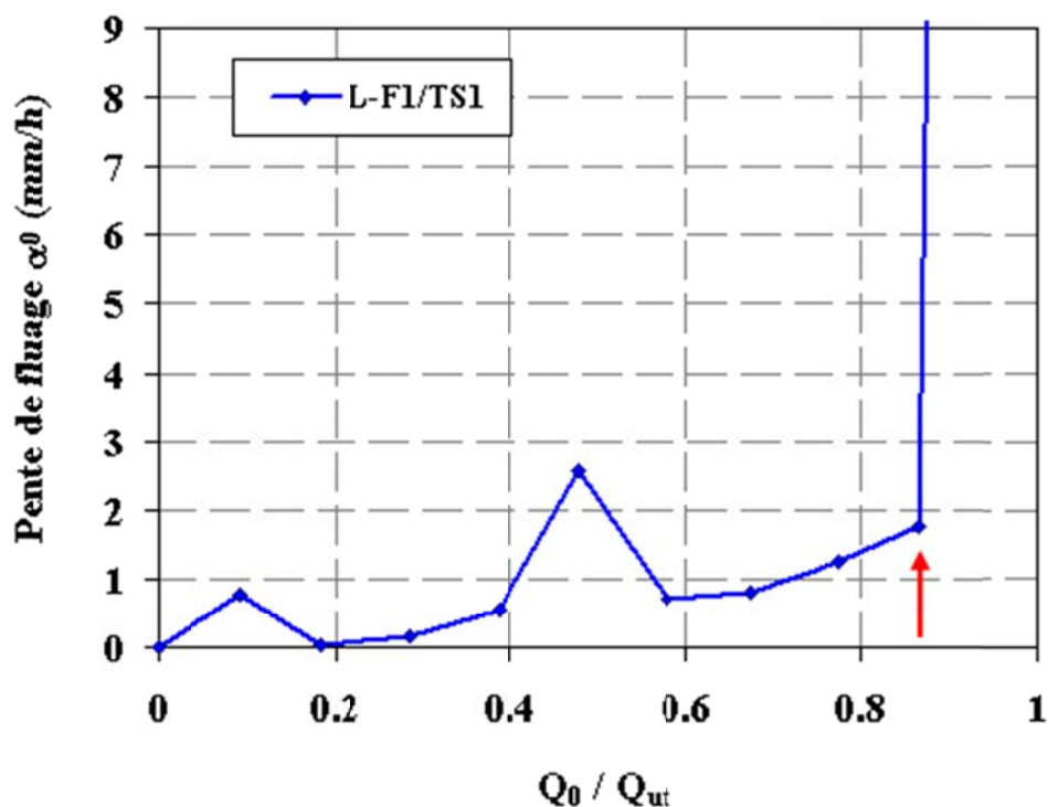
Figure IV-2 : Pente de fluage \alpha_0 en fonction du niveau du chargement Q_0 / Q_{ut} de l'essai L-F1/TS1
