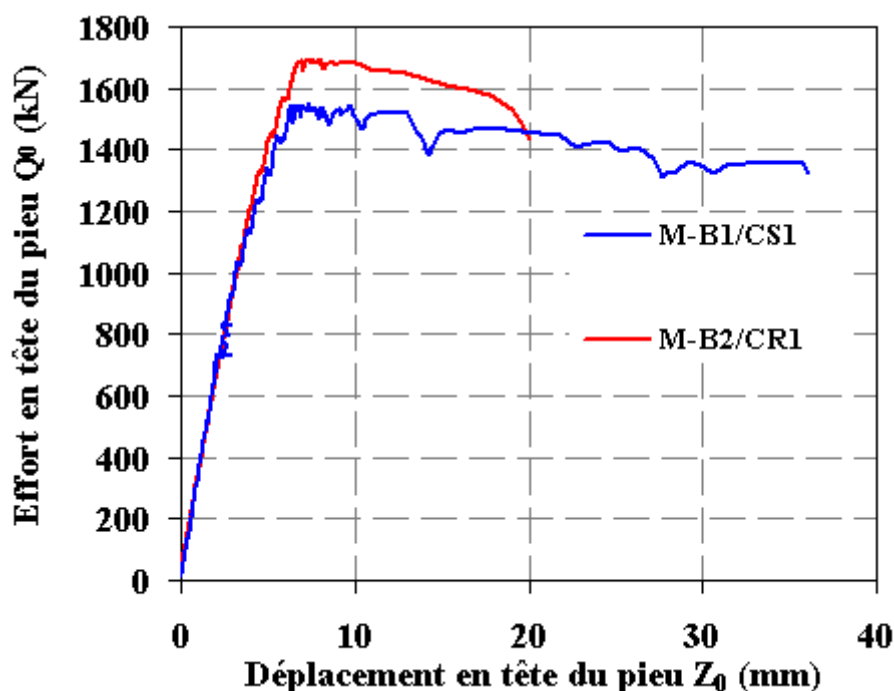
Figure III-12 : Comparaison des courbes effort-déplacement des essais de chargements rapides et celle de l’essai statique NF en compression sur les pieux battus (Merville)
