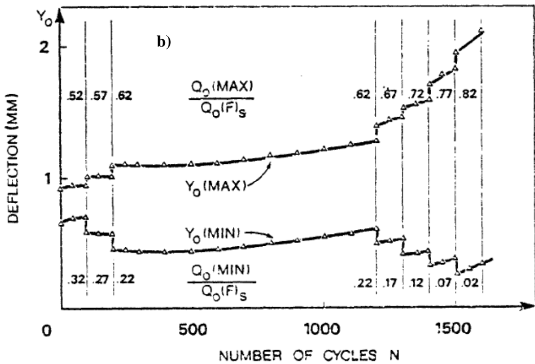
Figure I-21 : Évolution du déplacement du pieu de Plancoët pendant a) l'essai cyclique C11 b) l'essai cyclique T2
