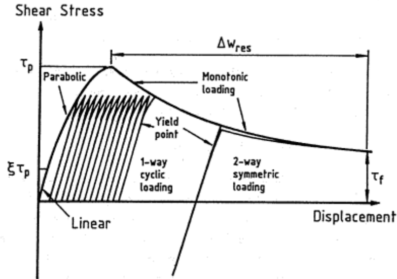
Figure I-45 : Courbe de transfert de charge cyclique utilisé dans le programme RATZ (Chin et Poulos, 1992).
