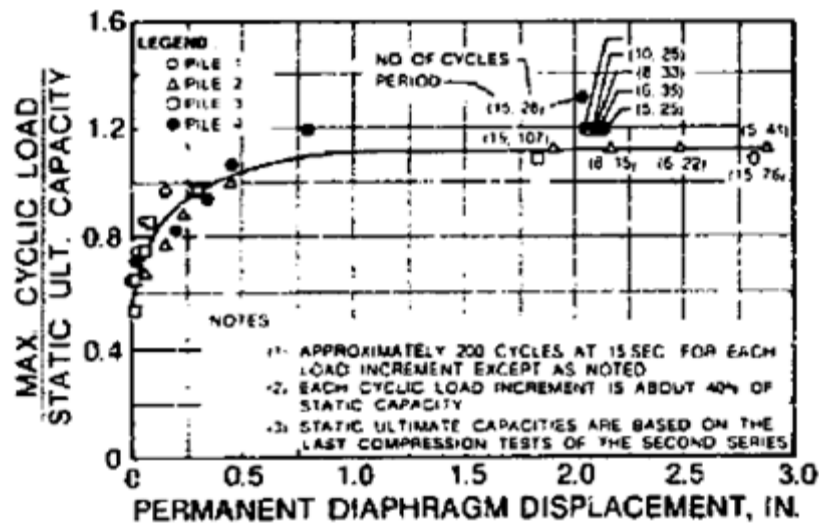
Figure I-16 : Influence du ratio du chargement ( Q_{\max}/Q_{uc} ) sur le déplacement des quatre pieux (Kraft et al., 1981a)
