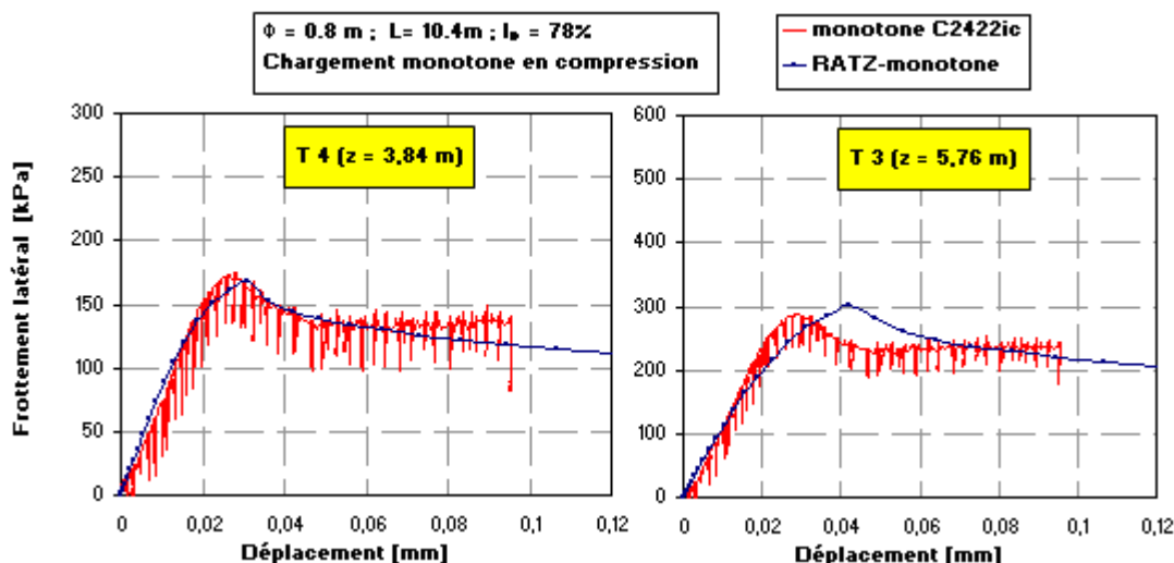
Figure 3. Comparaison entre les essais de compression monotones en centrifugeuse et la modélisation par le programme RATZ
