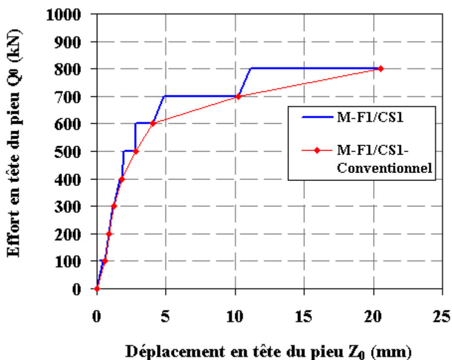
Figure III-1 : Courbe effort-déplacement de l’essai de chargement statique NF en compression M-F1/CS1 (Merville)
