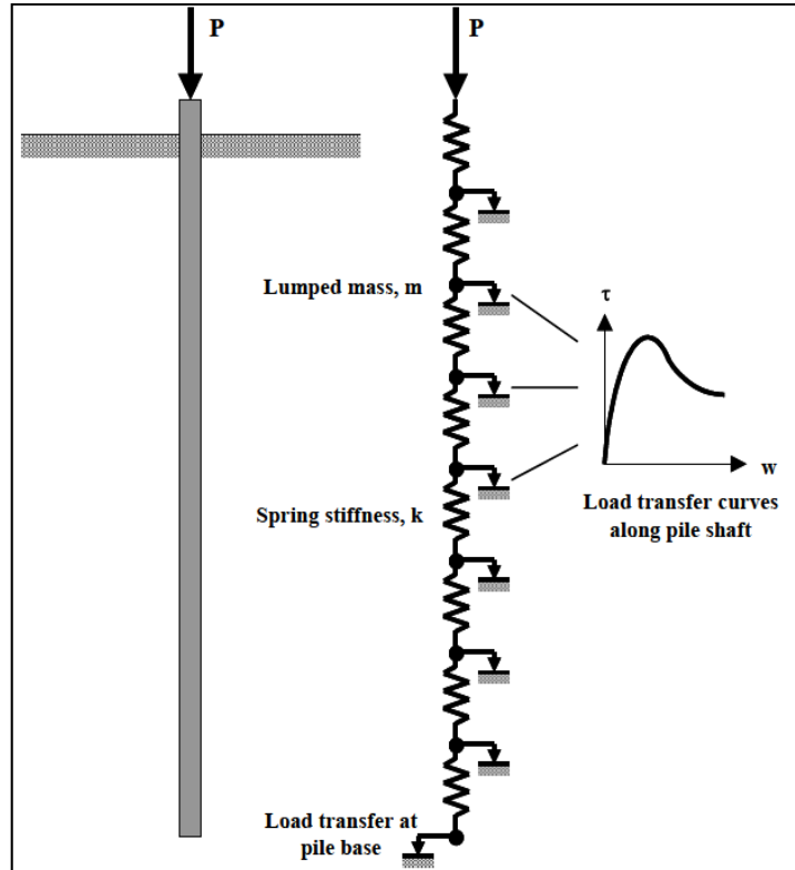
Figure I-43 : discrétisation du pieu dans le logiciel RATZ
