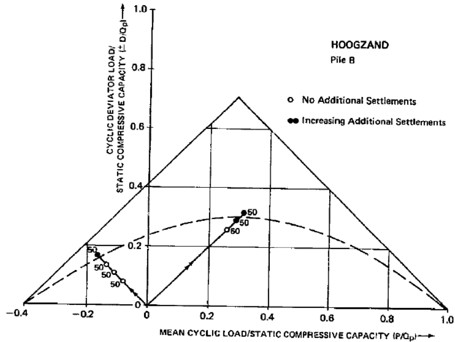
Figure I-35 : Enveloppe cyclique des essais cycliques traction et compression sur pieu B (Heins et Barends, 1979)
