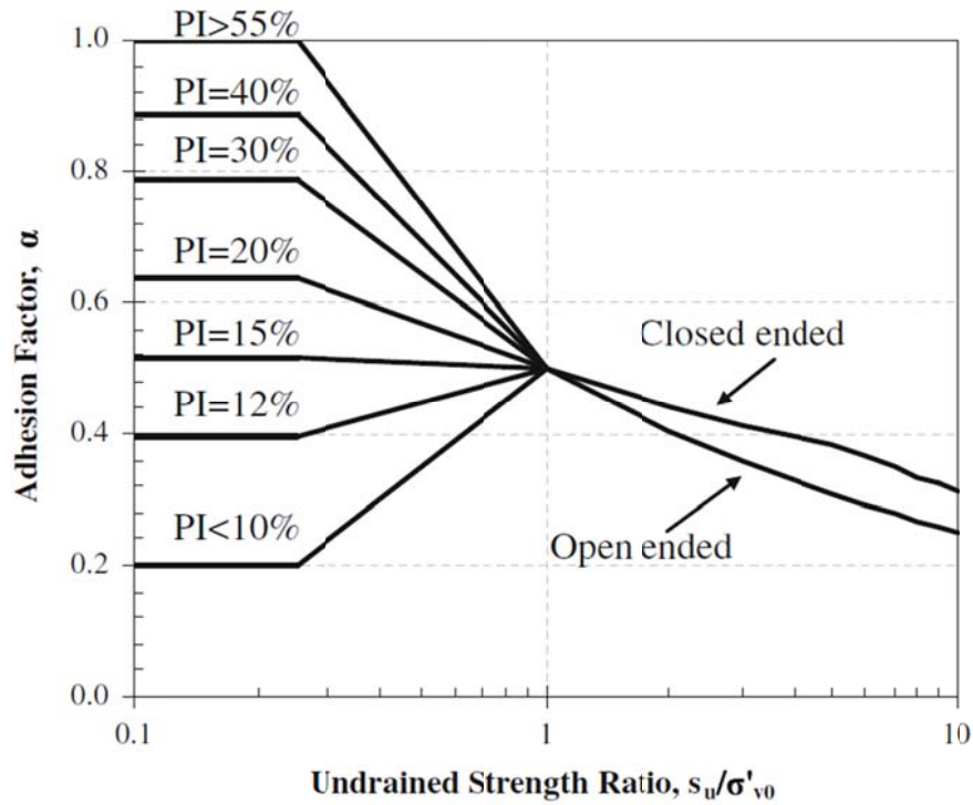
Figure I-9 : Évolution du facteur d'adhérence \alpha en fonction du ratio Cu (S_u)/\sigma'_{v0} (Karlsrud et al, 2005)
