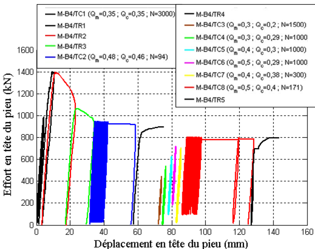
Figure III-49 : Historique de chargements en traction sur le pieu battu B4
