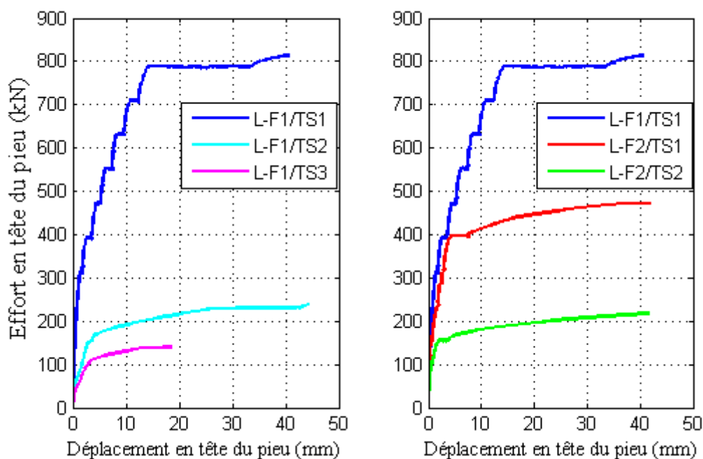
Figure IV-16 : Comparaison entre les différents essais statiques effectués sur le pieu F1 et F2.
