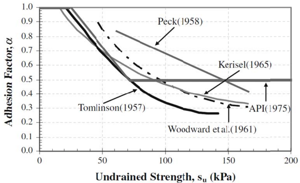
Figure I-8 : Évolution du facteur d'adhérence \alpha en fonction la résistance au cisaillement non drainée C_u ( S_u ) (Chow, 1997)
