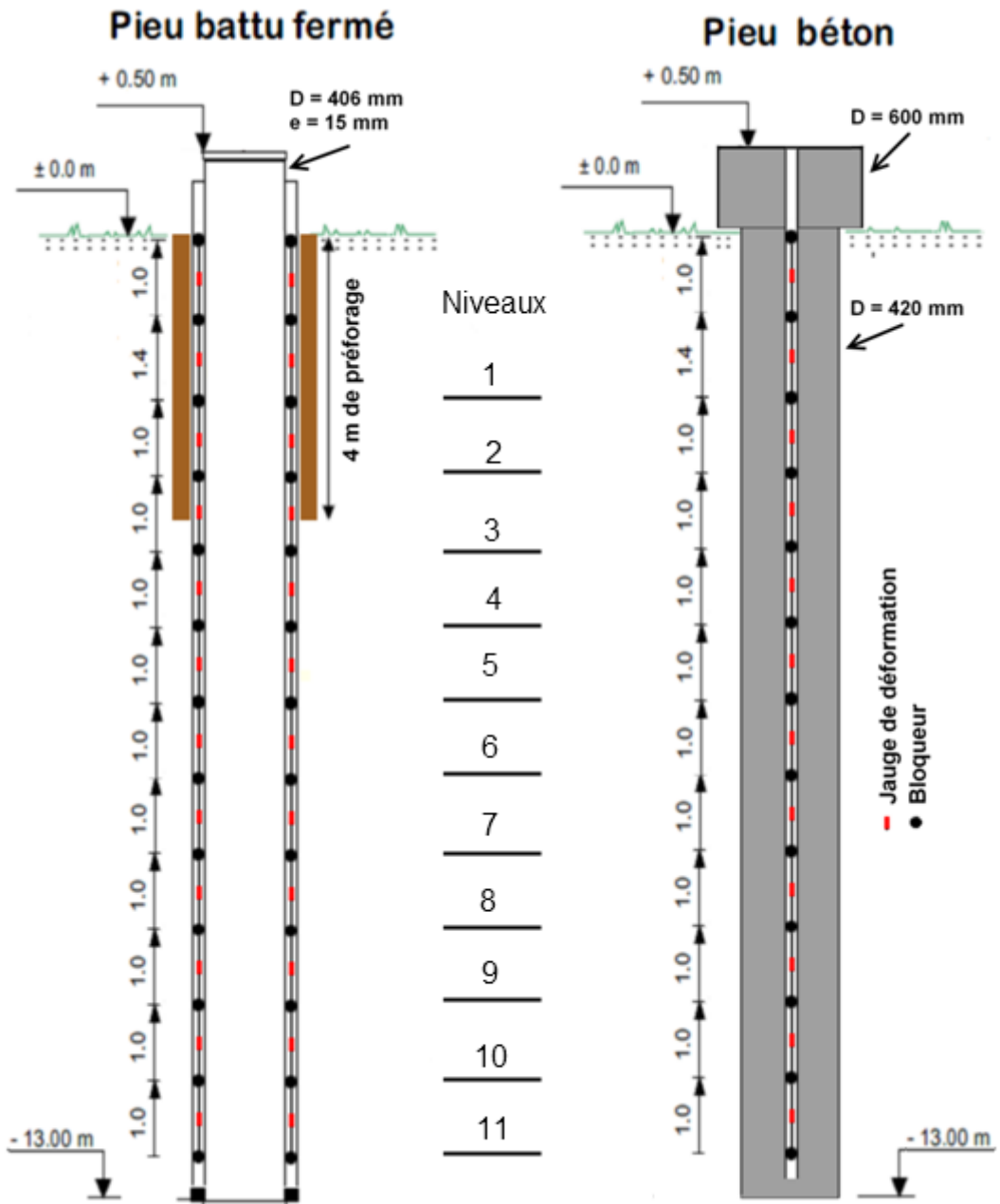
Figure II-24 : Schéma descriptif de l'instrumentation des pieux de Merville
