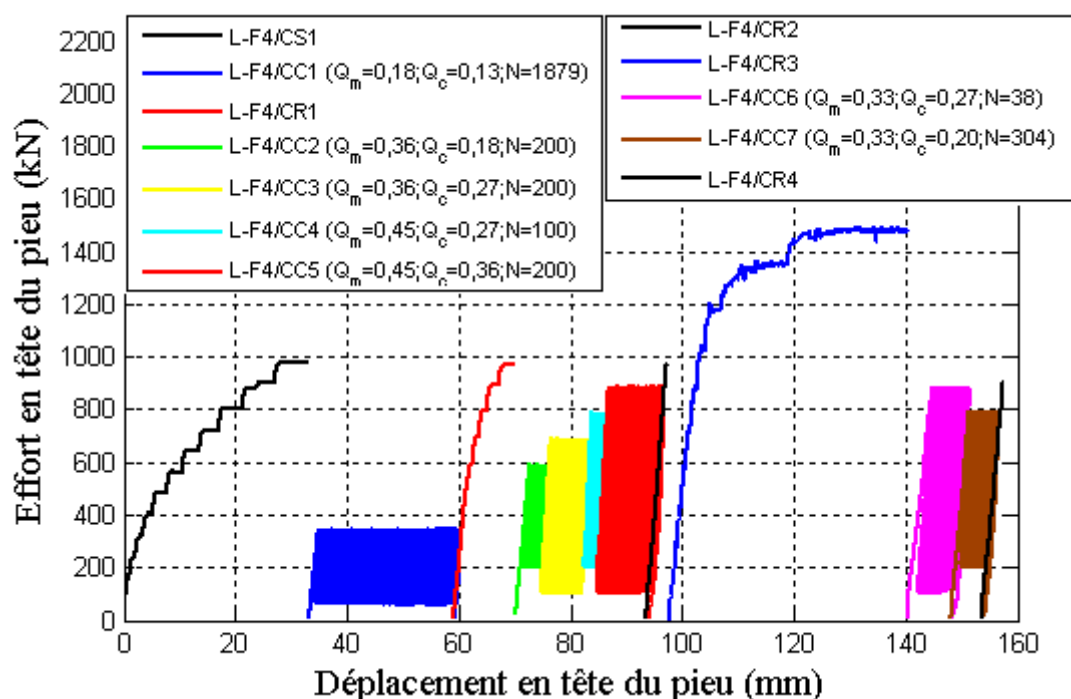
Figure IV-19 : Historique de chargements sur le pieu foré F4
