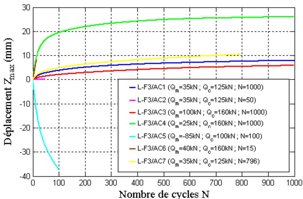
Figure IV-35 : Evolution du déplacement Z_{max} en fonction du nombre de cycle des différentes combinaisons cycliques effectuées sur le pieu F3.
