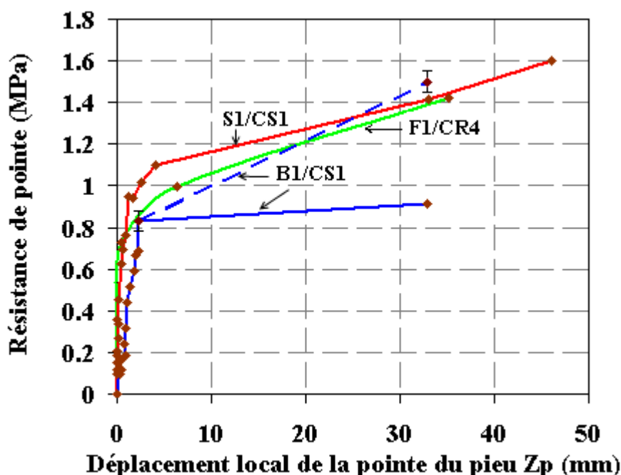
Figure III-21 : Comparaison de la mobilisation des résistances de pointe des trois types de pieu.
