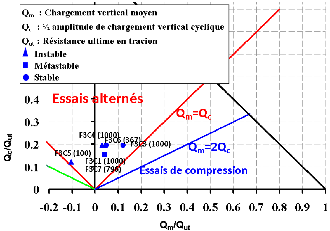
Figure IV-38 : Diagramme de stabilité cyclique des pieux forés en alternés à Loon-Plage
