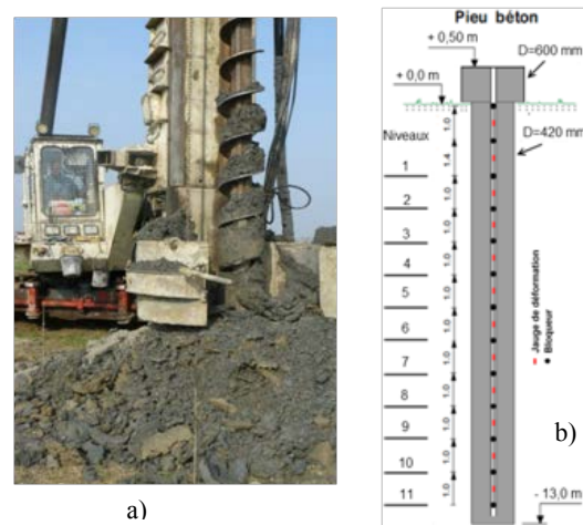
Figure 3. Pieux forés a) tarière à axe creux. b) schéma d'instrumentation à l'aide d'extensomètres amovibles de type LCPC.
