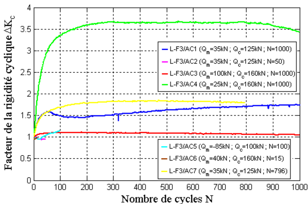
Figure IV-36 : Facteur d'évolution de la rigidité cyclique en fonction du nombre de cycle des différentes combinaisons cycliques effectuées sur le pieu F3.
