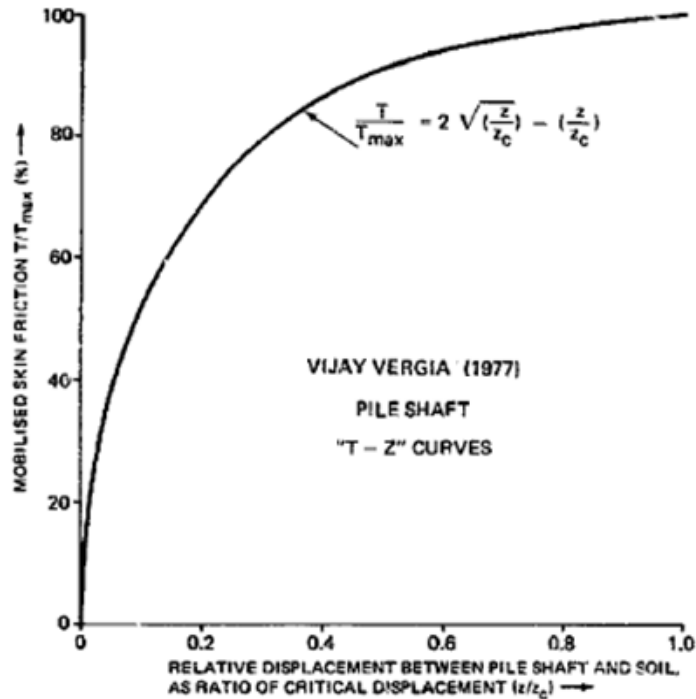
Figure I-10: Courbe T-Z proposé par VijayVergia (1977)
