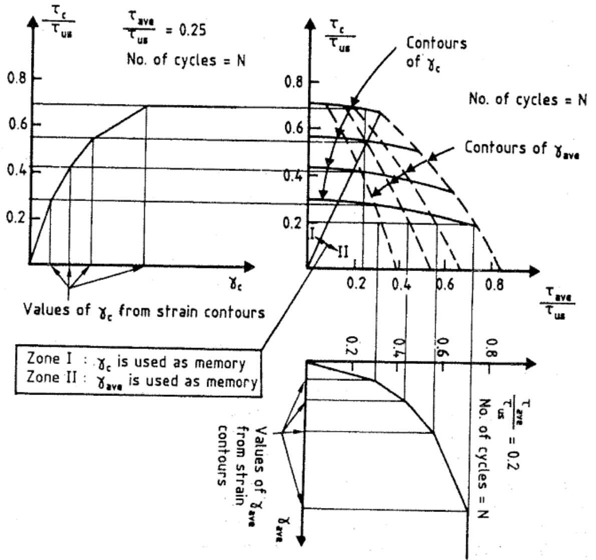
Figure I-49 : construction de T-Z à partir des diagrammes contours DSS (Karlsruud et al., 1986)
