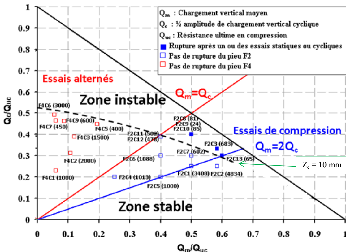
Figure III-42 : Diagramme de stabilité cyclique des pieux forés à Merville
