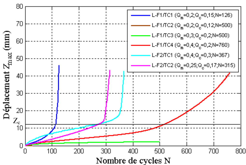
Figure IV-14 : Evolution du déplacement Z_{max} en fonction du nombre de cycle des différentes combinaisons cycliques effectuées sur les deux pieux F1 et F2.
