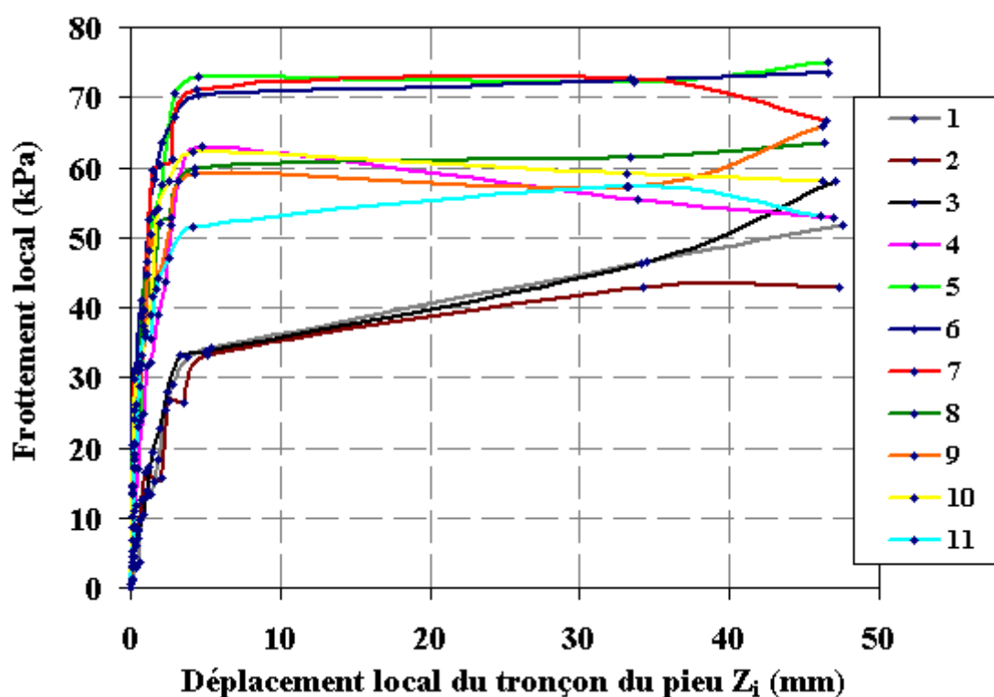
Figure III-17: Frottements latéraux mobilisés le long du pieu lors de l’essai du chargement statique pour l’essai M-S1/CS1
