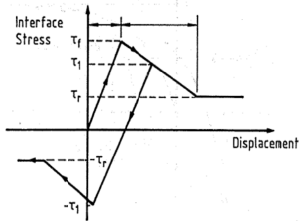
Figure I-39 : courbe d'interface avec radoucissement élasto-plastique de SCARP
