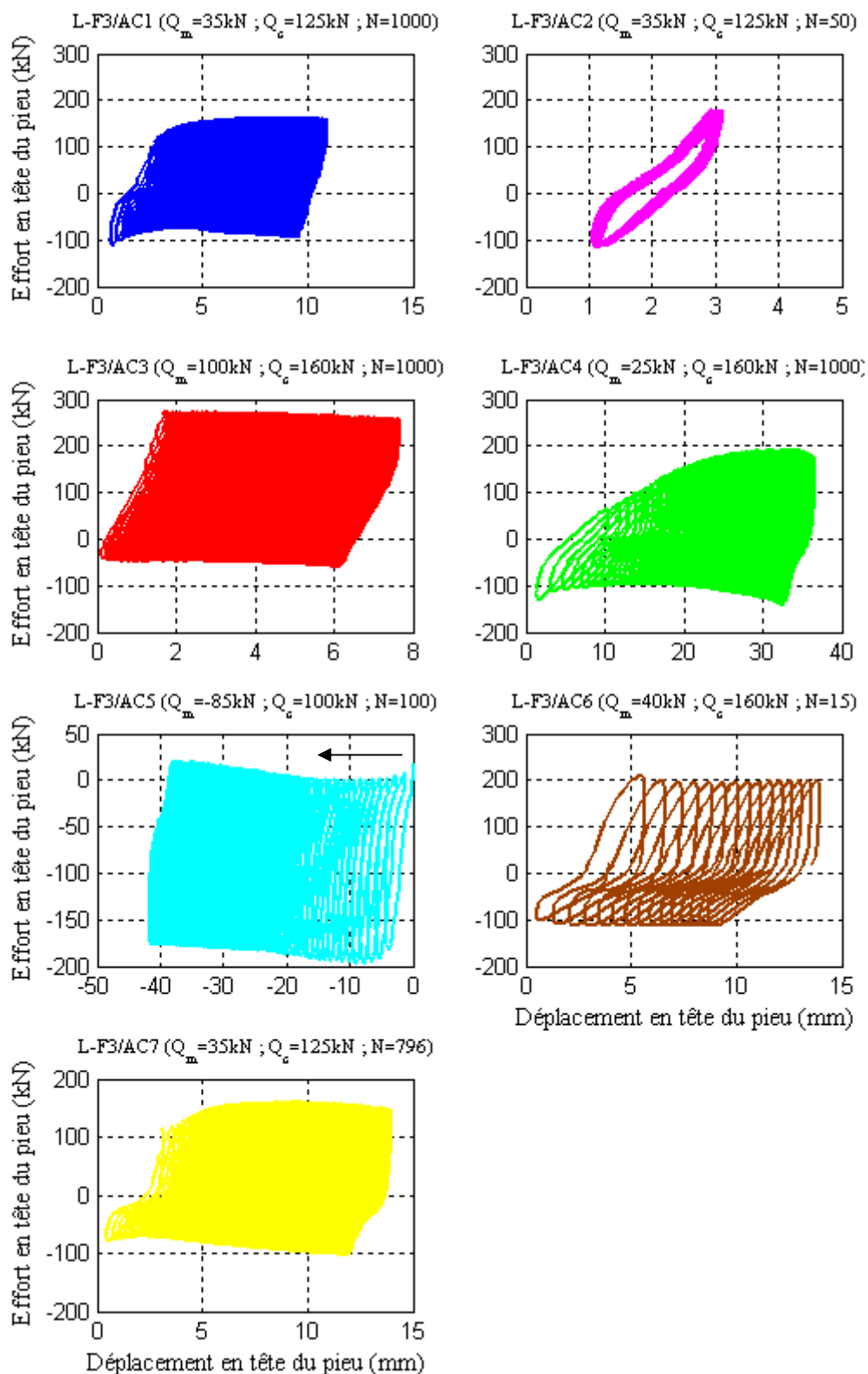
Figure IV-34 : Courbes effort-déplacement des essais cycliques sur le pieu F3
