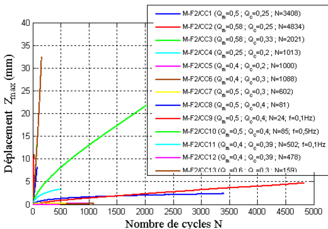
Figure III-27 : Evolution du déplacement Z_{max} en fonction du nombre de cycle des différentes combinaisons cycliques effectuées sur le pieu F2.
