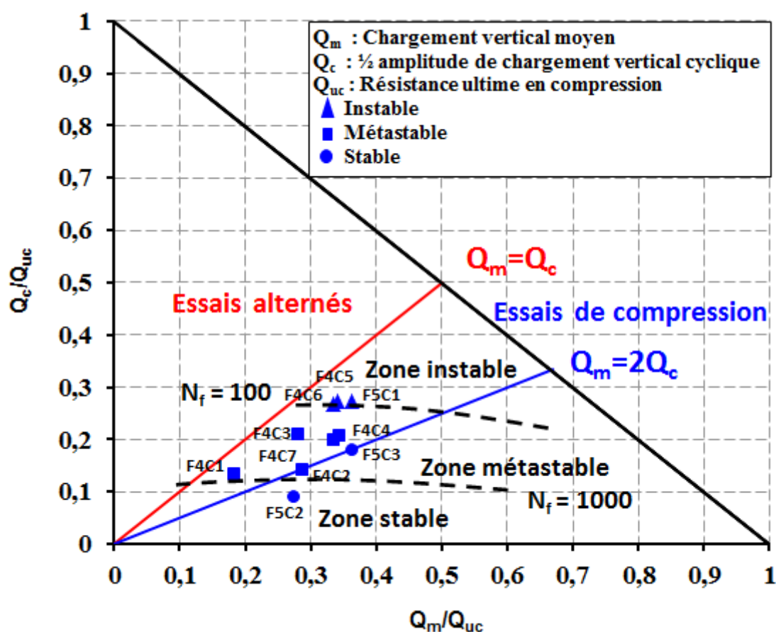
Figure IV-32 : Diagramme cyclique des pieux forés en compression à Loon-Plage
