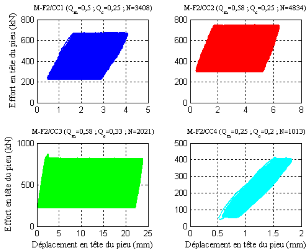
Figure III-25 : Courbes effort-déplacement des essais cycliques sur le pieu F2
