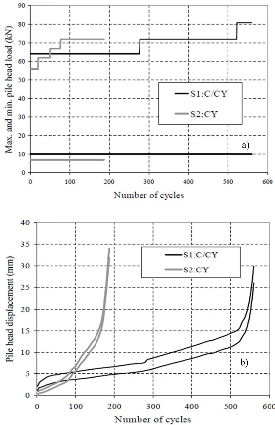
Figure I-32 : a) Les niveaux de chargements cycliques b) les déplacements en tête de pieux des deux pieux S1: C/CY et S2: CY.
