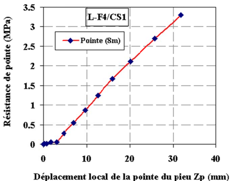
Figure IV-7 : Évolution de la résistance de pointe lors de l'essai du chargement statique L-F4/CS1
