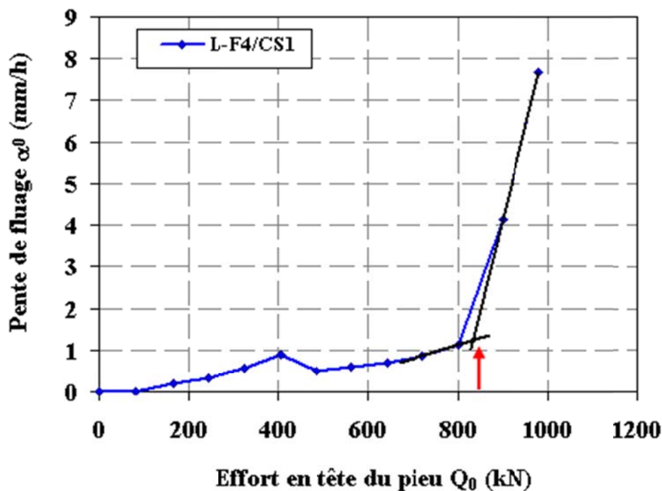
Figure IV-4 : Pente de fluage \alpha_0 en fonction du chargement en tête Q_0 de l'essai L-F4/CS1
