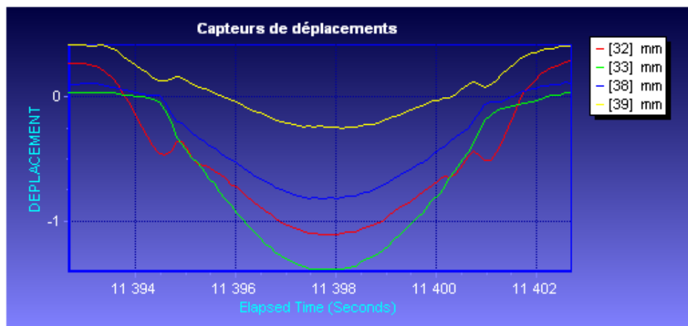
Figure II-30 : Mesure en temps réel des 4 capteurs de déplacement.
