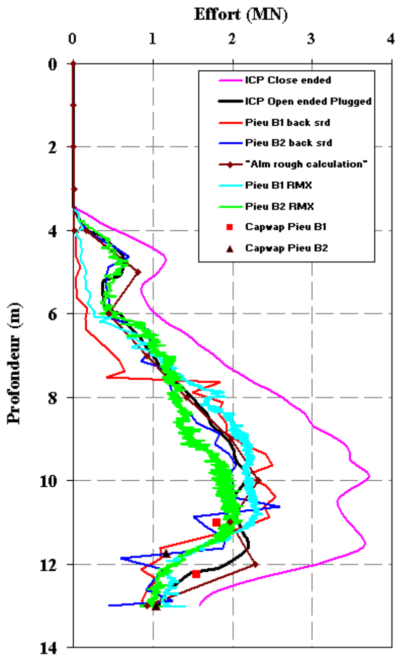
Figure IV-9 : La capacité des pieux battus estimée à partir de l'instrumentation du battage et les méthodes prévisionnelles.
