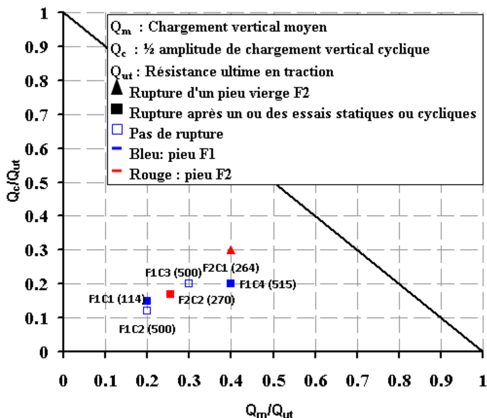
Figure IV-17 : Diagramme de stabilité cyclique des pieux forés en traction à Loon-Plage
