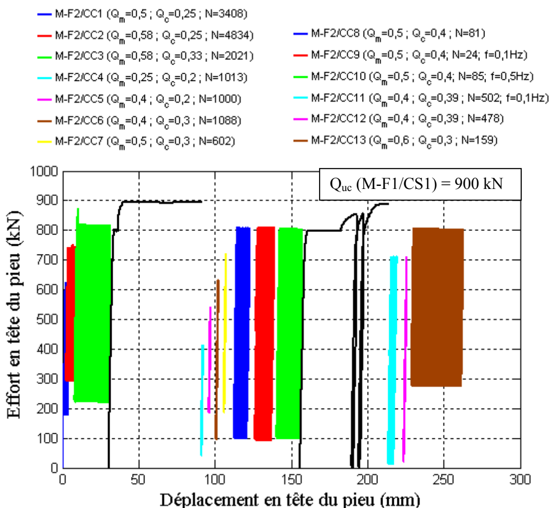
Figure III-24 : Historique de chargements sur le pieu foré F2
