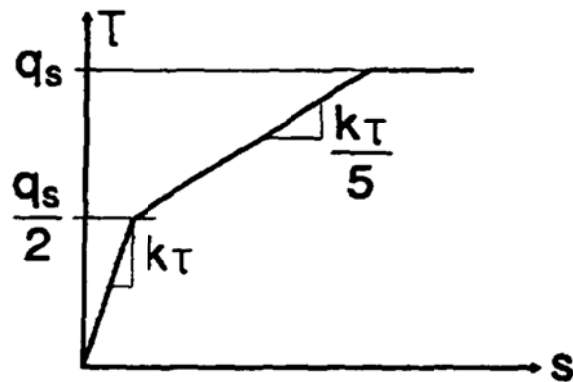
Figure I-12 : Courbe T-Z (Frank et Zhao, 1982)
