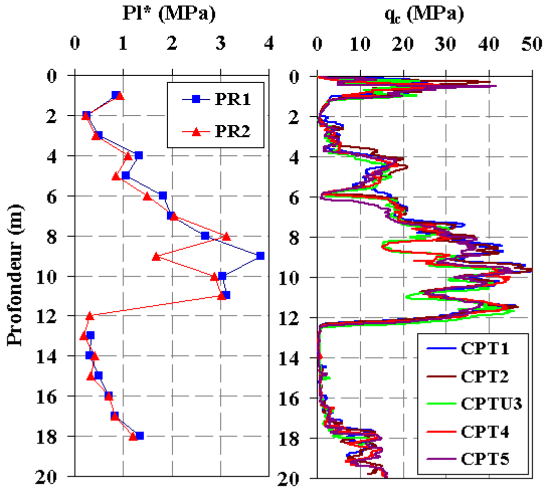
Figure II-8 : Variation de la pression limite nette (PI*) et la résistance de pointe (qc) en fonction de la profondeur (site de Loon-Plage).
