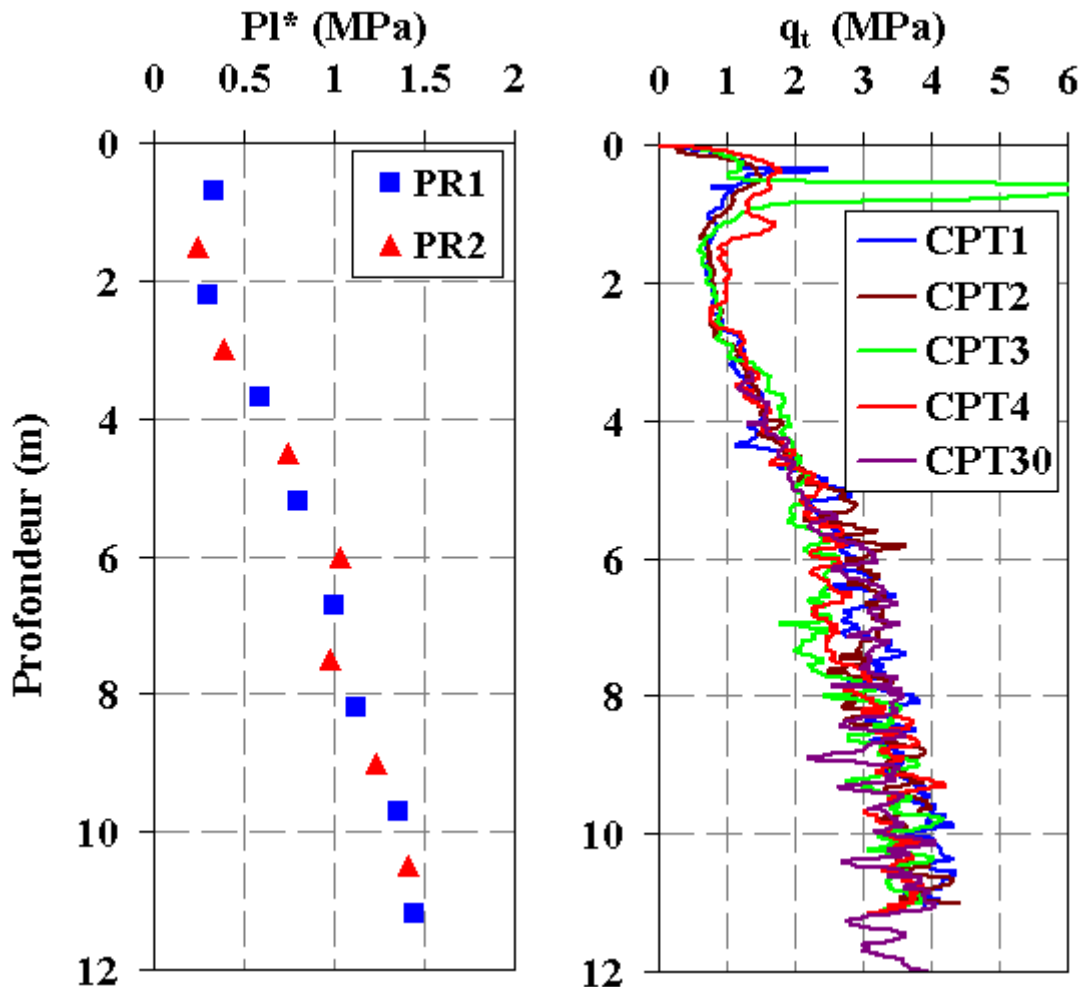
Figure II-3 : La variation de la pression limite nette ( PI^* ) et la résistance de pointe nette ( q_t ) en fonction de la profondeur (site de Merville).
