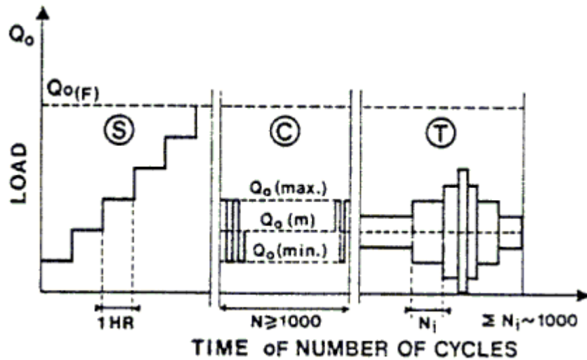
Figure I-19 : Types de chargements appliqués sur le pieu de Plancoët: charge statique (S), cyclique (C) et tempête (T)
