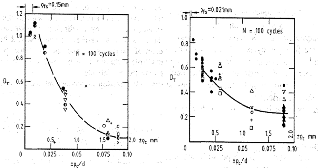
Figure I-41 : Evolution du ratio de dégradation du frottement en fonction de l'amplitude du déplacement cyclique imposé normalisé par le diamètre du pieu a) moulé b) foncé.
