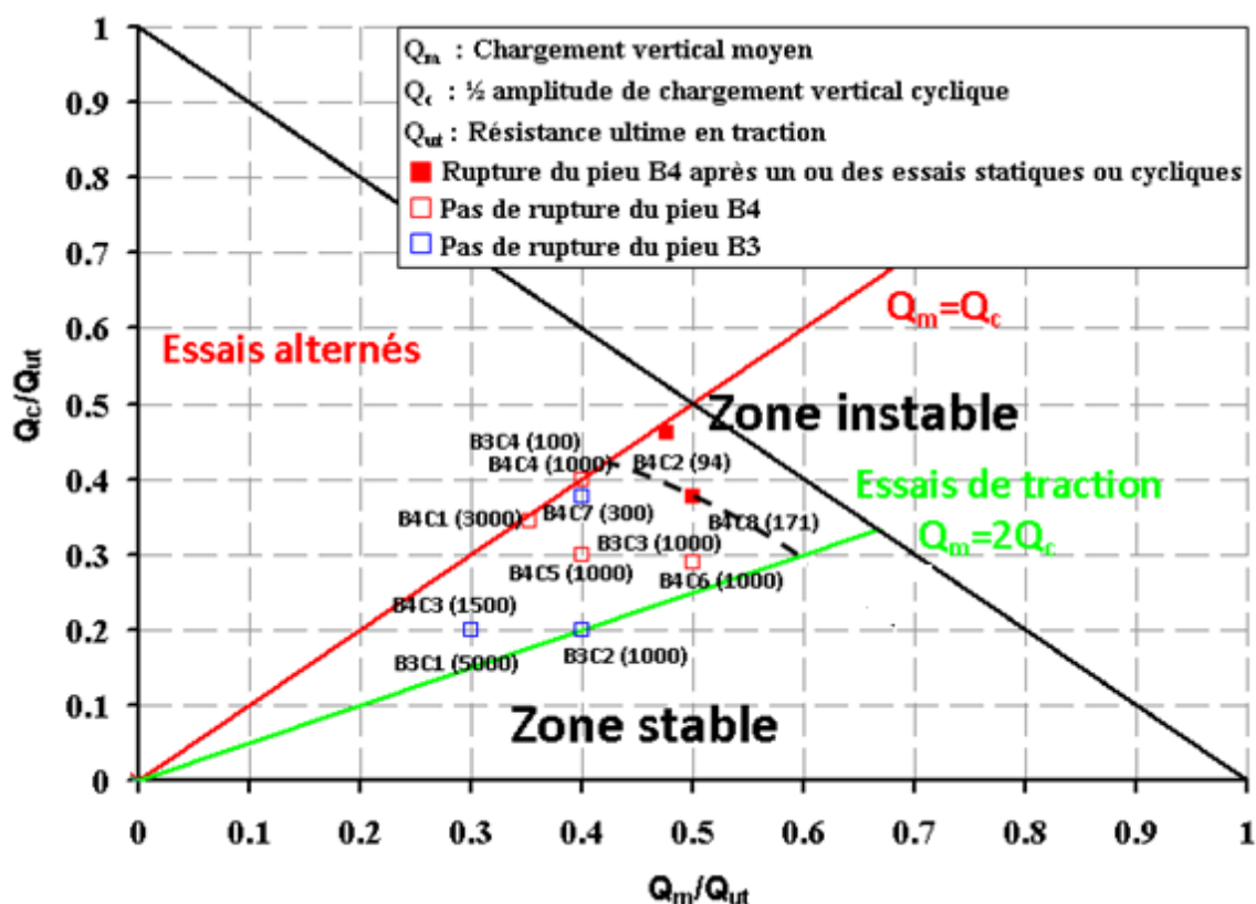
Figure III-54 : Diagramme de stabilité cyclique des pieux battus en traction à Merville
