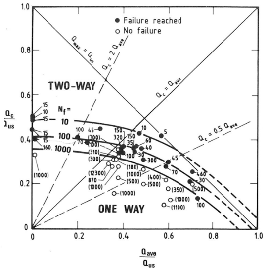
Figure I-29 : Le nombre de cycles à la rupture des pieux d'Haga en fonction de Q_{moy} et Q_{cyc} normalisés par la capacité statique Q_{us} de traction (Karlsrud et Haugen, 1985b).
