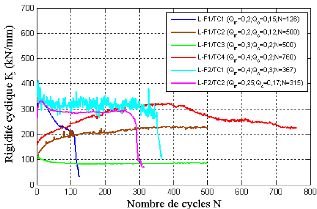
Figure IV-15 : Evolution de la rigidité cyclique en fonction du nombre de cycle des différentes combinaisons cycliques effectuées sur les deux pieux F1 et F2.
