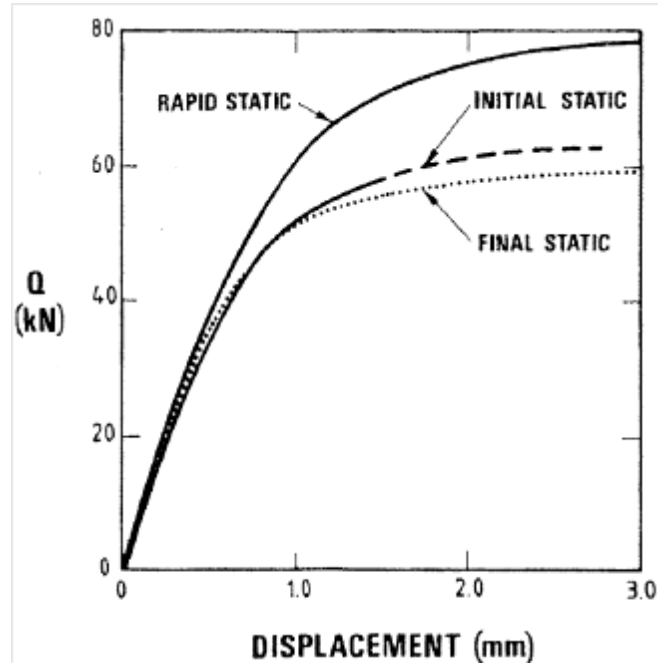
Figure I-7 : Courbes typiques effort-déplacement en tête du pieu dans l'argile de Haga (Karlsrud and Haugen, 1985b)
