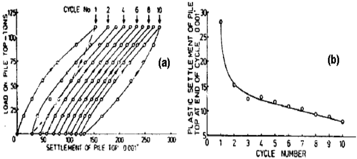
Figure I-33 : Courbes (a) efforts-déplacements (b) déformation plastique en fonction du nombre de cycles (Chan, 1975)
