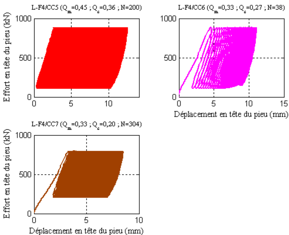
Figure IV-22 : Courbes effort-déplacement des essais cycliques sur le pieu F5
