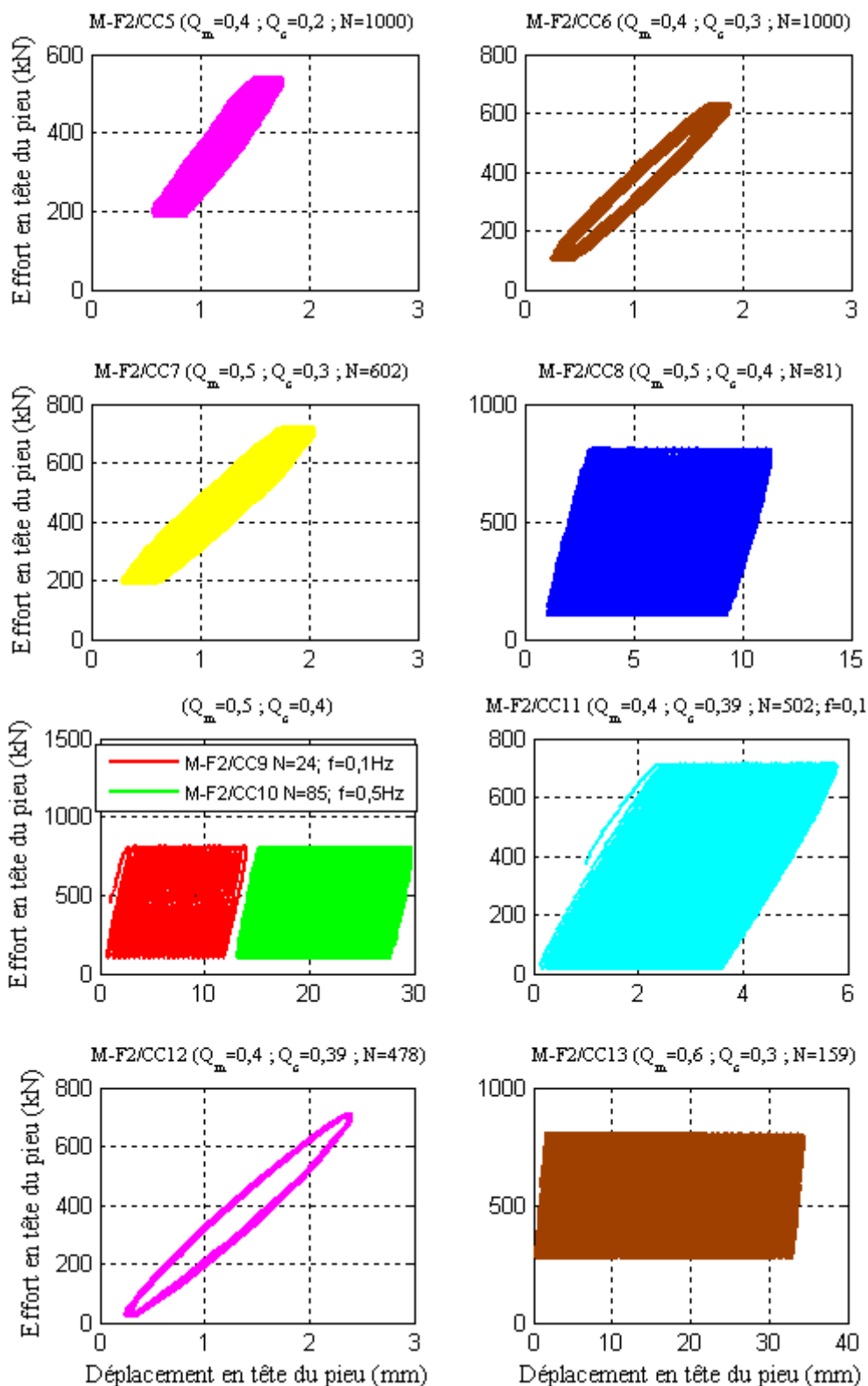
Figure III-26 : Courbes effort-déplacement des essais cycliques sur le pieu F2 (suite)
