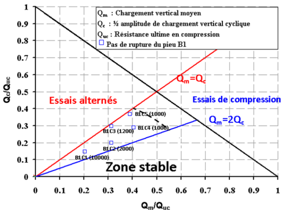
Figure III-53 : Diagramme de stabilité cyclique des pieux battus en compression à Merville
