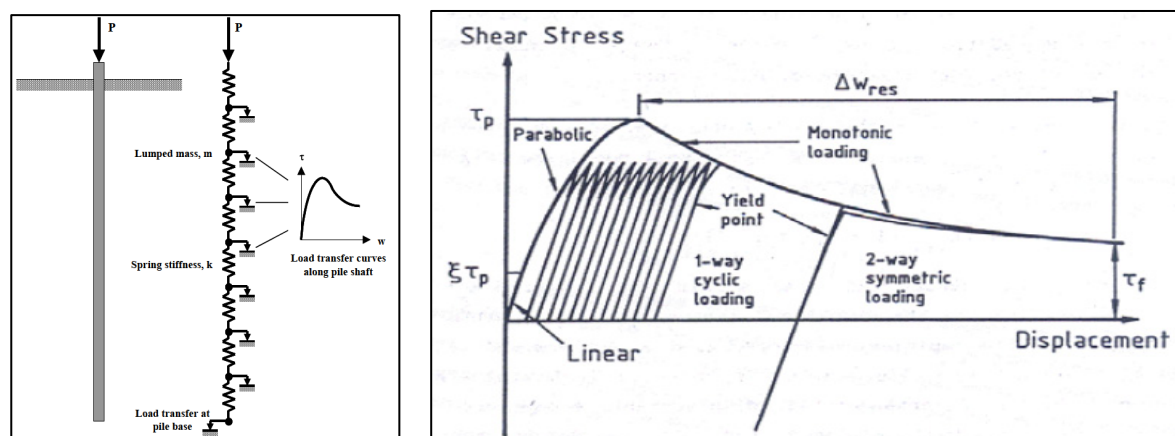
Figure 1. Courbe de transfert de charge utilisé dans le programme RATZ (Chin et Poulos, 1992).
