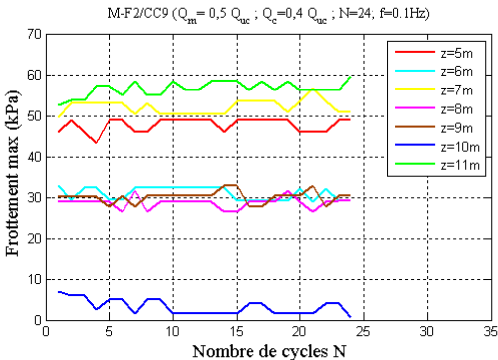
Figure III-37 : Frottement maximal développé sur les couches de l’argile des Flandres durant la séquence M-F2/CC9
