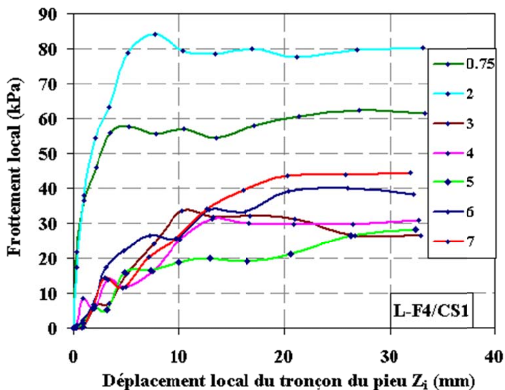
Figure IV-6: Frottements latéraux mobilisés le long du pieu lors de l'essai de chargement statique L-F4/CS1
