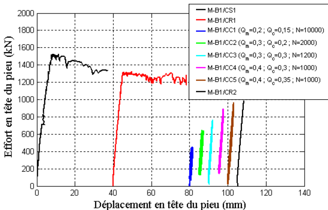
Figure III-46 : Historique de chargements en compression sur le pieu battu B1
