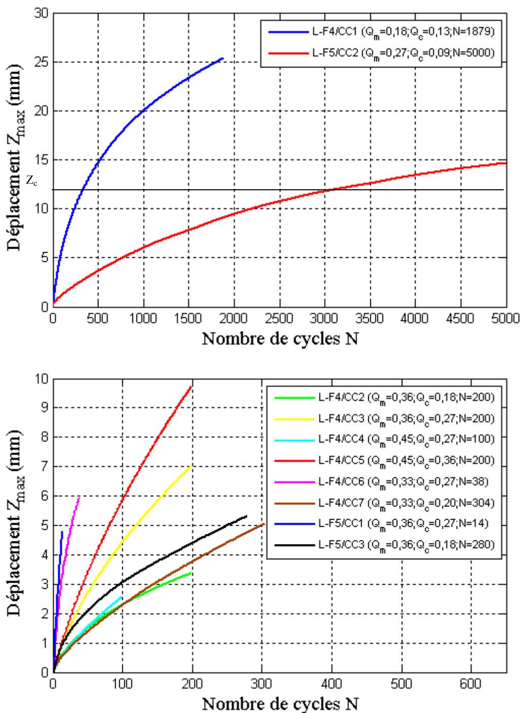
Figure IV-23 : Evolution du déplacement Z_{max} en fonction du nombre de cycle des différentes combinaisons cycliques effectuées sur les deux pieux F4 et F5.
