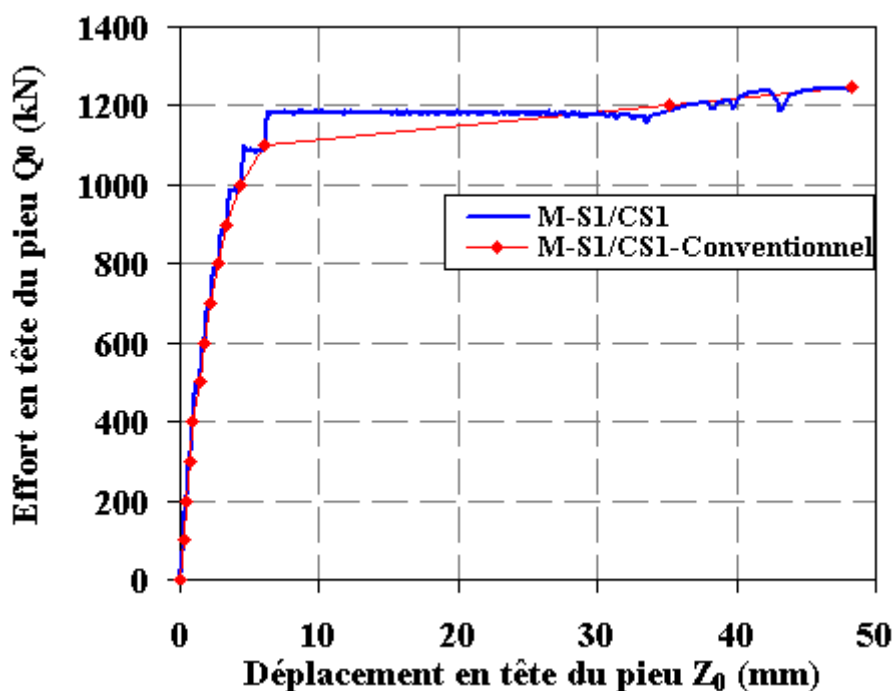
Figure III-14 : Courbe effort-déplacement de l’essai de chargement statique NF en compression M-S1/CS1 (Merville)
