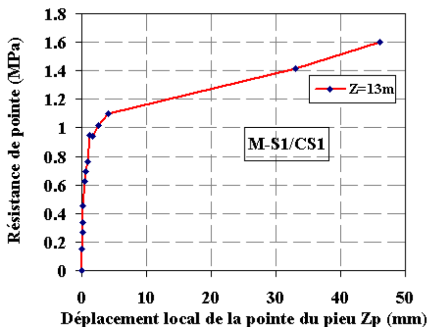
Figure III-18 : Évolution de la résistance de pointe lors de l’essai du chargement statique M-S1/CS1
