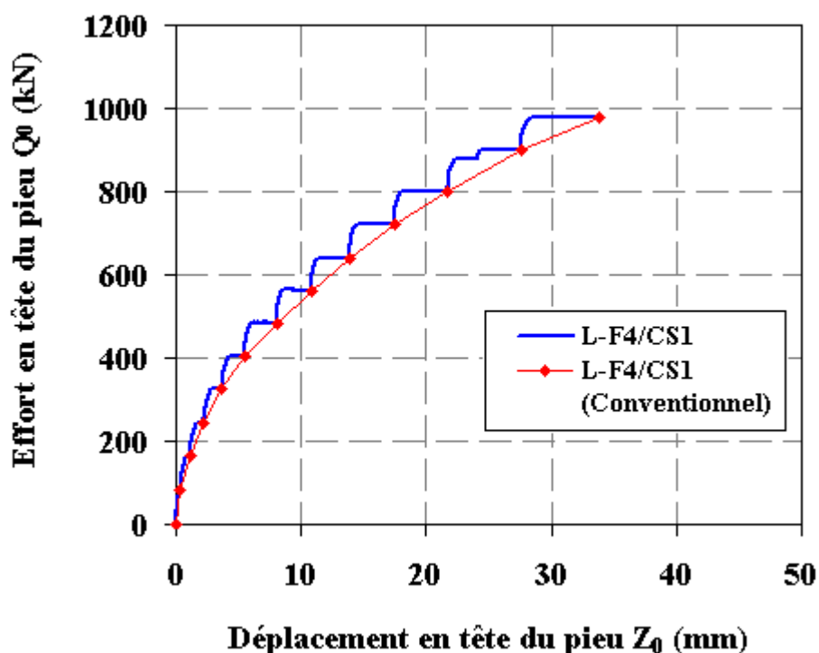
Figure IV-3 : Courbe effort-déplacement de l'essai de chargement statique NF en compression L-F4/CS1 (Loon-Plage)
