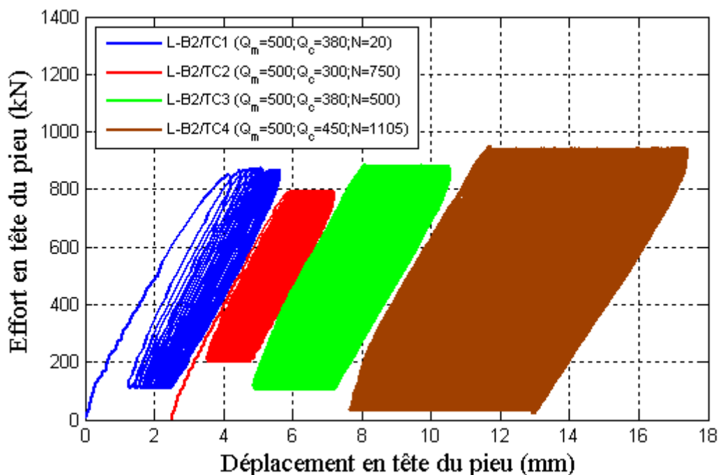
Figure IV-39 : Historique de chargements en traction sur le pieu battu B2
