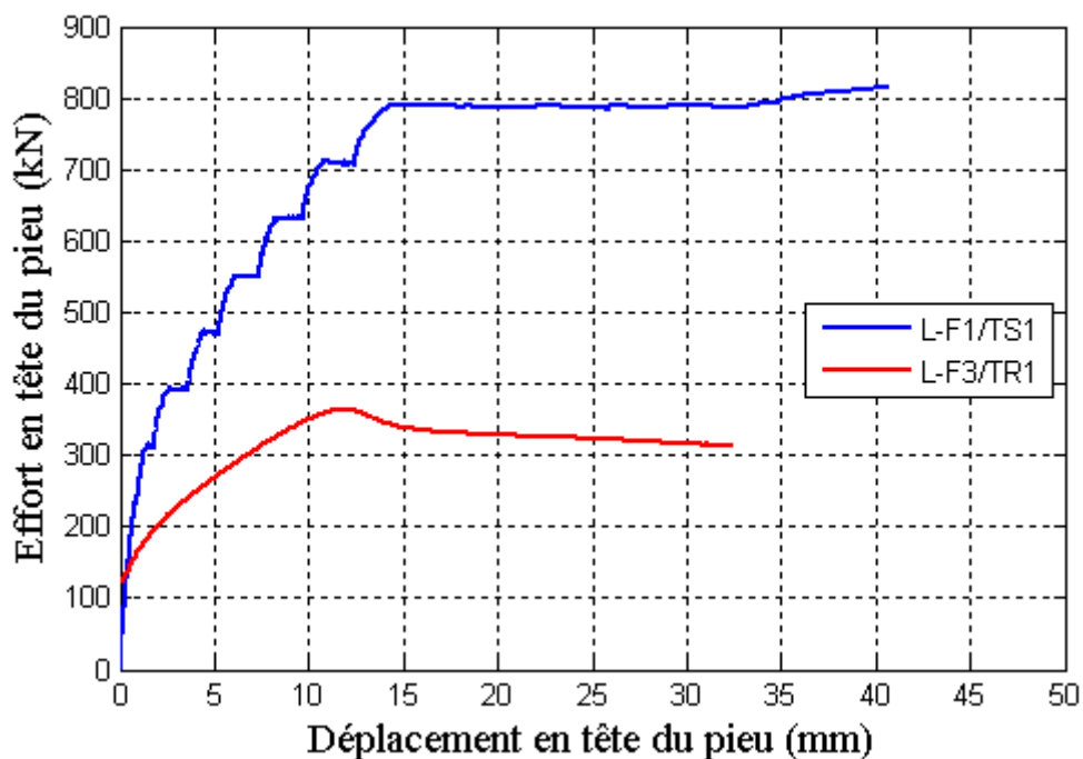
Figure IV-37 : Comparaison entre l'essai statique N-F en traction effectué sur le pieu F1 (L-F1/TS1) et l'essai rapide effectué sur le pieu F3 (L-F3/TR1).
