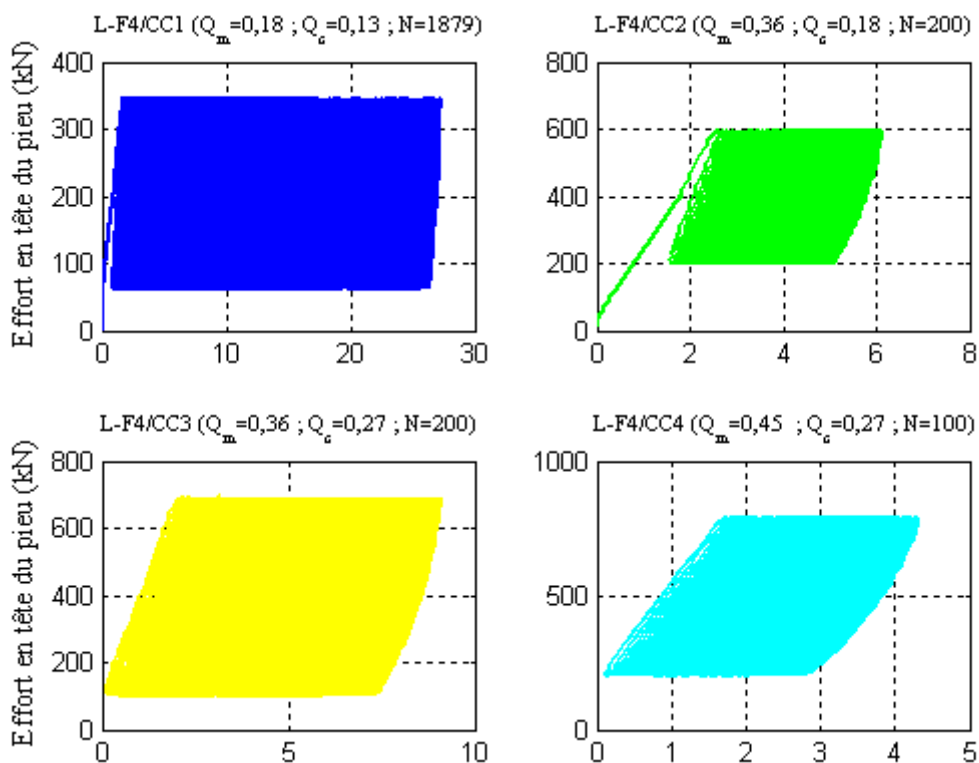
Figure IV-21 : Courbes effort-déplacement des essais cycliques sur le pieu F4
