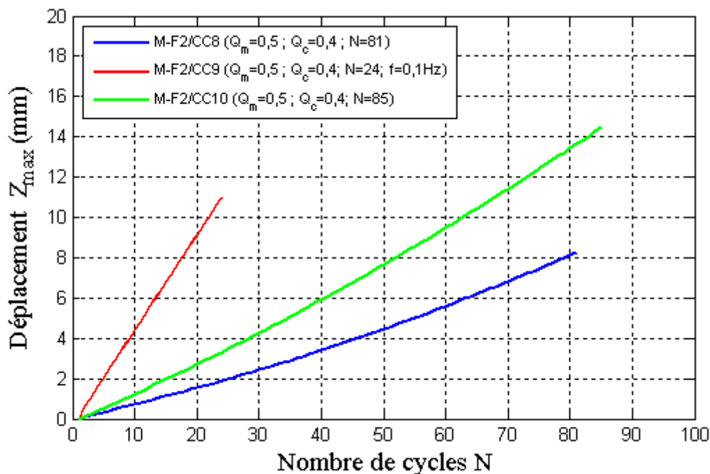
Figure III-29 : Influence de la fréquence sur l'accumulation de déplacement en tête du pieu F2 sous la combinaison de chargement cyclique ( Q_m= 0,5 et Q_c=0,4 )
