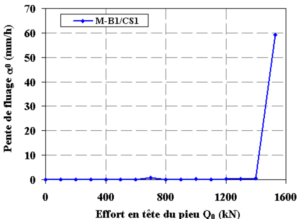
Figure III-8 : Pente de fluage \alpha_0 en fonction du chargement en tête Q_0 de l’essai M-B1/CS1
