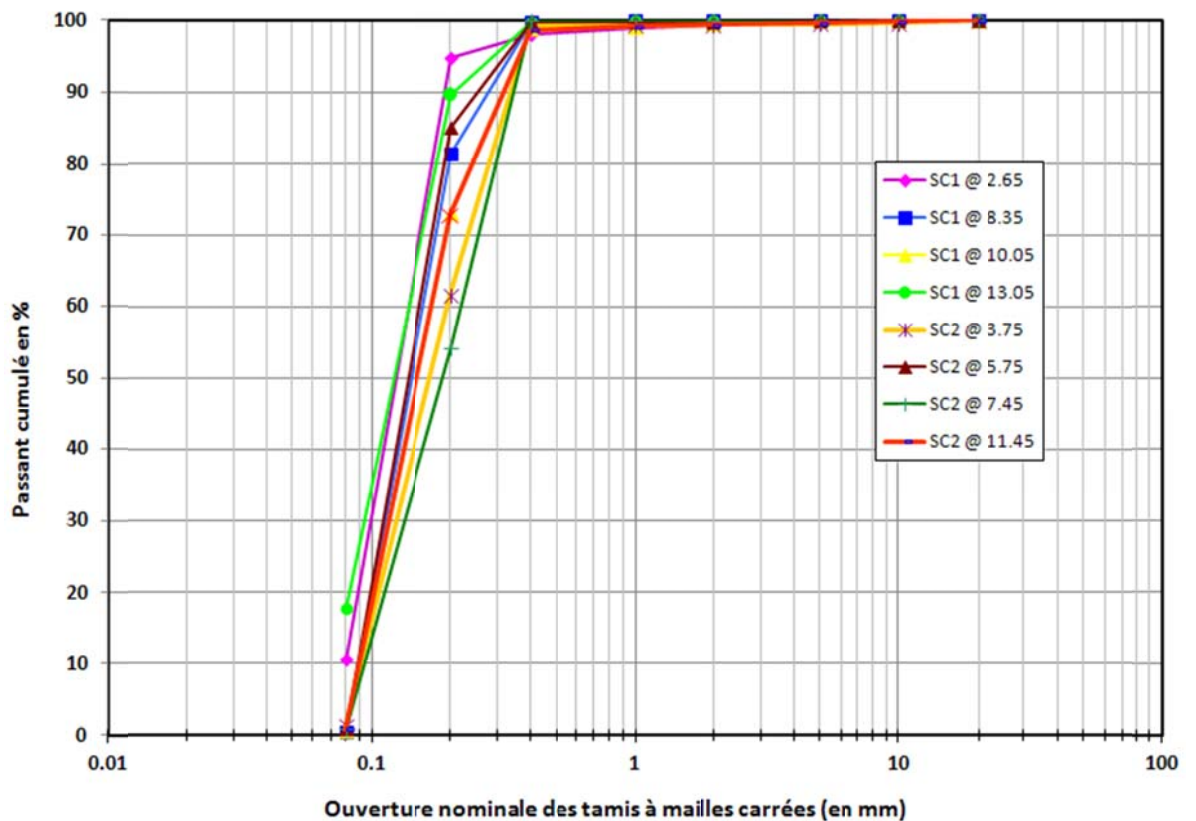
Figure II-9 : Courbes granulométriques du sable de Loon-Plage à différentes profondeurs
