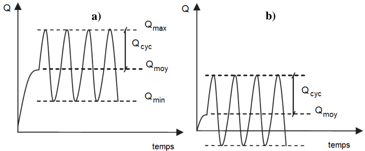
Figure I-15 : Schéma des différents types de chargement cyclique : a) non alterné b) alterné
