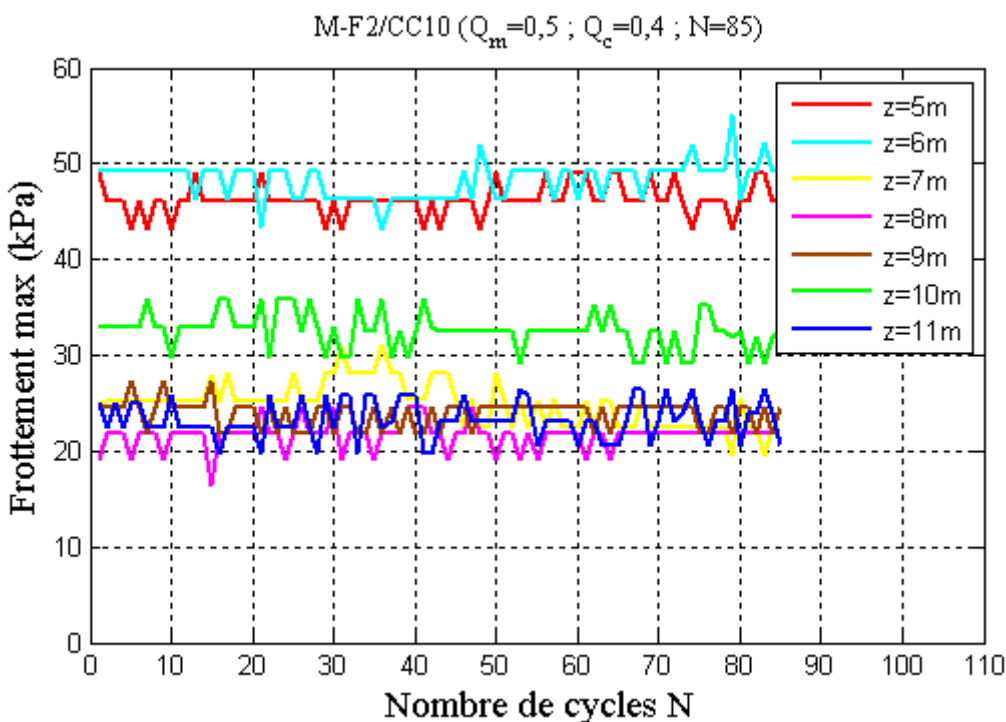
Figure III-38 : Frottement maximal développé sur les couches de l’argile des Flandres durant la séquence M-F2/CC10
