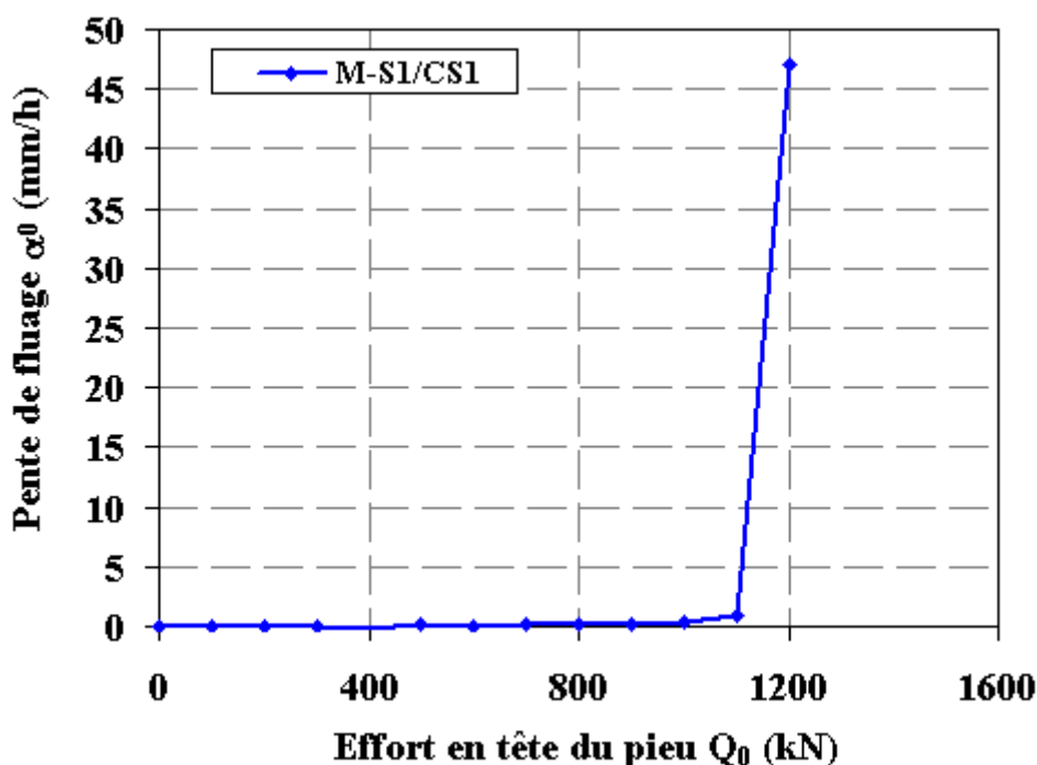
Figure III-15 : Pente de fluage \alpha_0 en fonction du chargement en tête Q_0 de l’essai M-S1/CS1
