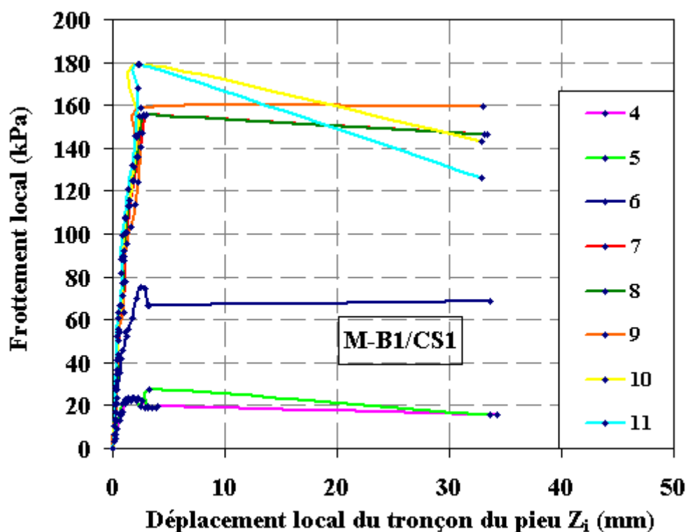
Figure III-10: Frottements latéraux mobilisés le long du pieu battu lors de l’essai du chargement statique pour l’essai M-B1/CS1
