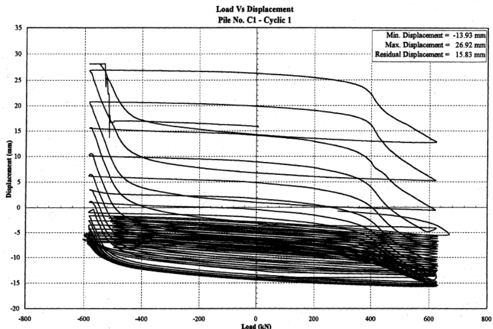
Figure I-36 : Courbe effort-déplacement pour le test 2.C1.CY3. (Jardine and Standing, 2000).
