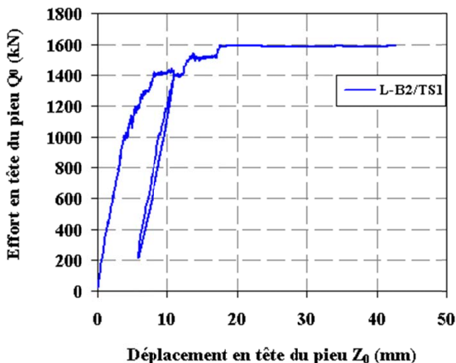
Figure IV-42 : Courbe effort-déplacement de l'essai de chargement statique en traction L-B2/TS1
