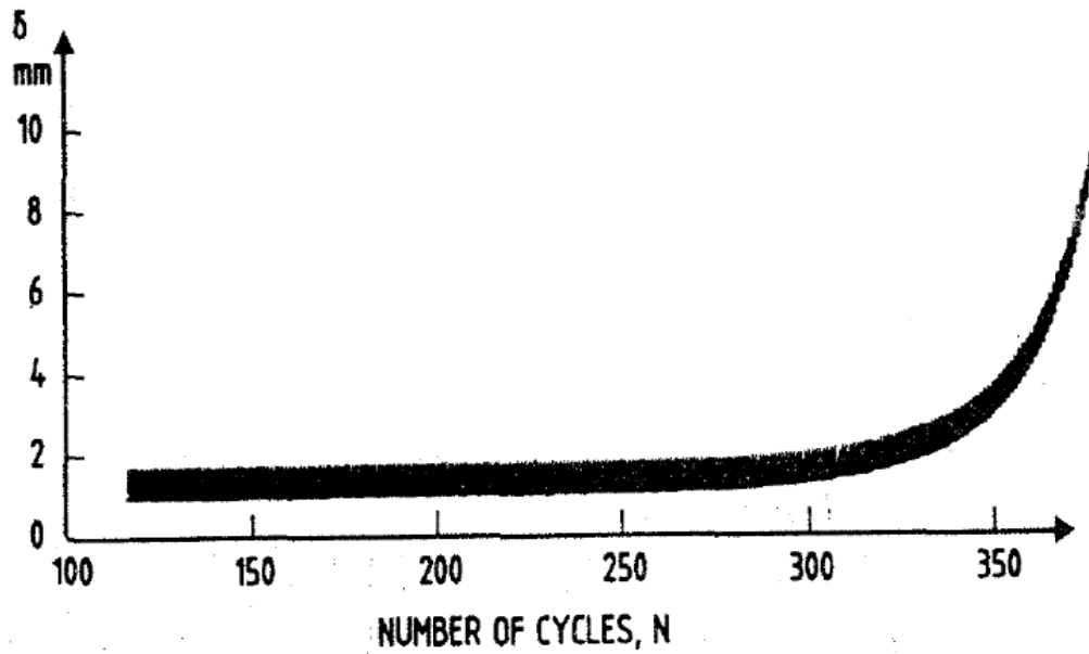
Figure I-27 : Évolution des déplacements en tête du pieu durant un essai de chargement cyclique répété ( Q_{min} = 0 et Q_{max} = 0,75 Q_{ut} ) (Karlsrud et Haugen, 1985)
