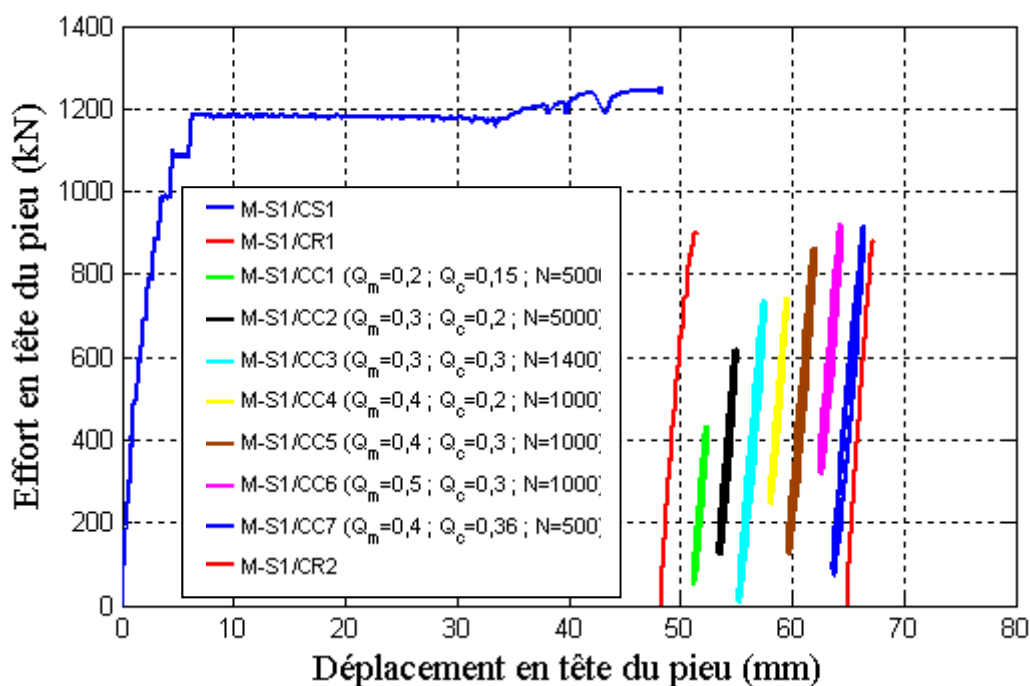
Figure III-43 : Historique de chargements en compression sur le pieu vissé S1
