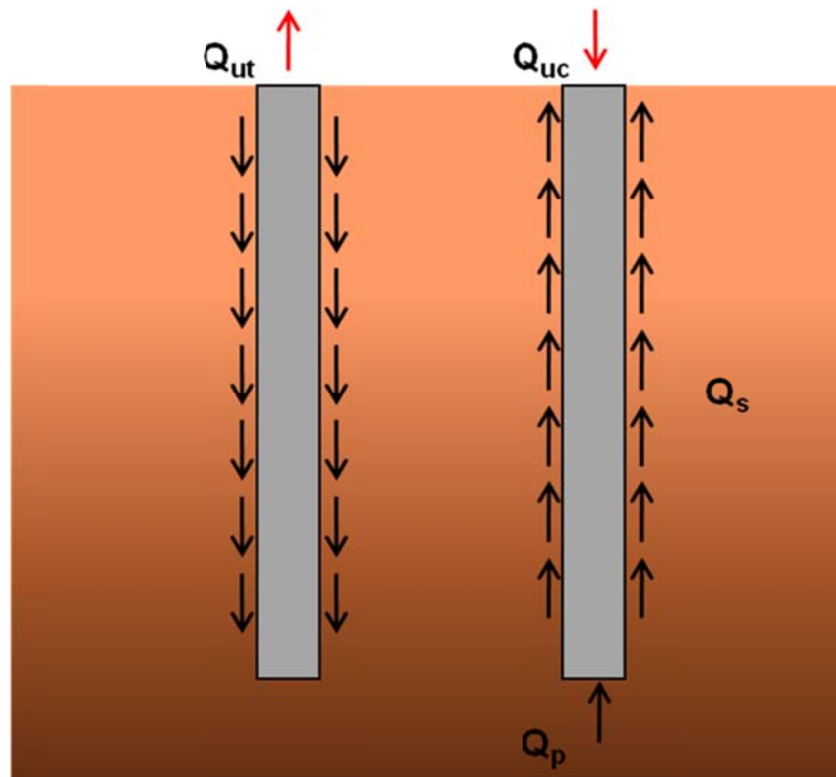
Figure I-1 : Schéma de la mobilisation du frottement latéral et la résistance de la pointe d'un pieu en compression et en traction
