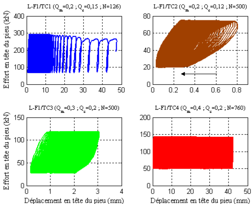
Figure IV-12 : Courbes effort-déplacement des essais cycliques sur le pieu F1
