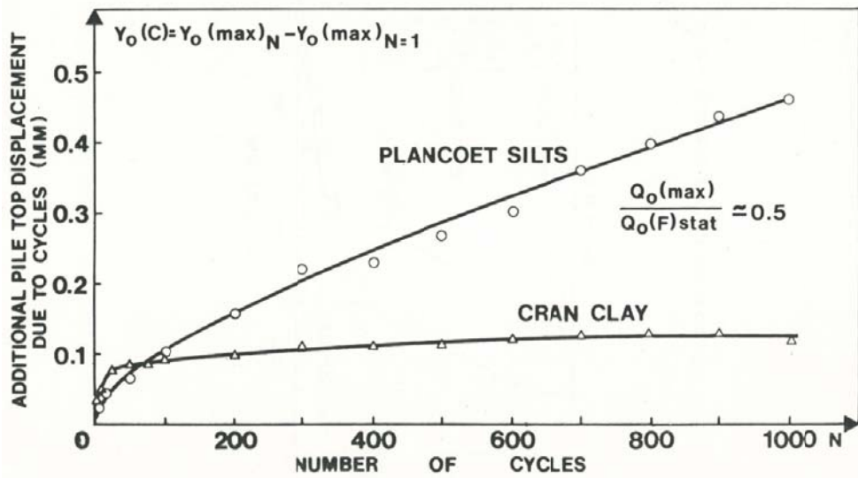
Figure I-24 : Courbes de fluage statique et cyclique du pieu de Plancoët
