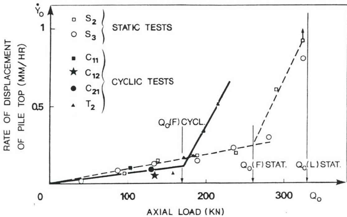
Figure I-23 : Courbes de fluage statique et cyclique du pieu de Plancoët
