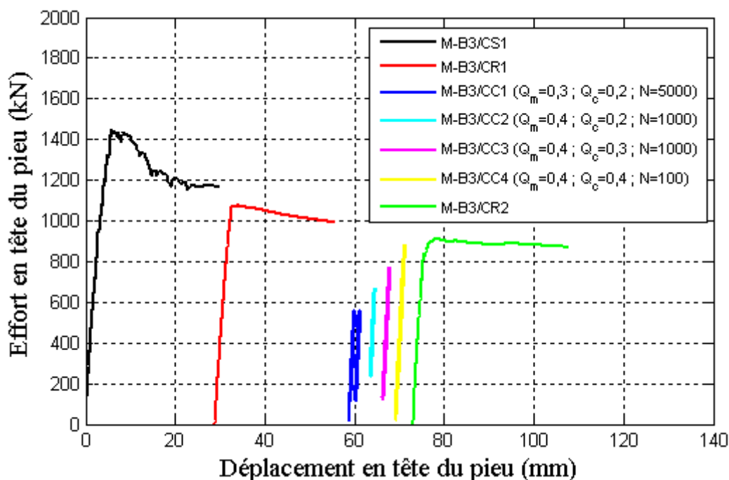
Figure III-48 : Historique de chargements en traction sur le pieu battu B3
