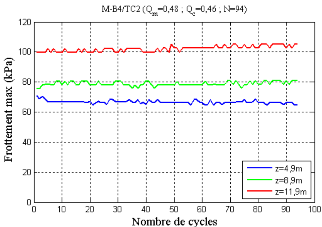
Figure III-51 : Frottement maximal développé sur les couches de l’argile des Flandres durant la séquence M-B4/TC2
