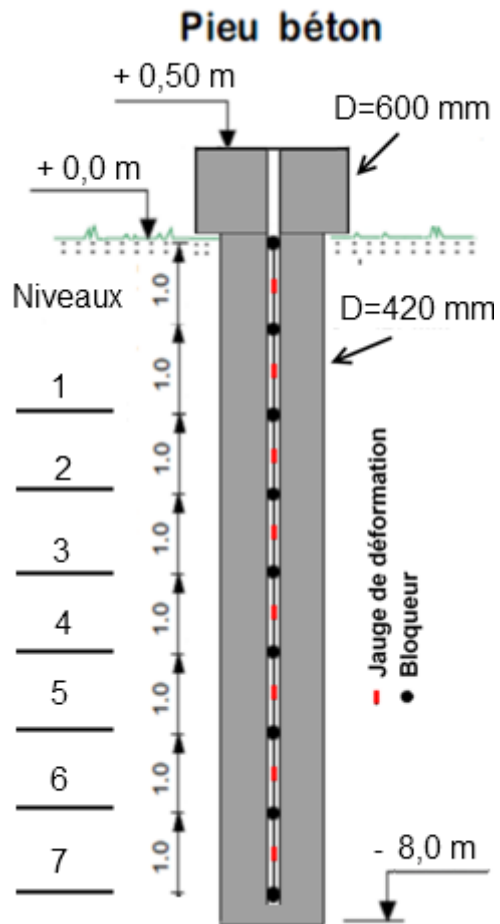
Figure II-25 : Schéma descriptif de l'instrumentation des pieux forés en compression de Loon-Plage
