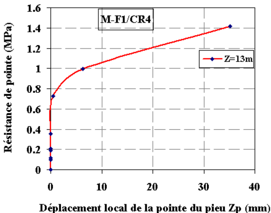
Figure III-5 : Évolution de la résistance de pointe lors de l’essai du chargement statique M-F1/CR4
