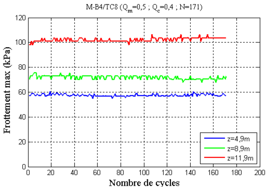
Figure III-52 : Frottement maximal développé sur les couches de l'argile des Flandres durant la séquence M-B4/TC8
