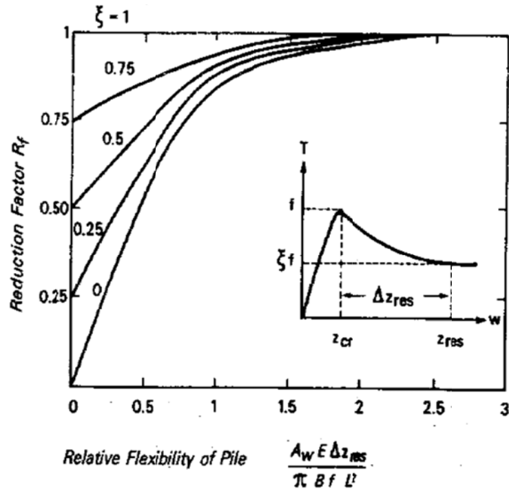
Figure I-3 : Coefficient de réduction R_f en fonction de la flexibilité du pieu ( 1/K ) et du degré de radoucissement \xi (Randolph, 1983).
