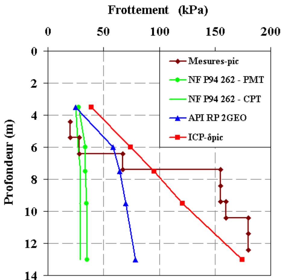
Figure III-22 : Comparaison des valeurs du frottement local mesurées et calculées sur le pieu battu B1.
