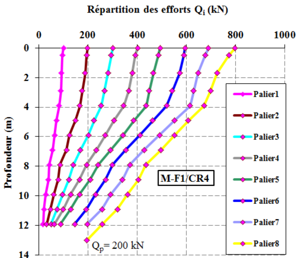
Figure III-3 : Répartition des efforts Q_i le long du pieu lors de l'essai du chargement statique M-F1/CR4
