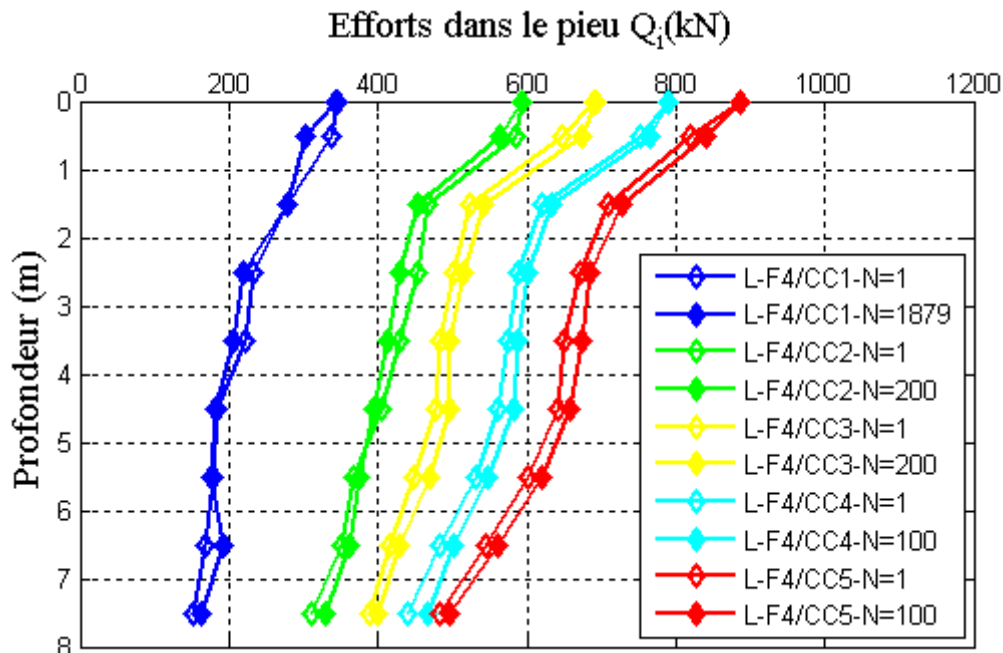
Figure IV-26 : Les efforts mesurés le long du pieu F4 au premier et au dernier cycle des cinq premiers essais cycliques.
