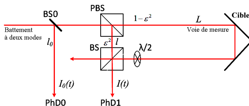
Fig. 3-1. Schéma de principe du télémètre ILIADE
