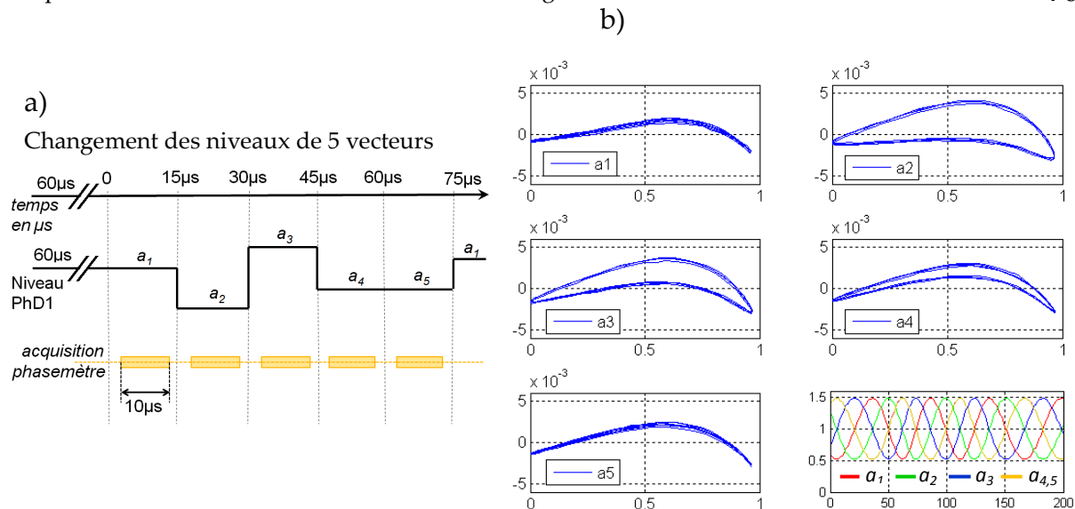
Fig. 5-18. Les segments créés par les 5 vecteurs, pendant un balayage de \lambda_{\text{opt}}
