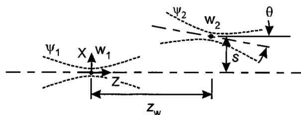
Fig. A4.1. Deux faisceau gaussiens tiltés et décalés
