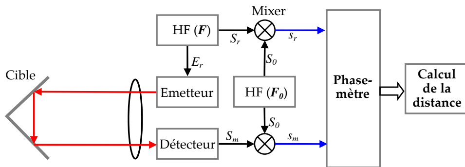
Fig. 2-2. Schéma de principe de la télémétrie par mesure de déphasage.
