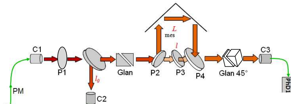
Fig. 5-13. Schéma optique avec un polariseur de Glan avant le polariseur P2 de l'interféromètre
