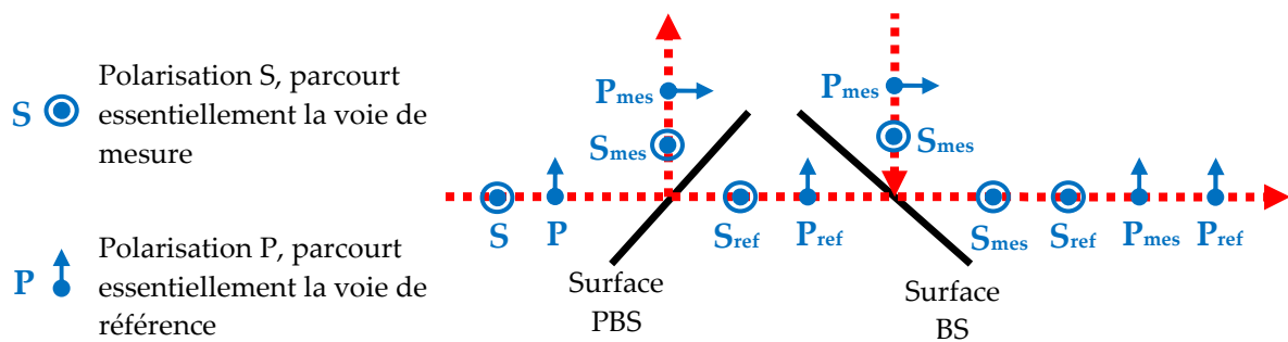
Fig. A8-1. La diaphonie de polarisation dans l'interféromètre
