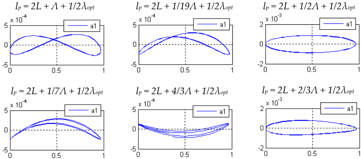
Fig. 5-4. Le segment zoomé avec un faisceau parasite, l_p \sim 2L Le faisceau parasite représente 2.5 \times 10^{-7} de la puissance totale
