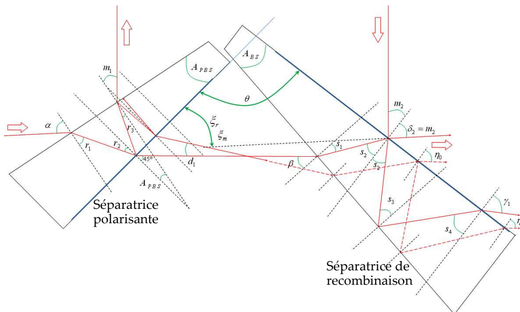
Fig. 5-9. Le trajet des faisceaux dans l'interféromètre utilisant des optiques prismatiques
