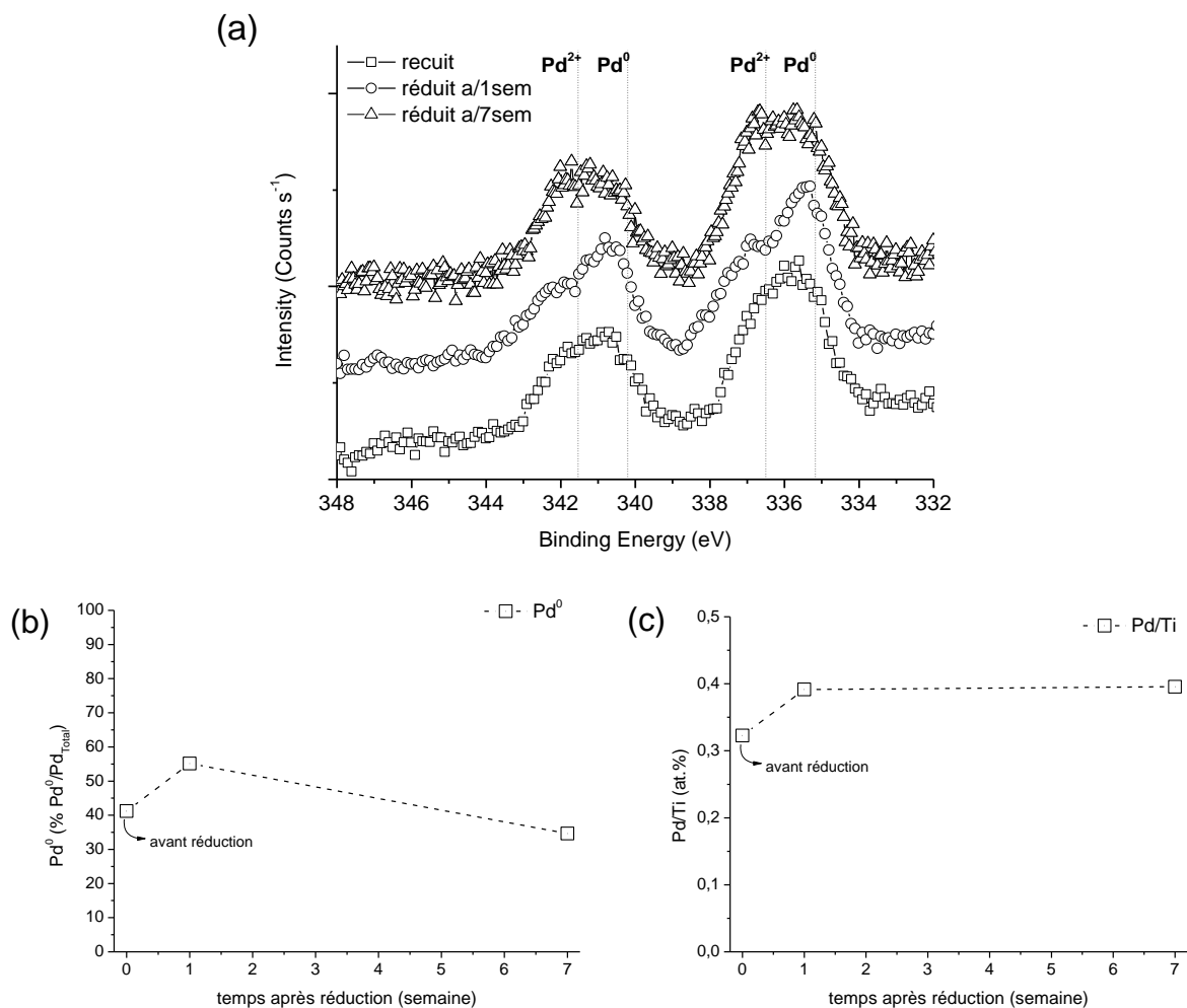
Figure 3-18 Effet du temps après réduction sur la distribution du Pd pour Pd-TiO 2 avec 0,39 at.% Pd/Ti réduction sous H 2 à 300°C, (a) spectres des massif du Pd 3d, (b) pourcentage de Pd 0 par rapport au Pd total et (c) pourcentage de Pd total par rapport au Ti.
