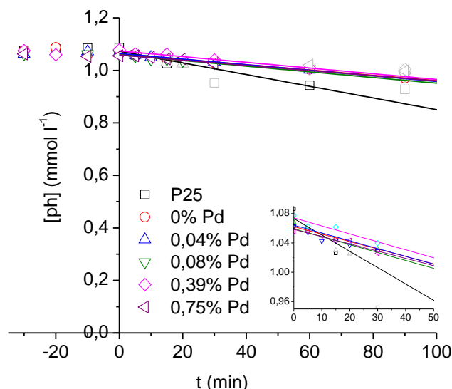
Figure 3-27 Evolution de la concentration de phénol en fonction du temps d'exposition aux UV (365nm) en présence des nanoparticules des Pd-TiO 2 recuites sous air à 400^\circ C . Les droites correspondent aux vitesses v_0 initiales de réaction.
