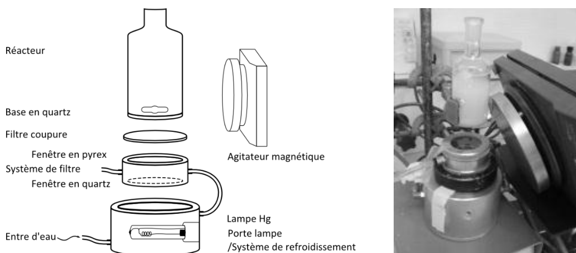
Figure 2-5 Schéma du réacteur IRCELYON
