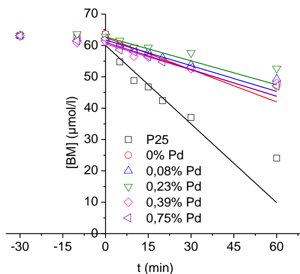
Figure 3-20 Evolution de la concentration de bleu de méthylène en fonction du temps d'exposition aux UV (365nm) et en présence des nanoparticules de Pd- TiO_2 recuits sous air à 400^\circ\text{C} . Les droites correspondent aux vitesses initiales v_0 de réaction.
