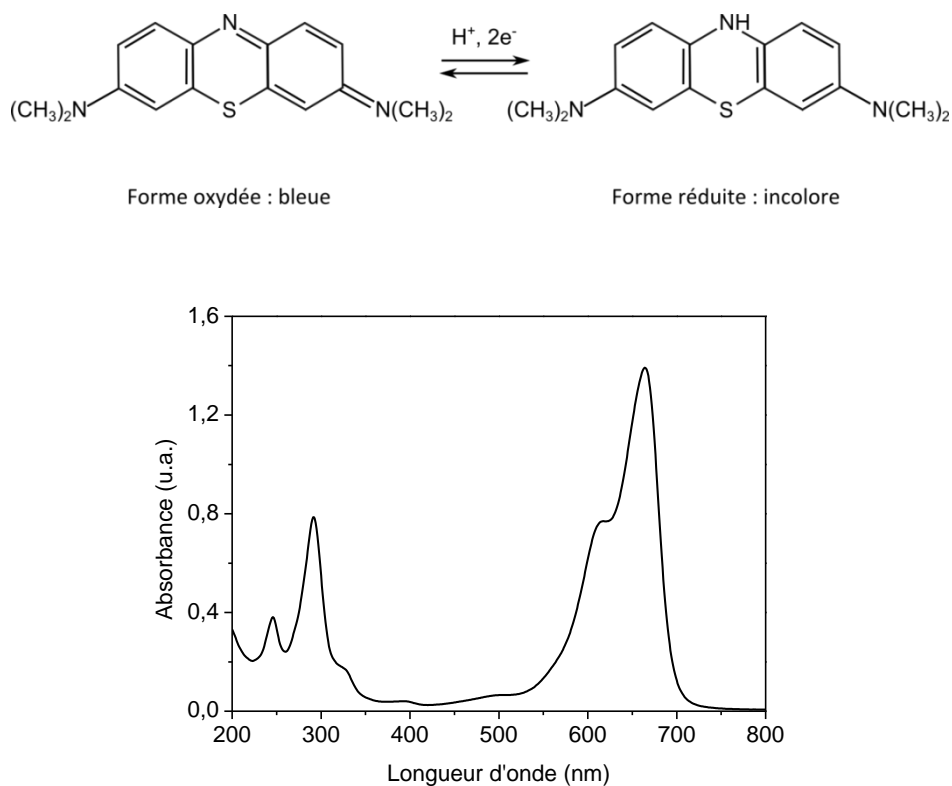
Figure 2-9 Structure chimique et spectre d'absorption UV-Vis du bleu de méthylène.
