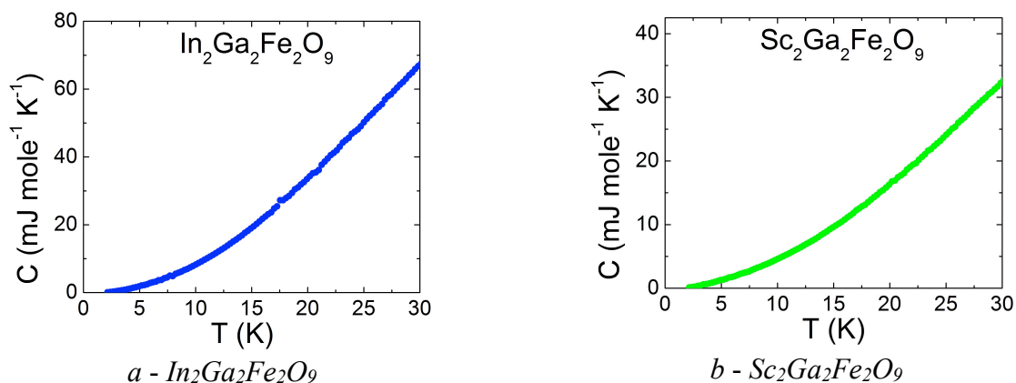
Figure VI.11. Chaleur spécifique en fonction de la température pour les composés M_2Ga_2Fe_2O_9 ( M=In, Sc ).
