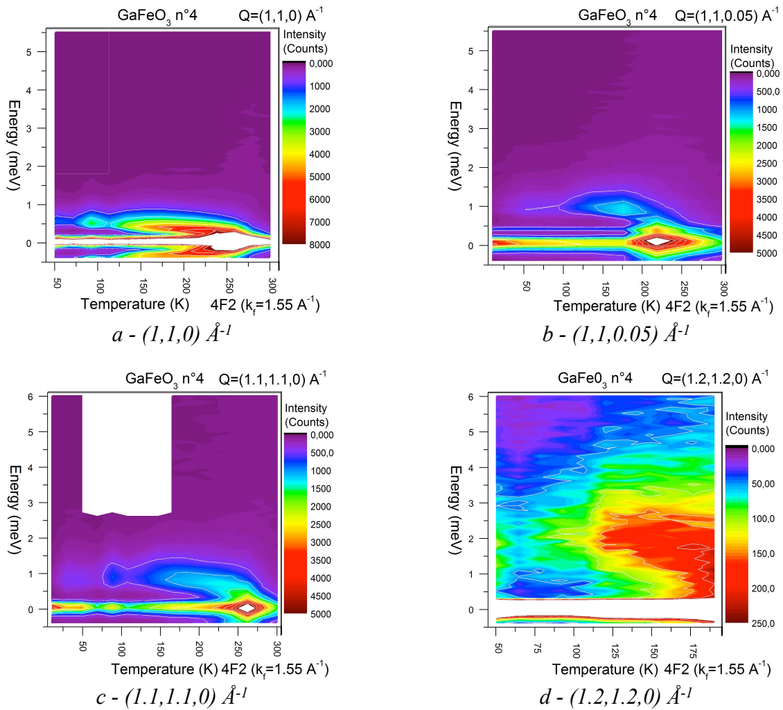
Figure IV.15. Evolution de l'énergie \omega_0 de l'onde de spin pour différents valeurs de Q le long de (q_h, q_h, 0) en fonction de la température pour l'échantillon GaFeO 3 n°4.
