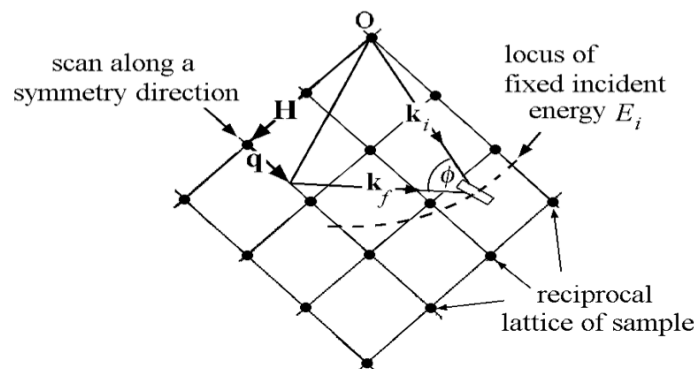
Figure IV.4. Techniques de mesure (mesure à vecteur d'onde constant, selon q , ou mesure à transfert d'énergie constant, selon E_i ) sur un spectromètre trois axes.
