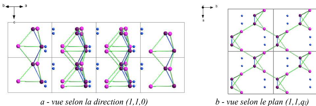
Figure IV.12. Vue des interactions magnétiques selon la direction (1, 1, 0) et selon le plan (1, 1, q_l) (les sites natifs de fer Fe1 et Fe2 sont représentés en couleur violet et rose, le site Ga2 en couleur bleu et les couplages magnétiques possibles entre les ions de Fe^{3+} sont symbolisés par des liaisons de couleur vert AFM et bleu FM).
