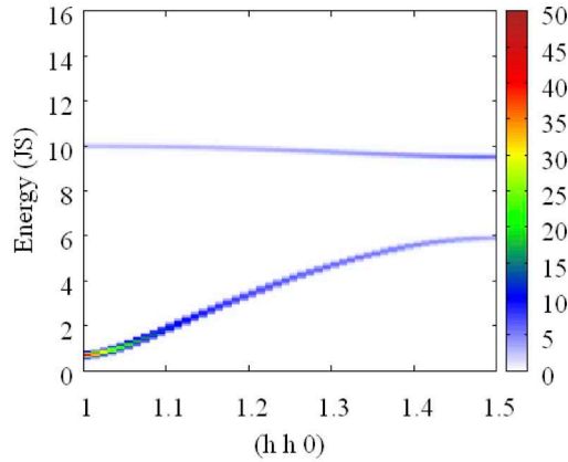
Figure IV.7. Carte en «fausses couleurs» de la dispersion des ondes de spin dans la direction (q_h, q_h, 0) pour les composés Ga_{2-x}Fe_xO_3 .
