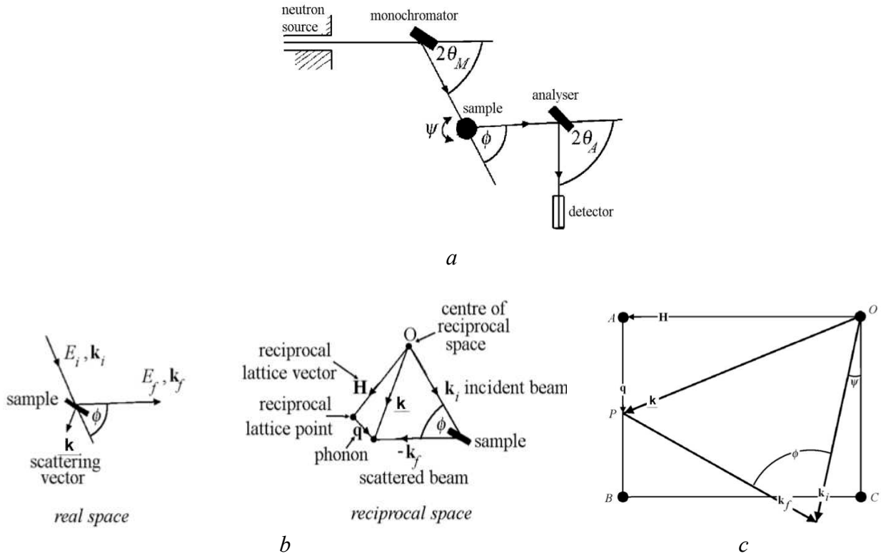
Figure IV.3. Schéma d'un spectromètre trois axes et principe de la mesure de diffusion inélastique. La réflexion de Bragg du monocristal monochromateur, la diffusion de l'échantillon et la réflexion de l'analyseur est montrée en (a). Le processus de diffusion inélastique des neutrons par un échantillon est illustré dans l'espace réel, ainsi que dans l'espace réciproque (b). Le diagramme vectoriel (c) montre le rapport entre les échanges de moment et d'énergie dans une expérience de diffusion inélastique.
