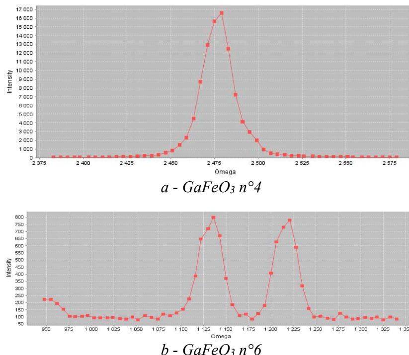
Figure III.5. «Scan» autour des réflexions (064) et (600) des cristaux de Ga_{2-x}Fe_xO_3 ( x=1.00 ). Mesure réalisée sur le spectromètre 5C2 ( \lambda=0.83 \text{ \AA} ), à T=300 \text{ K} , avec un temps/pas de 1.5 s.
