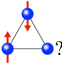
Figure V.2. Principe de la frustration magnétique, illustré pour le réseau triangulaire antiferromagnétique, complètement frustré : spins Ising (spin «up» ou «down») disposés aux sommets d'un triangle. Le dernier spin non représenté ne sera jamais satisfait.
