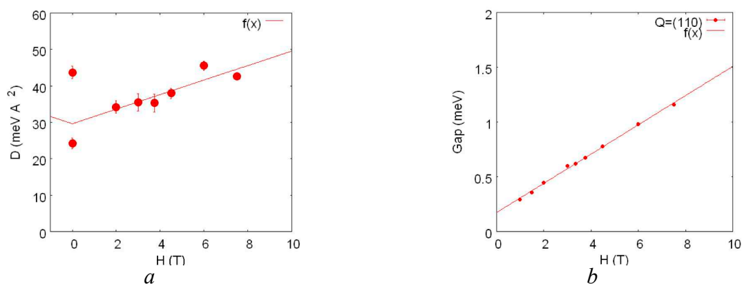
Figure IV.21. Evolution de la constante de raideur magnétique D et du gap de spin E_g en centre de zone en fonction du champ magnétique à 220 K pour l'échantillon \text{GaFeO}_3 n°4.
