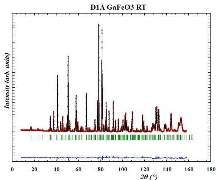
Figure II.4. Diagramme de diffraction des neutrons à température ambiante (spectromètre D1A, \lambda=1.91 \text{ \AA} ) et résultat de l'affinement pour l'échantillon \text{GaFeO}_3 n°1.
