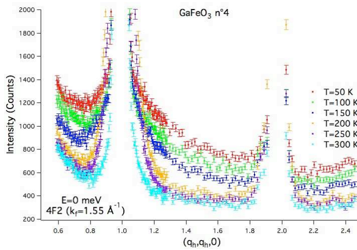
b - GaFeO 3 n°4 selon (q h , q h , 0)
