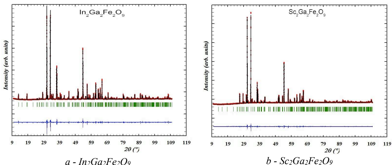
Figure VI.1. Diagrammes de diffraction (~15 heures) des rayons X ( \lambda=1.5406 \text{ \AA} ) et résultats de l'affinement d'échantillons M_2Ga_2Fe_2O_9 ( M=In, Sc ).
