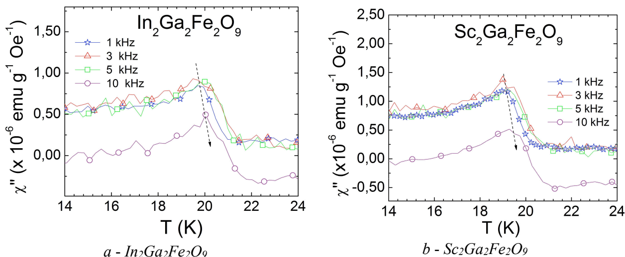
Figure VI.9. Dépendance en température de la composante imaginaire de la susceptibilité ac mesurée à différentes fréquences pour les composés M_2\text{Ga}_2\text{Fe}_2\text{O}_9 ( M=\text{In}, \text{Sc} ).
