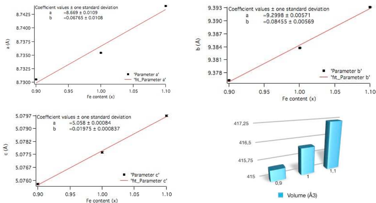
Figure III.4. Evolution de chaque paramètre de maille et du volume de la maille en fonction de la teneur en fer (valeur de x) (la droite d'ajustement est obtenue grâce à une régression linéaire de type y=ax+b ).
