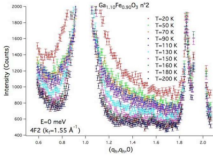
a - Ga 1.10 Fe 0.90 O 3 n°2 selon (q h , q h , 0)
