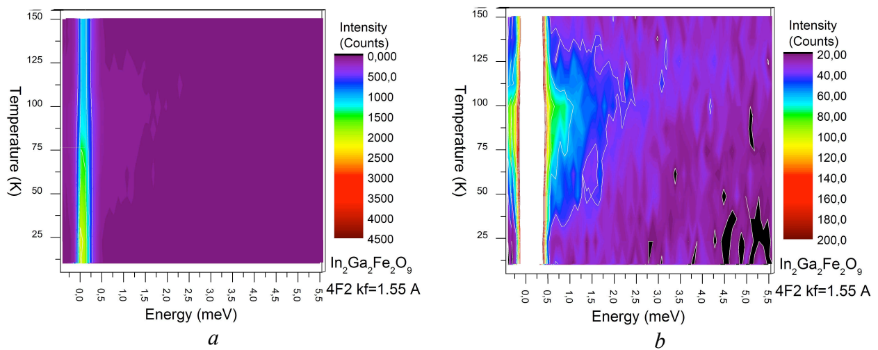
Figure VI.17. Cartes en fausses couleurs présentant l'évolution du diffus en fonction de l'énergie à Q=(1.4\ 0\ 0) , à des différentes échelles d'intensité (a et b), dans le composé In_2Ga_2Fe_2O_9 .
