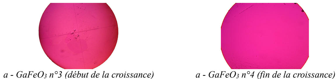
Figure III.3. Clichés de cristaux analysés au microscope optique (en lumière polarisée) avec un grossissement de \times 10 .
