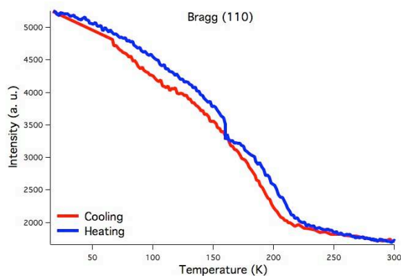
Figure III.13. Evolution de l'intensité du pic de Bragg (110) en fonction de la température. Mesure de l'échantillon \text{GaFeO}_3 n°4 réalisée sur le spectromètre D9 ( \lambda=0.83 \text{ \AA} ).
