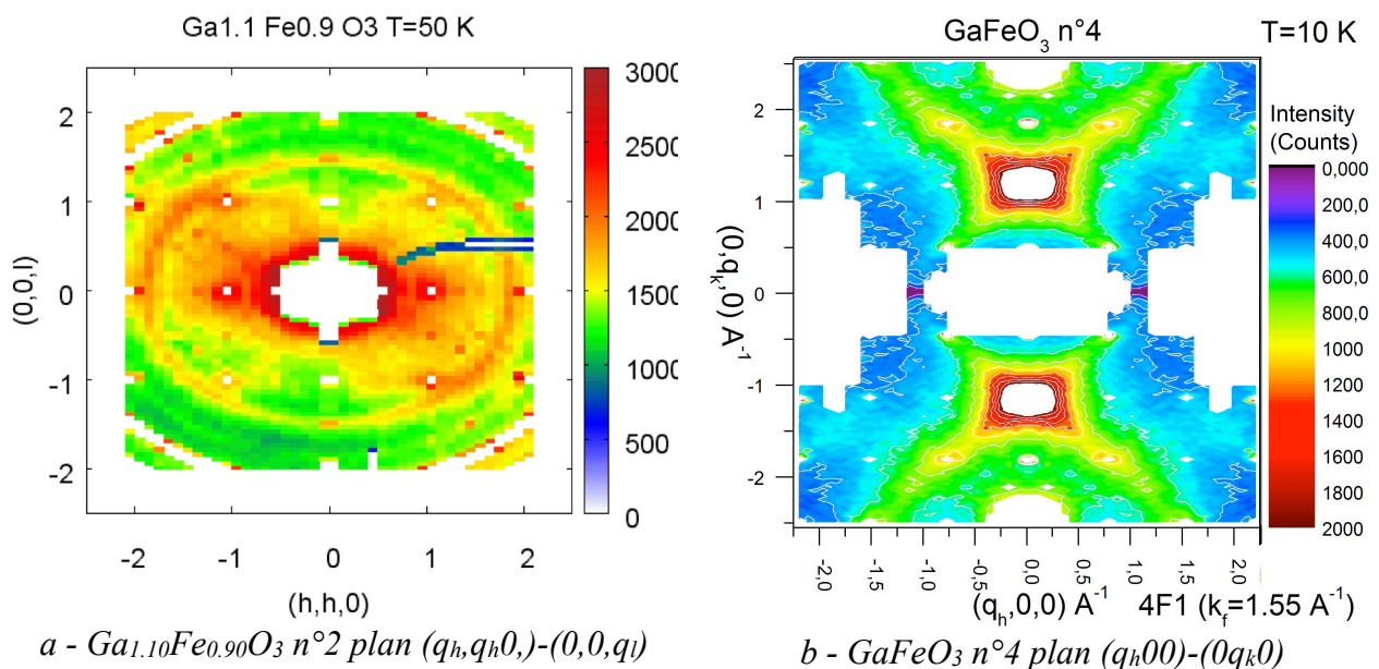
Figure IV.11. Carte de la diffusion diffuse élastique à basse température dans les plans de diffusion (q_h, q_h 0) - (0, 0, q_l) et (q_h 0 0) - (0 q_k 0) sur deux échantillons représentatifs de Ga_{2-x}Fe_xO_3 ( x=0.90 et 1.00 ).
