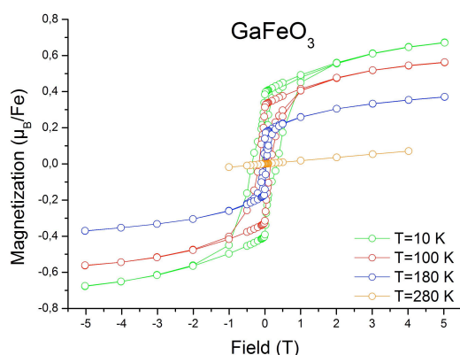
Figure II.12. Variation de l'aimantation du composé GaFeO_3 n^{\circ}1 en fonction du champ magnétique appliqué ( T=10 K, 100 K, 180 K et 280 K).
