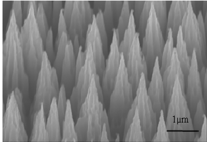
Figure IV-1. Image MEB du Black Silicon typique fabriqué par DRIE cryogénique.
