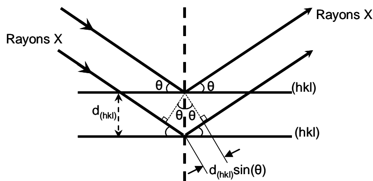
Figure III-21. Schéma du principe de la diffraction des rayons X par les plans réticulaires.
