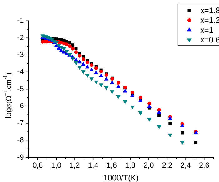
Figure IV-2-5 : Variation de la conductivité \sigma avec la température, pour les 4 compositions.
