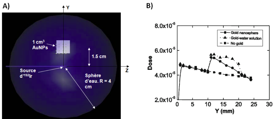
Figure 1.24: A : Schéma de la géométrie simulée. B : Comparaison de profils de dose calculés selon l'axe Y considérant un faisceau parallèle de photons arrivant sur le volume cible pour les trois conditions [Zhan 09]
