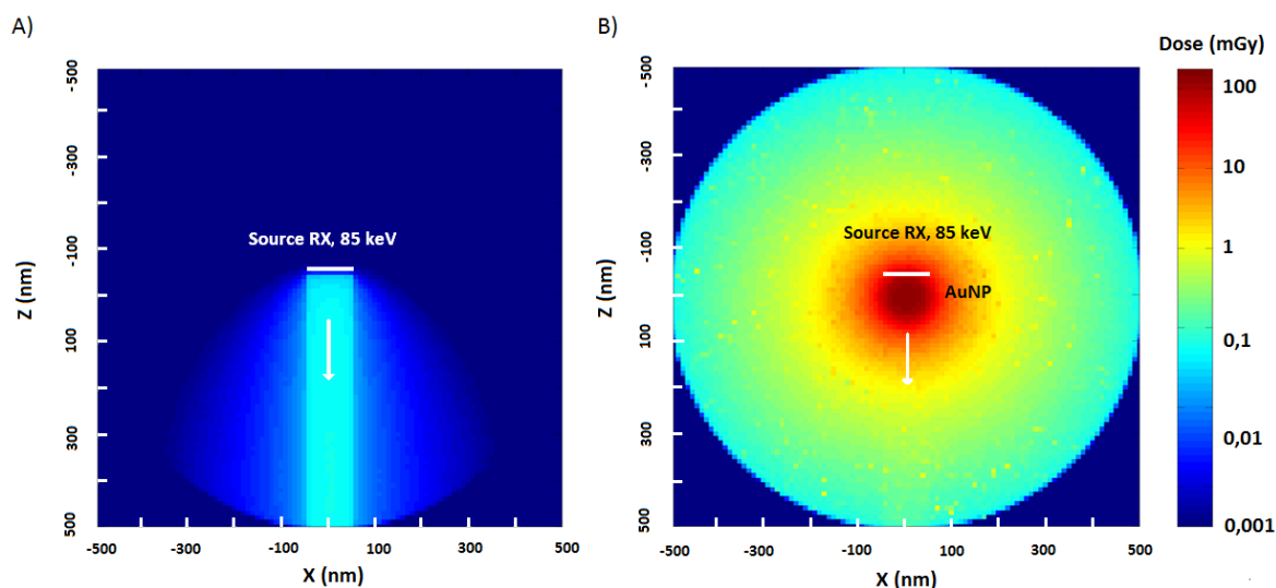
Figure 4.9: Profil de dose dans le plan XZ dans le cas d'une NP de 50 nm de rayon centrale remplie d'eau (A) et remplie d'or (B).
