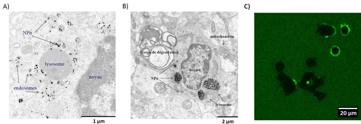
Figure 3.17: A et B : images réalisées par microscopie électronique sur des tissus tumoraux d'un rat euthanasié 24h (A) et 6 jours (B) après injection de AuNP de 15 nm [Boby 10]. C : image réalisée par microscopie à fluorescence sur cellules F98 après 5 h d'incubation avec des GdNP (Florence Taupin).
