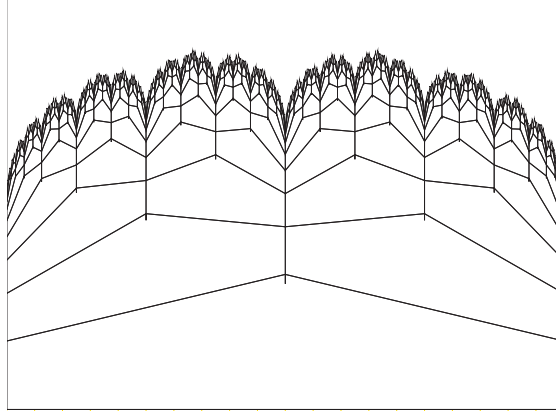
FIGURE 1.7 – La courbe délimitant \widehat{\Omega}
