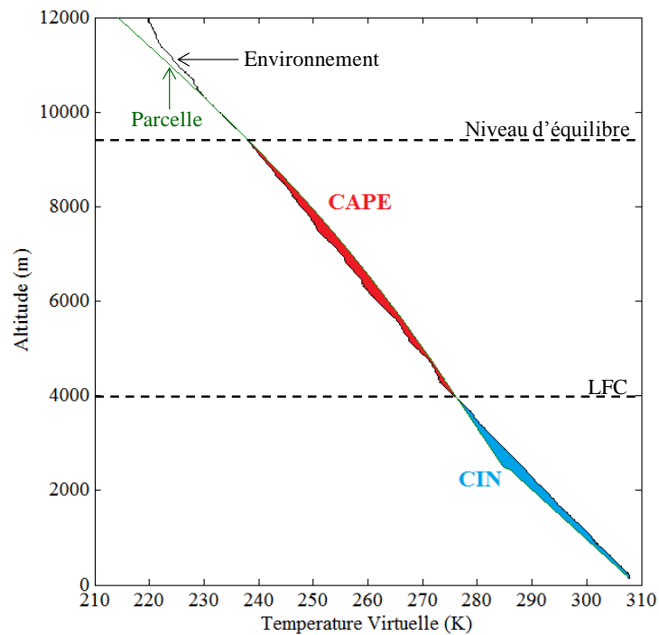
Figure 1.1. Température virtuelle de l'environnement (noir) et d'une parcelle d'air soulevée adiabatiquement depuis le sol (vert). Les aires colorées correspondent à la CIN (bleu) et à la CAPE (rouge). Les lignes pointillées indiquent le niveau d'équilibre et le niveau de convection libre (LFC).
