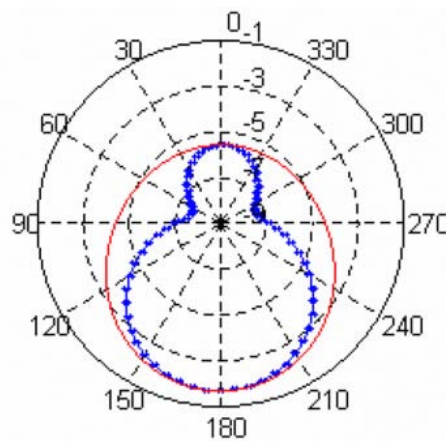
FIGURE 1.31 – Diagrammes de rayonnement de l'antenne dipôle réalisée sur silicium
