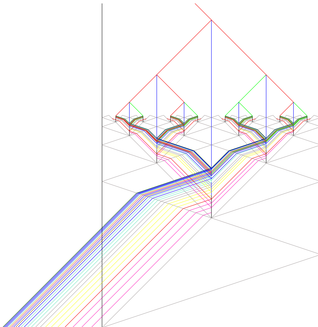
FIGURE 8.8 – Diagramme global de résolution générique de la formule \exists x_1 \forall x_2 \forall x_3 (x_1 \wedge \neg x_2) \vee x_3 .
