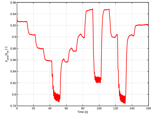
(d) Pressure Ratio across the hole @2000 rpm
