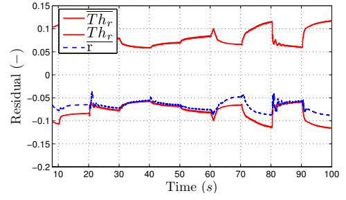
(d) High Load, \Delta\eta_t = 0 , \Delta p_{exh} = 200\text{mbar}
