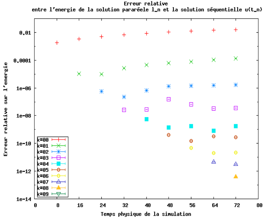
FIGURE 3.19 – Evolution de l’erreur relative, entre les énergies pararéelles et fines de référence, avec un modèle réduit (absence des groupes de précurseurs) et un scénario statique, \tau_F = 10^{-1} , \tau_G = 4 et \hat{n} = 10 .
