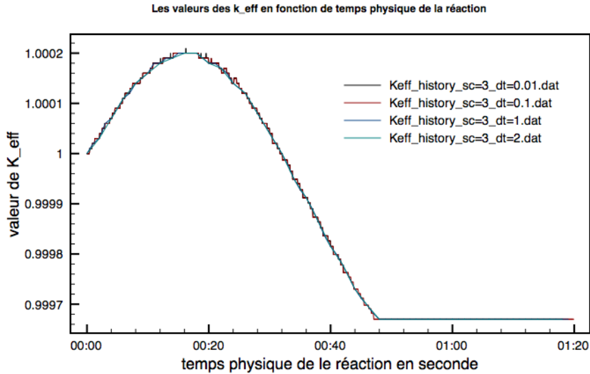
FIGURE 3.8 – Variation des k_{eff} en fonction du temps.
