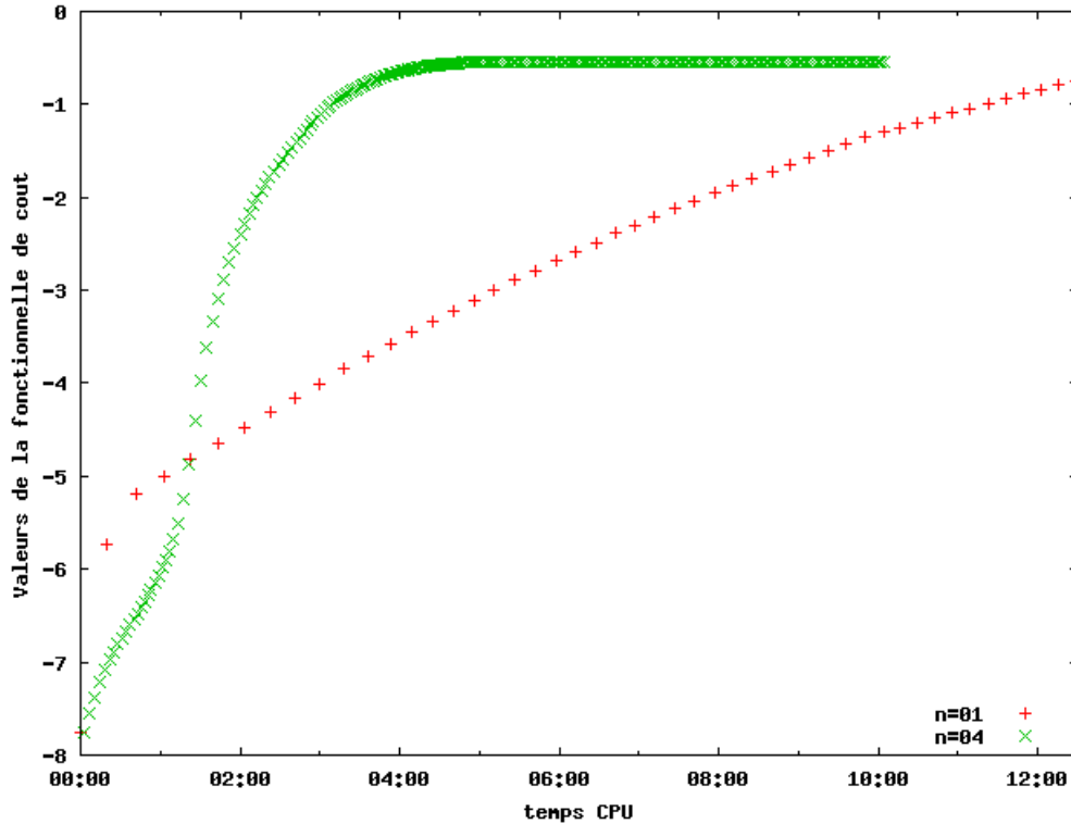
FIGURE 4.3 – Accélération de la résolution en temps Wallclock, interprétation par maximisation de la fonctionnelle de coût -J avec 4 processeurs en parallèle (courbe verte) et en séquentiel (courbe rouge) 1 processeur.
