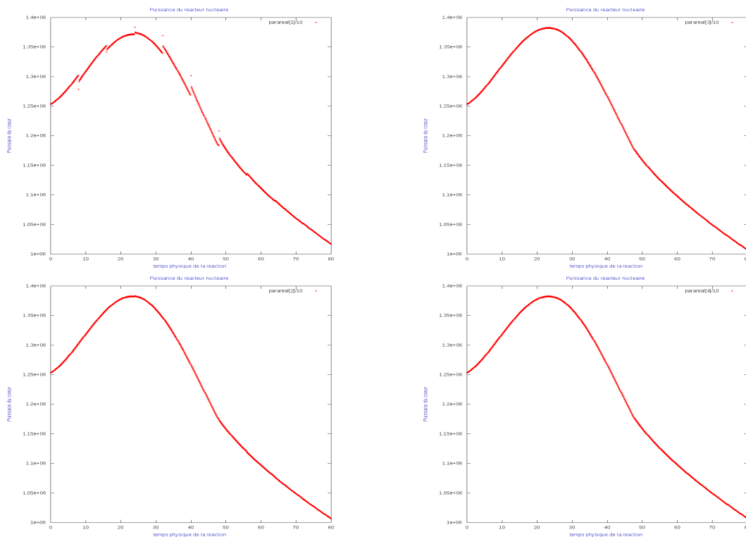
FIGURE 3.14 – Comportement du pararéel (itérations 1-2-3-4 ) sur la norme du flux neutronique du cœur avec le modèle complet pour le scénario dynamique, \tau_F = 10^{-1} , \tau_G = 4 et \hat{n} = 10 .
