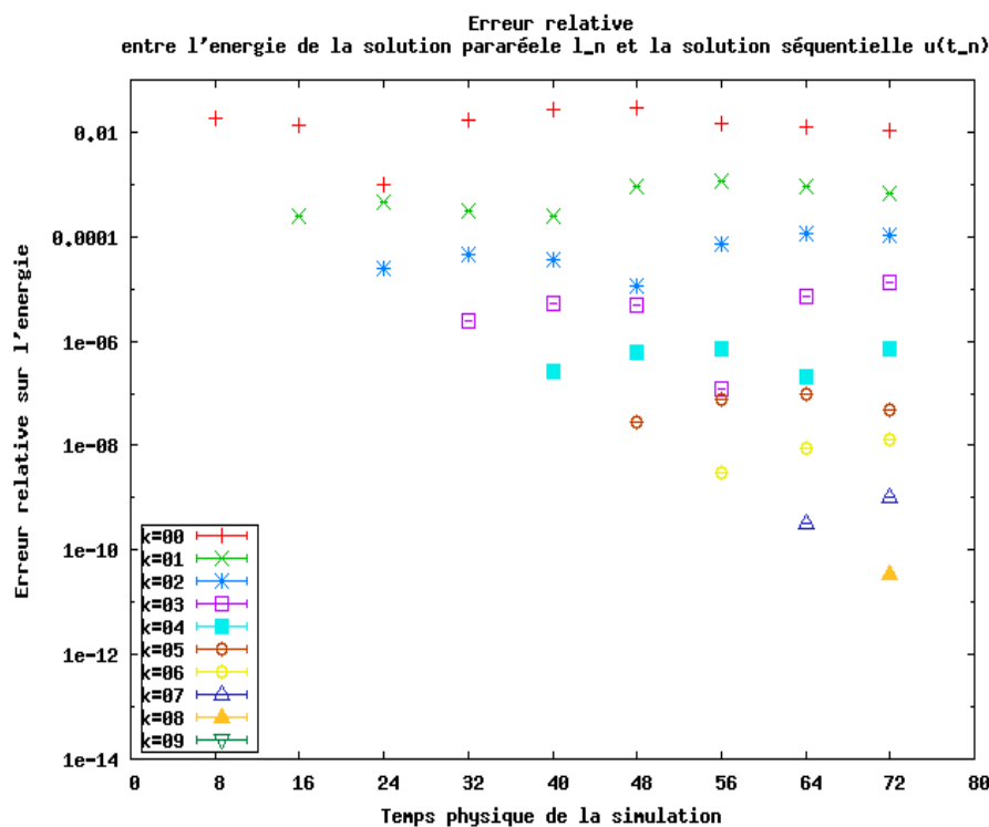
FIGURE 3.16 – Evolution de l’erreur relative entre les énergies pararéelles et fines de référence. Evolution avec un modèle complet (6 groupes de précurseurs) avec un scénario dynamique, \tau_F = 10^{-1} , \tau_G = 4 et \hat{n} = 10 .
