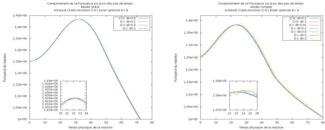
FIGURE 3.12 – Valeurs de la norme du flux moyen de réacteur avec le scénario dynamique .
