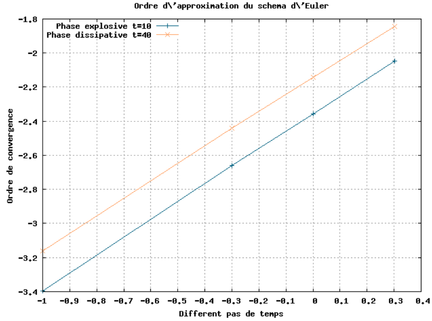
FIGURE 3.11 – Ordre de convergence du schéma d'Euler implicite, pour le scénario dynamique du modèle complet (six groupes de précurseurs) : échelle logarithmique décimale sur les axes “ x ” et “ y ”.
