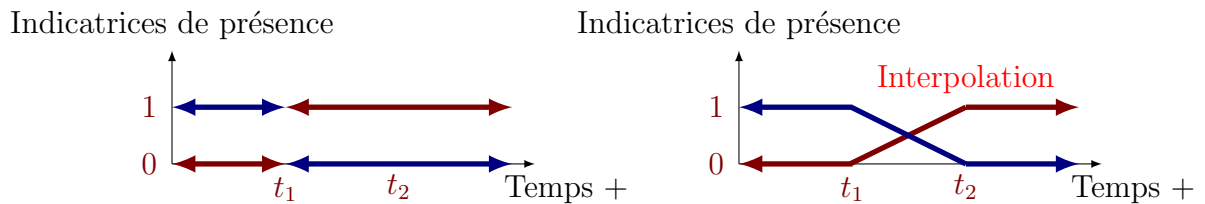
FIGURE 3.5 – Indicatrices des taux de présence des grappes (courbe rouge) et du combustible (courbe bleu) dans un tétraèdre.
