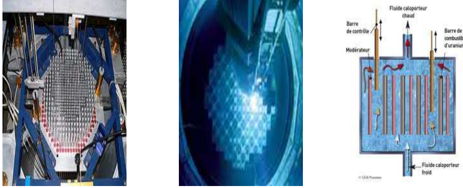
FIGURE 3.3 – Le cœur nucléaire à l’assemblage (à gauche), à l’état de fonctionner (au milieu) et sous forme de schéma (à droite).
