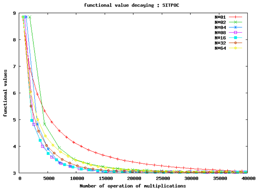
FIGURE 2.4 – Gain en nombre d’opérations de multiplication par itération de l’algorithme SITPOC.
