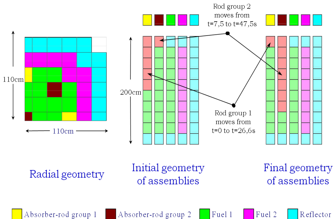
FIGURE 3.7 – Géométrie du cœur et positionnement initial des grappes d'absorption.
