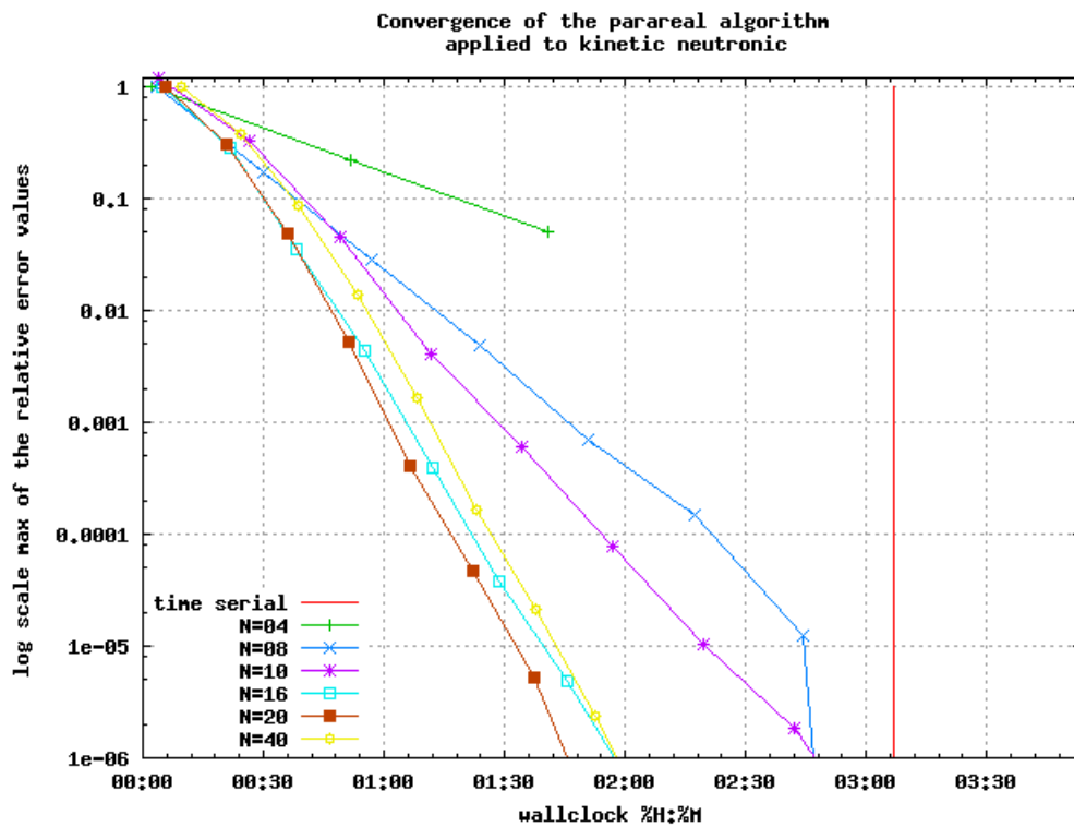
FIGURE 3.21 – Temps réel de simulation CPU (Wallclock sous format h :m) pour les erreurs commises par l’algorithme pararéel en temps appliqué selon le nombre de processeurs (ou sous-intervalles) utilisés à un modèle dans la physique est dégradée pour le solveur grossier. \tau_F = 10^{-1} , \tau_G = 2 et \hat{n} \in \{1, 4, 8, 10, 16, 20, 40\} .
