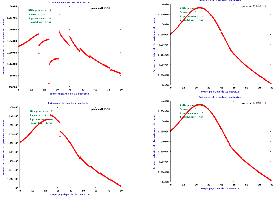
FIGURE 3.17 – Comportement de la norme de flux neutronique (itérations 1-2-3-4) avec un modèle complet et un scénario statique pour le calcul grossier et un scénario dynamique pour le calcul fin, \tau_F = 10^{-1} , \tau_G = 2 et \hat{n} = 10 .
