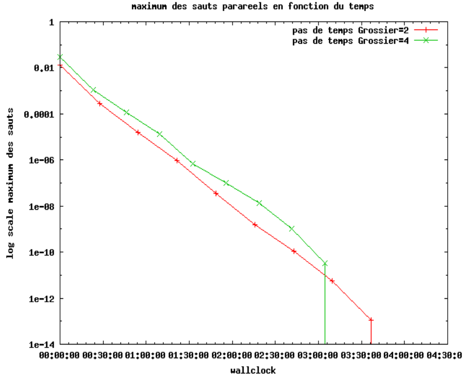
FIGURE 3.20 – Temps réel de simulation CPU (Wallclock sous format h :m :s), modèle complet avec un scénario dynamique selon une variation du pas de temps grossier \tau_G , \tau_F = 10^{-1} , \tau_G = \{2(\text{rouge}), 4(\text{verte})\} .
