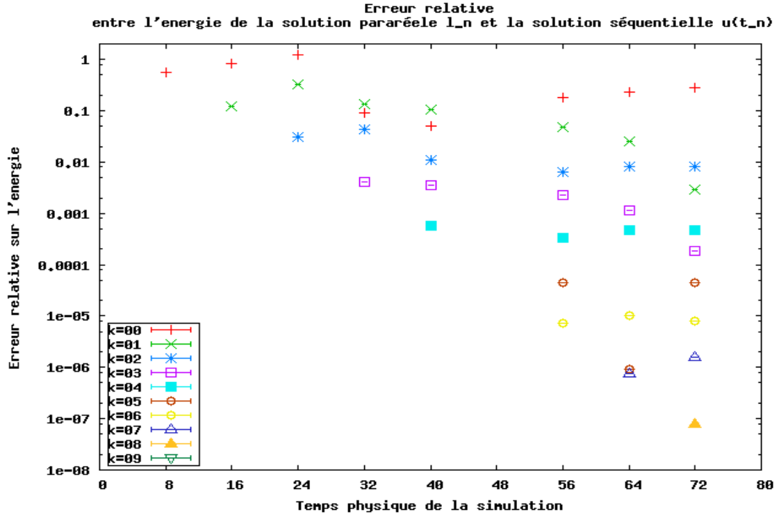
FIGURE 3.18 – Convergence du pararéal appliqué à la neutronique (itérations 00-09), un modèle complet avec un scénario dynamique pour le calcul fin et utilisant un scénario statique pour le calcul grossier. \tau_F = 10^{-1} , \tau_G = 2 et \hat{n} = 10 .
