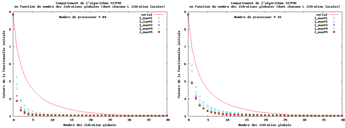
FIGURE 2.7 – L'algorithme SITPOC en 4 subdivisions à gauche et 16 subdivisions à droite : variation du nombre des itérations locales l_{\max} .
