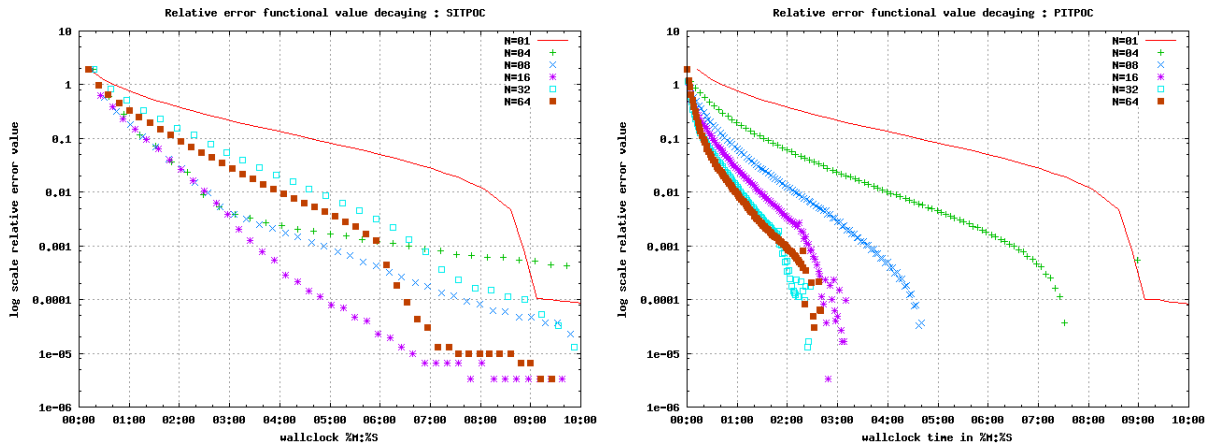
FIGURE 2.6 – Gain en temps réel de simulation machine : SITPOC (gauche) et PITPOC(droite).
