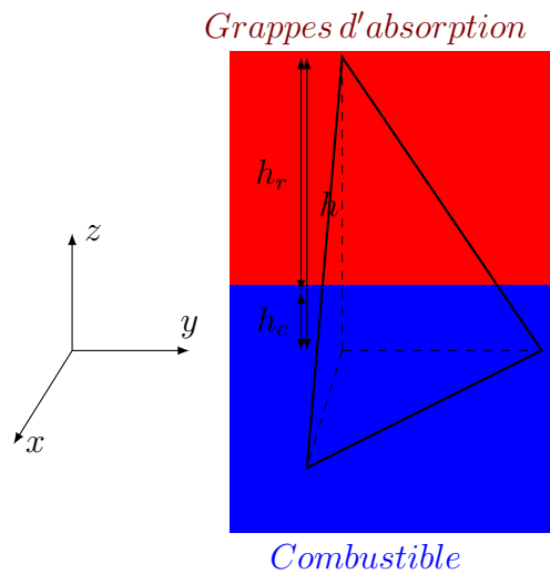
FIGURE 3.6 – Coefficients de la fonction indicatrice 3d pour les grappes absorbantes.
