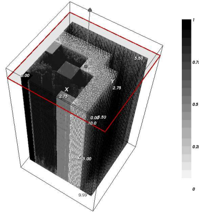
FIGURE 3.4 – Maillage en trois dimensions d'un quart du cœur nucléaire.
