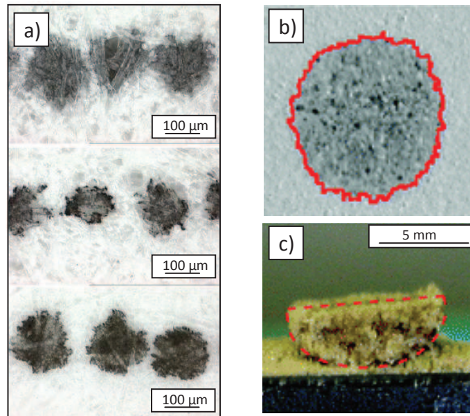
Figure I.1 : a) Photographies (vue de dessus) de l'empreinte laissée après imbibition d'encre dans des papiers de différentes textures [53], b) et c) photographies du volume de sable imbibé par un agent neurotoxique respectivement vue de dessus, et après extraction du volume imbibé [50].
