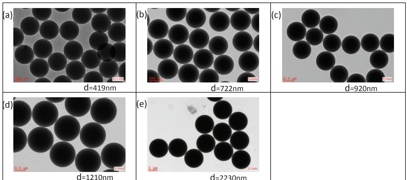
Figure II.2 : Images en microscopie électronique à transmission des microbilles de PS : (a) d=419 nm, (b) d=722 nm, (c) d=920 nm, (d) d=1210 nm et (e) d=2230 nm
