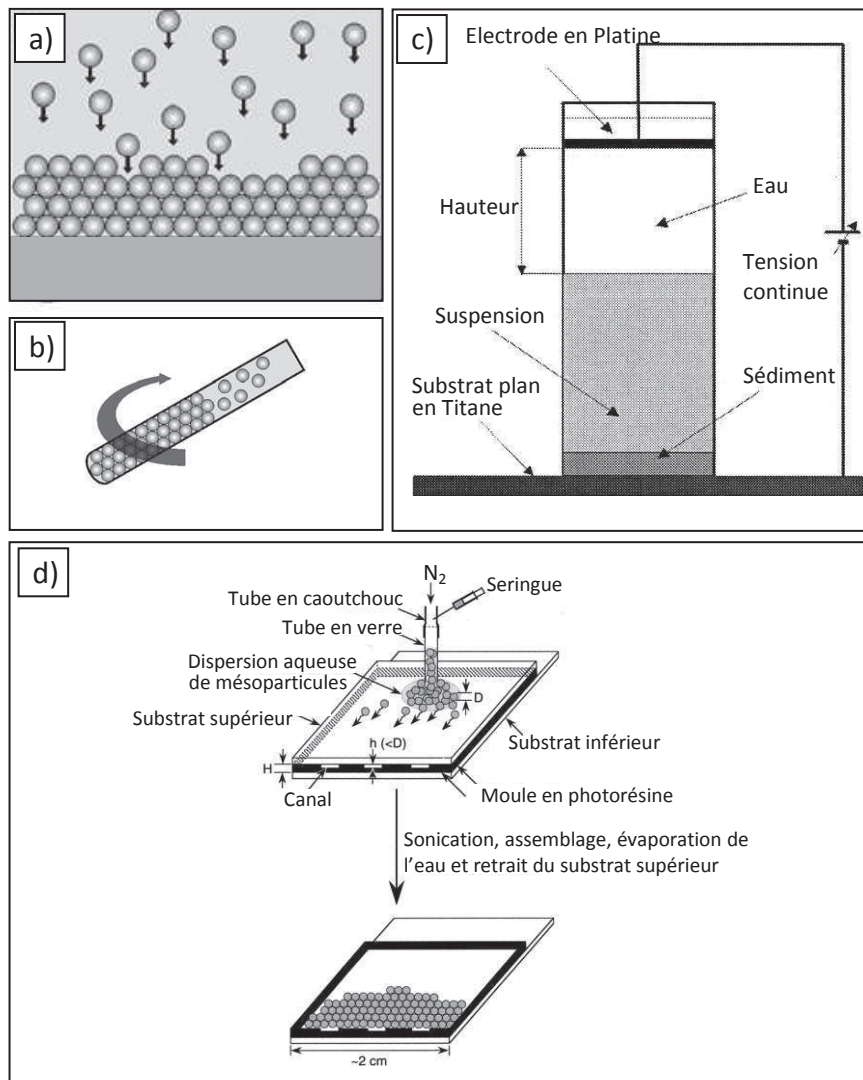
Figure 1.7 : Représentation schématique de différentes méthodes d'assemblage tridimensionnel de microbilles : (a) par sédimentation [101], (b) par centrifugation [101], (c) dispositif expérimental de la cellule électrophorétique, (d) dispositif expérimental de l'auto-assemblage sous confinement physique [94, 102]
