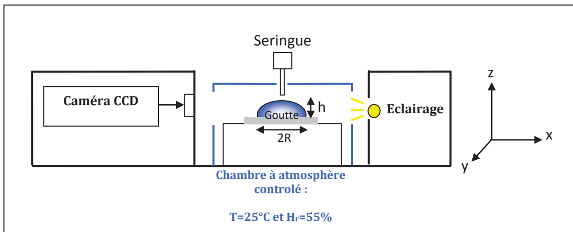
Figure III.4 : Schéma du dispositif expérimental (goniomètre Krüss)
