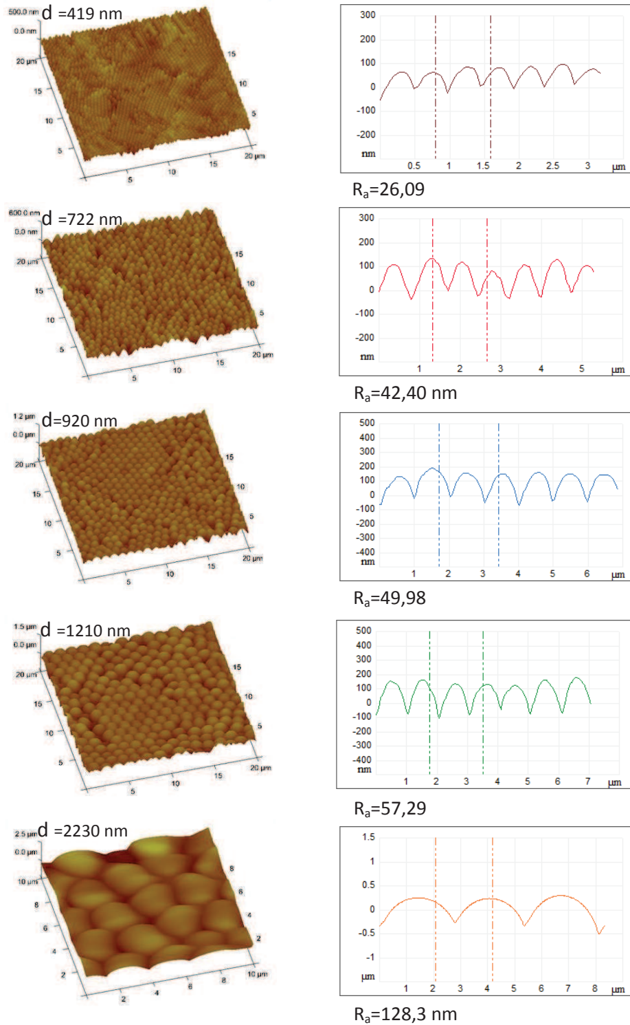
Figure 11.11 : Image de la surface réalisée par Microscopie à Force Atomique en mode intermittent, pour les différentes tailles de microbilles, avec une représentation du profil de hauteur correspond ainsi qu'une mesure de la rugosité
