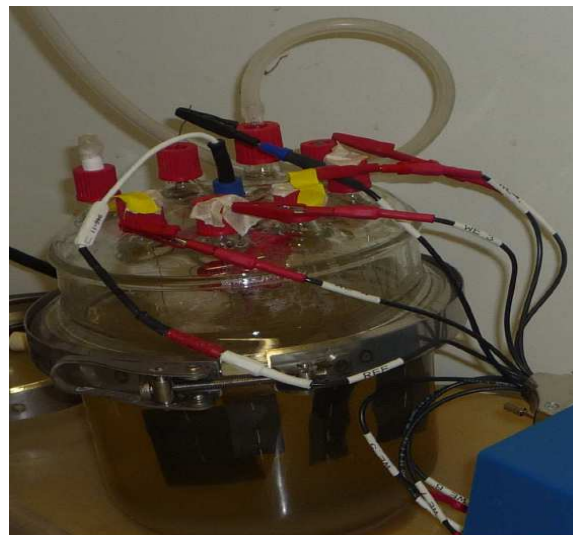
Figure 28: Photos du montage expérimental. A) montage simple à 3 électrodes, B) montage avec dispositif N-STAT.
