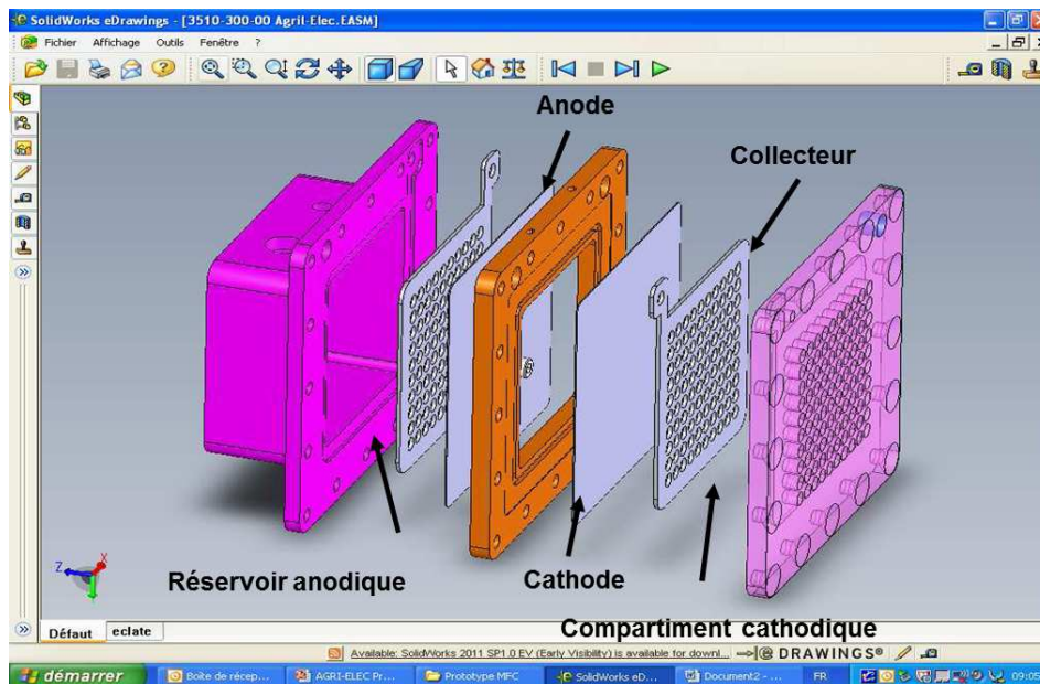
Figure 33: Première version du prototype de PAC. (Schéma PaxiTech).
