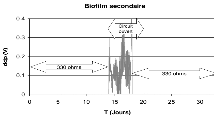
Figure 108: Evolution de la différence de potentiel en inoculant la pile avec le biofilm de la Figure 106 ; la pile est connectée à une résistance de 330 ohms.
