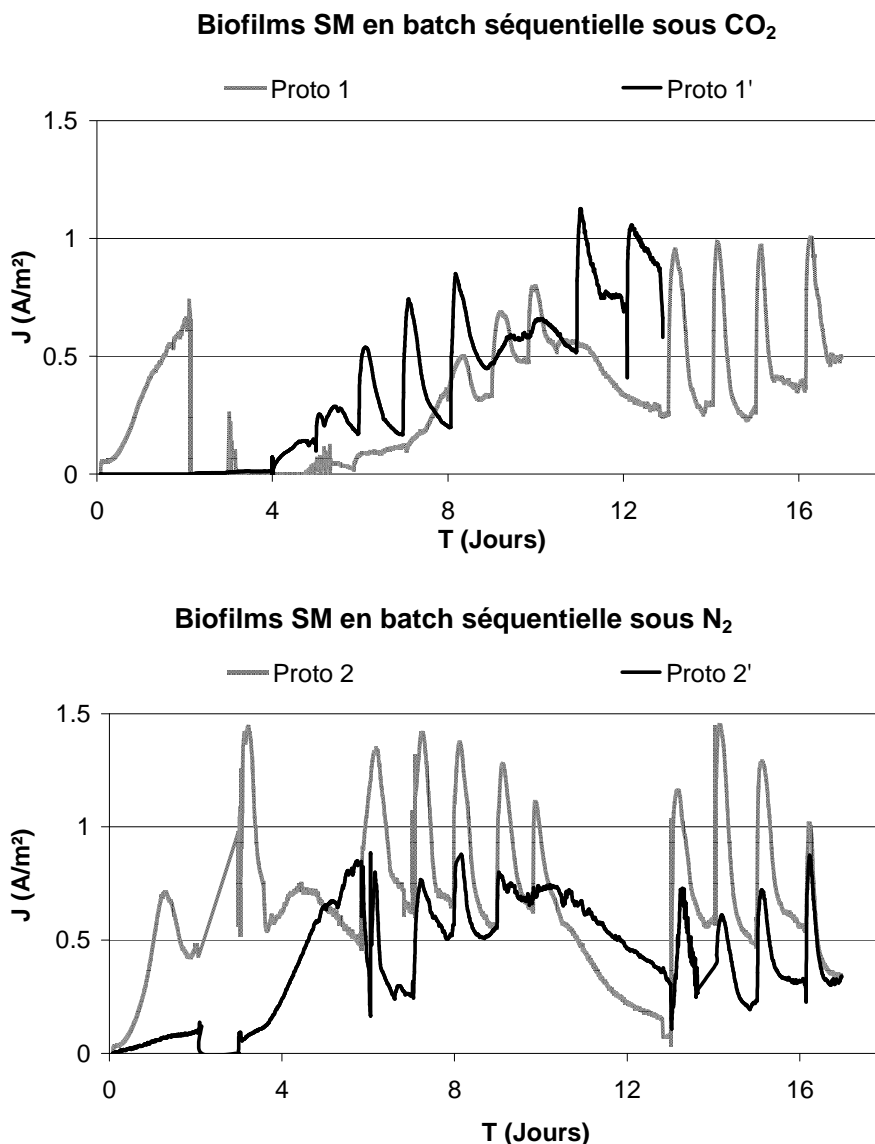
Figure 103: Duplicats de biofilms formés dans les prototypes en alimentation batch séquentielle (TRH 48h) avec l'effluent sortie méthaniseur (SM). Les conditions anaérobies sont maintenues avec les barbotages des gaz N_2 ou CO_2 .
