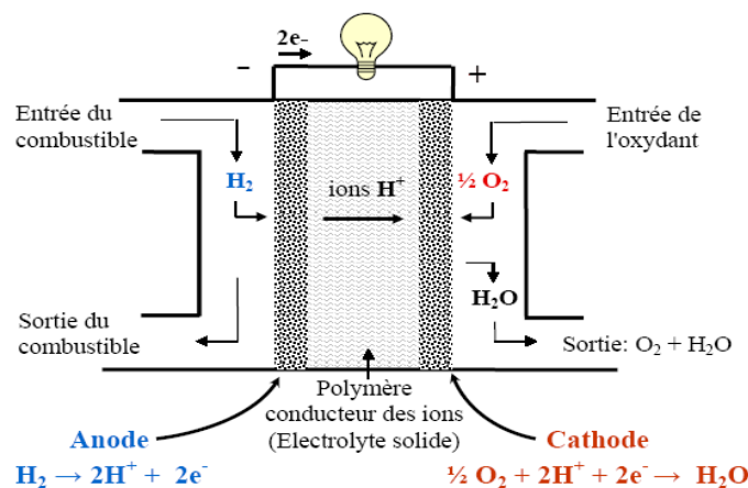
Figure 2: Principe de fonctionnement d'une pile à membrane échangeuse de protons.
