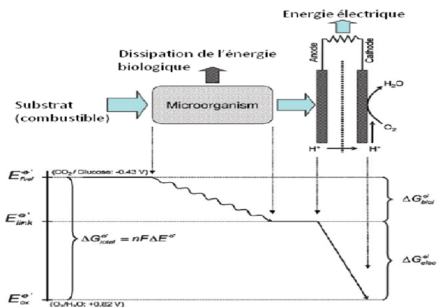
Figure 22: Schéma du flux énergétique dans les PACMs. Adapté de (Schroder 2007)
