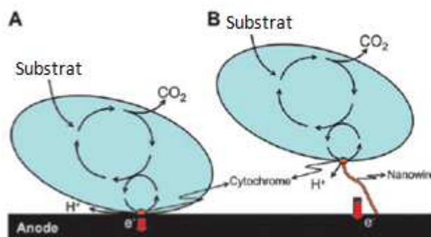
Figure 8: Deux mécanismes de transfert possibles: A= via les cytochromes membranaires; B= via les pilis ou «nanowires» conducteurs (Schroder 2007).
