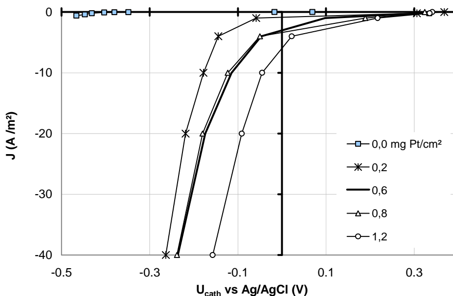
Figure 96: Performances des cathodes à air en fonction de la charge en Pt dans des piles à hydrogène. Expérience réalisée par PaxiTech.
