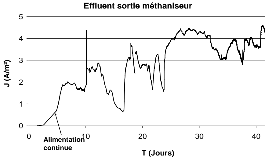
Figure 66: Biofilm EA primaire formé avec l'effluent sortie méthaniseur brut à -0,3V et sous barbotage de N_2 continu. Le réacteur est laissé en mode batch pendant 5 jours puis mis en alimentation continue avec un TRH de 24 h.
