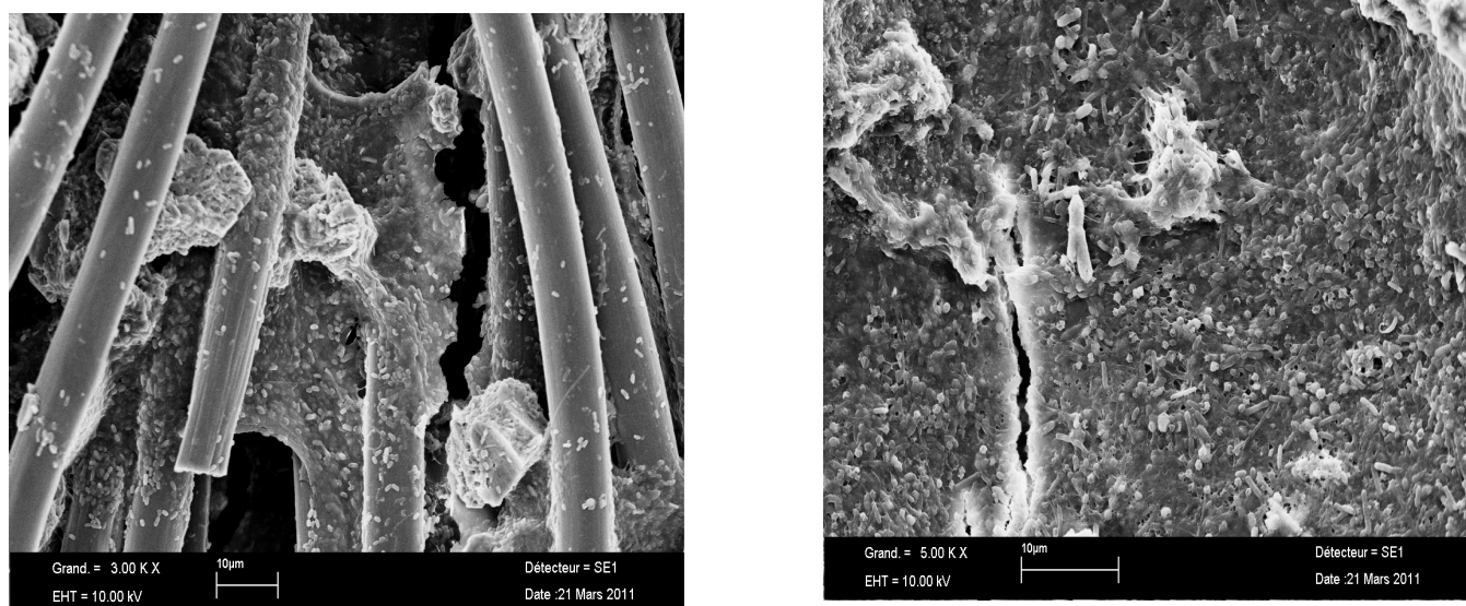
Figure 94: Photos MEB de l'anode colonisée à la fin de la caractérisation à 2 grossissements différents. Photos réalisées par le LGC.
