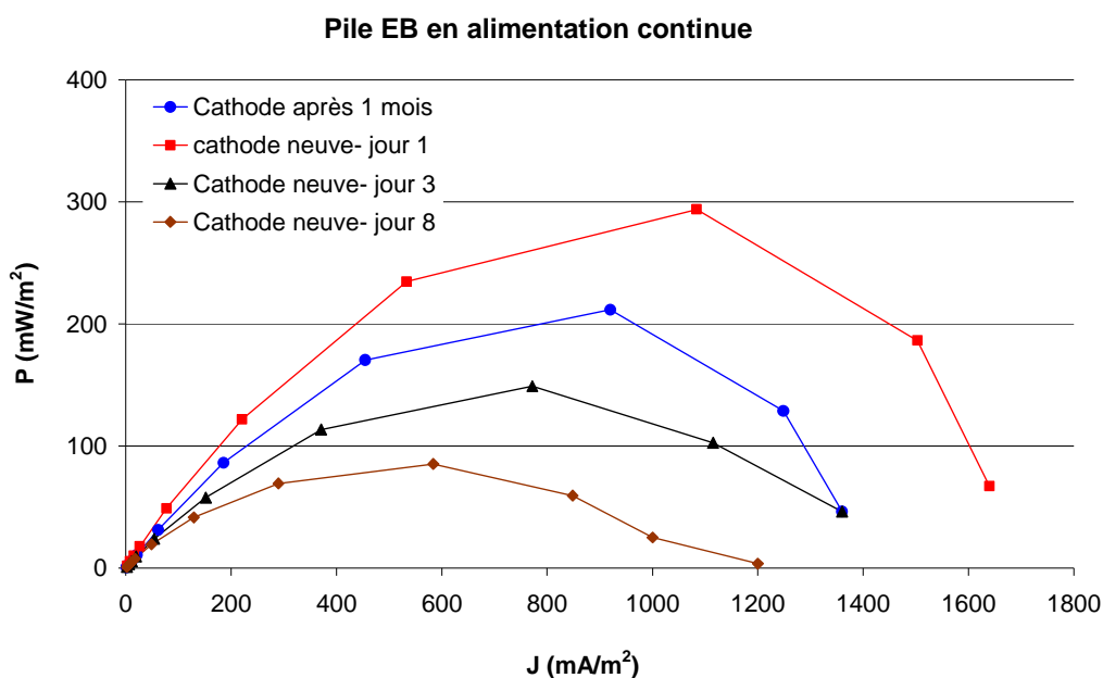
Figure 99: Caractérisation de la pile à la fin de la formation du biofilm sous polarisation en alimentation continue avec l'effluent entrée biologique brut avec 2 cathodes différentes. Courbe bleu: cathode ayant servi pendant un mois à la formation du biofilm EA (1,5 mg/cm 2 en Pt et 60% PTFE, sans membrane). Courbe rouge: cathode standard neuve au jour 1; courbe noire: cathode standard au jour 3; courbe marron: cathode standard au jour 8.
