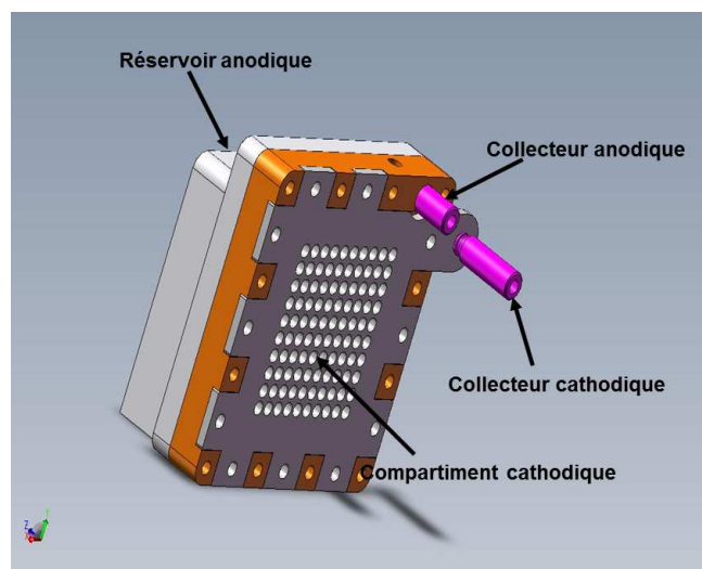
Figure 101: Vue de la deuxième version du prototype de pile complète.
