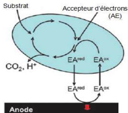
Figure 6: Transfert d'électrons à l'anode via les médiateurs artificiels (Schroder 2007)
