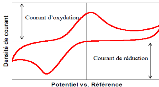
Figure 31: Allure d'un voltammogramme
