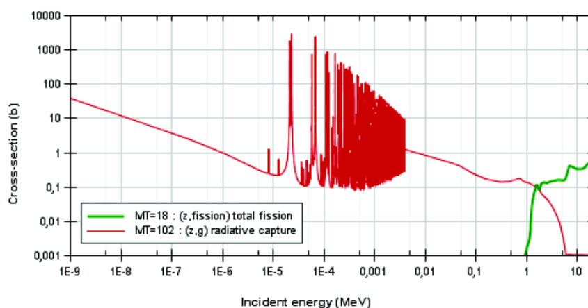
(b) ^{232}\text{Th}
