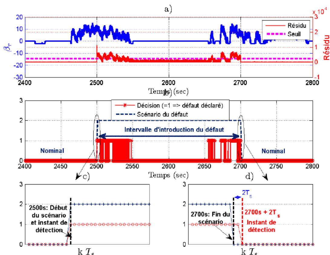
FIG. 7.8 – Résultat de détection du défaut de type FG = 5 affectant le signal \beta_{2,m_2} délivré par le capteur 1 mesurant l'angle de la troisième pale, \beta_2 dans l'intervalle [2500s, 2700s] . Le subplot b) donne le signal binaire qui est de valeur 1 lors de la présence du défaut. Les deux ellipses font référence au zoom effectué pour montrer la détection au début et à la fin de l'intervalle de présence du défaut, présentée resp. sur les deux subplot c) et d).
