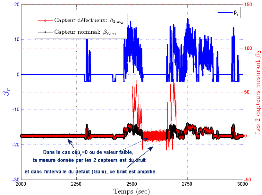
FIG. 7.7 – Les 2 signaux \beta_{2,m_1} et \beta_{2,m_2} en configuration nominale et défectueuse ( FG = 5 ) resp. Pour \beta_{r_2} = 0 la seule mesure vient du bruit.
