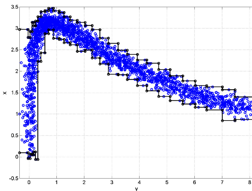
FIG. 4.4 – Enveloppe bornée obtenue en commutant les rôles remplis par x et y . Notons que la qualité de l'enveloppe bornée est considérablement améliorée du fait que sa surface A_\theta(\mathcal{S}) est réduite de 19.9 à 6.75 environ.
