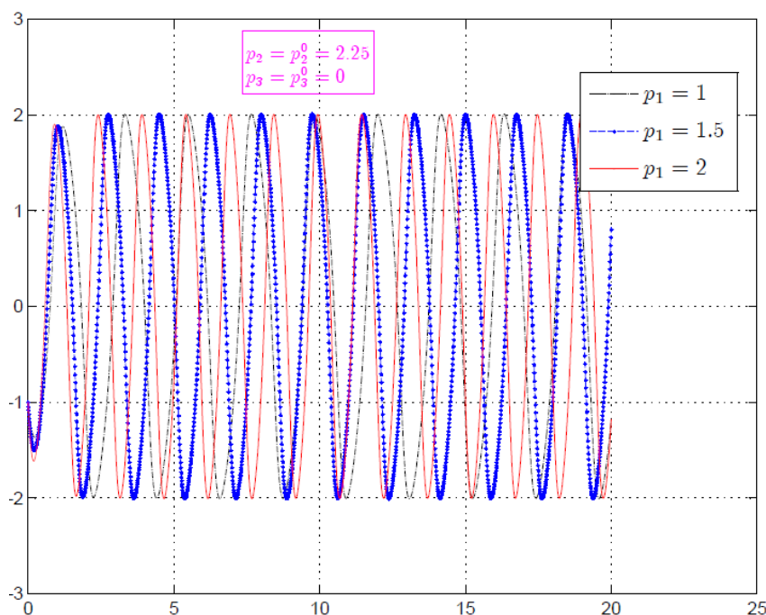
FIG. 2.10 – Sortie de l'oscillateur dans le cas des variations de p_1 , (p_2, p_3) = (2.25, 0) .
