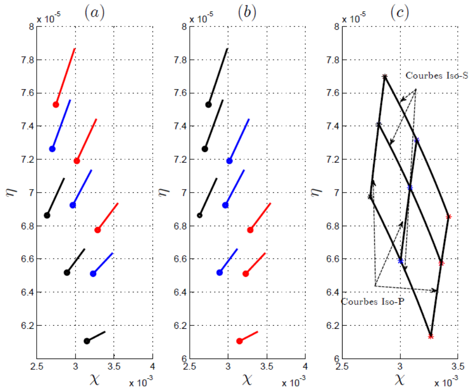
FIG. 4.29 – Allures des 9 signatures \mathcal{S}^{(6)}(z^{(1)} | X = 0.5) pour z^{(1)} \in \mathbb{Z}_d^{(1)} obtenues en utilisant N = 6 . Notons que chaque signature contient M = N_O - N = 2 points. Subplot (a) représente toutes les signatures ayant la même valeur de S par la même couleur alors que le subplot (b) utilise la même couleur pour tracer les signatures qui ont la même valeur de P . Subplot (c) montre le système de coordonnées curvilignes qui peut être utilisé pour obtenir d'un seul coup une formule d'estimation de S et de P connaissant X
