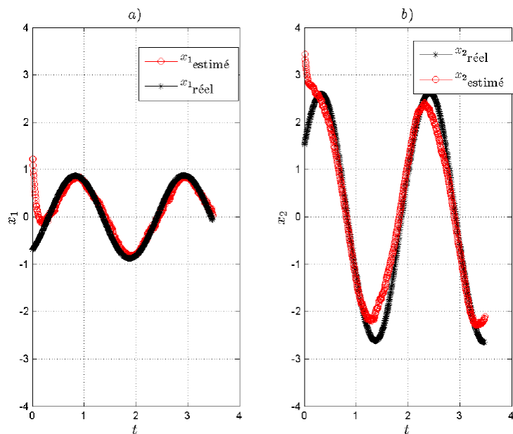
FIG. 4.17 – Comportement de l'état estimé \hat{x}_2 obtenu à l'aide de l'observateur (4.6.8) et dans la présence de bruit sur la sortie y conduisant à l'erreur relative présentée sur la figure 4.16 avec q = 0.01 .
