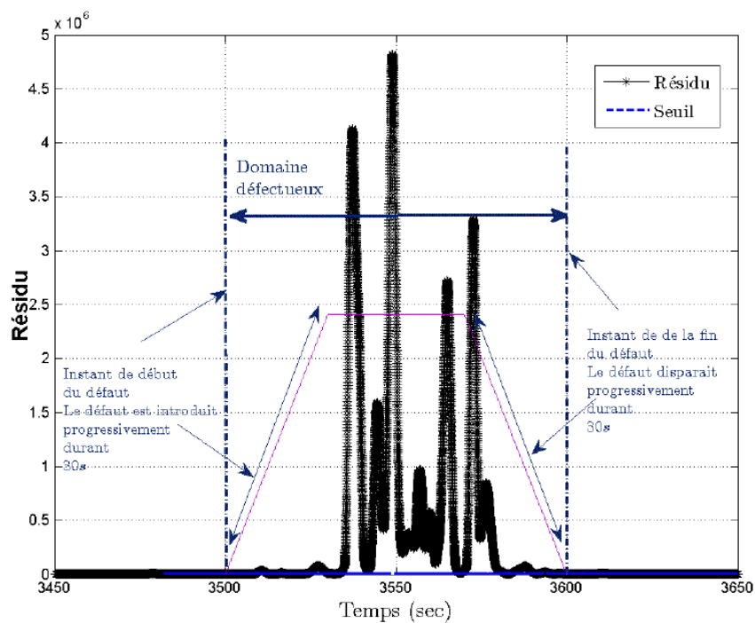
FIG. 7.10 – Résidu de détection dans le cas du défaut actionneur de type hydraulique sur \beta_3 .
