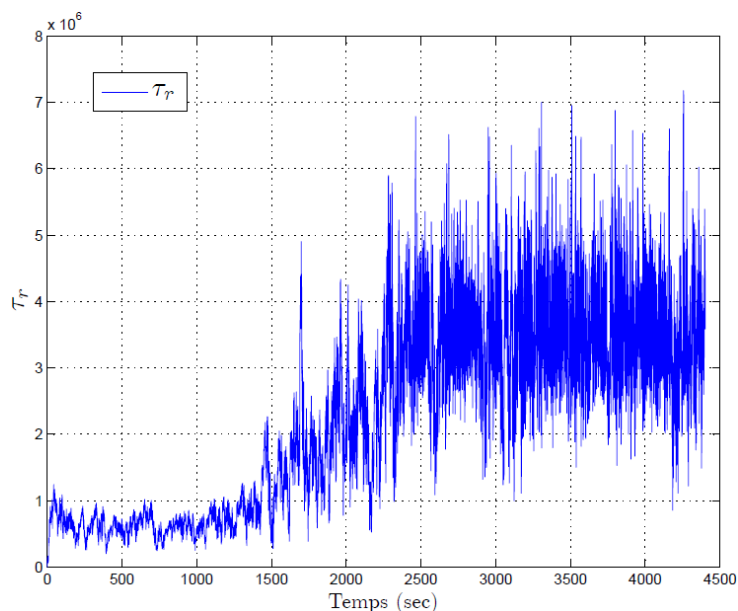
FIG. 7.15 – Estimation de l'entrée \tau_r (Cas nominal)
