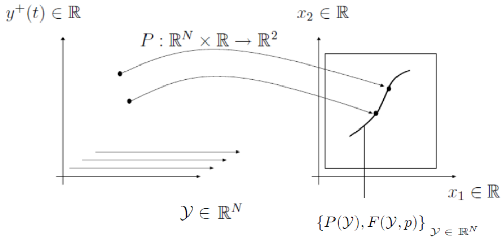
FIG. 2.2 – Signature graphique de la fonction F . A chaque couple (\mathcal{Y}(t), y^+(t)) , il est associé un point dans un plan 2D (plan de la signature). La signature 2D obtenue contient un nombre de points égal au nombre de valeurs prises par \mathcal{Y}(t) en glissant la fenêtre de longueur N sur le train de mesures considéré.
