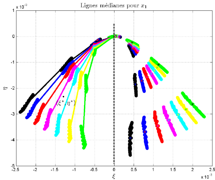
FIG. 4.23 – Lignes médianes regroupant les médianes des signatures partageant les mêmes valeurs de x_1 .
