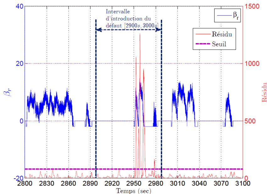
FIG. 7.9 – Résidu de détection dans le cas du défaut actionneur causé par l'augmentation de niveau d'air dans l'huile sur \beta_2
