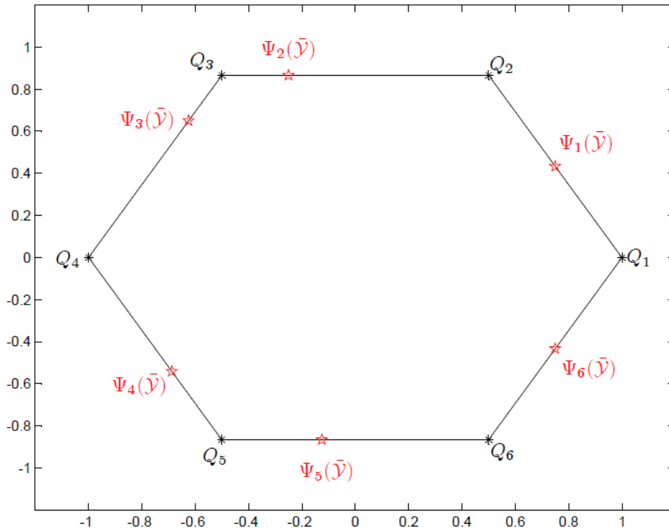
FIG. 2.6 – Définition des points Q_i et \Psi_i(\bar{\mathcal{Y}}) dans le cas N = 6 et \bar{\mathcal{Y}} = (0, 0.5, -0.5, 0.25, -0.25, 0)^T . Q_i représentent les N sommets du polygone régulier. \Psi_i(\bar{\mathcal{Y}}) est un point sur le segment Q_i Q_{i+1} placé selon la valeur de \bar{\mathcal{Y}}_i
