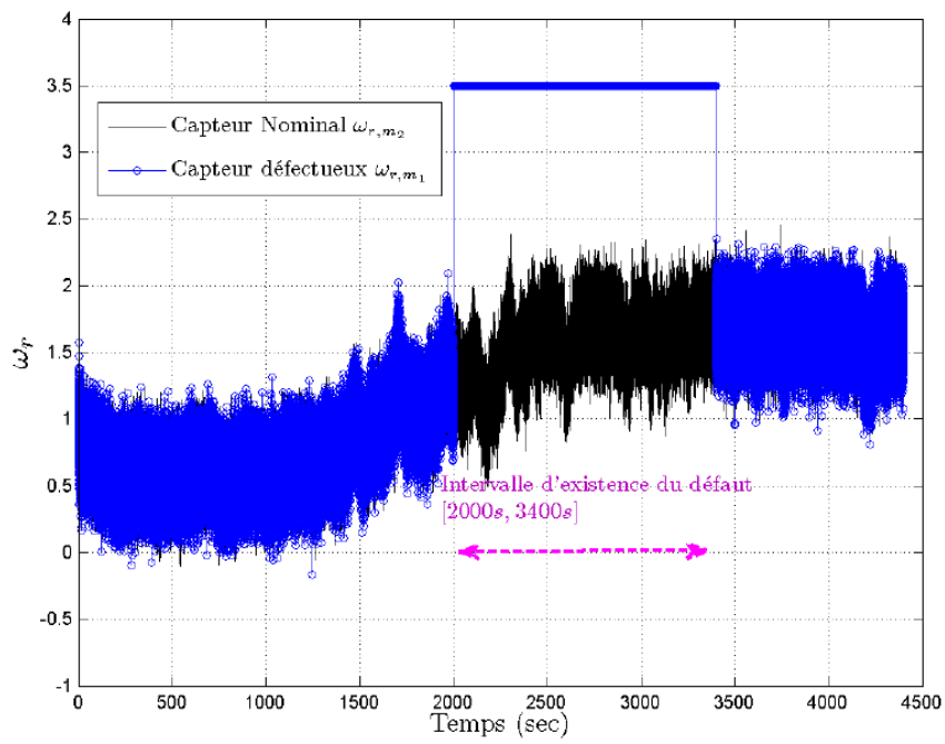
FIG. 7.17 – Les 2 signaux \omega_{r,m_2} et \omega_{r,m_1} en configuration nominale et défectueuse ( VF = 3.5 )
