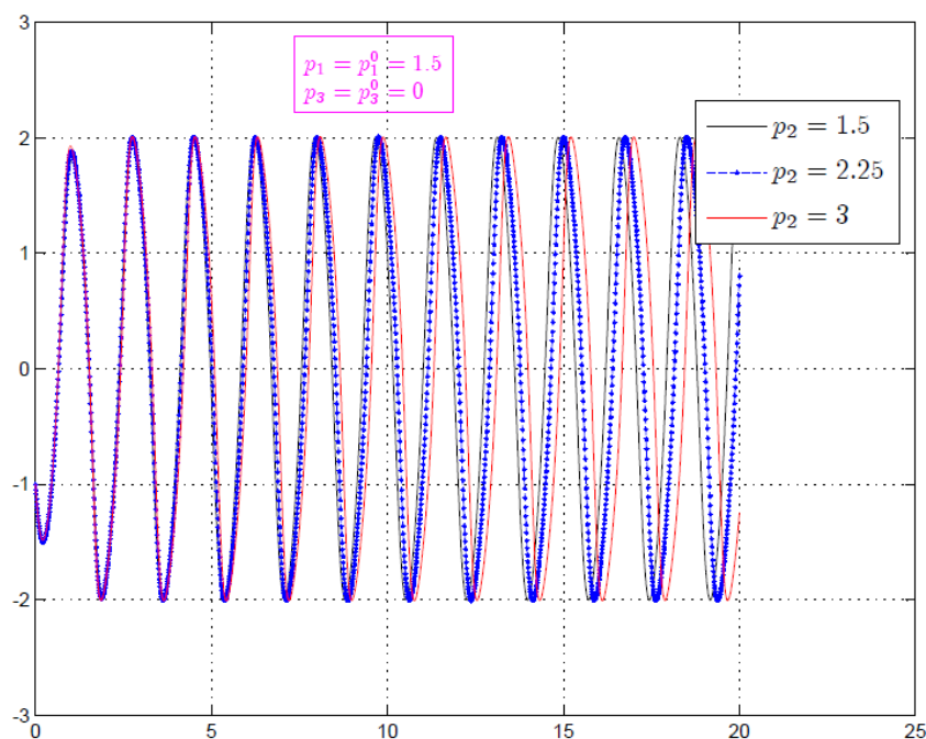
FIG. 2.13 – Sortie de l'oscillateur dans de cas des variations de p_2 , (p_1, p_3) = (1.5, 0) .
