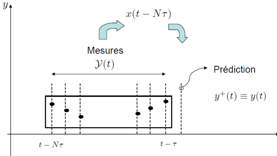
FIG. 2.1 – La connaissance de N mesures passées (vecteur \mathcal{Y}(t) ) permet la détermination de l'état observable x(t) et donc la sortie à l'instant suivant t + (N + 1)\tau est obtenue uniquement par \mathcal{Y}(t)
