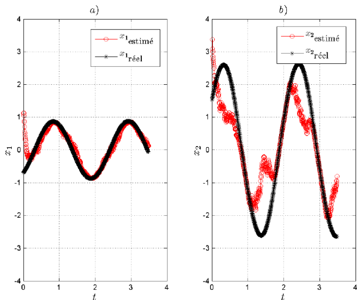
FIG. 4.15 – Comportement des états estimés \hat{x}_1 et \hat{x}_2 obtenus à l'aide de l'observateur (4.6.8) et dans la présence de bruit sur la sortie y conduisant à l'erreur relative présentée sur la figure 4.16 avec q = 0.1 .
