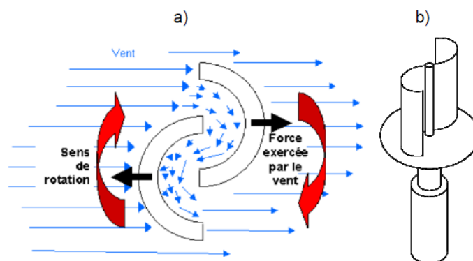
FIG. 6.6 – a) Schéma de principe du rotor de Savonius. b) Schéma du rotor de Savonius
