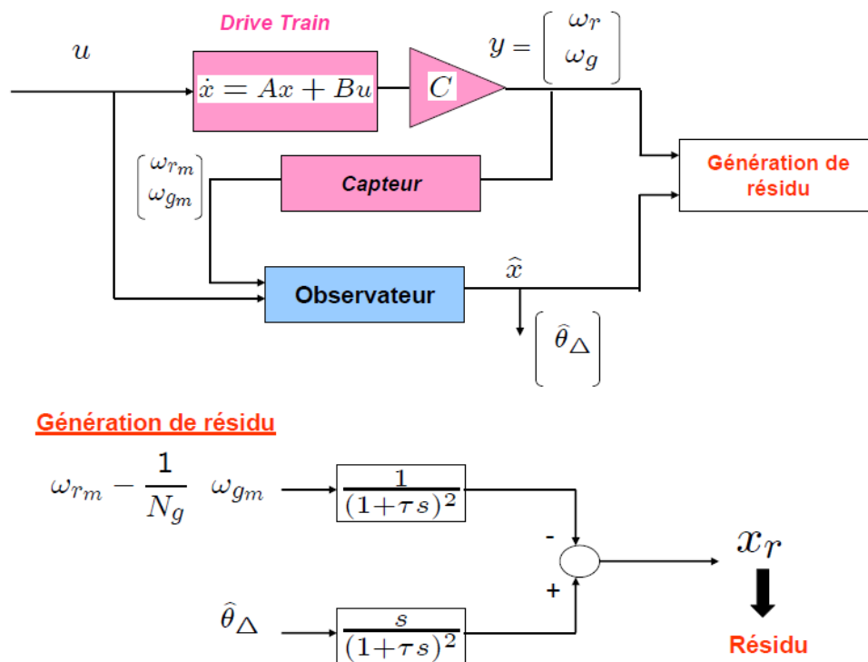
FIG. 7.14 – Schéma général proposé pour la génération des résidus dans le cas des défauts capteurs (Bloc 2)(7.1)
