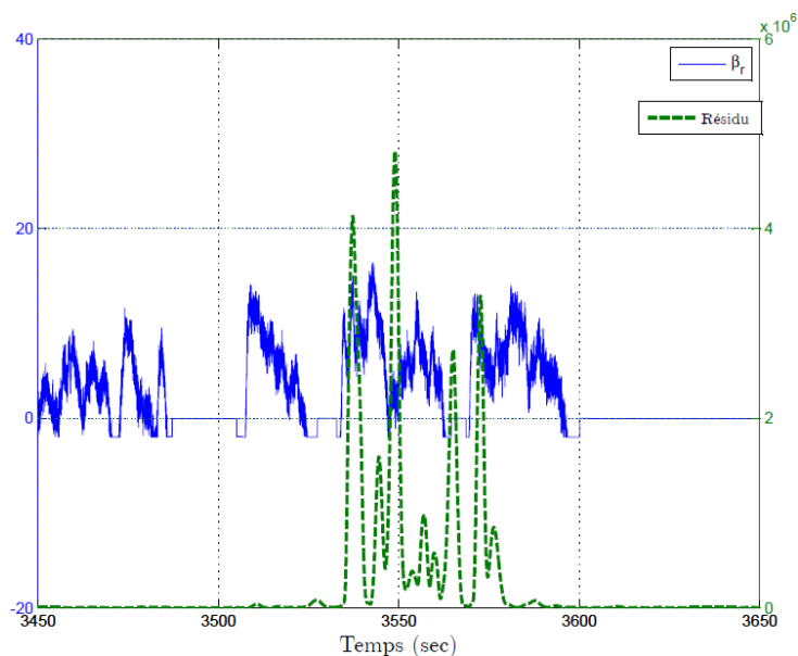
FIG. 7.11 – Dépendance du résidu obtenu dans le cas du défaut 9 par rapport au signal d'entrée \beta_{r2} .
