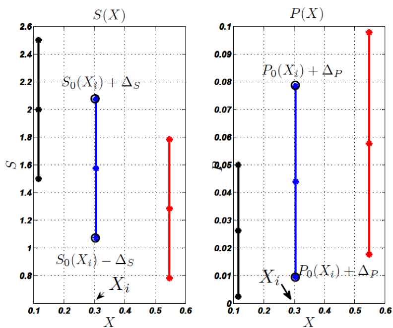
FIG. 4.27 – Exemple de la projection de l'ensemble admissible \mathbb{Z}_d^{(1)}(X) pour trois valeurs différentes de X \in \{0.11, 0.3, 0.55\}
