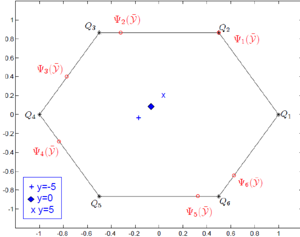
FIG. 2.7 – Définition des points P_\varepsilon(\mathcal{Y}, y) dans le cas N = 6 et \mathcal{Y} = (5, 2, 0, -1, 3, -2)^T . P_\varepsilon(\mathcal{Y}, y) se trouve sur la ligne définie par le centre de gravité des points \Psi_i(\bar{\mathcal{Y}}) et le centre de gravité de \Psi_i(\bar{\mathcal{Y}}) pondéré avec \bar{\mathcal{Y}}_i , selon la valeur de y (la sortie suivante au vecteur de mesures passées)
