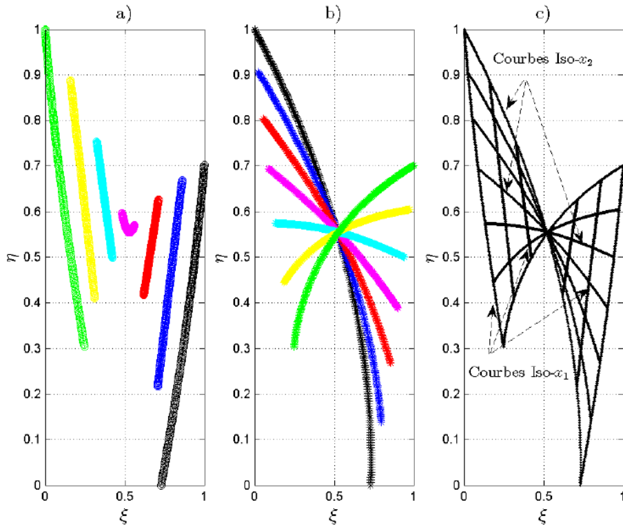
FIG. 4.12 – Vue sur la grille fine des signatures \mathcal{S}(z^{(1)}) pour z^{(1)} \in \mathbb{Z}_d^{(1)} . subplot a) regroupe toutes les signatures partageant la même valeur de x_1 en utilisant la même couleur alors que le subplot b) les regroupe en se basant sur la valeur de x_2 . subplot c) montre le système de coordonnées curvilignes qui peut être utilisé pour obtenir une formule d'estimation de x_1 et de x_2
