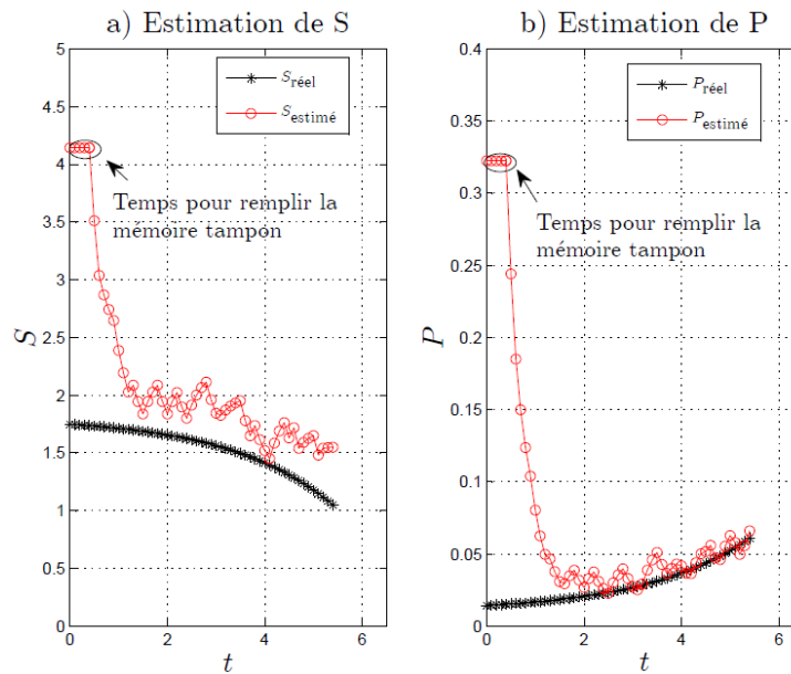
FIG. 4.30 – Comportement des états estimés \hat{S}(k) et \hat{P}(k) obtenus à laide de l'observateur (4.7.9) avec q = 0.3 et dans la présence de bruit de mesure sur les mesures X et L conduisant à l'erreur relative donnée dans les figures 4.31 et 4.32
