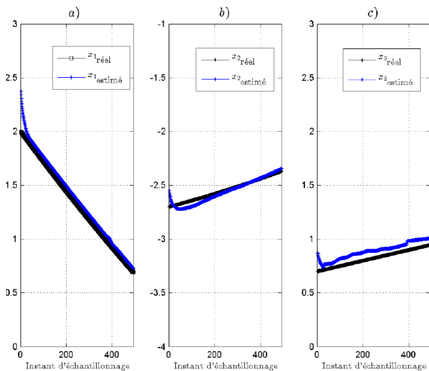
FIG. 4.25 – Exemple 2 : Estimation des trois états x_1 , x_2 et x_3 .
