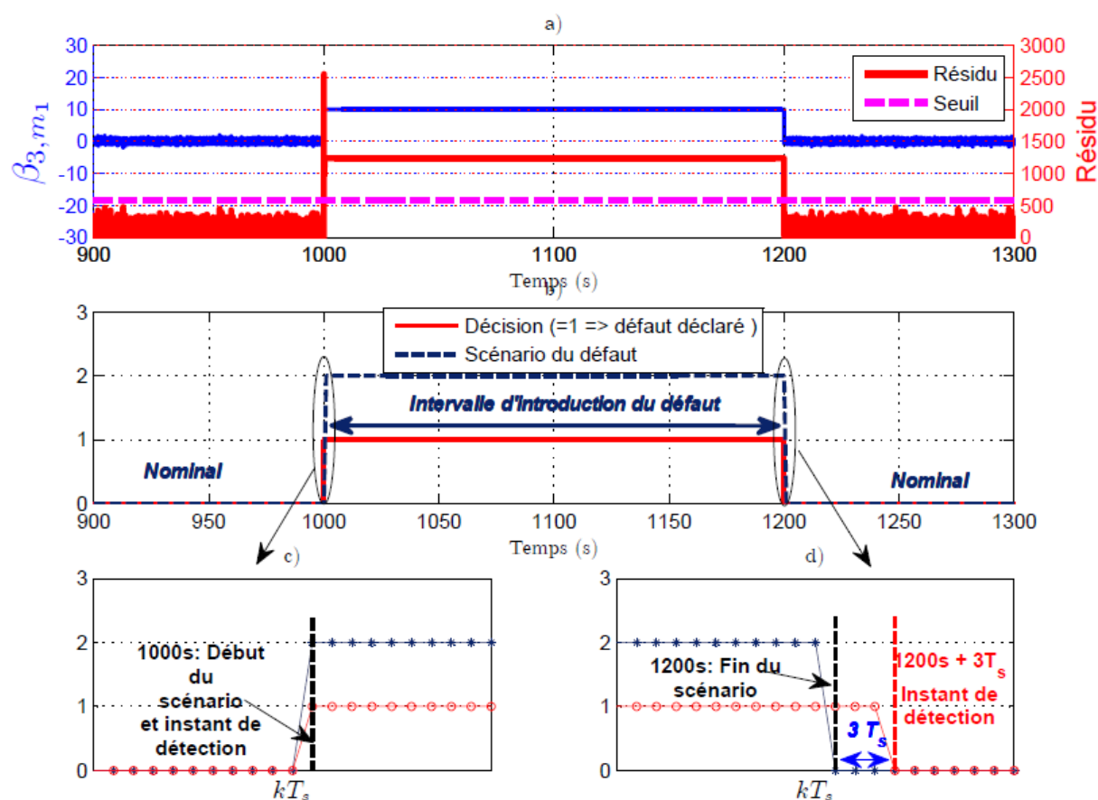
FIG. 7.5 – Résultat de détection du défaut de type VF = 10 remplaçant le signal \beta_{3,m_1} délivré par le capteur 1 mesurant l'angle de la troisième pale, \beta_3 dans l'intervalle [1000s, 1200s] . Le subplot b) donne le signal binaire qui est de valeur 1 lors de la présence du défaut. Les deux ellipses font référence au zoom effectué pour montrer la détection au début et à la fin de l'intervalle de présence du défaut, présentée resp. sur les deux subplot c) et d).
