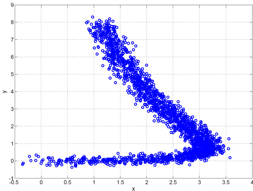
FIG. 4.2 – Exemple d'une signature pour laquelle toute enveloppe convexe ne conviendrait pas.
