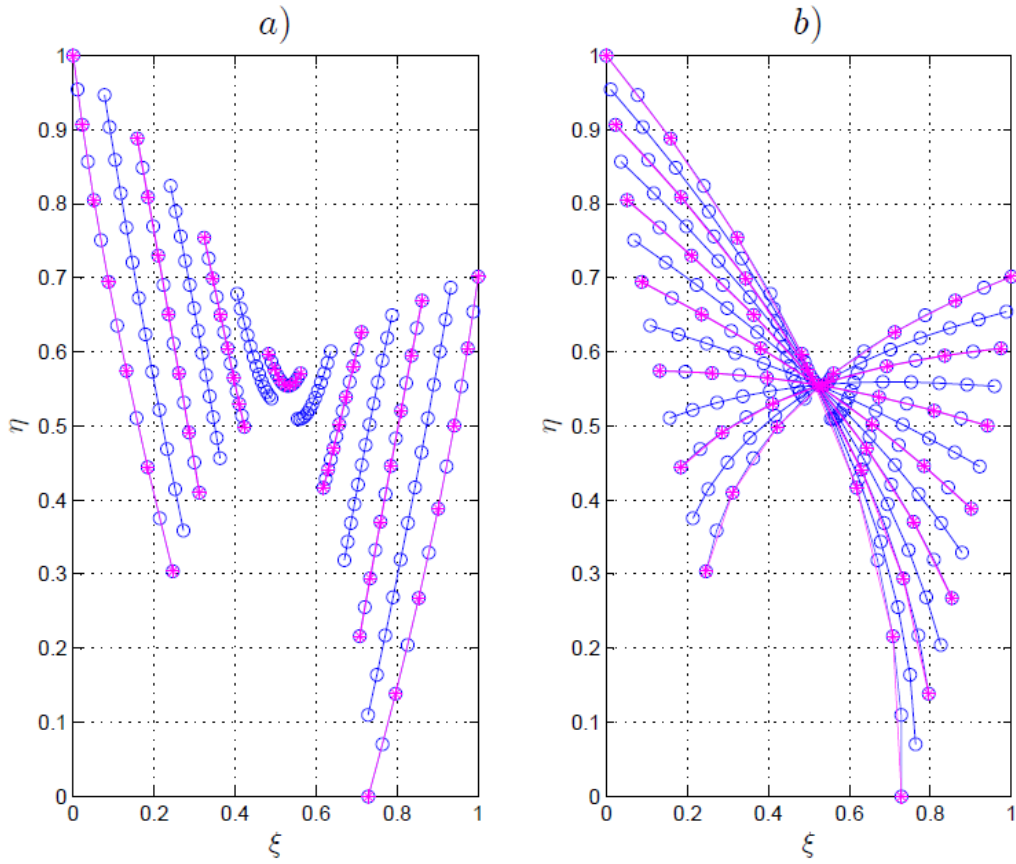
FIG. 4.11 – Vue sur la grille fine des signatures \mathcal{S}(z^{(1)}) pour z^{(1)} \in \mathbb{Z}_d^{(1)} . subplot a) regroupe toutes les signatures classifiées selon la valeur de x_1 alors que le subplot b) les regroupe en se basant sur la valeur de x_2 . subplot c) montre le système de coordonnées curvilignes qui peut être utilisé pour obtenir une formule d'estimation de x_1 et de x_2 .
