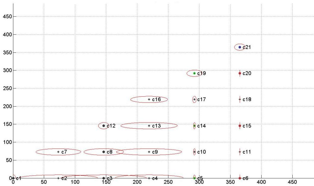
FIG. 3.7 – Vue de l'erreur d'estimation lorsque les lois d'estimation (3.5.5) et (3.5.7) sont appliquées à l'ensemble complet des données expérimentales. Rappelons que la phase d'apprentissage utilise seulement 11 des 21 points où la sonde a été positionnée et les données mesurées sont acquises. On notera en particulier que les points \{2, 7, 4, 9, 13, 16, 10, 17, 11, 18\} ne sont pas utilisés dans la phase d'apprentissage.
