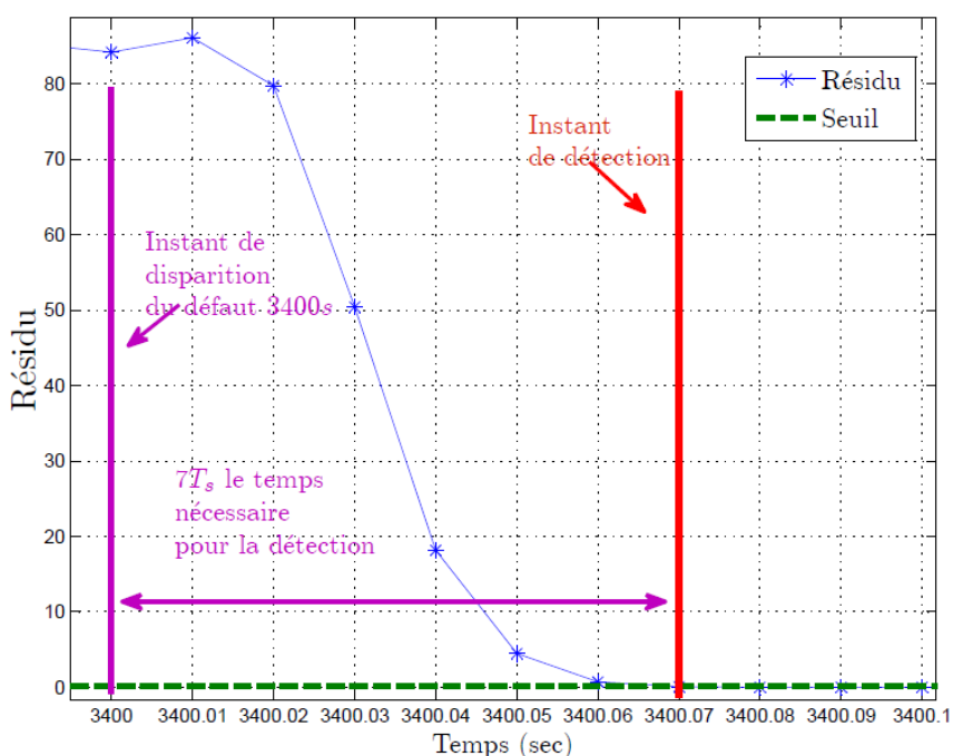
FIG. 7.24 – Résidu de détection dans le cas du défaut FG = 5 sur \omega_{r,m_2} . Zoom sur la détection vers la fin du défaut
