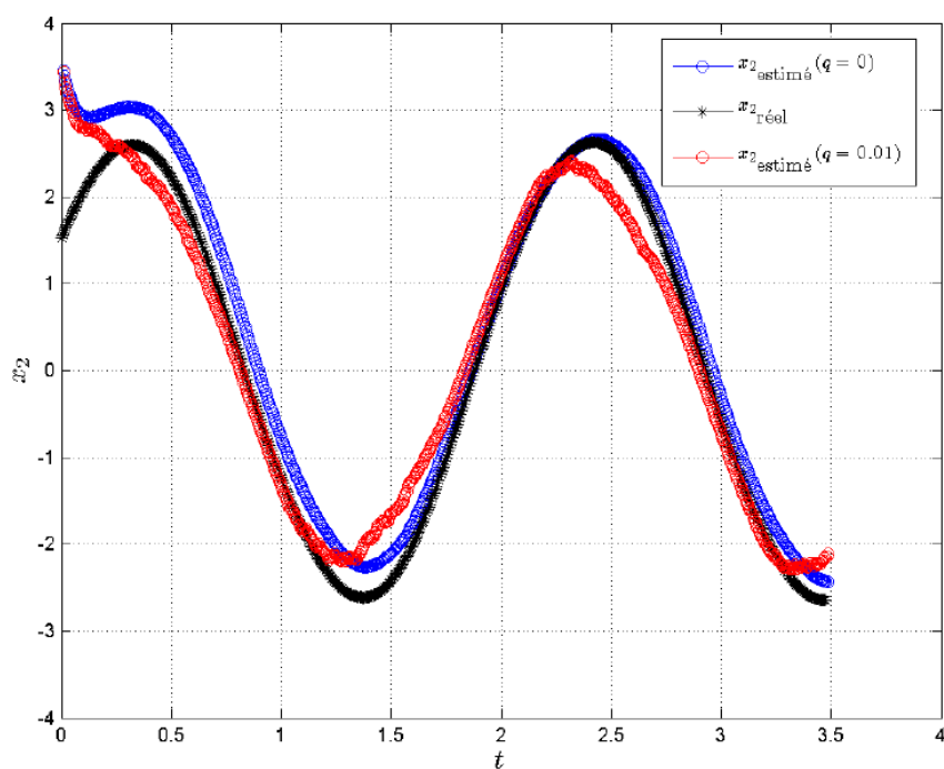
FIG. 4.18 – Comparaison avec l'estimation boucle ouverte de x_2 ( q = 0 ).
