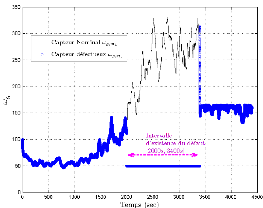
FIG. 7.25 – Les 2 signaux \omega_{g,m_2} et \omega_{g,m_1} en configuration nominale et défectueuse ( VF = 50 )
