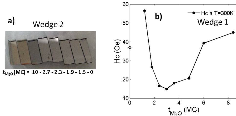
FIGURE 19.3 – a) Photographie du wedge 2 Cr/MgO/Fe et épaisseur de MgO dans chaque tricouche ( t_{\text{MgO}} ). b) Evolution du champ coercitif des couches de Fe avec l'épaisseur du MgO dans le wedge 1.
