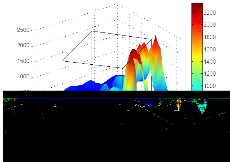
FIGURE 1.2.1: Géométrie de la topographie. L'échelle verticale est en mètres. Le parallépipède indique la zone du modèle.
