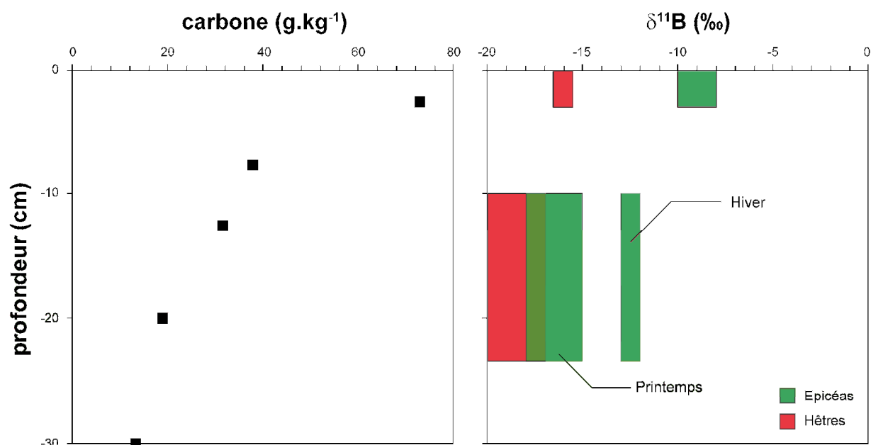
Figure VI-3 : évolution de la teneur en carbone du sol en fonction de la profondeur (profil de référence) (Mareschal, 2008) par rapport à l'évolution de la composition isotopique du bore pour les deux profondeurs étudiées.
