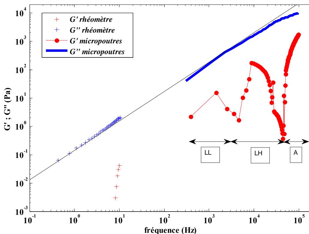
Figure 18 - G' et G'' mesurés au rhéomètre (+) puis calculés après calibration dans les trois plages de fréquences des micropoutres de type LL, LH et A (- et o) immergées dans de l'huile silicone de viscosité 20 cP.
